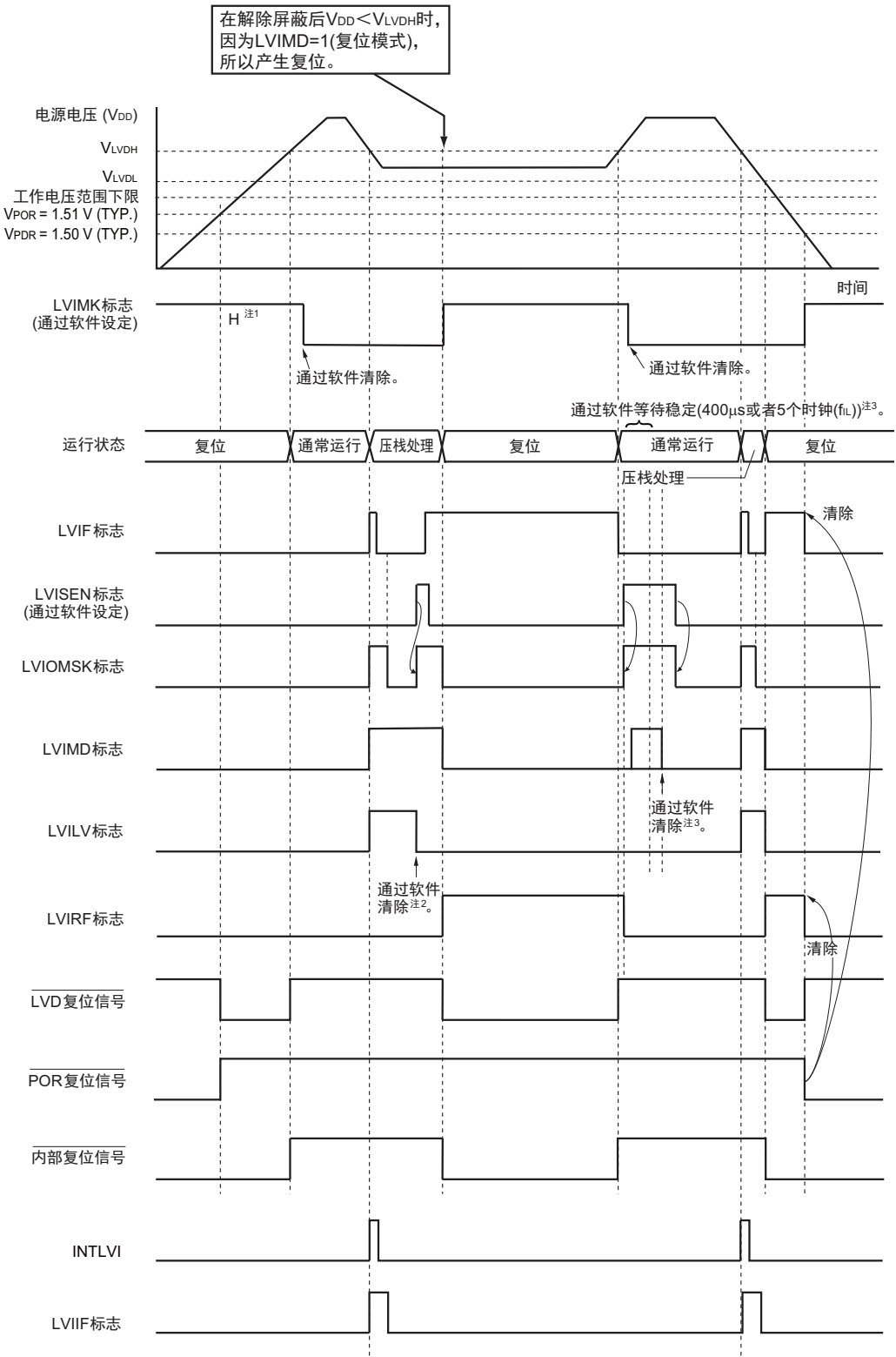
图 19-6 中断 & 复位信号的发生时序（选项字节的 LVIMDS1、LVIMDS0=1、0）(2/2)
