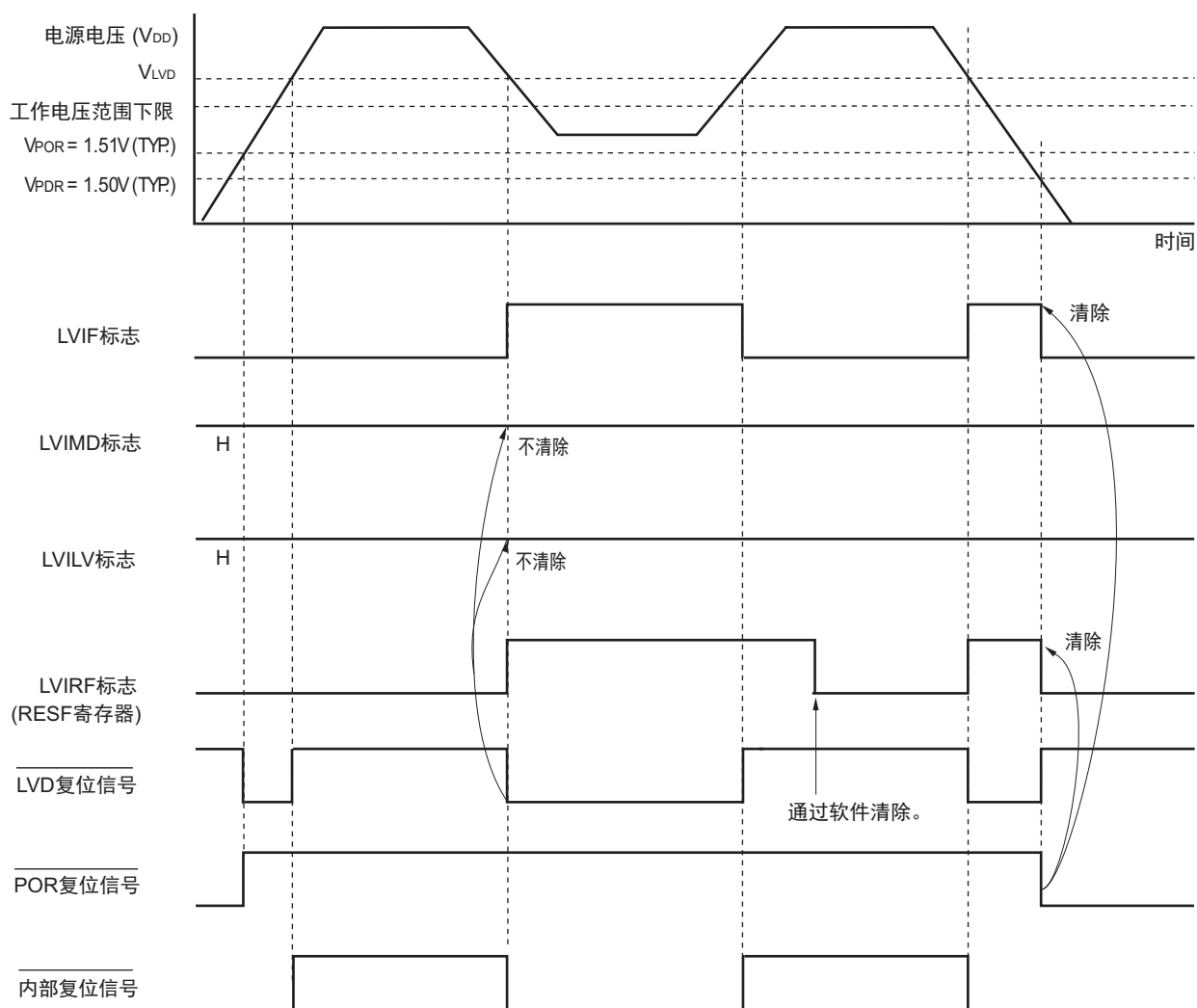
图 19-4 内部复位信号的产生时序（选项字节的 LVIMDS1、LVIMDS0=1、1）
