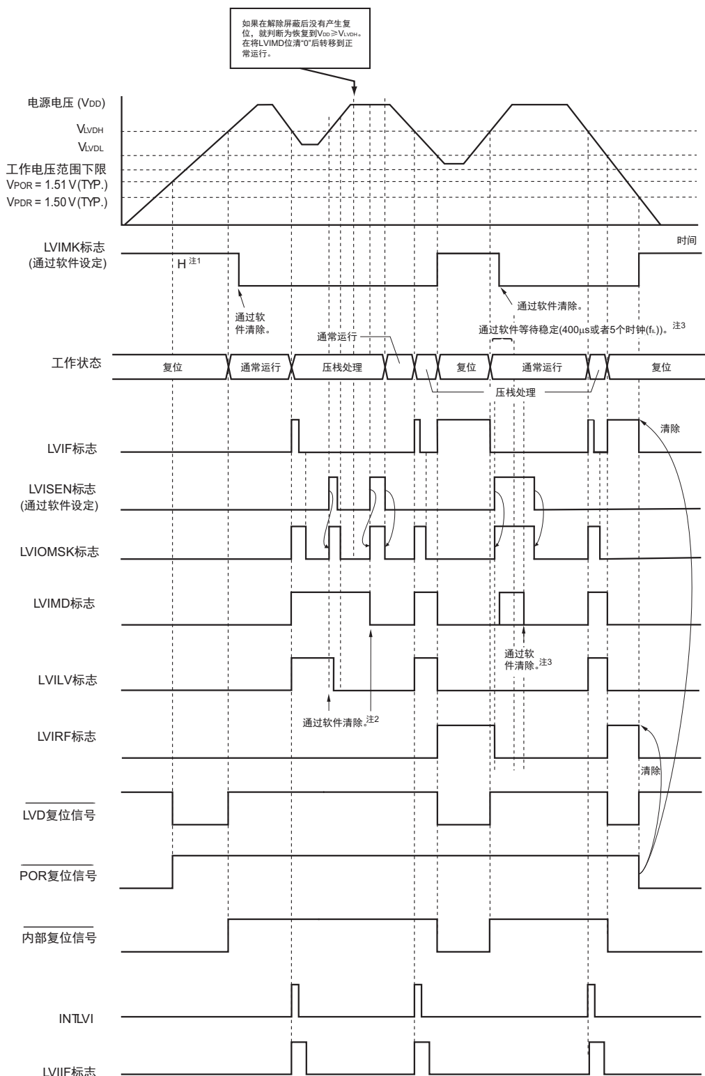
图 19-6 复位 & 中断信号的发生时序 (选项字节的 LVIMDS1、LVIMDS0=1、0) (1/2)
