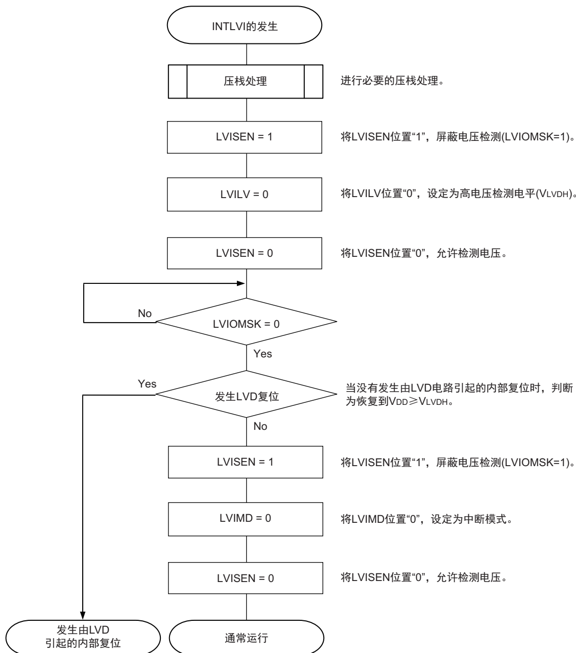
图 19-7 工作电压的确认 / 复位的设定步骤
