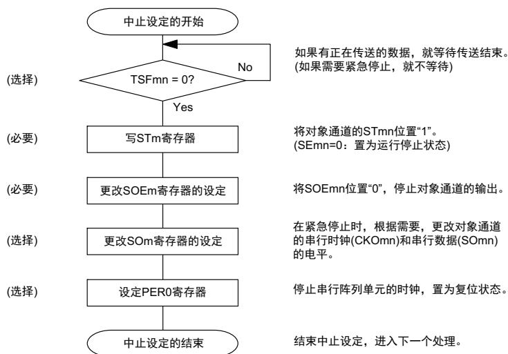
图 12-40 主控发送和接收的中止步骤
