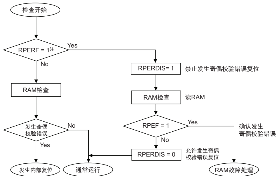
图 20-8 RAM 奇偶校验检查的流程图
