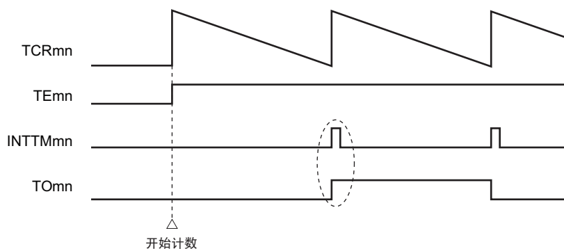
图 6-40 MDmn0 位为“0”的情况
