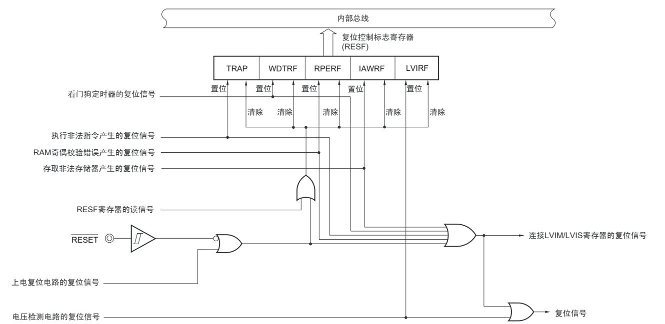
图 17-1 复位功能的框图
