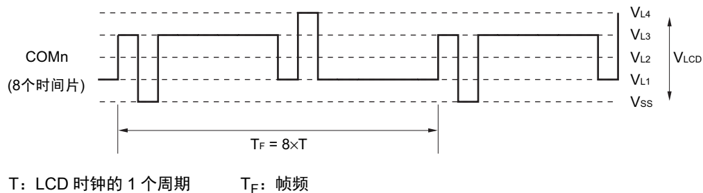
(d) 1/4 偏压法
