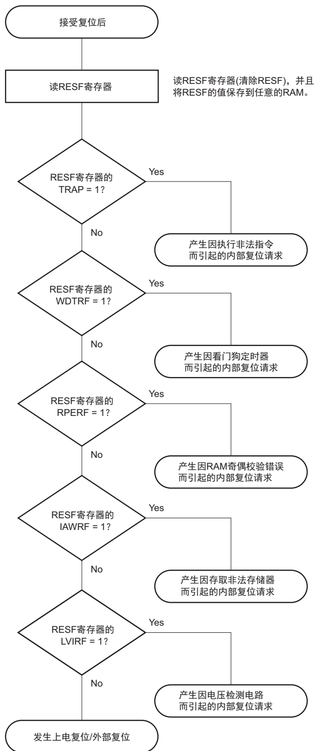
图 17-5 复位源的确认步骤
