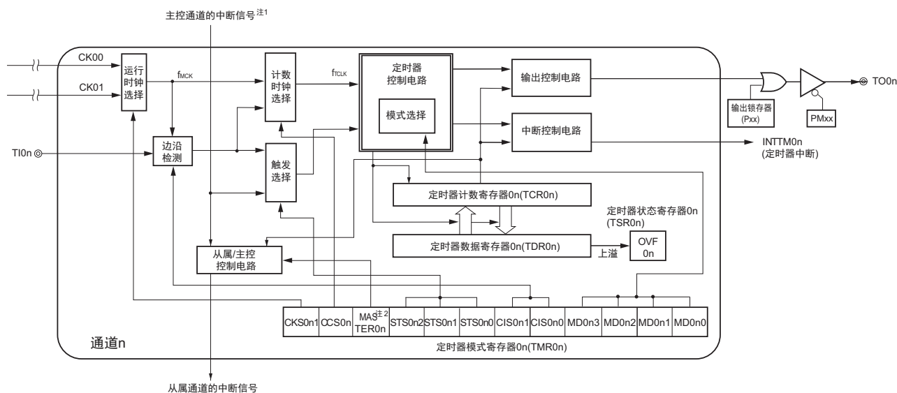
图 6-2 定时器阵列单元的通道 0、2、6 的内部框图
