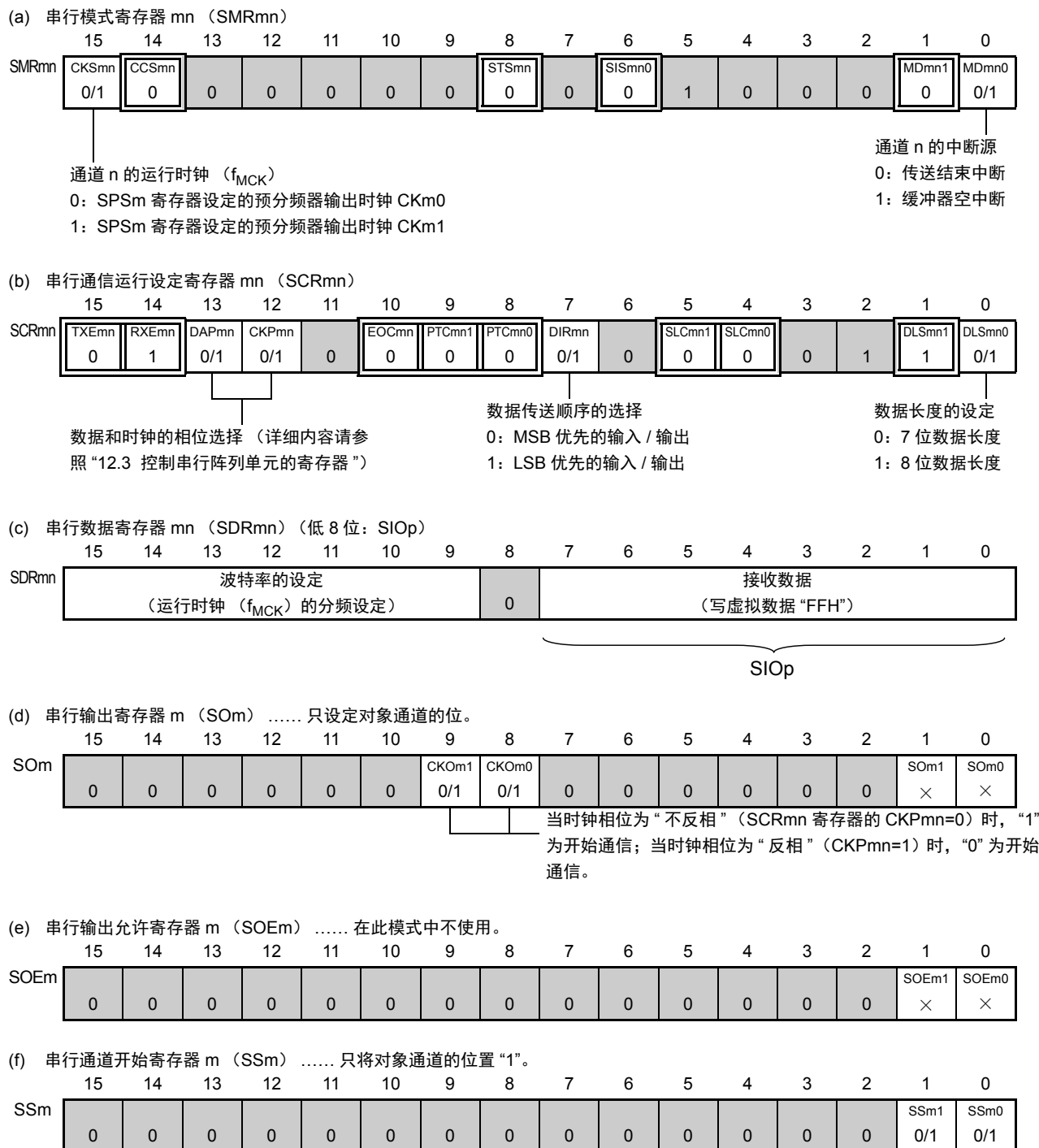
图 12-30 3 线串行 I/O (CSI00、CSI01) 主控接收时的寄存器设定内容例子
