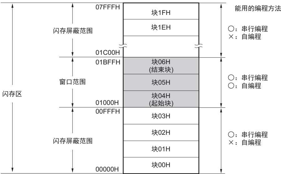
图 23-9 闪存屏蔽窗口的设定例子 (对象器件: R7F0C002G、R7F0C002L, 起始块: 04H, 结束块: 06H)
