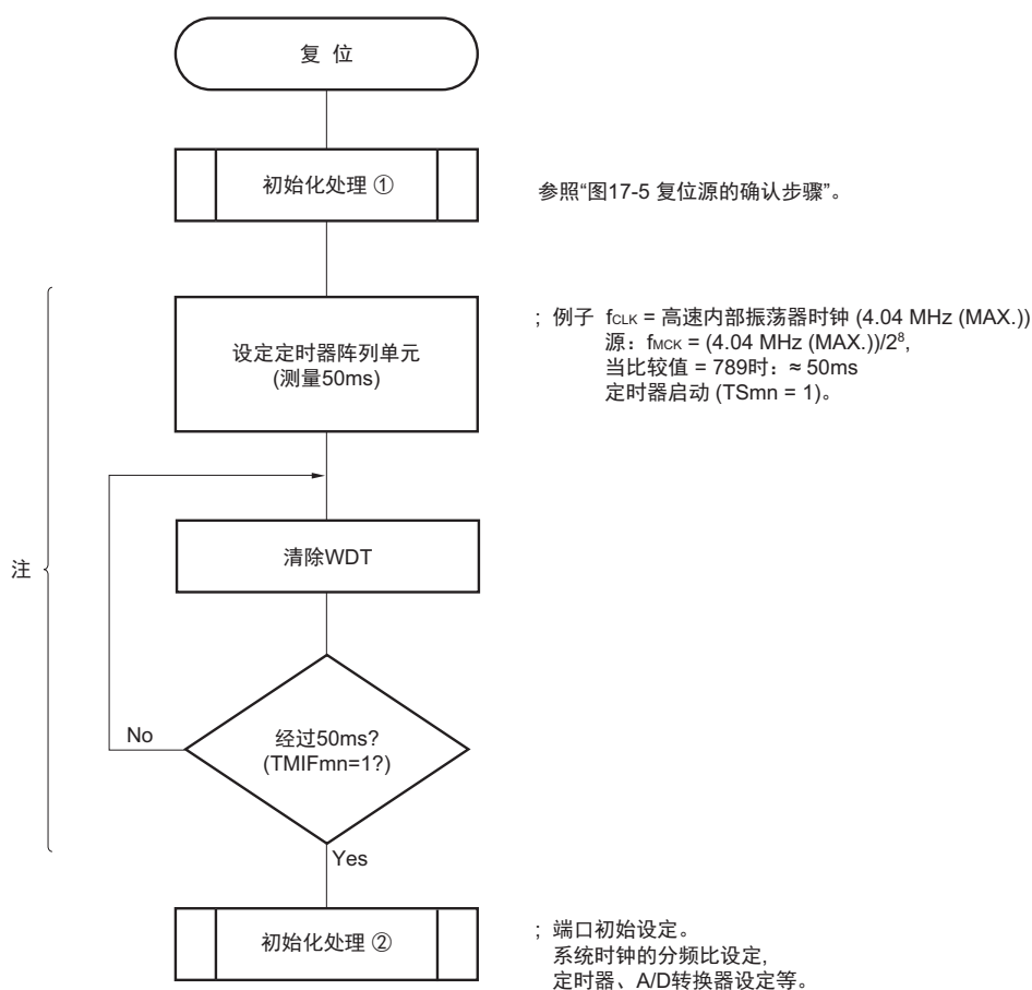
图 19-9 当 LVD 检测电压附近的电源电压波动不超过 50ms 时的软件处理例子
