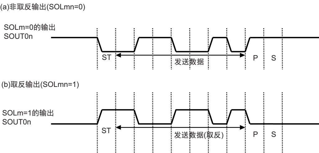
图 12-16 发送数据的电平取反例子
