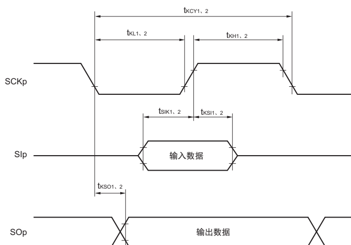
CSI 模式的串行传送时序 (同电位的通信) (DAPmn=0、CKPmn=0 或者 DAPmn=1、CKPmn=1 的情况)
