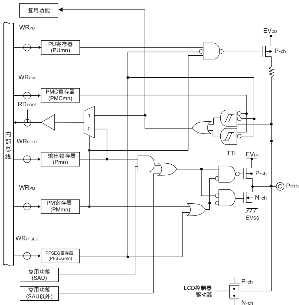
图 2-10 引脚类型 8-5-1 的引脚框图
