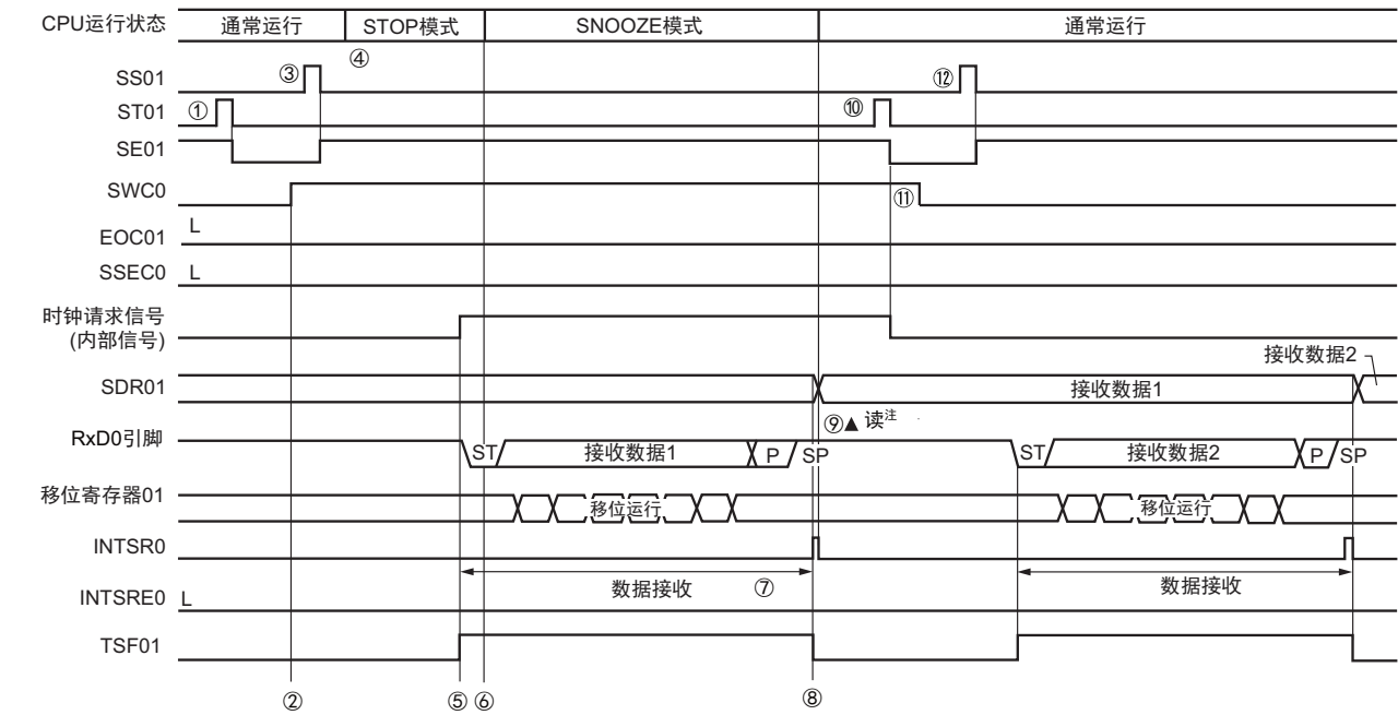
图 12-87 SNOOZE 模式运行（EOCm1=0、SSECm=0/1）的时序图
