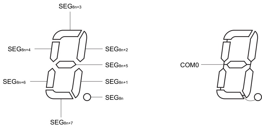
图 13-27 静态 LCD 的显示图形和电极连线
