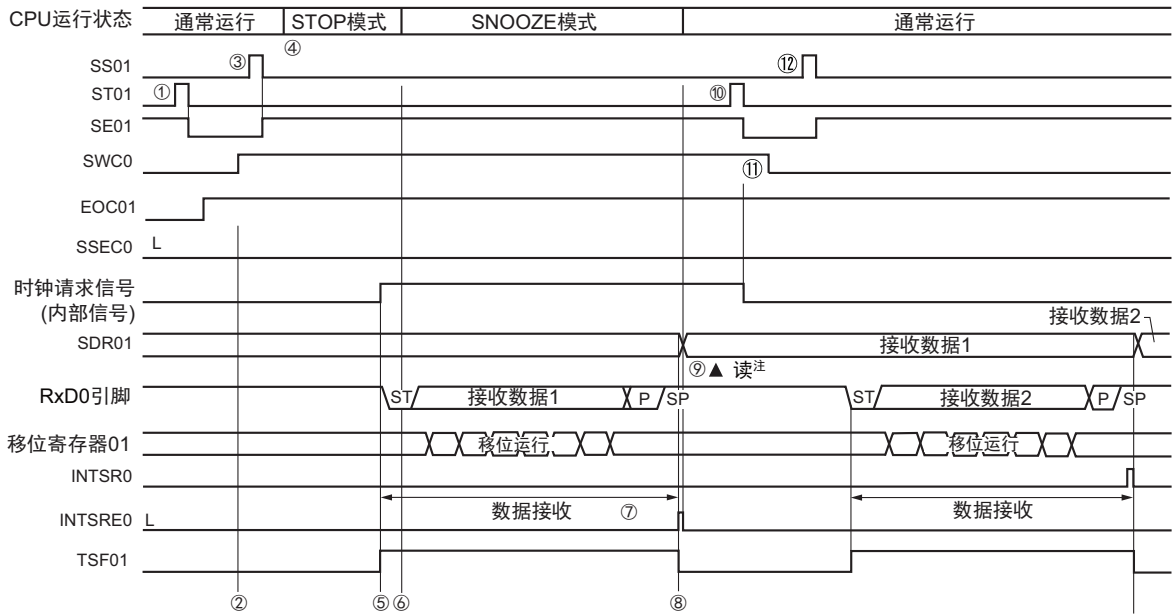
图 12-88 SNOOZE 模式运行 (EOCm1=1、SSECm=0) 的时序图
