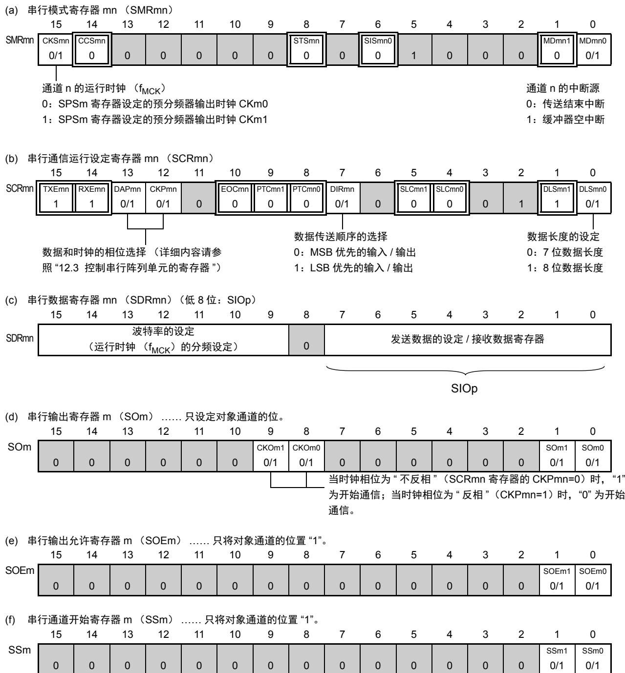
图 12-38 3 线串行 I/O (CSI00、CSI01) 主控发送和接收时的寄存器设定内容例子
