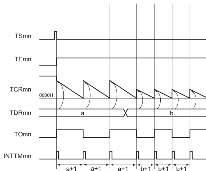
图 6-44 作为间隔定时器 / 方波输出运行的基本时序例子 (MDmn0=1)
