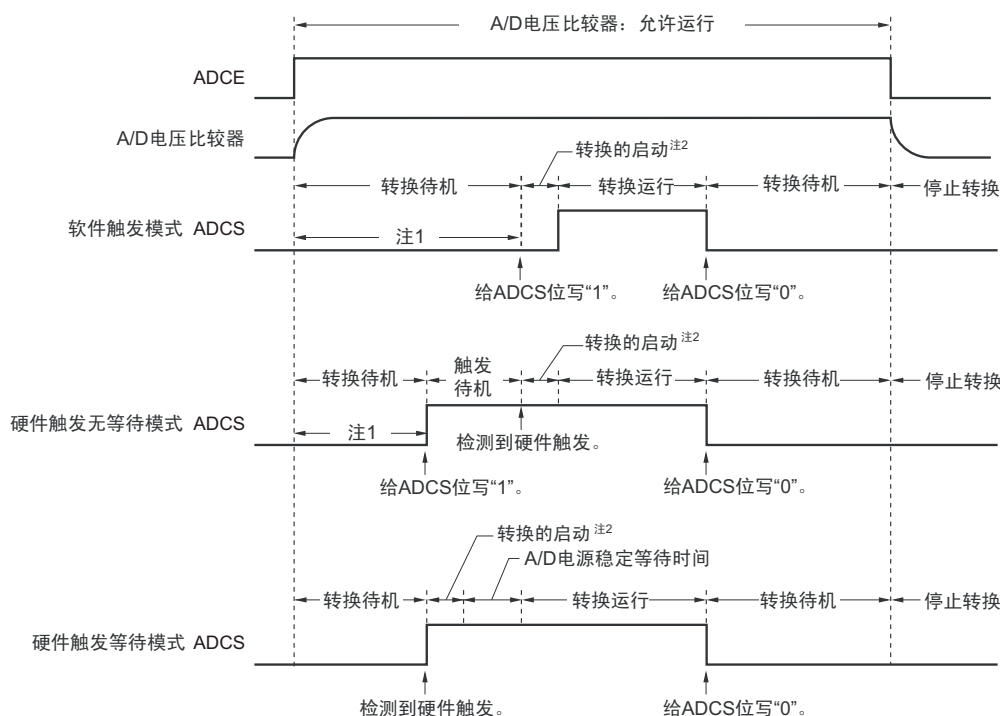
图 11-4 使用 A/D 电压比较器时的时序图
