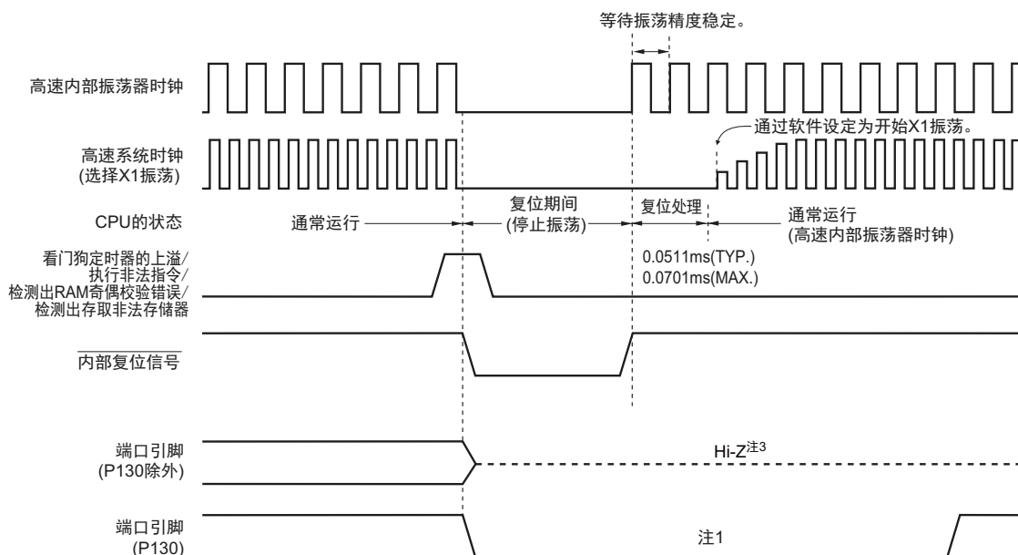
图 17-3 因执行非法指令 / 看门狗定时器的上溢 / RAM 奇偶校验错误 / 存取非法存储器而引起的复位的时序
