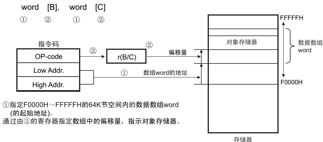
图 3-27 word[BC] 的例子
