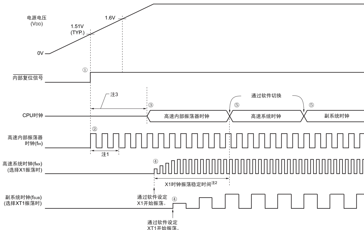
图 5-13 接通电源时的时钟发生电路的运行
