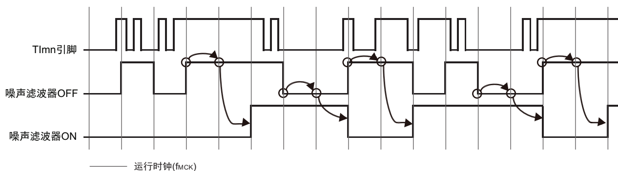
图 6-42 TImn 输入引脚的噪声滤波器 ON/OFF 时的采样波形
