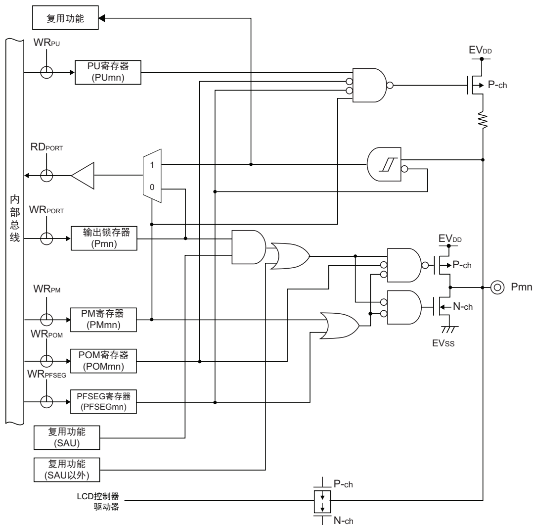
图 2-8 引脚类型 7-5-7 的引脚框图
