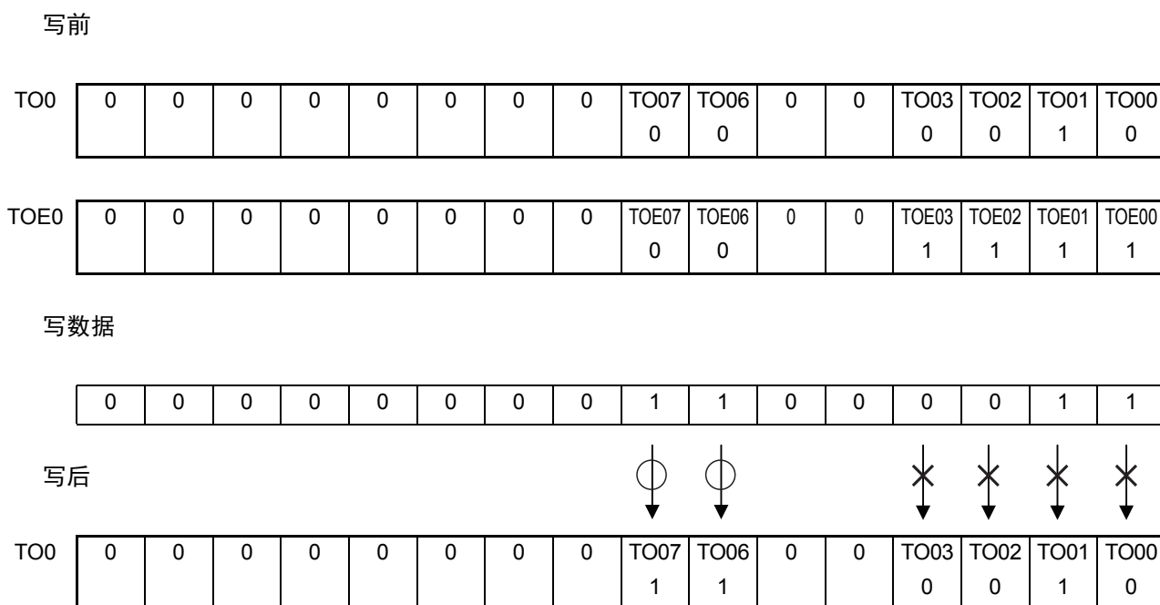
图 6-37 TO 0_n 位的一次性操作例子
