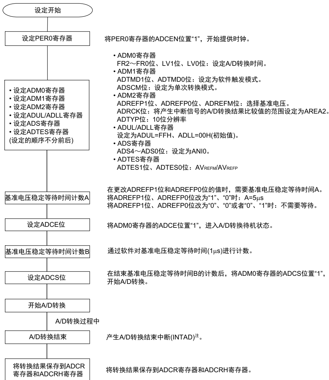
图 11-27 测试触发模式的设定
