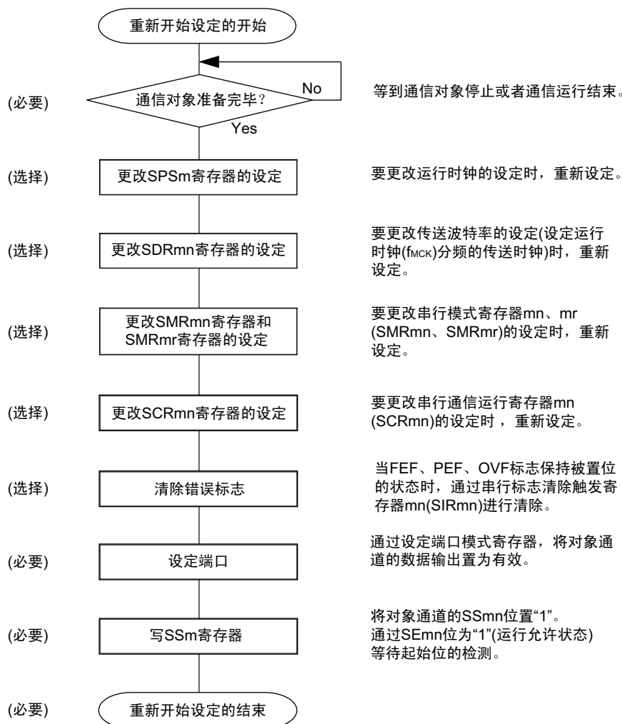
图 12-84 UART 接收的重新开始设定步骤
