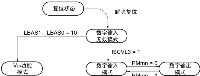
图 13-9 V L3 /P125 引脚功能的状态转移图
