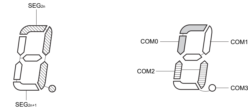
图 13-37 4 个时间片的 LCD 显示图形和电极连线
