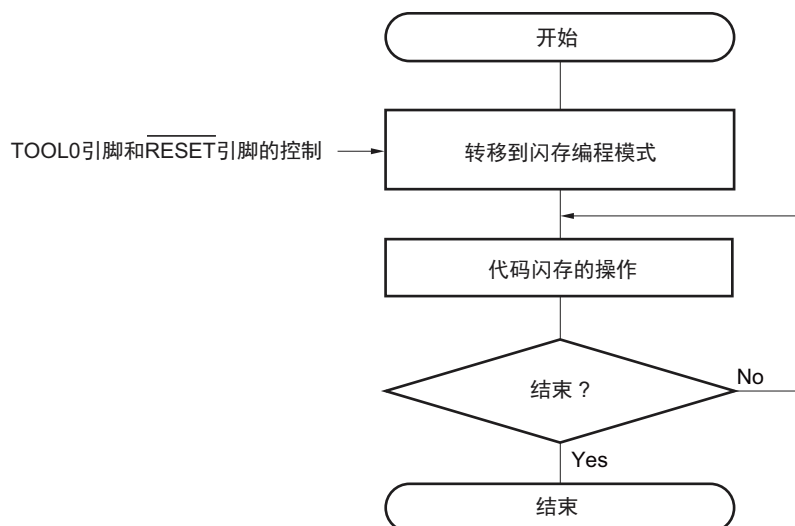
图 23-6 代码闪存的操作步骤
