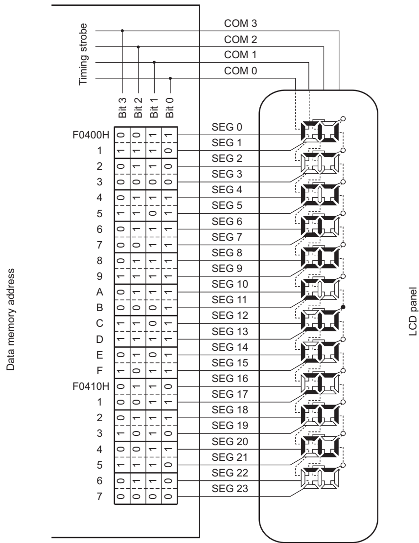
图 13-38 4 个时间片的 LCD 显示屏的连线例子
