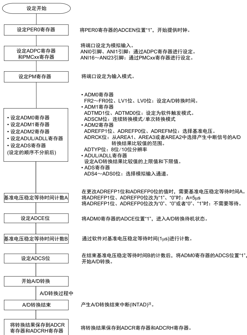
图 11-23 软件触发模式的设定
