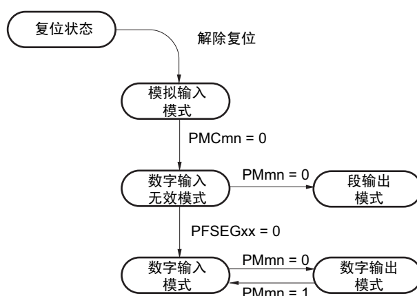
图 13-13 ANLxx/SEGxx/ 端口引脚功能的状态转移图
