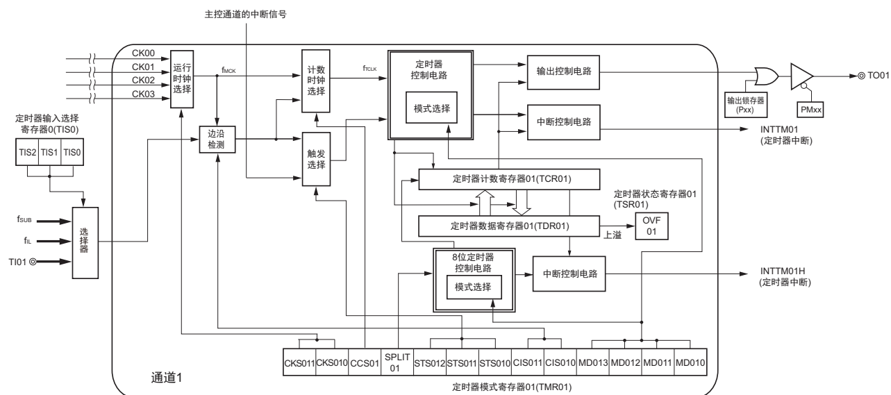
图 6-3 定时器阵列单元的通道 1 的内部框图
