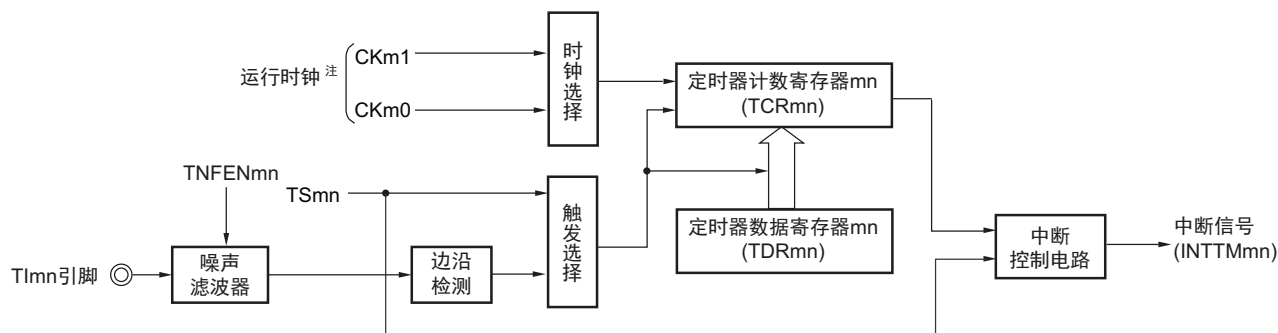
图 6-63 作为延迟计数器运行的框图
