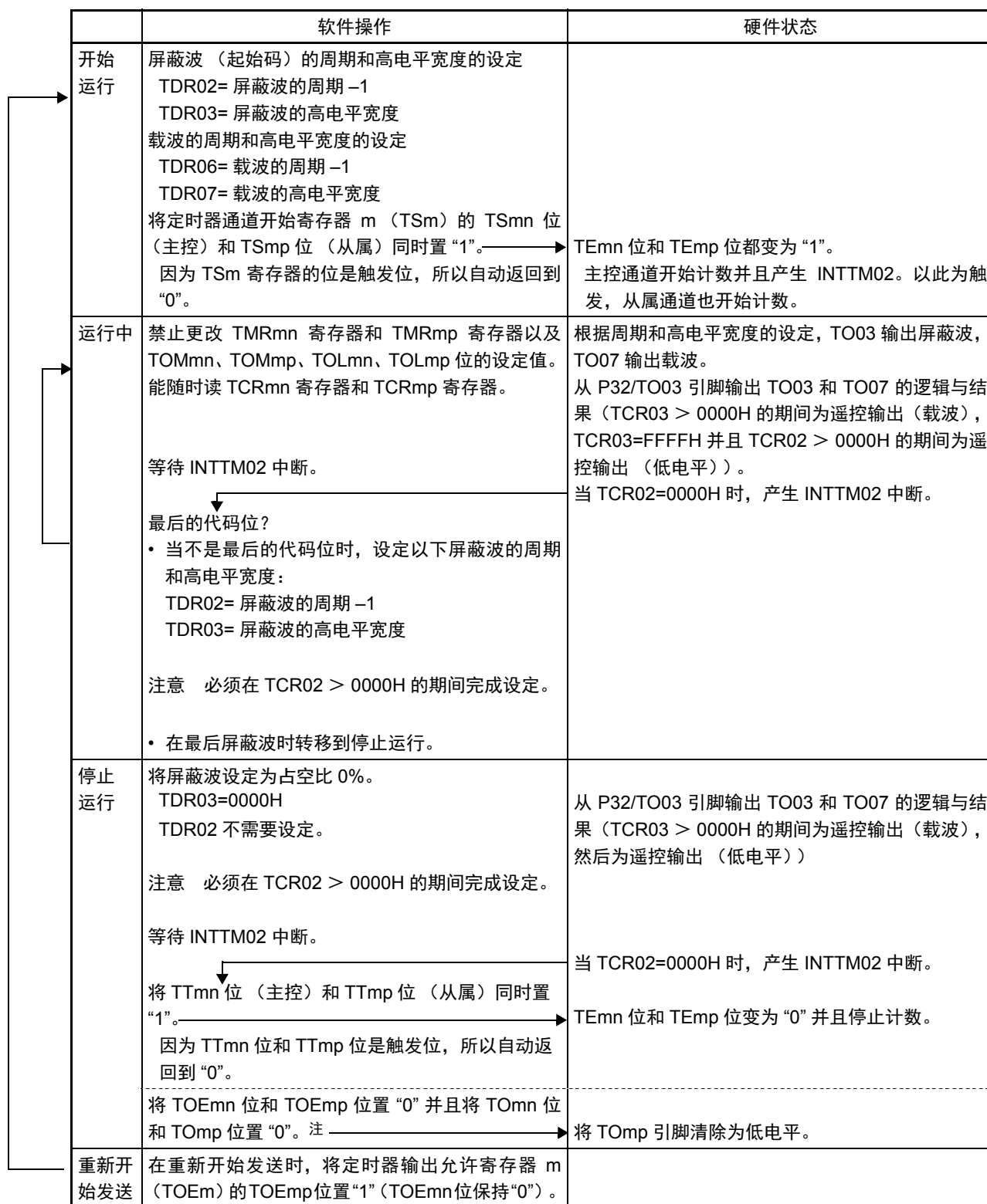
图 6-83 遥控输出功能的设定步骤 (2/2)
