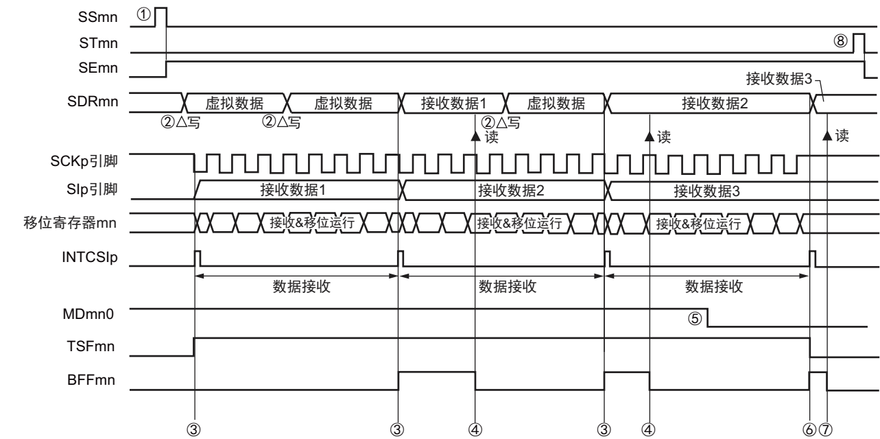
图 12-36 主控接收（连续接收模式）的时序图（类型 1：DAPmn=0、CKPmn=0）
