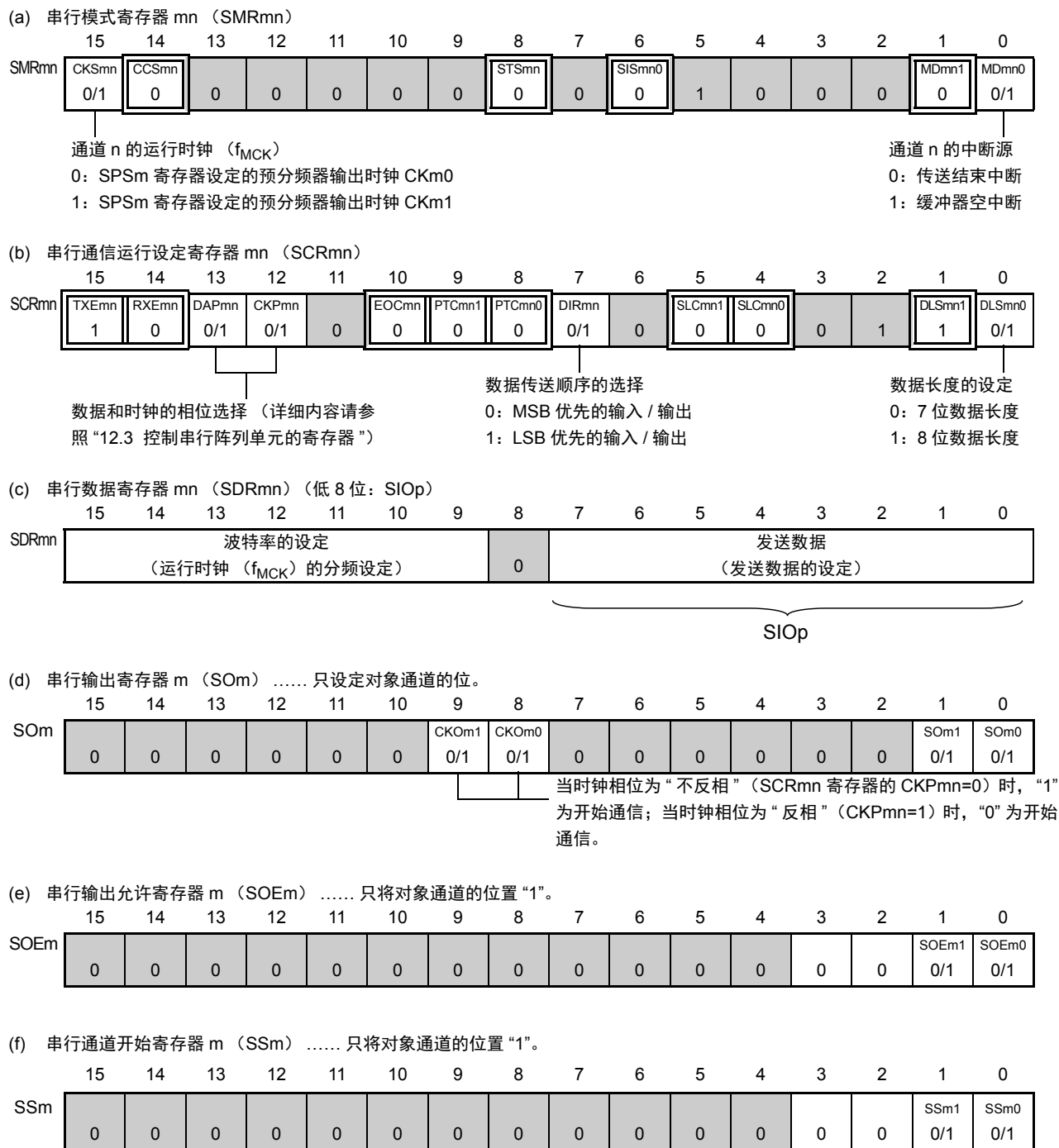
图 12-22 3 线串行 I/O (CSI00、CSI01) 主控发送时的寄存器设定内容例子
