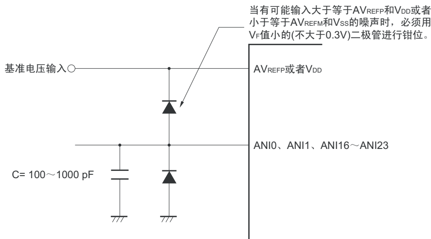
图 11-38 模拟输入引脚的处理
