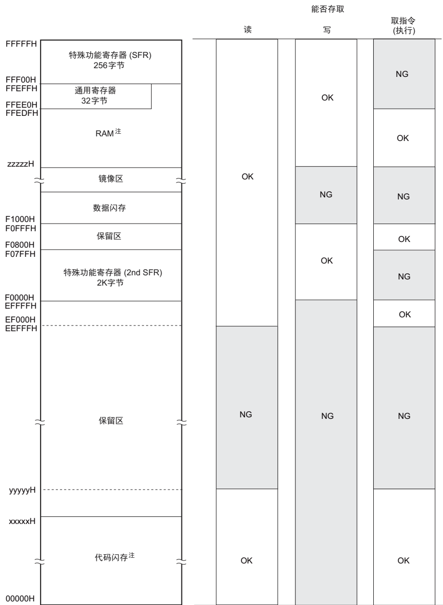
图 20-11 非法存取检测空间
