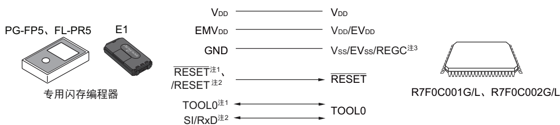
图 23-2 和专用闪存编程器的通信
