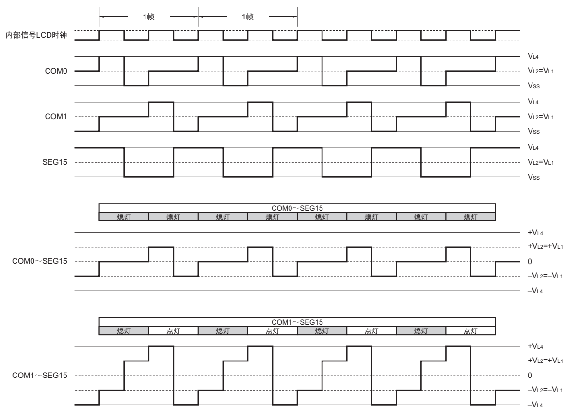
图 13-32 SEG15 和各公共信号之间的 2 个时间片的 LCD 驱动波形例子 (1/2 偏压法)
