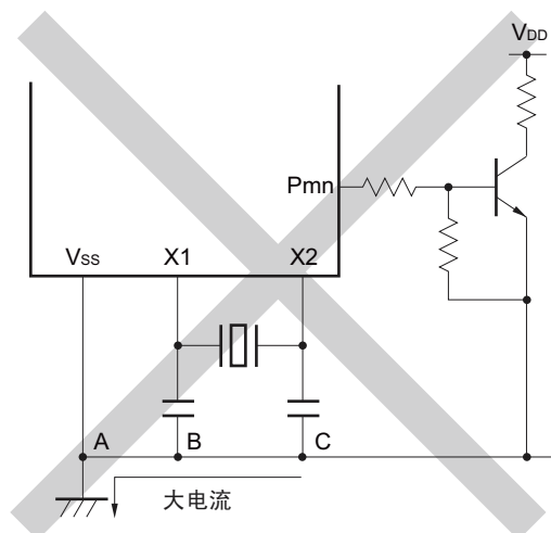
(f) 振荡电路的接地线上方有电流流过 (A 点、B 点、C 点的电位发生变动)
