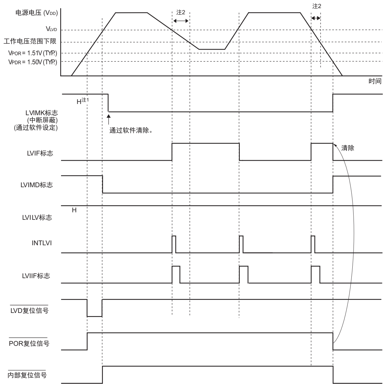
图 19-5 中断信号的产生时序（选项字节的 LVIMDS1、LVIMDS0=0、1）
