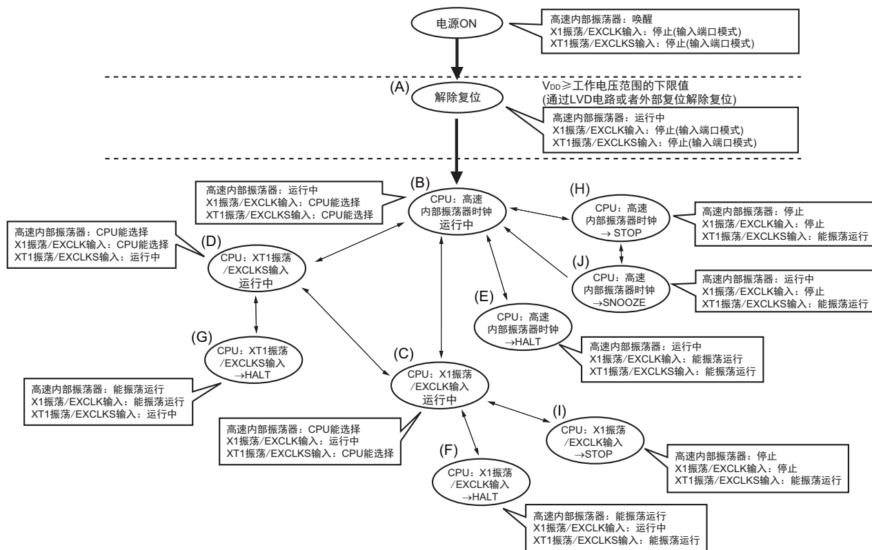
图 5-14 CPU 时钟的状态转移图
