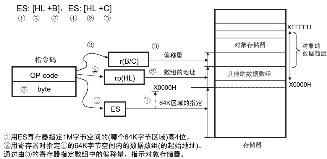
图 3-32 ES:[HL+B]、ES:[HL+C] 的例子
