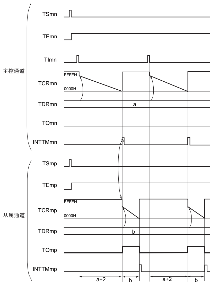
图 6-66 作为单发脉冲输出功能的运行基本时序例子
