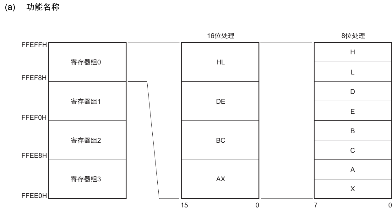
图 3-10 通用寄存器的结构
