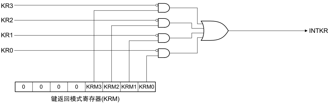
图 17-1 键中断的框图
