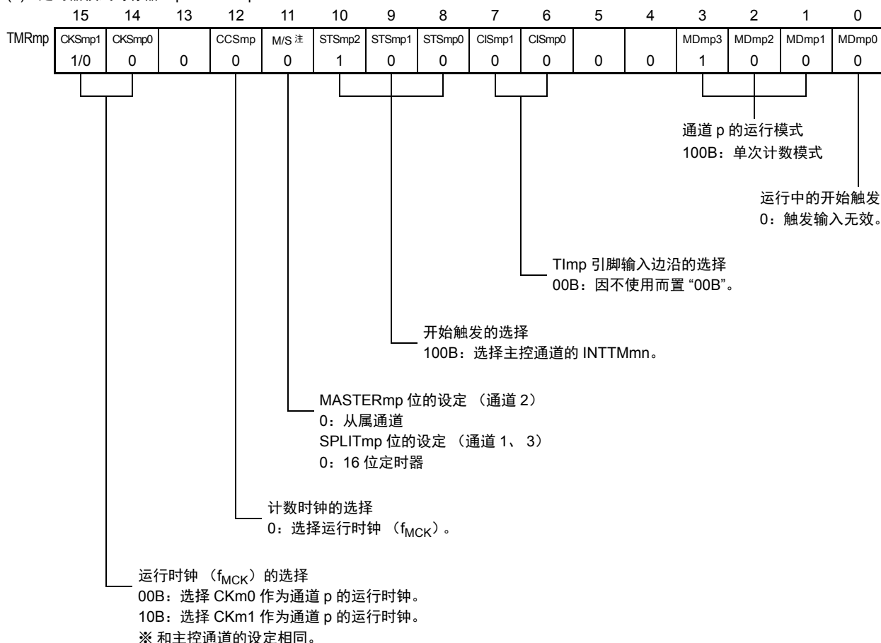
(a) 定时器模式寄存器 mp (TMRmp)
