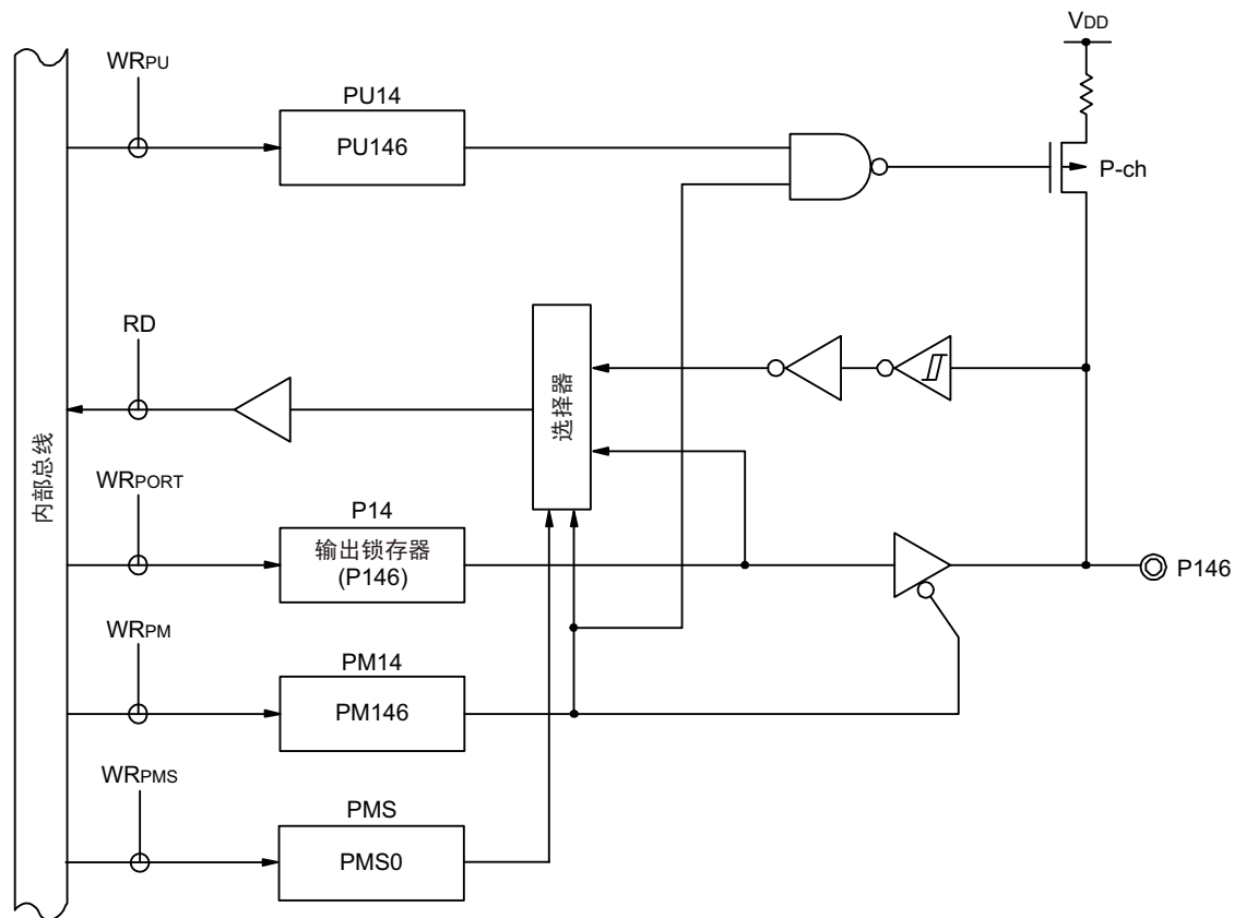
图 4-24 P146 的框图
