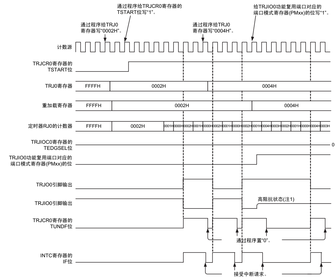
图 7-12 脉冲输出模式的运行例子
