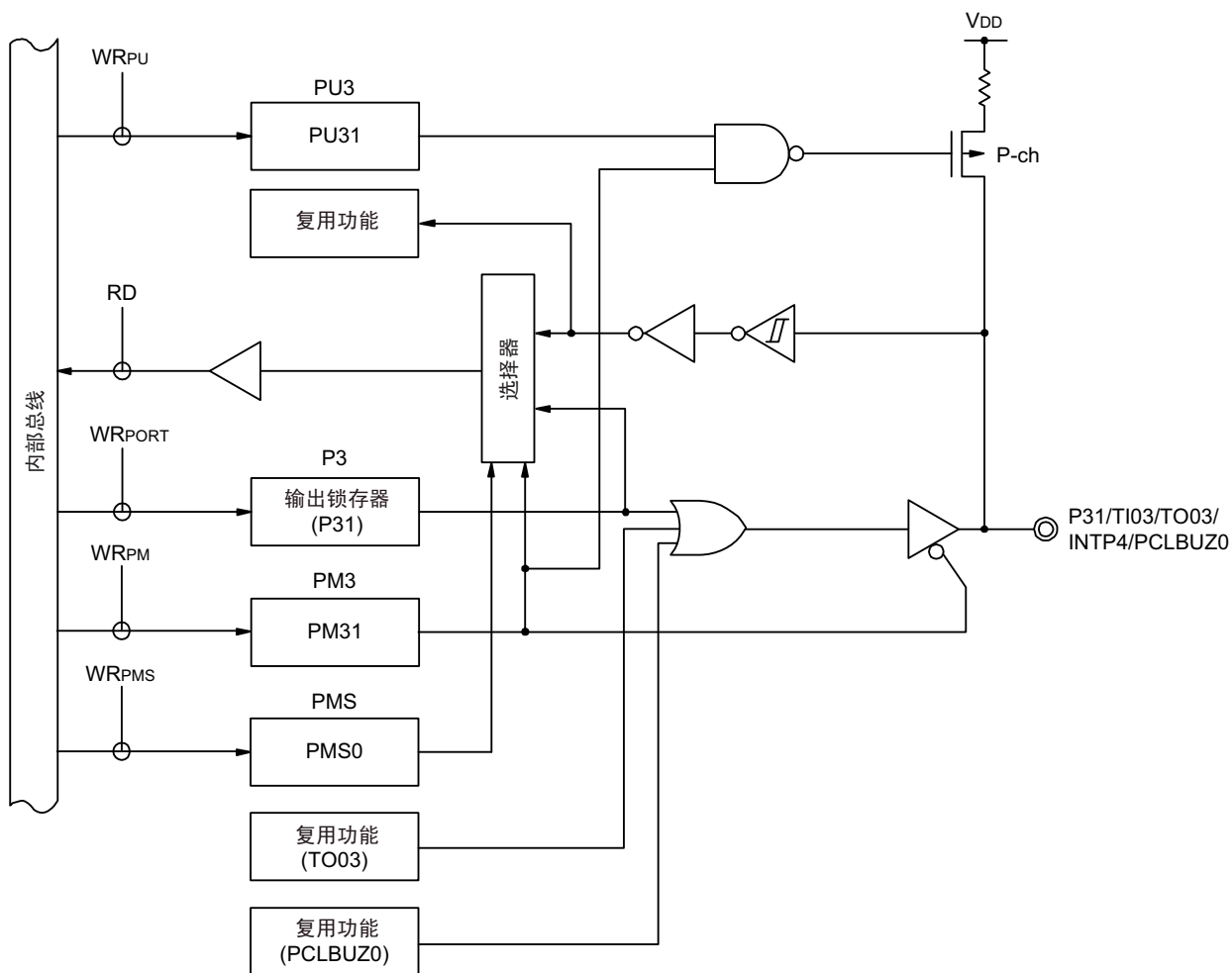
图 4-13 P31 的框图
