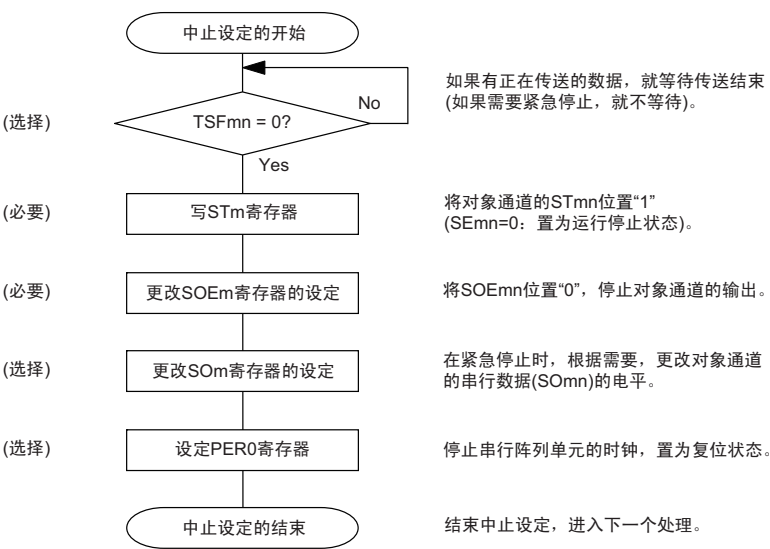
图 14-64 从属发送和接收的中止步骤
