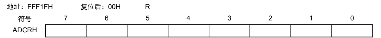
图 12-10 8 位 A/D 转换结果寄存器（ADCRH）的格式
