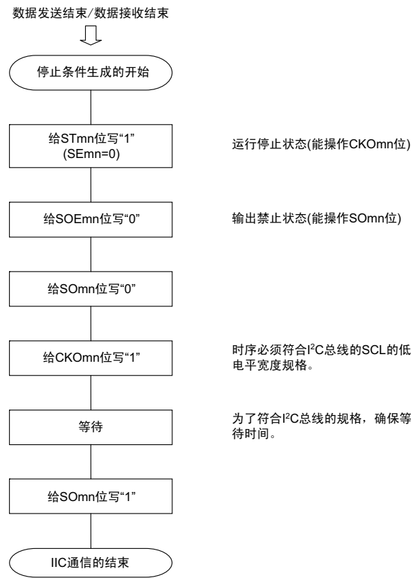
图 14-133 产生停止条件的流程图
