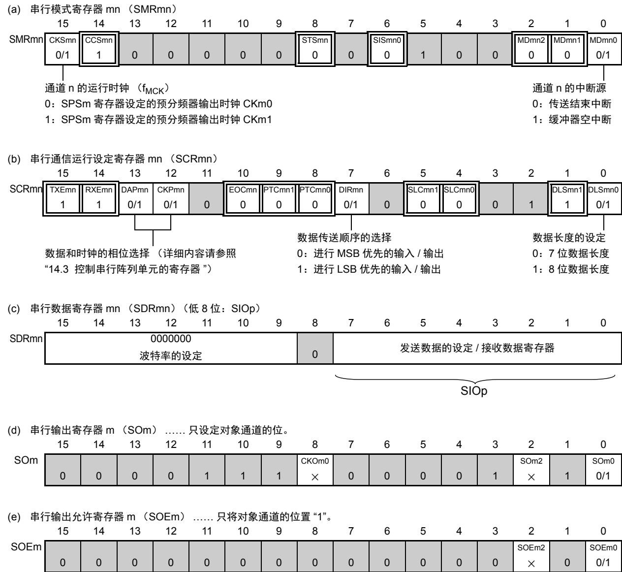
图 14-91 从属选择输入功能（CSI00）从属发送和接收时的寄存器设定内容例子 (1/2)
