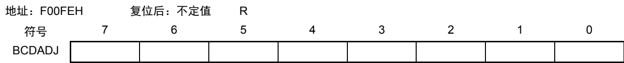
图 27-1 BCD 校正结果寄存器（BCDADJ）的格式
