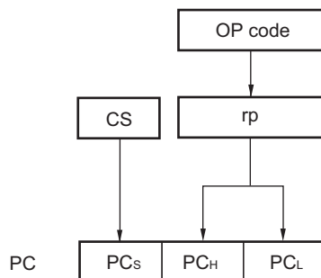
图 3-17 寄存器直接寻址的概要
