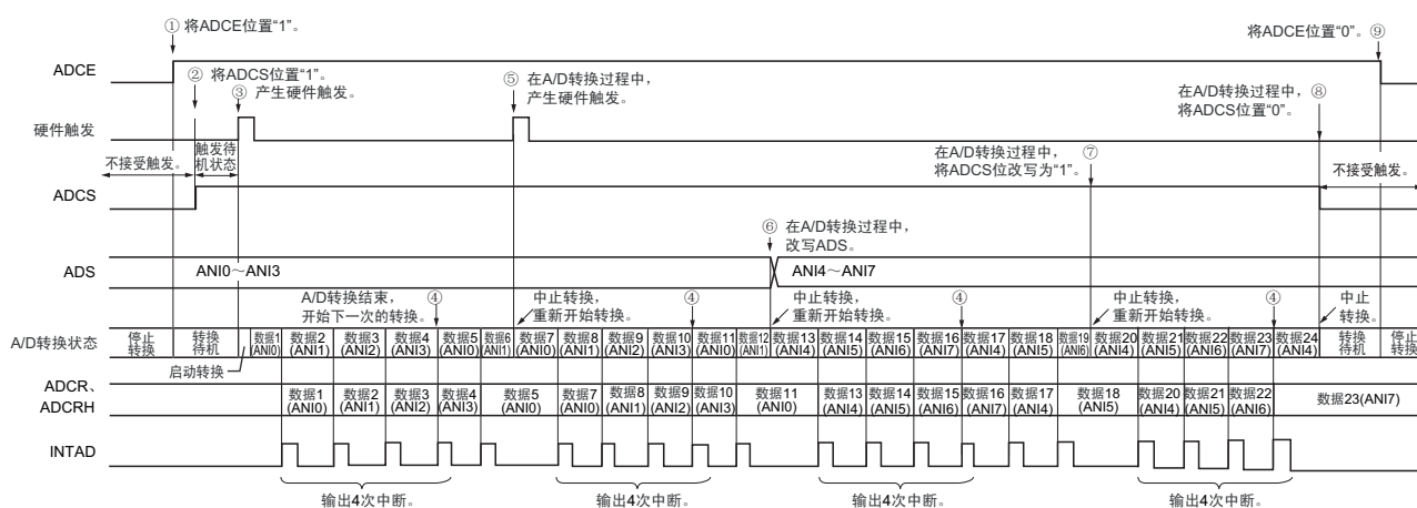
图 12-23 硬件触发无等待模式（扫描模式、连续转换模式）的运行时序例子
