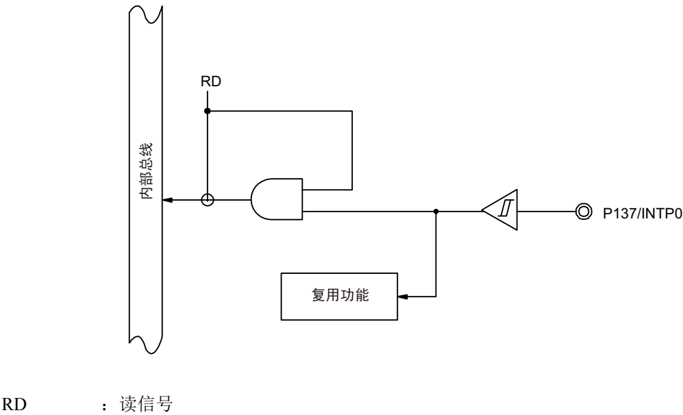
图 4-23 P137 的框图
