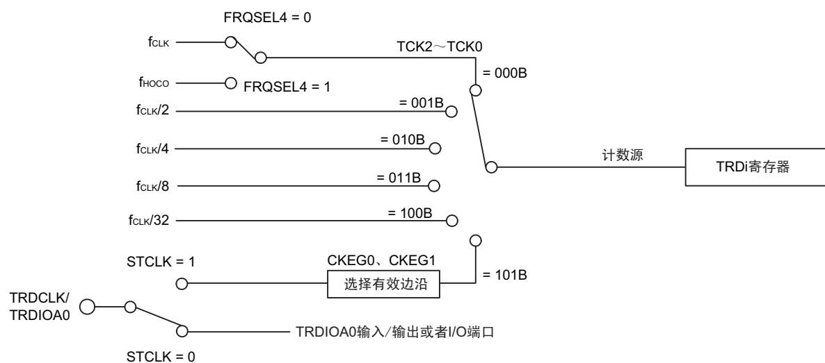
图 8-41 计数源的框图
