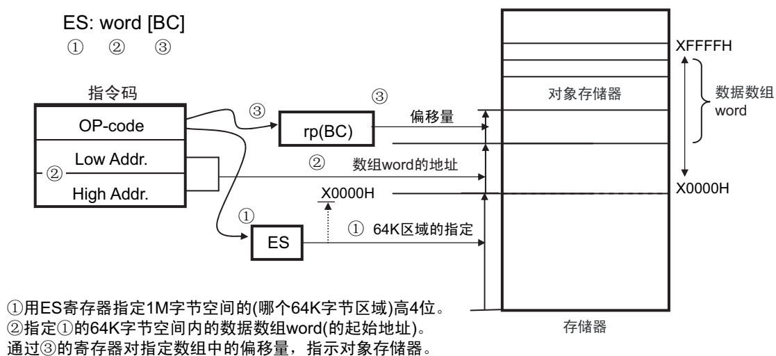
图 3-32 ES:word[BC] 的例子
