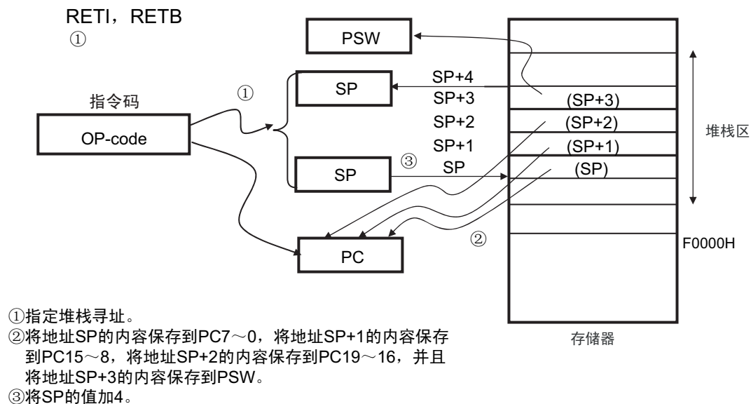
图 3-40 RETI、RETB 的例子
