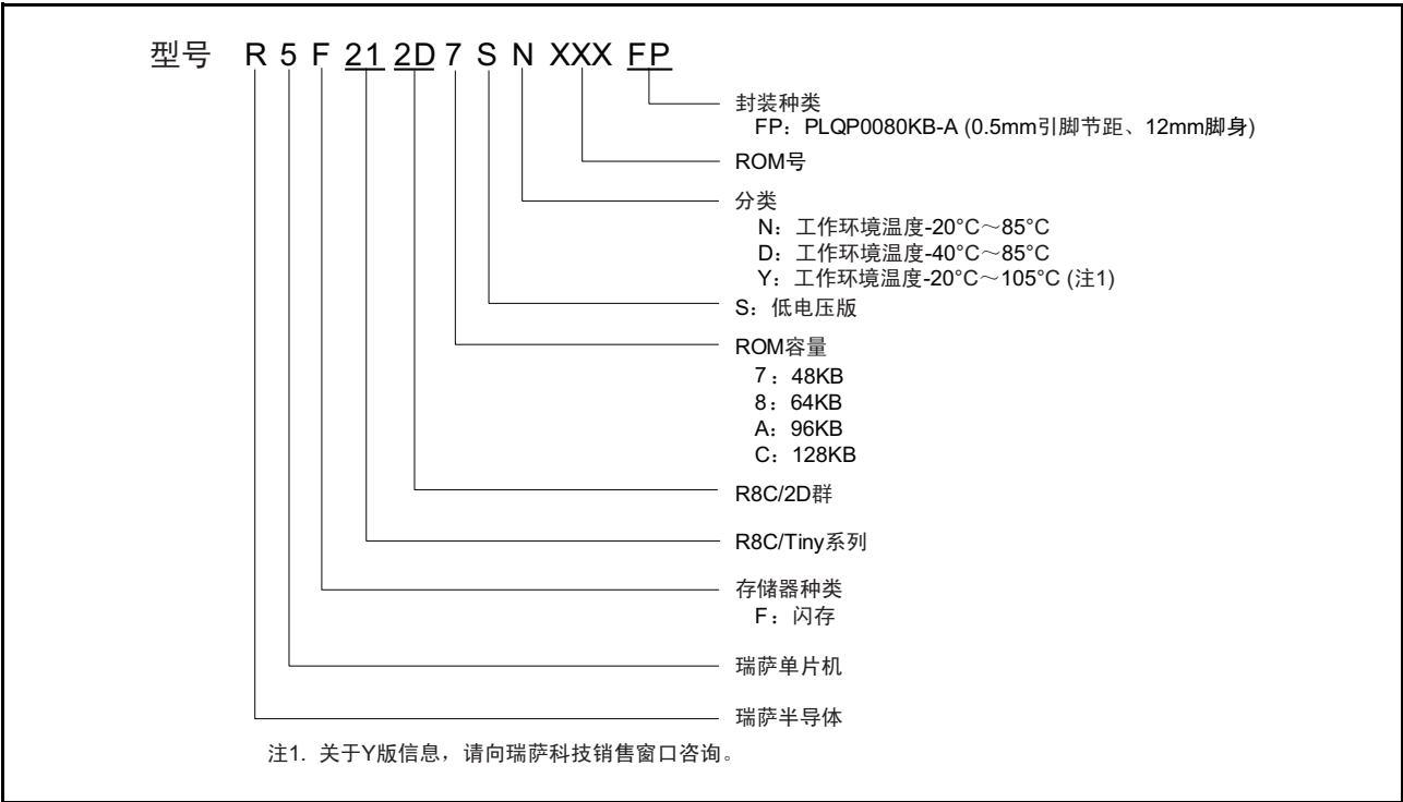
图 1.2 R8C/2D 群的型号和存储器容量、封装
