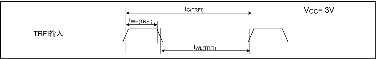
图 22.15 V_{CC}=3V 时的 TRFI 输入时序
