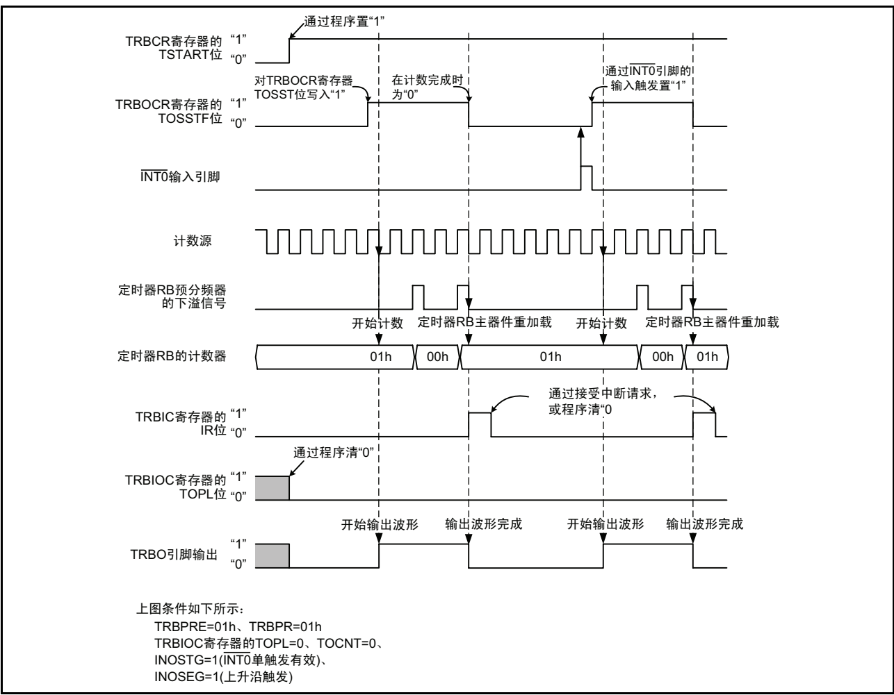
图 15.21 可编程单触发产生模式时的运行例
