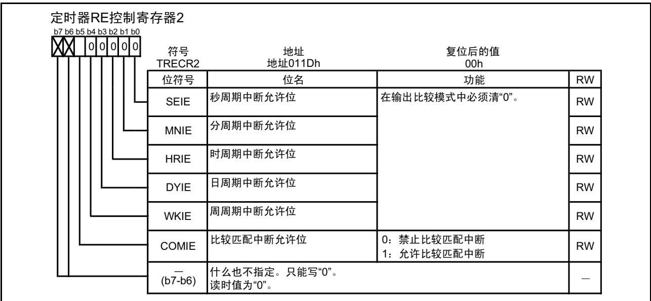
图 15.166 输出比较模式时的 TREC2 寄存器
