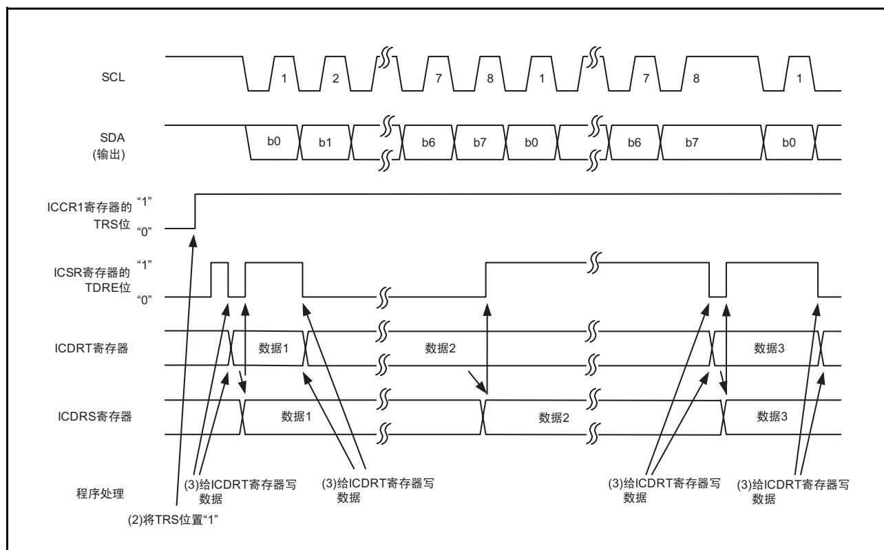
图 17.43 发送模式的运行时序（时钟同步串行模式）
