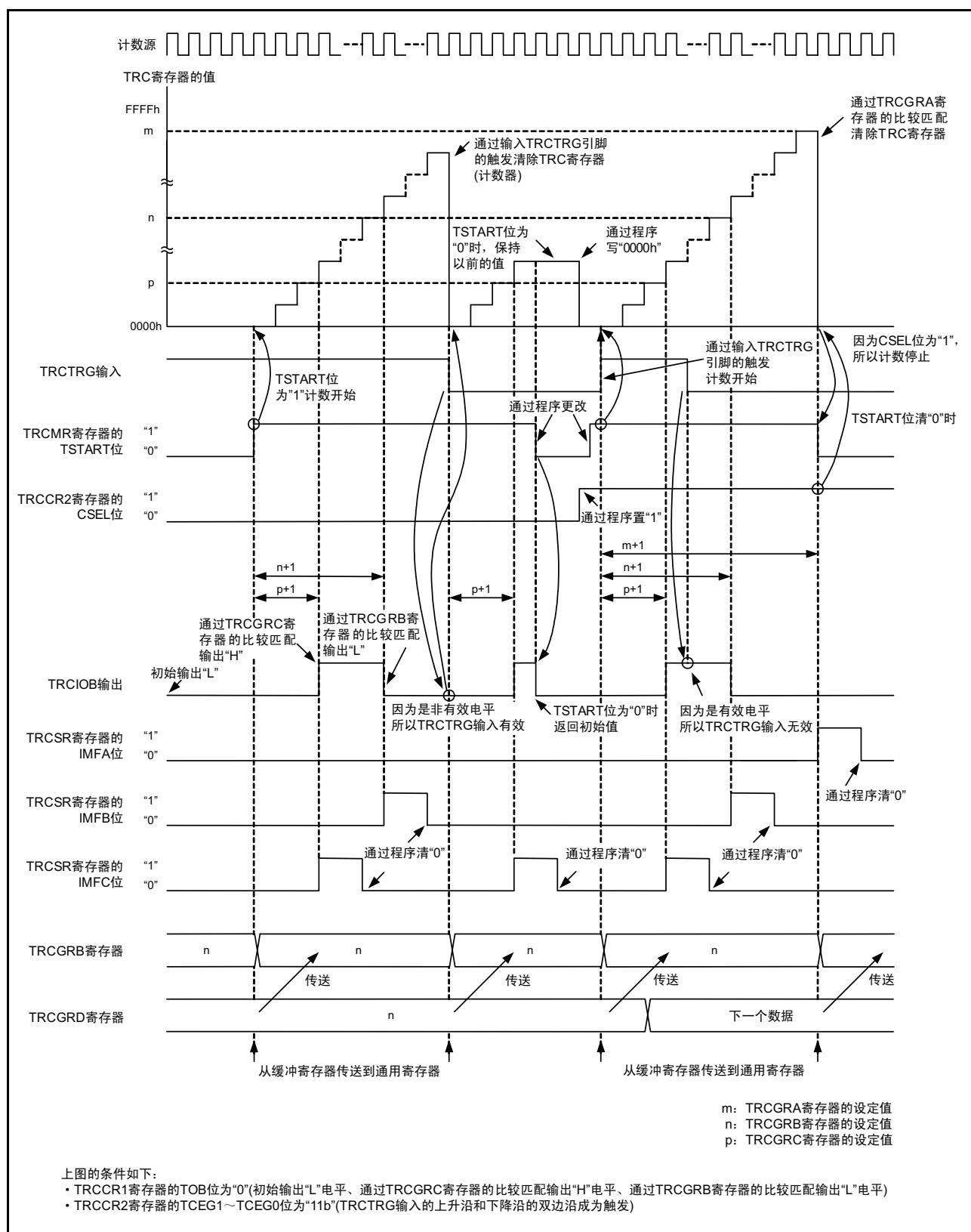
图 15.59 PWM2 的运行例 (允许 TRCTRG 触发输入时)
