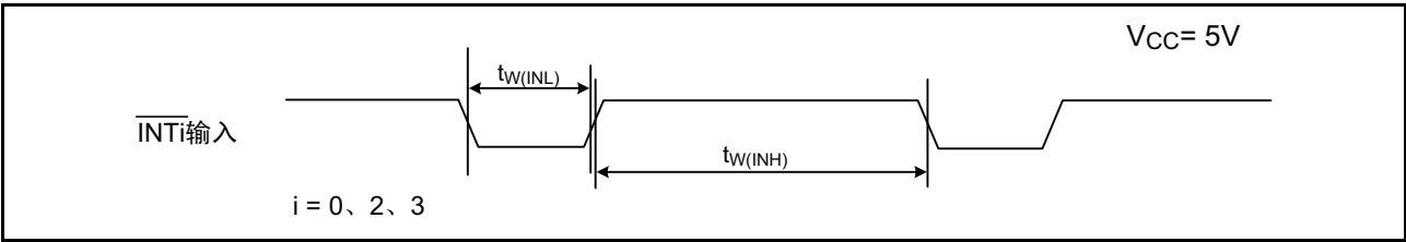
图 22.12 V_{CC}=5V 时的外部中断 \overline{\text{INTi}} 输入时序
