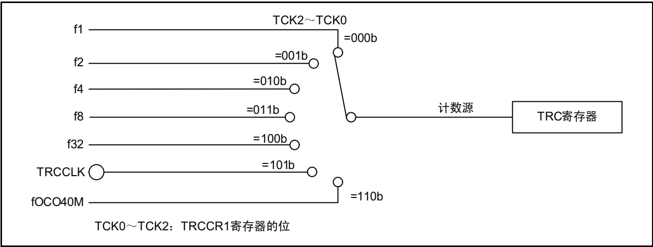
图 15.38 计数源的框图
