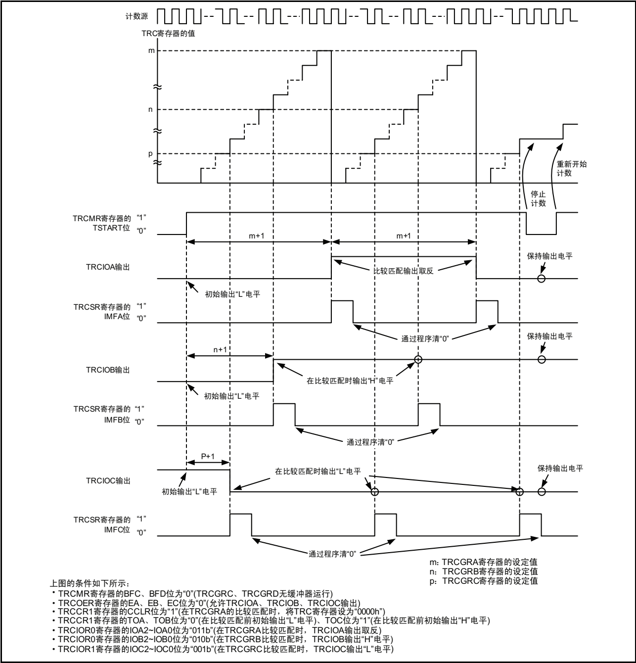
图 15.51 输出比较功能的运行例
