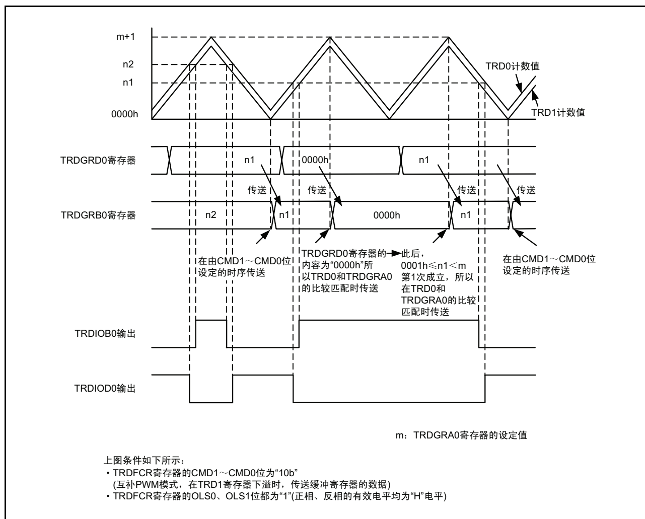
图 2.7 互补 PWM 模式时的缓冲寄存器的值为“0000h”时的运行例
