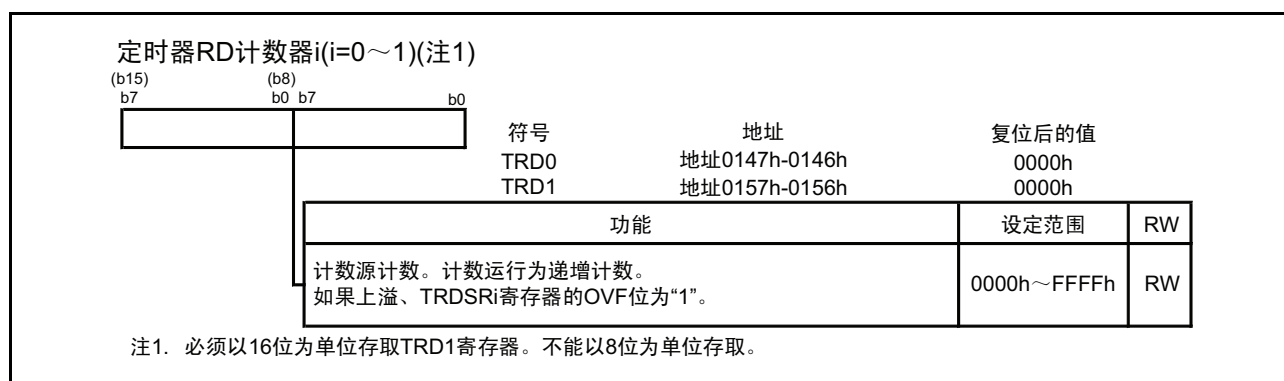
图 15.109 PWM 模式时的 TRD0 ~ TRD1 寄存器
