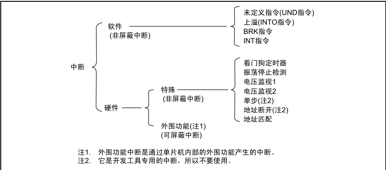
图 13.1 中断分类
