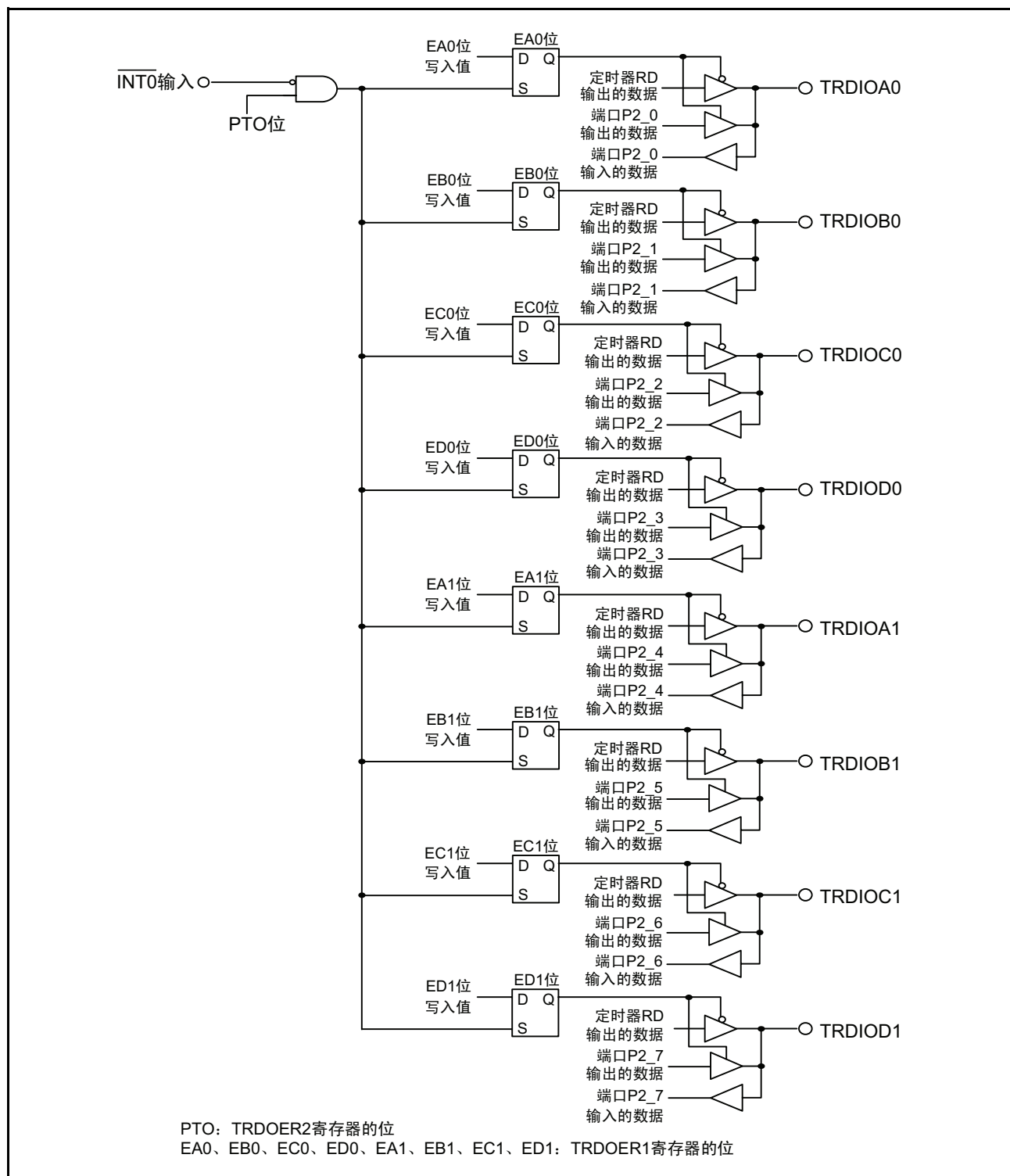
图 15.67 脉冲输出强制截止
