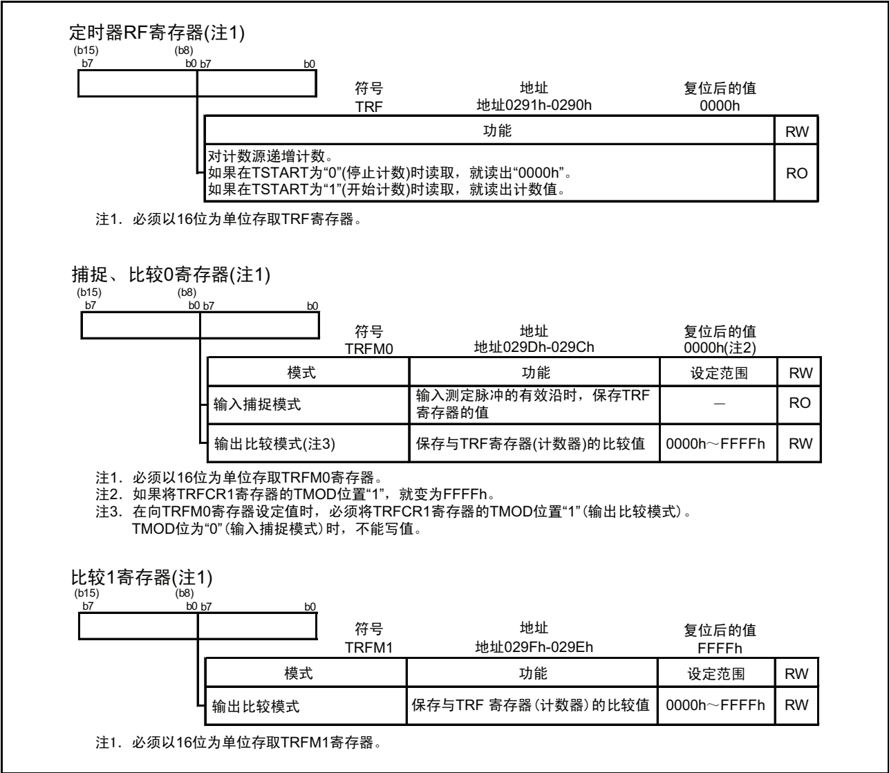
图 15.173 TRF、TRFM0、TRFM1 寄存器
