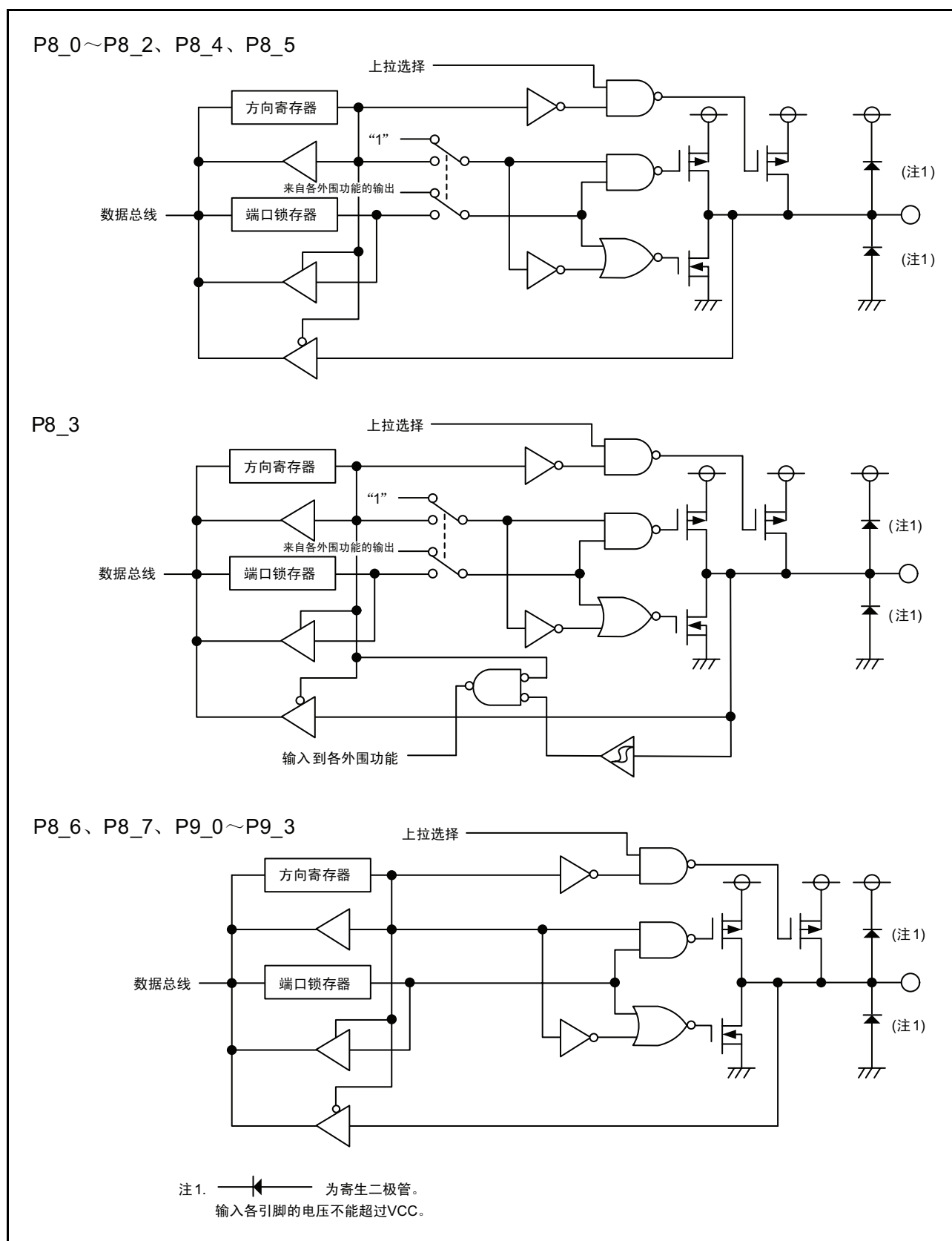
图 8.11 可编程输入 / 输出端口的结构 (11)
