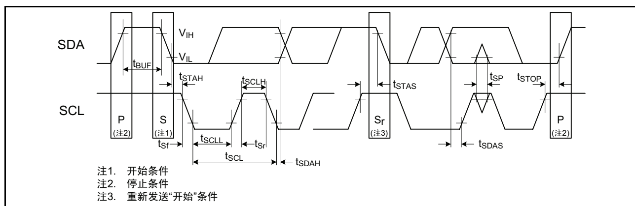
图 22.7 I 2 C 总线接口的输入 / 输出时序
