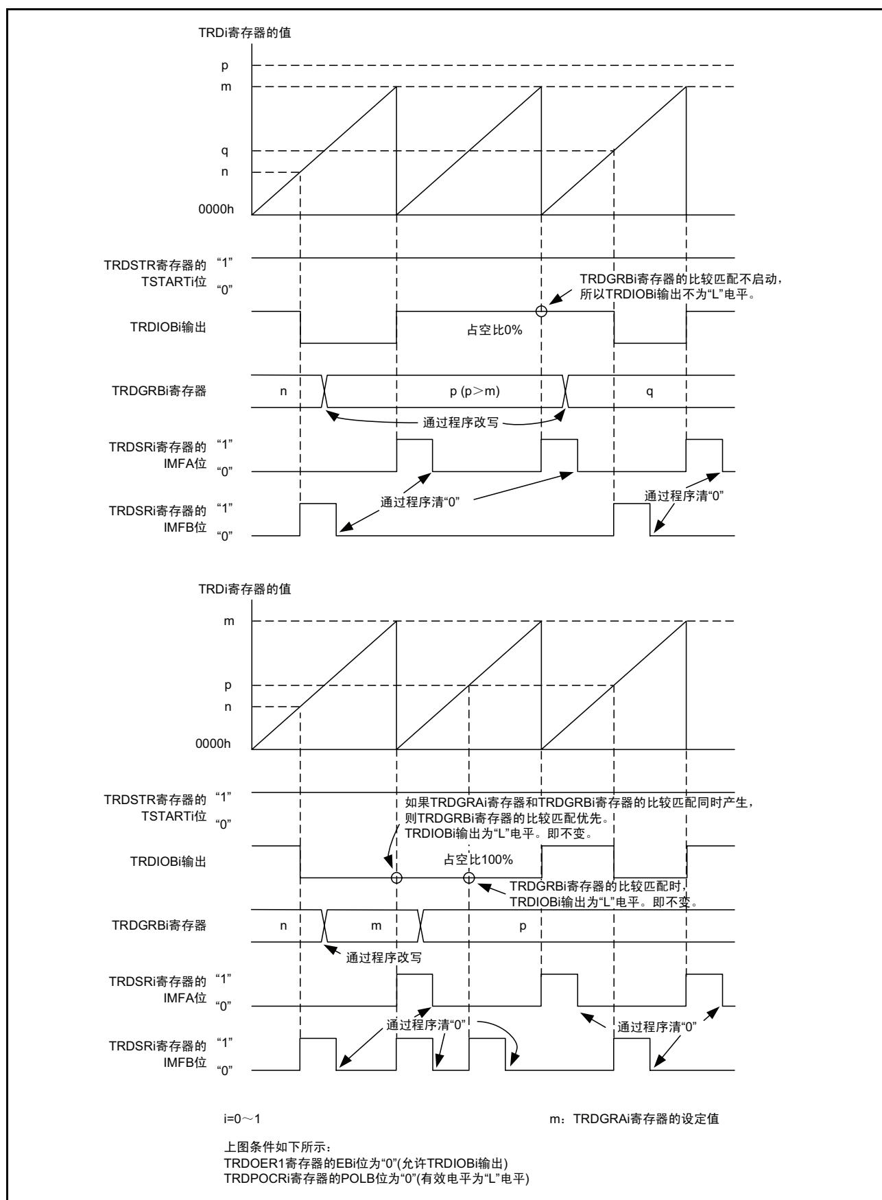
图 15.112 PWM 模式时的运行例（占空比 0%、占空比 100%）
