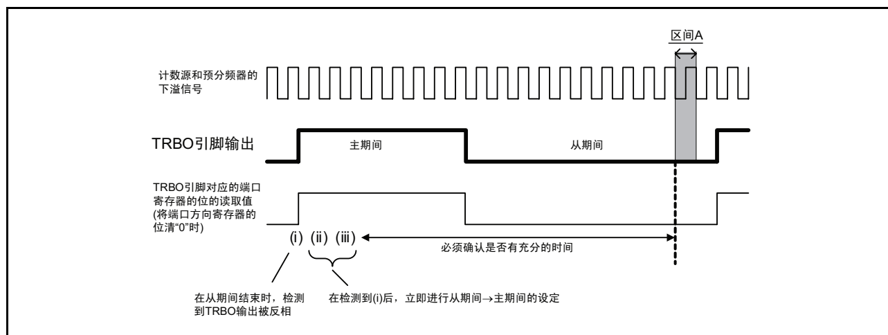
图 2.3 读对策 (b) 的 TRBO 引脚输出值的例
