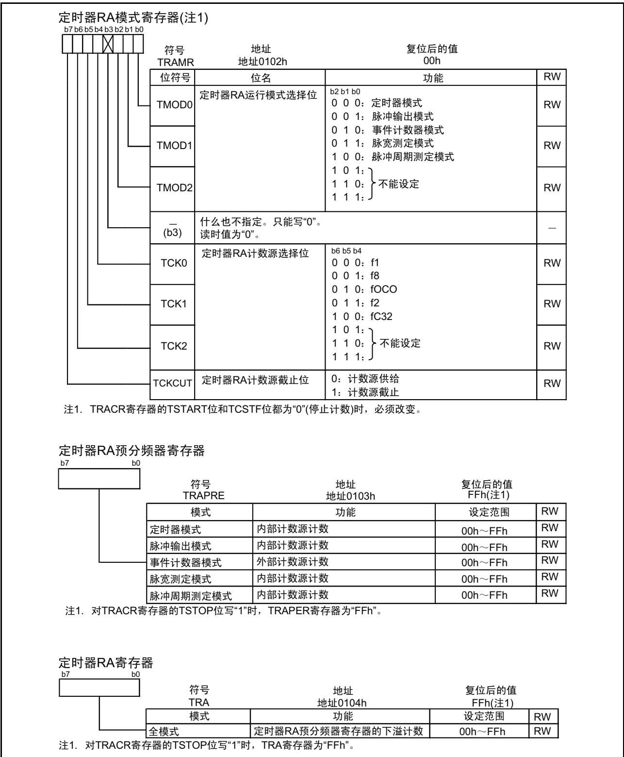
图 15.3 TRAMR、TRAPRE、TRA 寄存器
