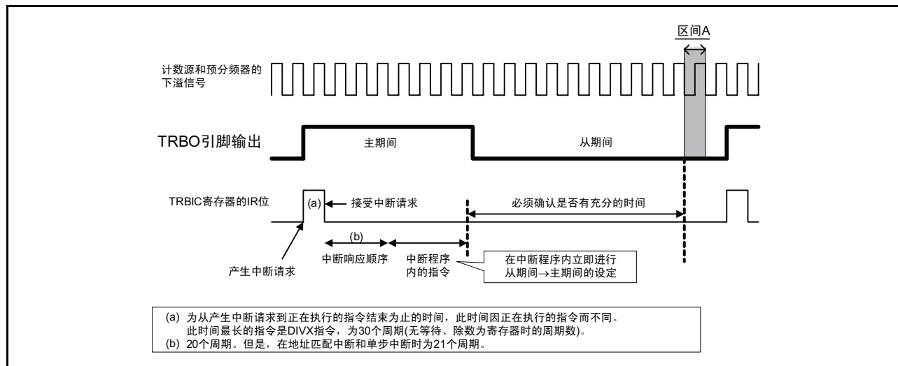
图 2.2 使用对策 (a) 的定时器 RB 中断的例
