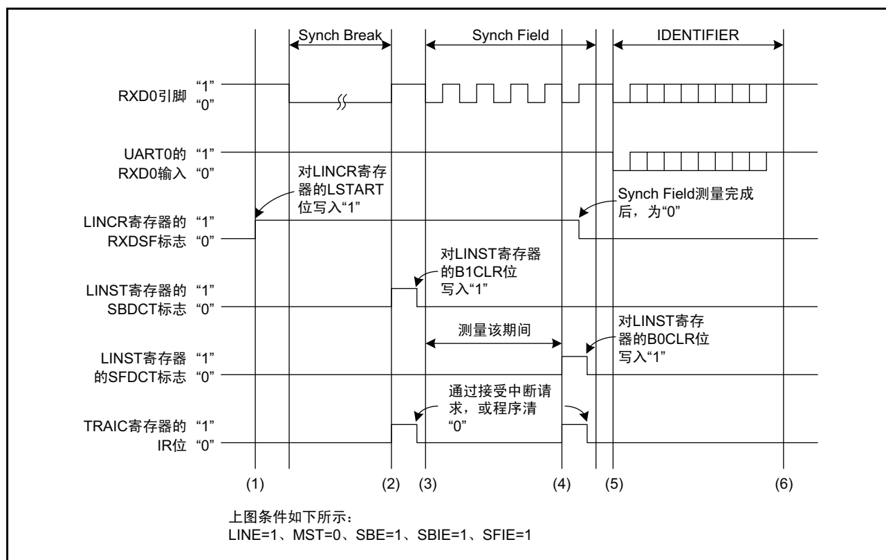
图 18.7 接收头字段时的运行例
