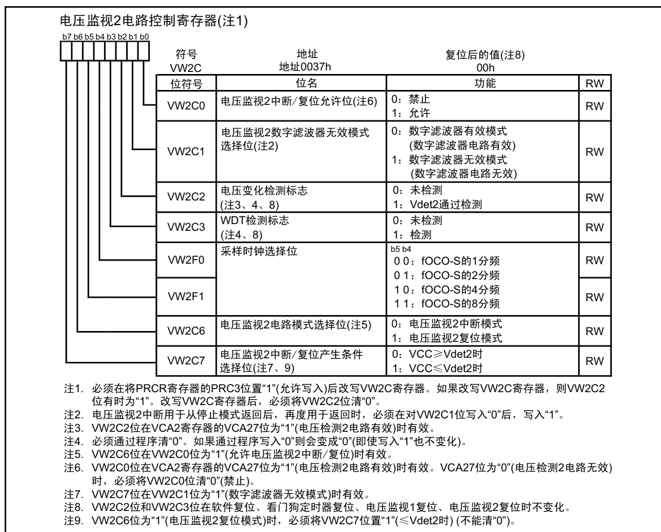
图 7.8 VW2C 寄存器
