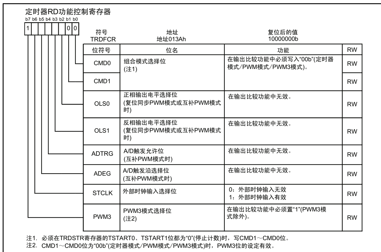
图 15.87 输出比较功能时 TRDFCR 寄存器
