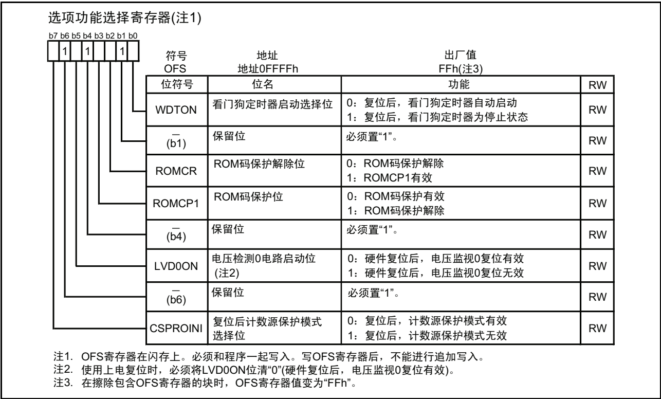
图 6.4 OFS 寄存器
