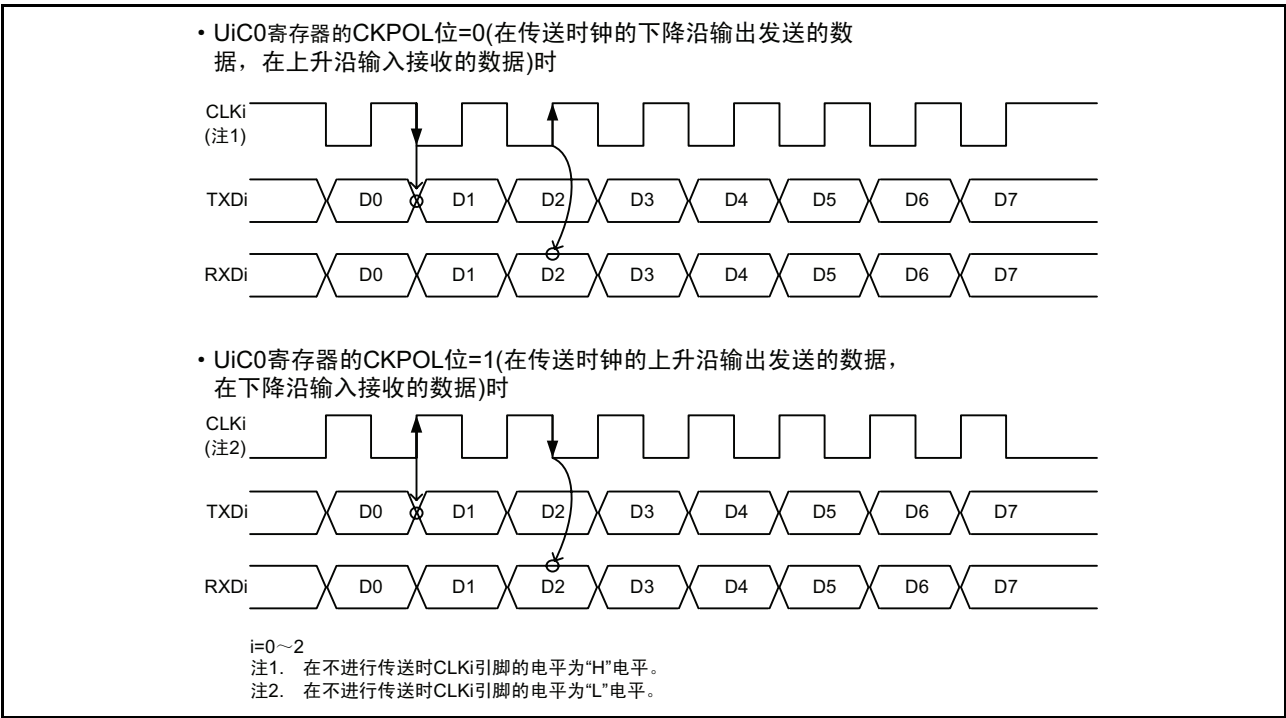
图 16.10 传送时钟的极性
