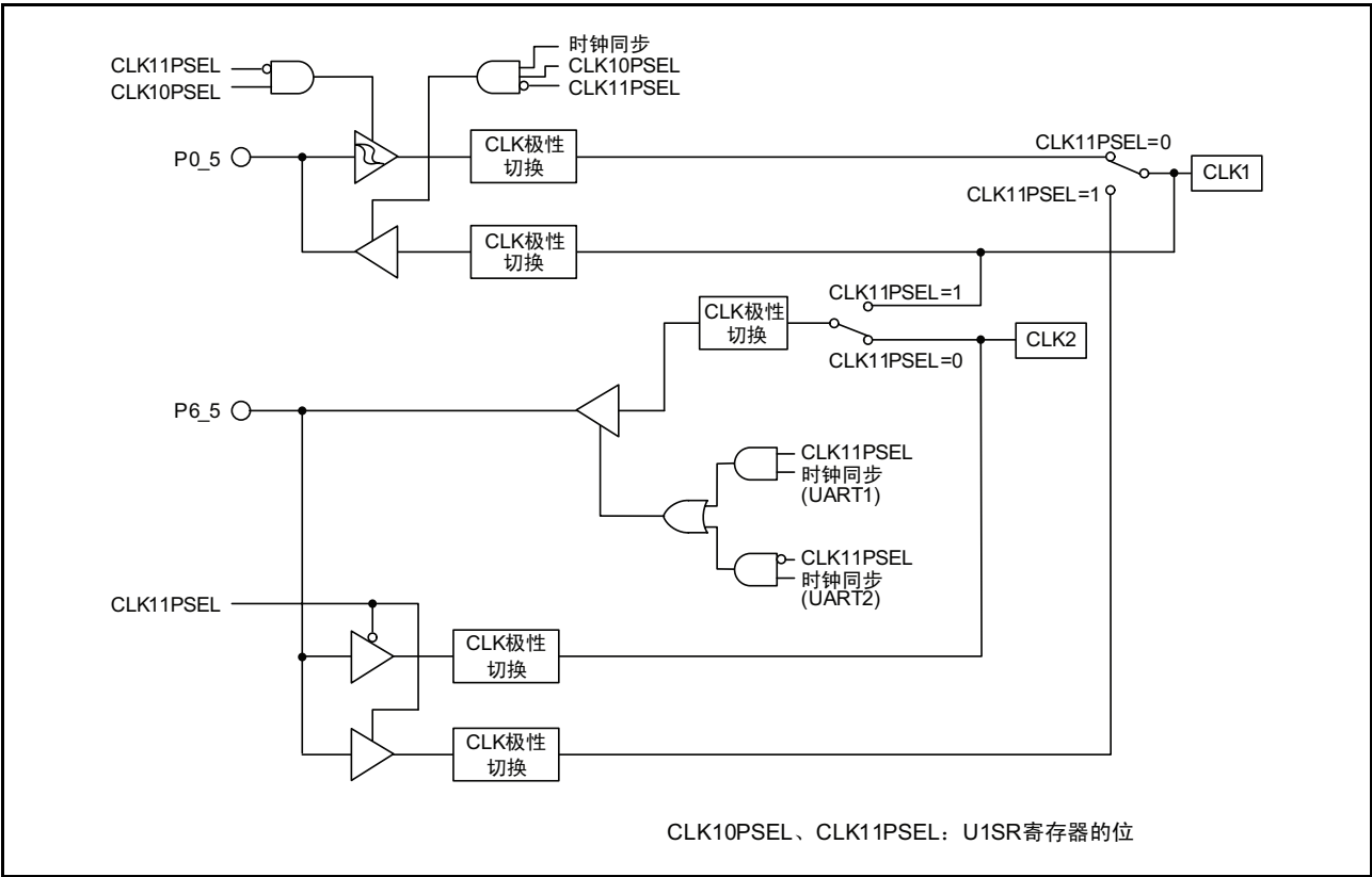
图 16.3 CLK1、CLK2 引脚切换部分的框图
