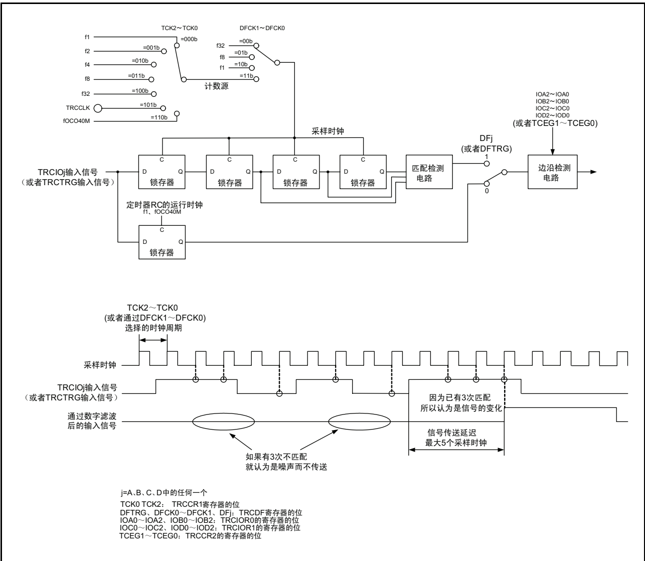
图 15.41 数字滤波器的框图
