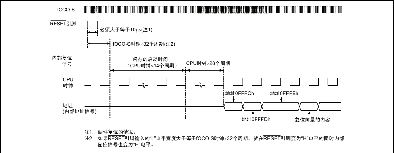
图 6.3 复位顺序
