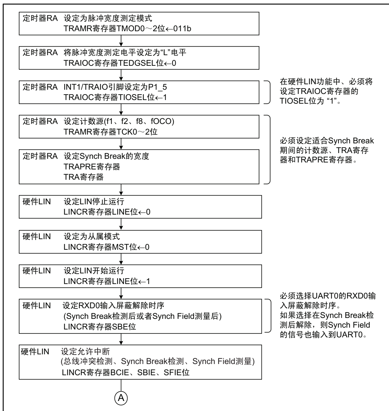
图 18.8 接收头字段的流程图的例子 (1)
