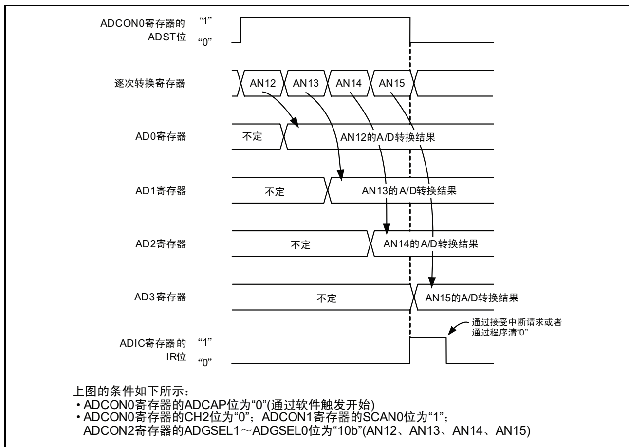
图 19.9 单次扫描模式时的运行示例
