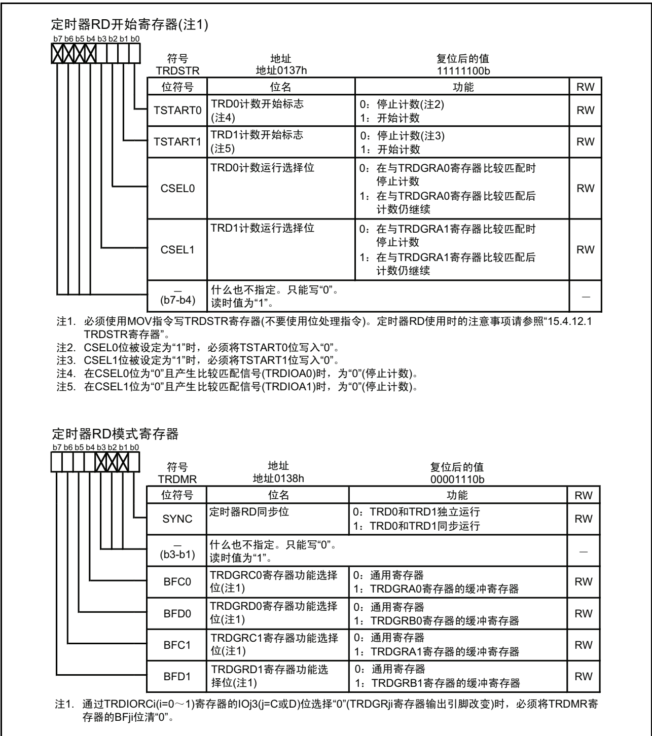
图 15.85 输出比较功能时的 TRDSTR、TRDMR 寄存器
