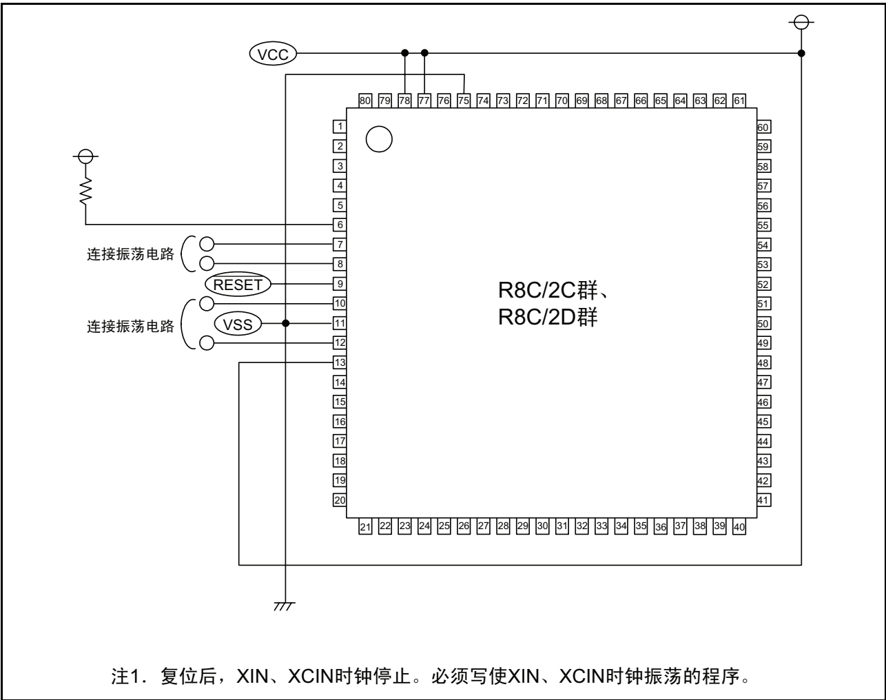
附图 3.1 振荡评价电路例
