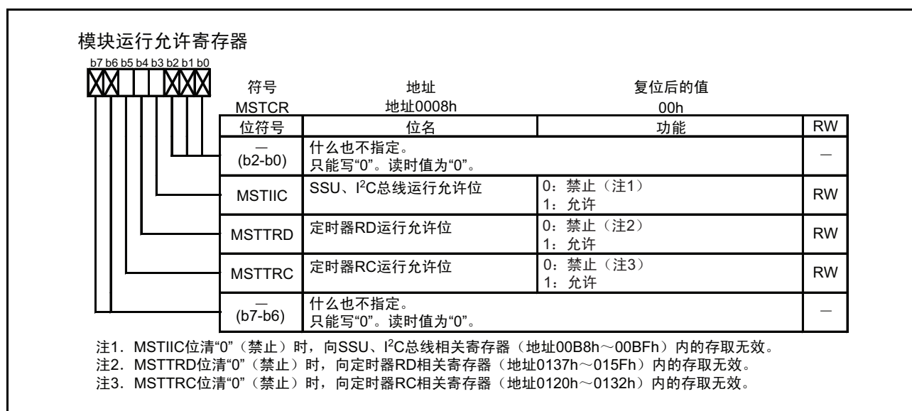
图 15.27 MSTCR 寄存器
