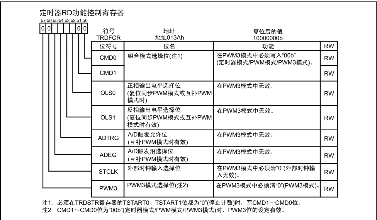
图 15.139 PWM3 模式时的 TRDFCR 寄存器
