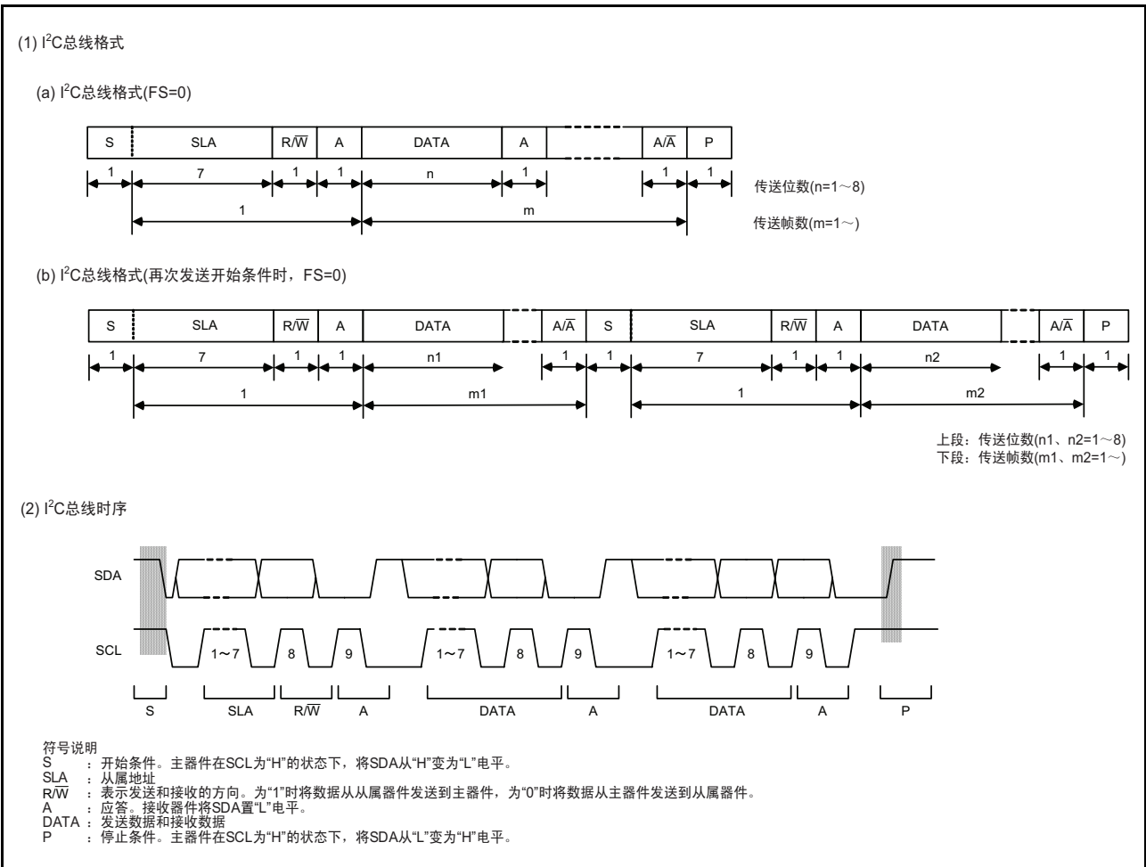
图 17.33 I 2 C 总线格式和总线时序
