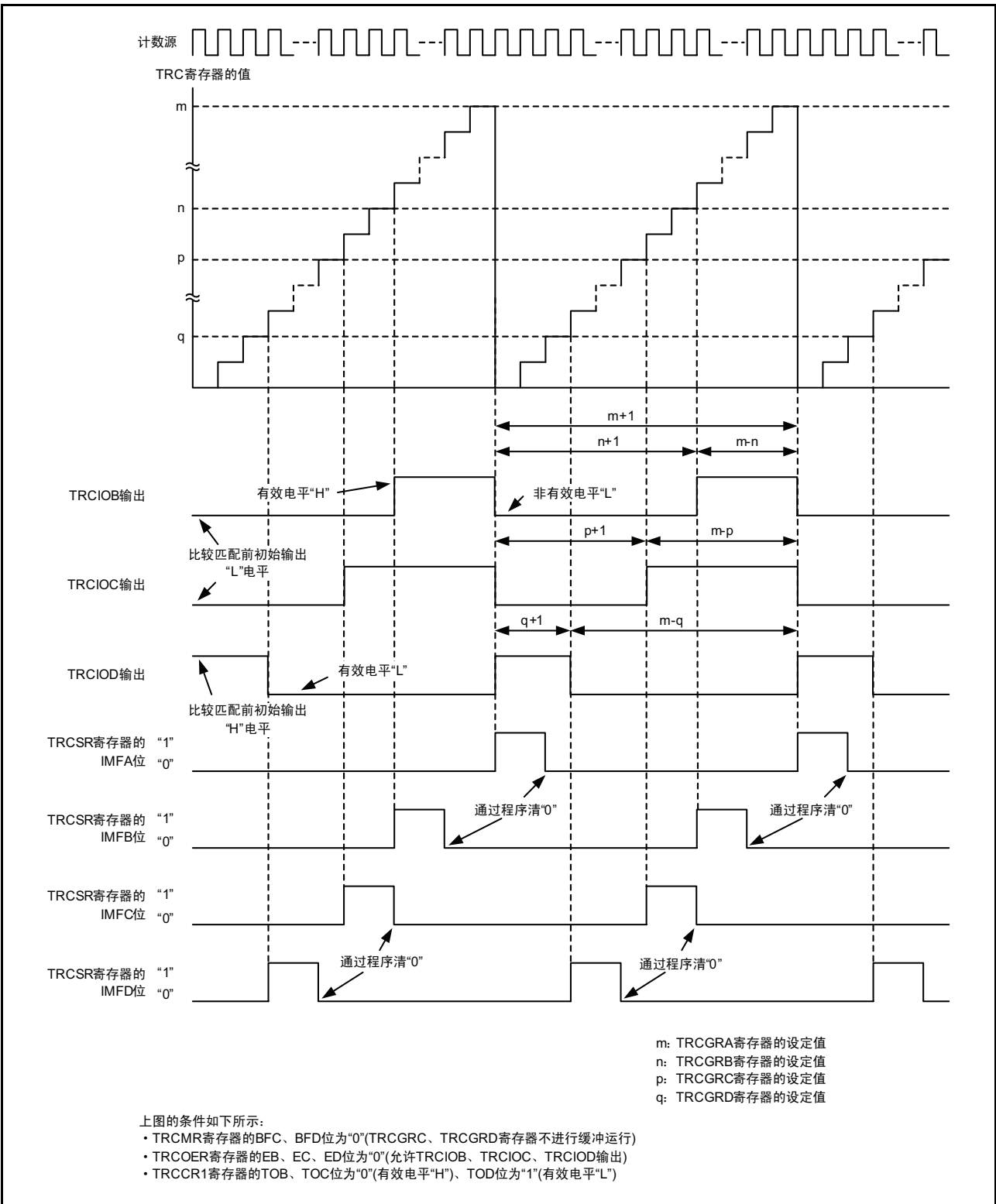
图 15.54 PWM 模式的运行例
