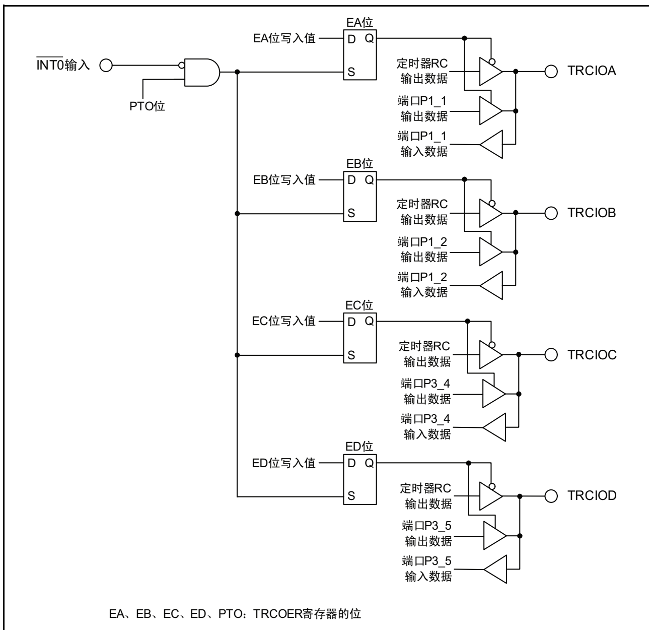
图 15.42 脉冲输出强制截止
