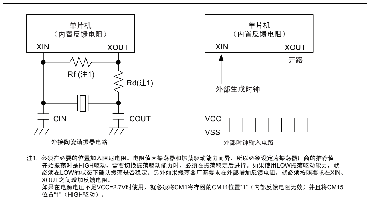
图 11.11 XIN 时钟的连接电路例
