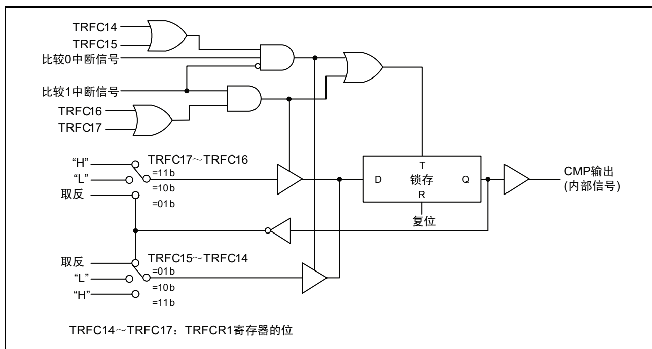
图 15.171 CMP 波形产生部框图
