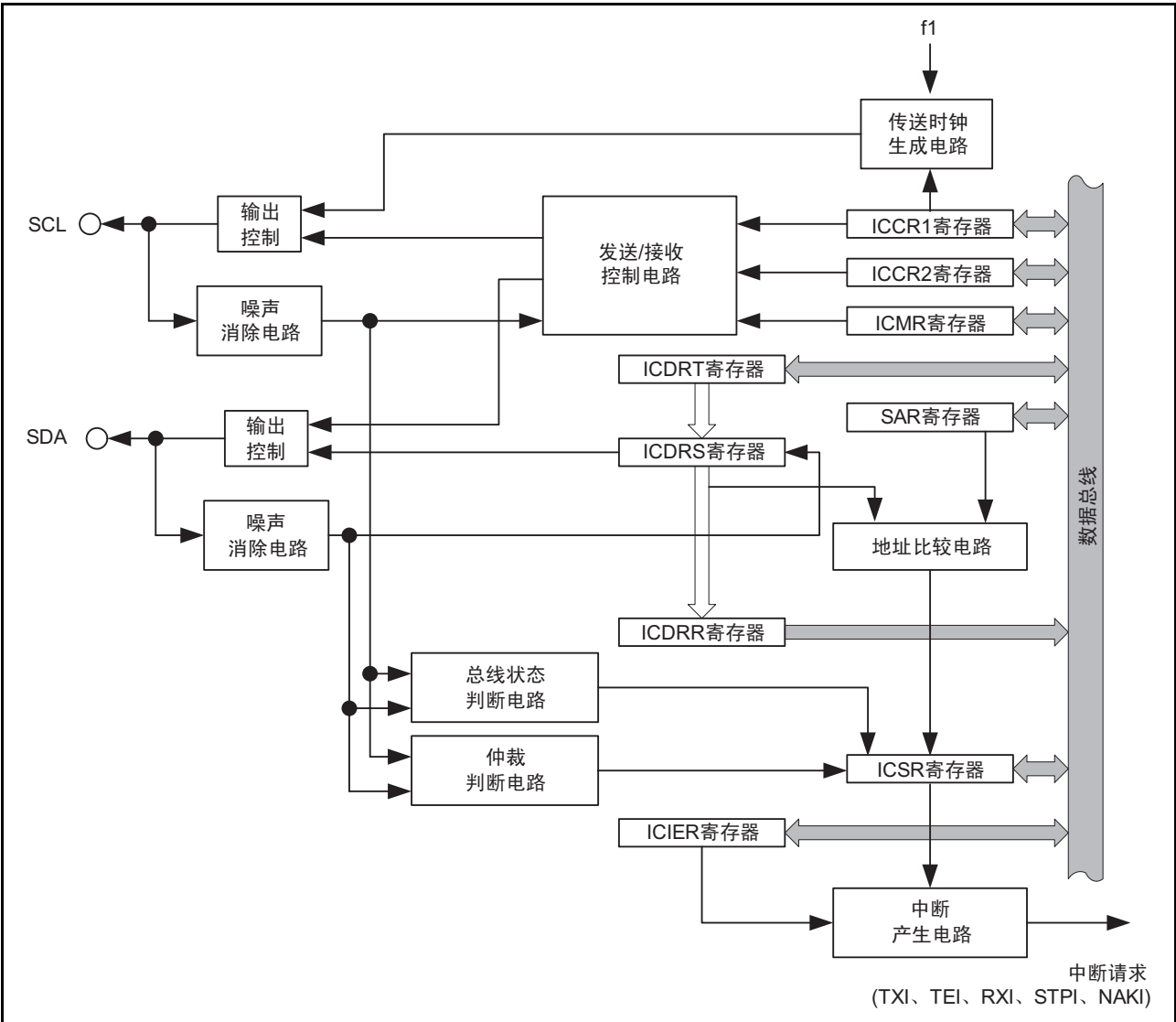
图 17.23 I 2 C 总线接口的框图
