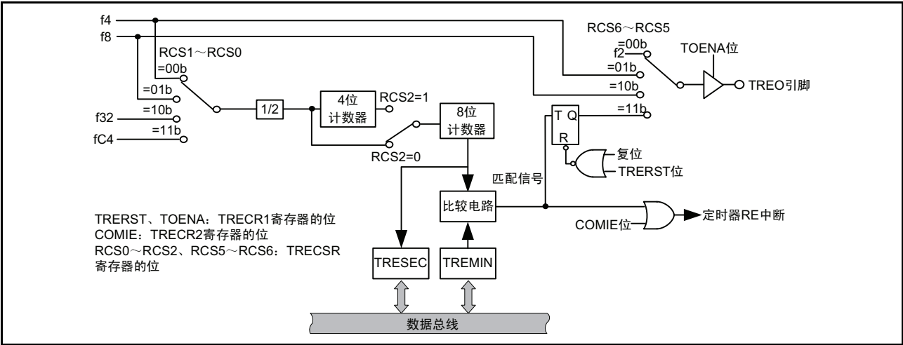
图 15.162 输出比较模式的框图
