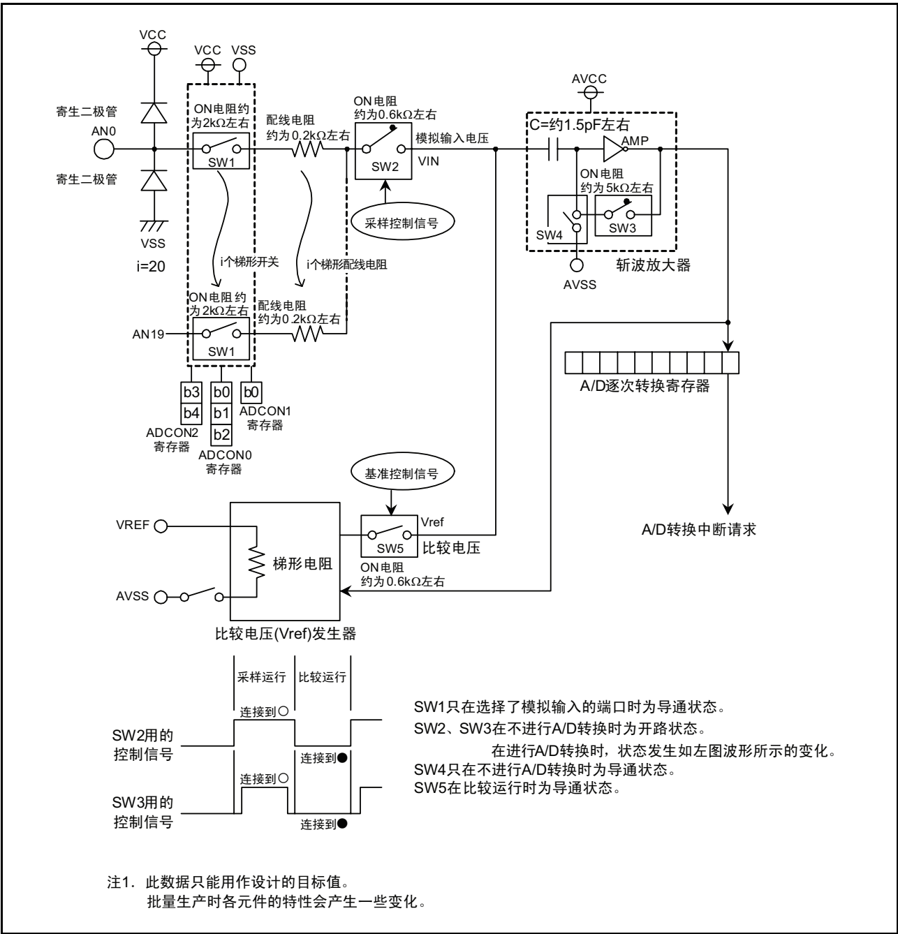
图 19.11 模拟输入内部等效电路
