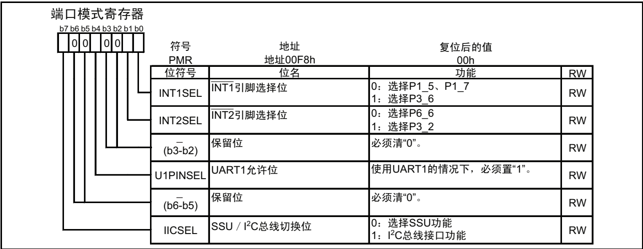
图 17.32 PMR 寄存器
