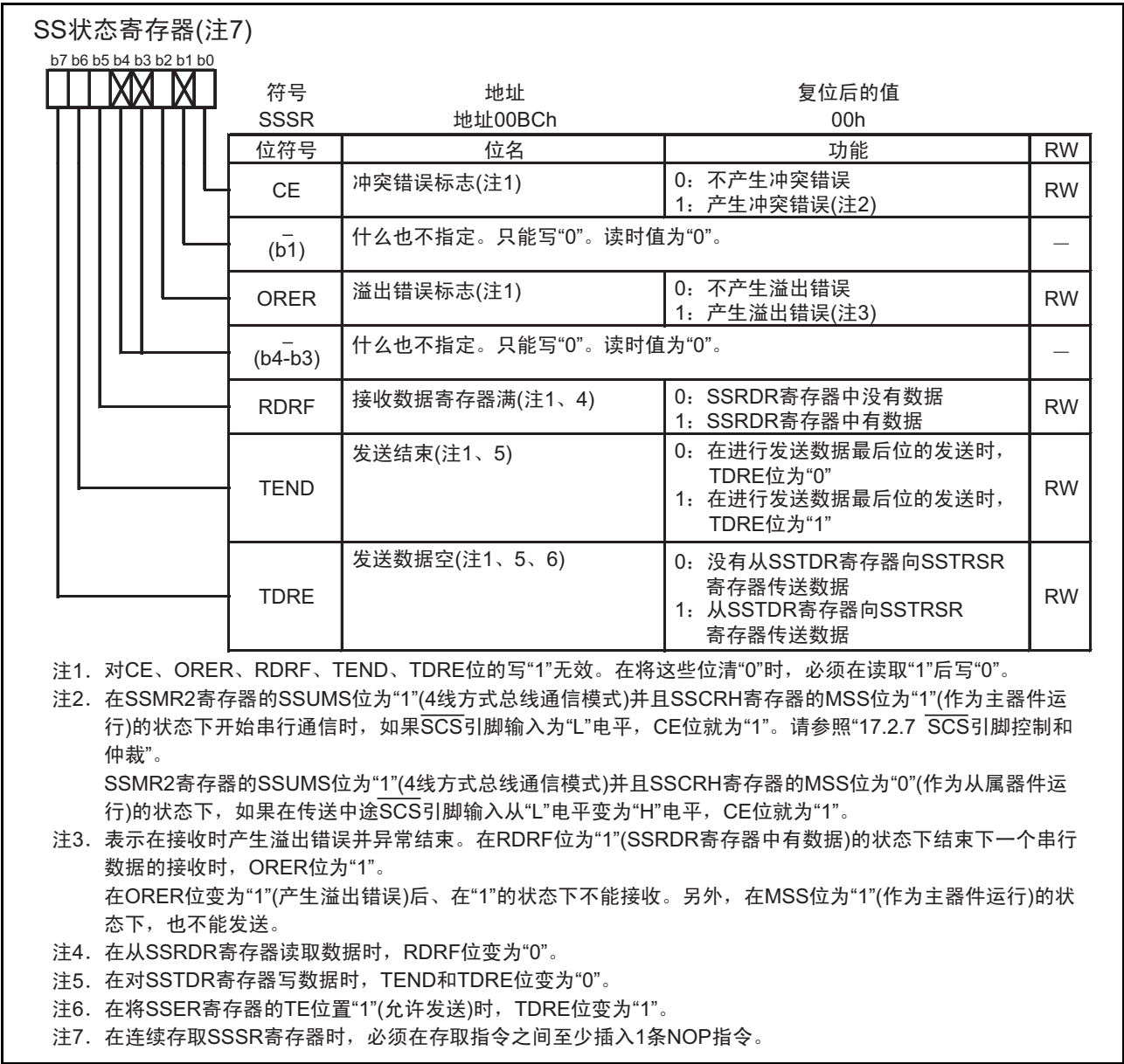
图 17.7 SSSR 寄存器
