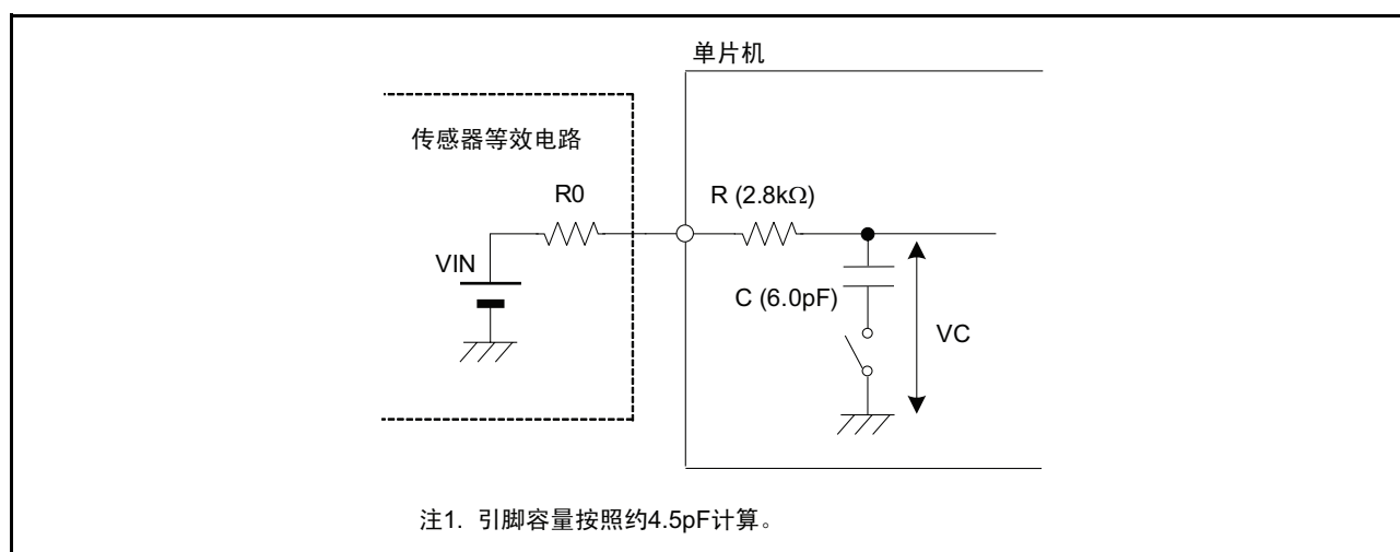
图 19.12 模拟输入引脚和外部传感器的等效电路例
