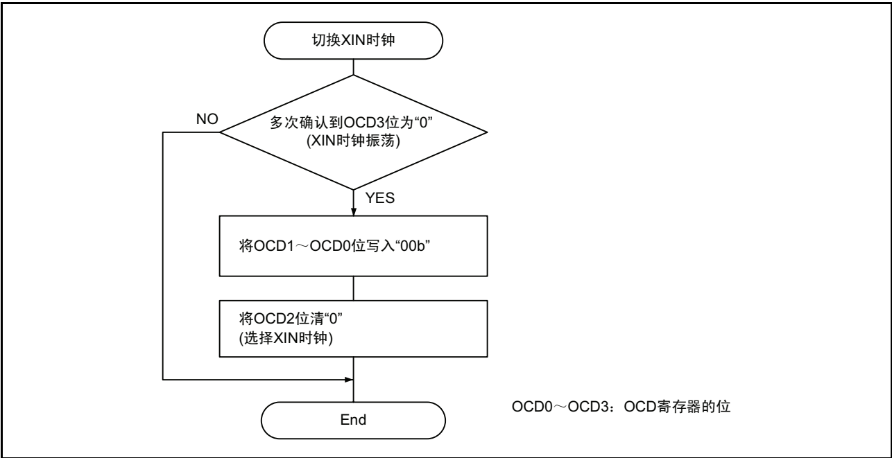
图 11.17 从低速内部振荡器转换到 XIN 时钟的步骤
