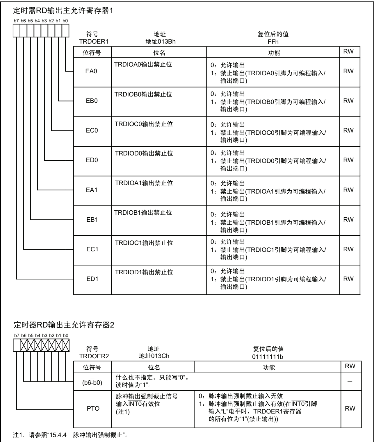
图 15.88 输出比较功能时的 TRDOER1 ~ TRDOER2 寄存器
