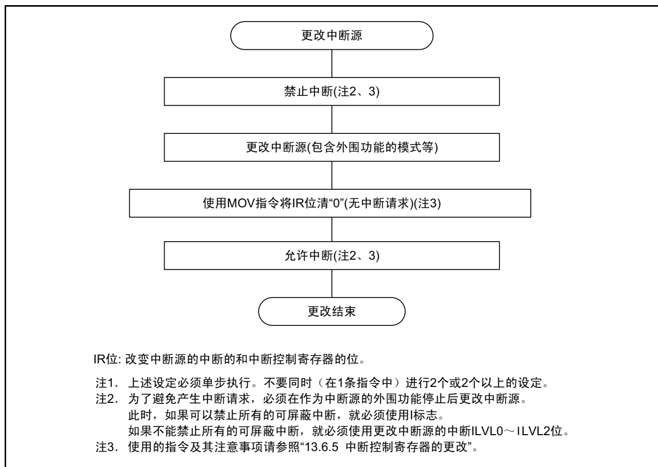
图 2.1 中断源更改步骤的例
