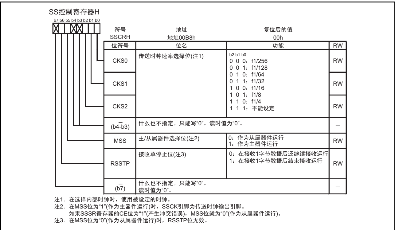
图 17.3 SSCRH 寄存器
