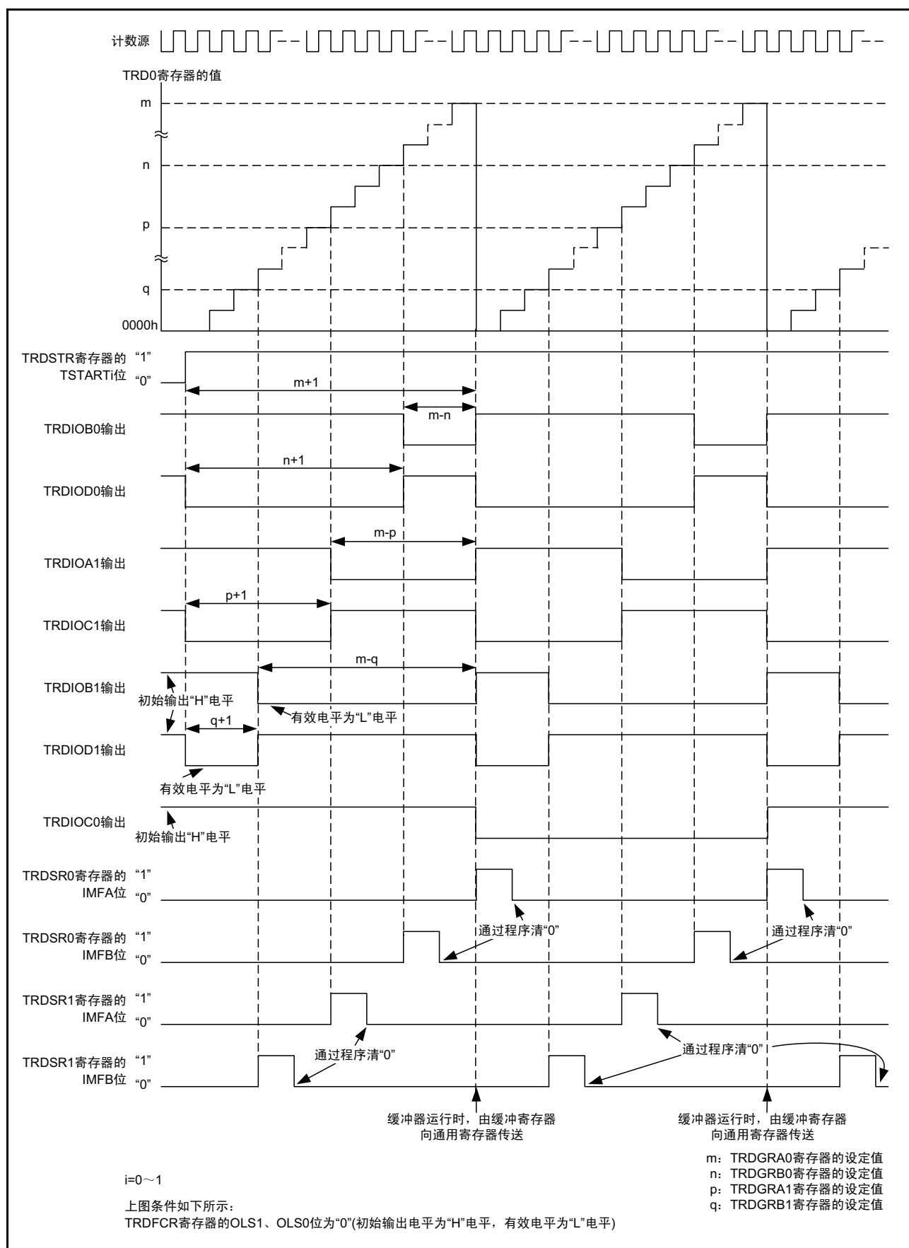
图 15.123 复位同步 PWM 模式的运行例
