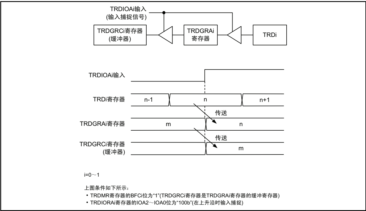
图 15.64 输入捕捉功能的缓冲器运行
