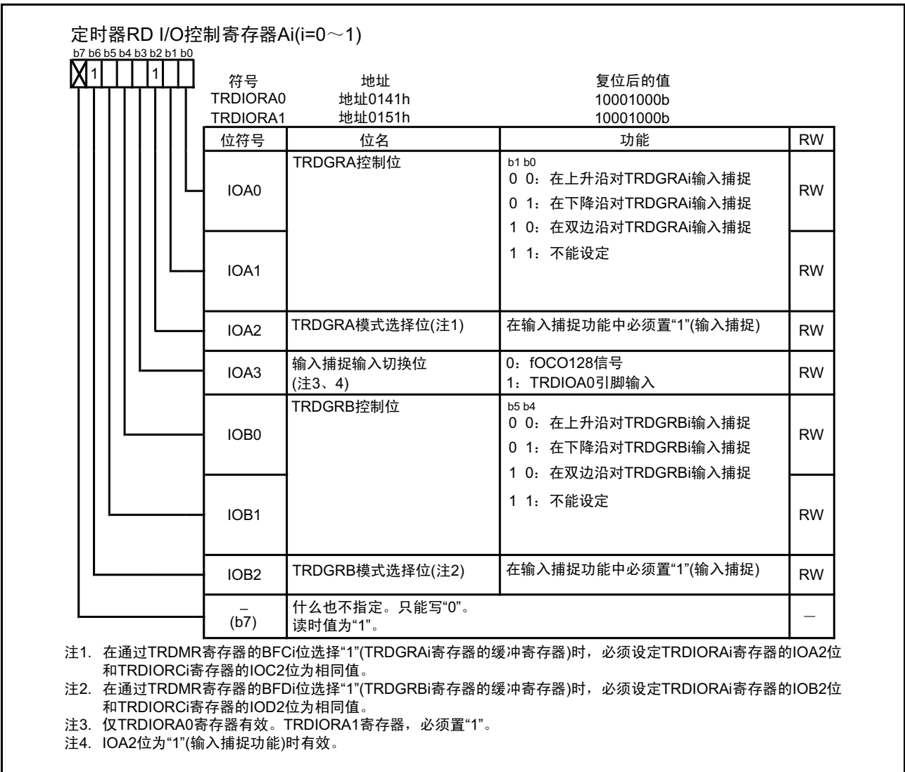
图 15.75 输入捕捉功能时的 TRDIORA0 ~ TRDIORA1 寄存器
