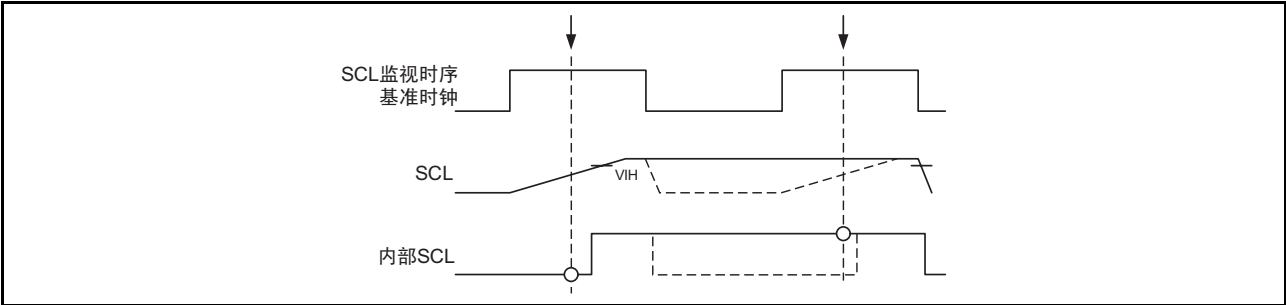
图 17.50 位同步电路的时序
