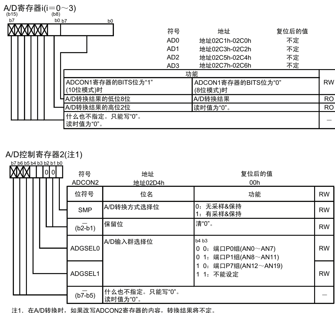
图 19.2 AD0 ~ AD3、ADCON2 寄存器
