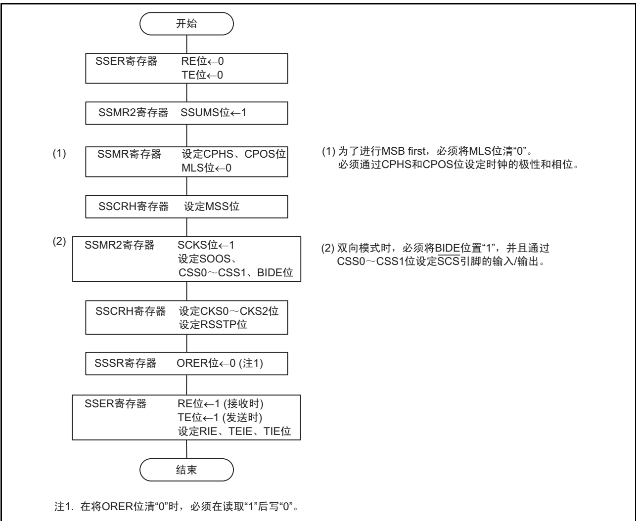
图 17.19 4 线方式总线通信模式的初始化
