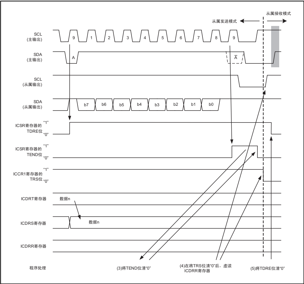
图 17.39 从属发送模式的运行时序（I 2 C 总线接口模式）（2）
