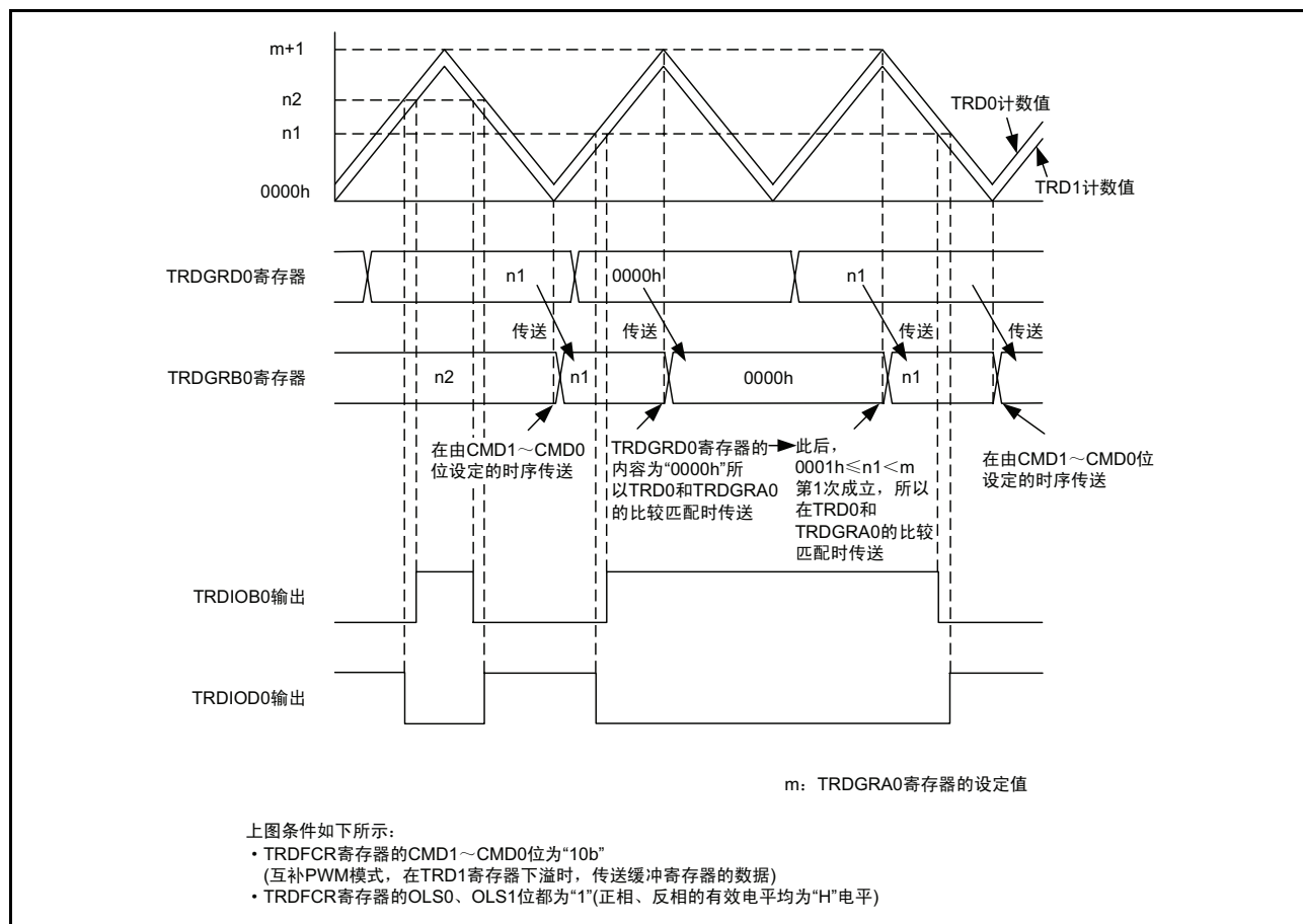
图 15.151 互补 PWM 模式时的缓冲寄存器的值为“0000h”时的运行例
