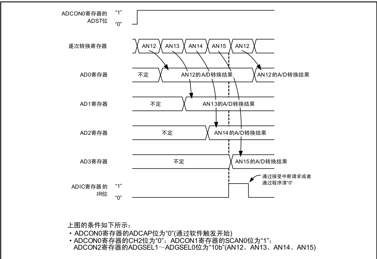
图 19.10 重复扫描模式时的运行示例
