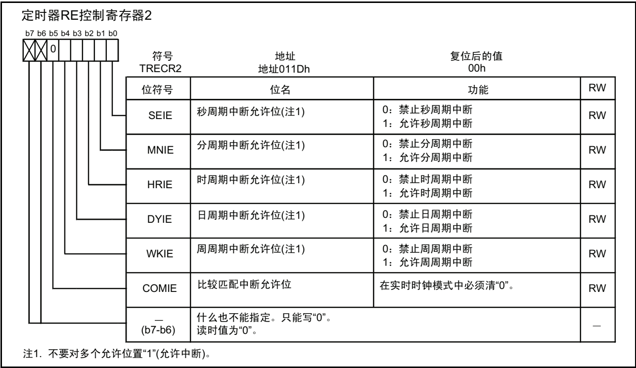
图 15.159 实时时钟模式时的 TREC2 寄存器
