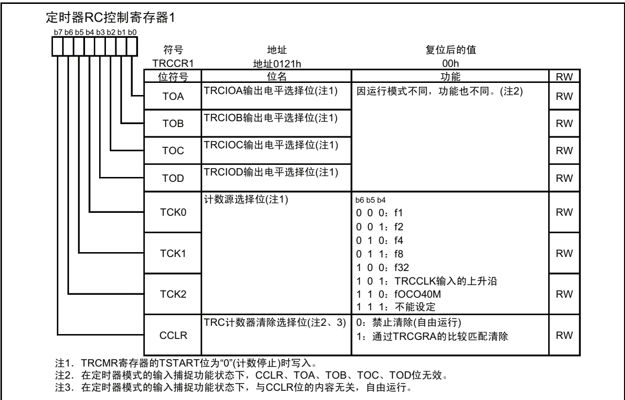
图 15.29 TRCCR1 控制寄存器
