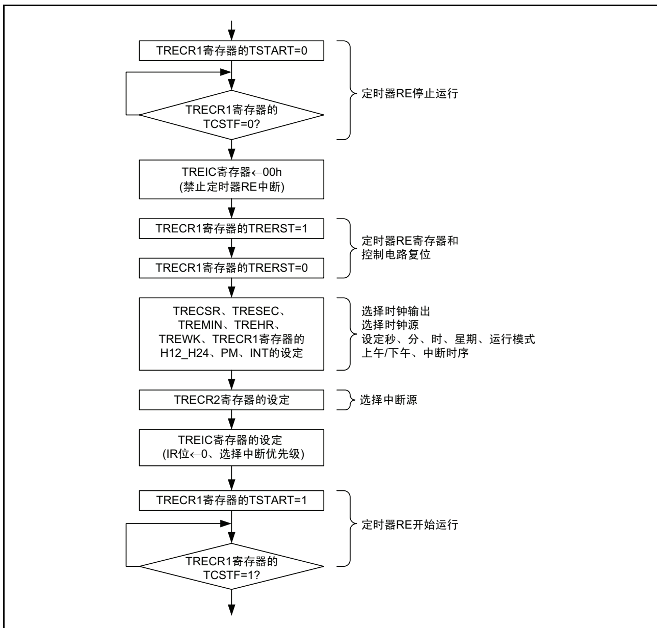
图 15.169 实时时钟模式时的设定例
