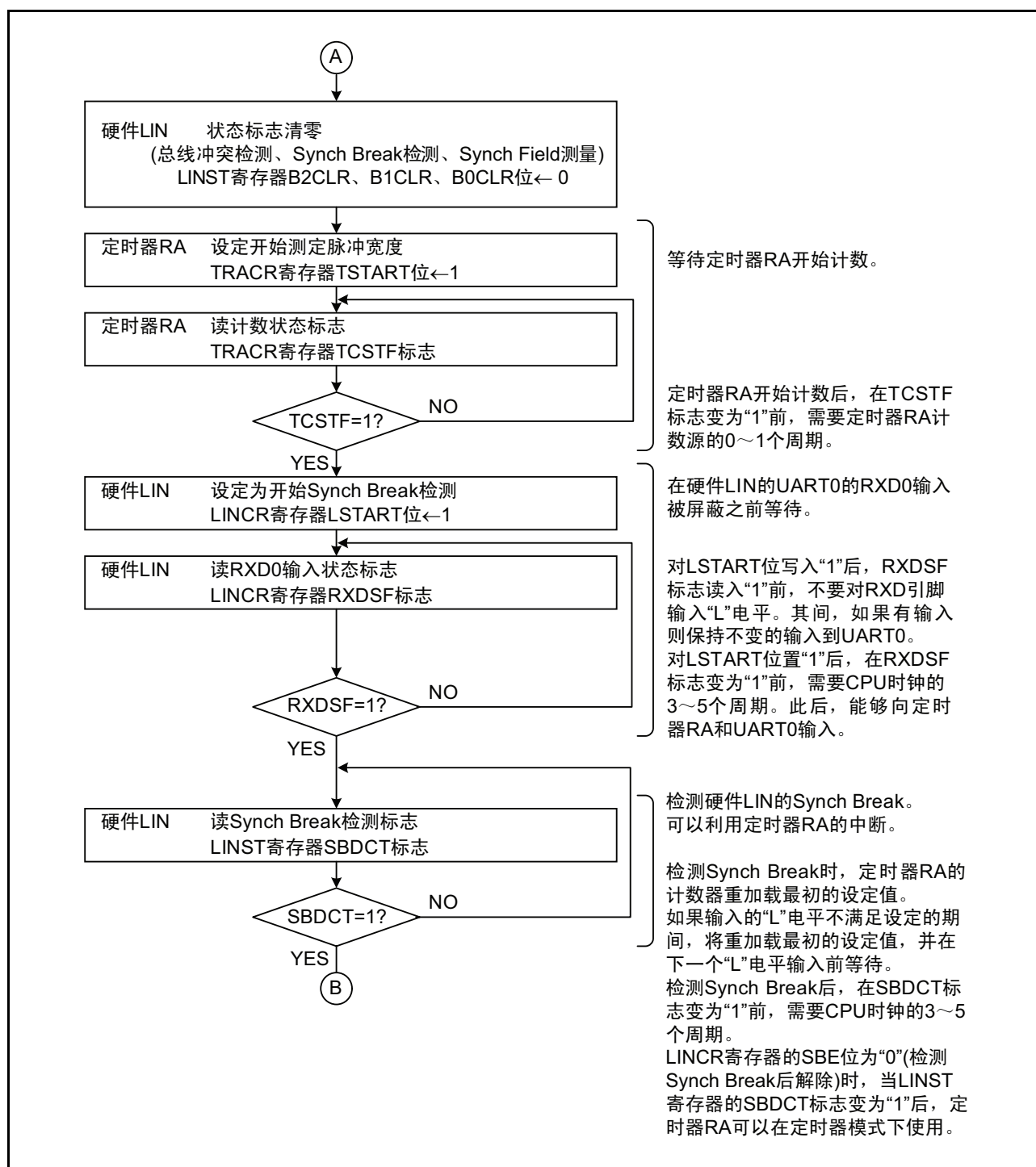
图 18.9 接收头字段的流程图的例子 (2)
