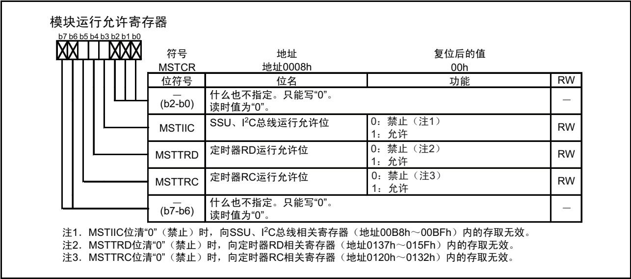
图 15.114 MSTCR 寄存器
