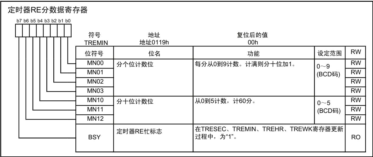
图 15.154 实时时钟模式时的 TREMIN 寄存器
