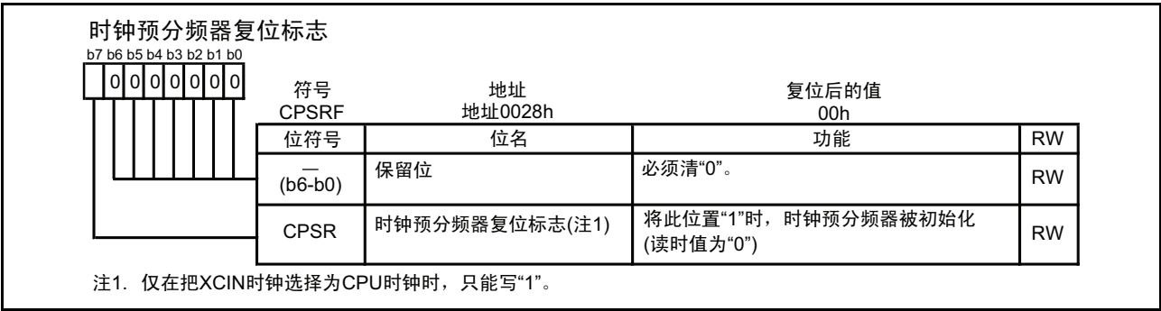
图 11.8 CPSRF 寄存器
