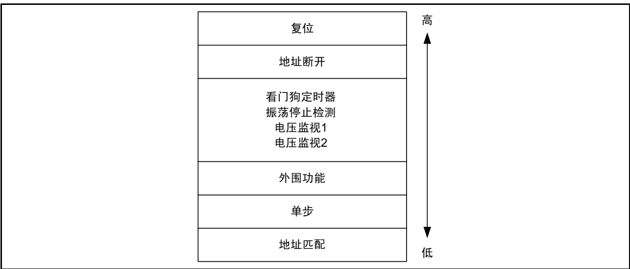
图 13.10 硬件中断的中断优先权
