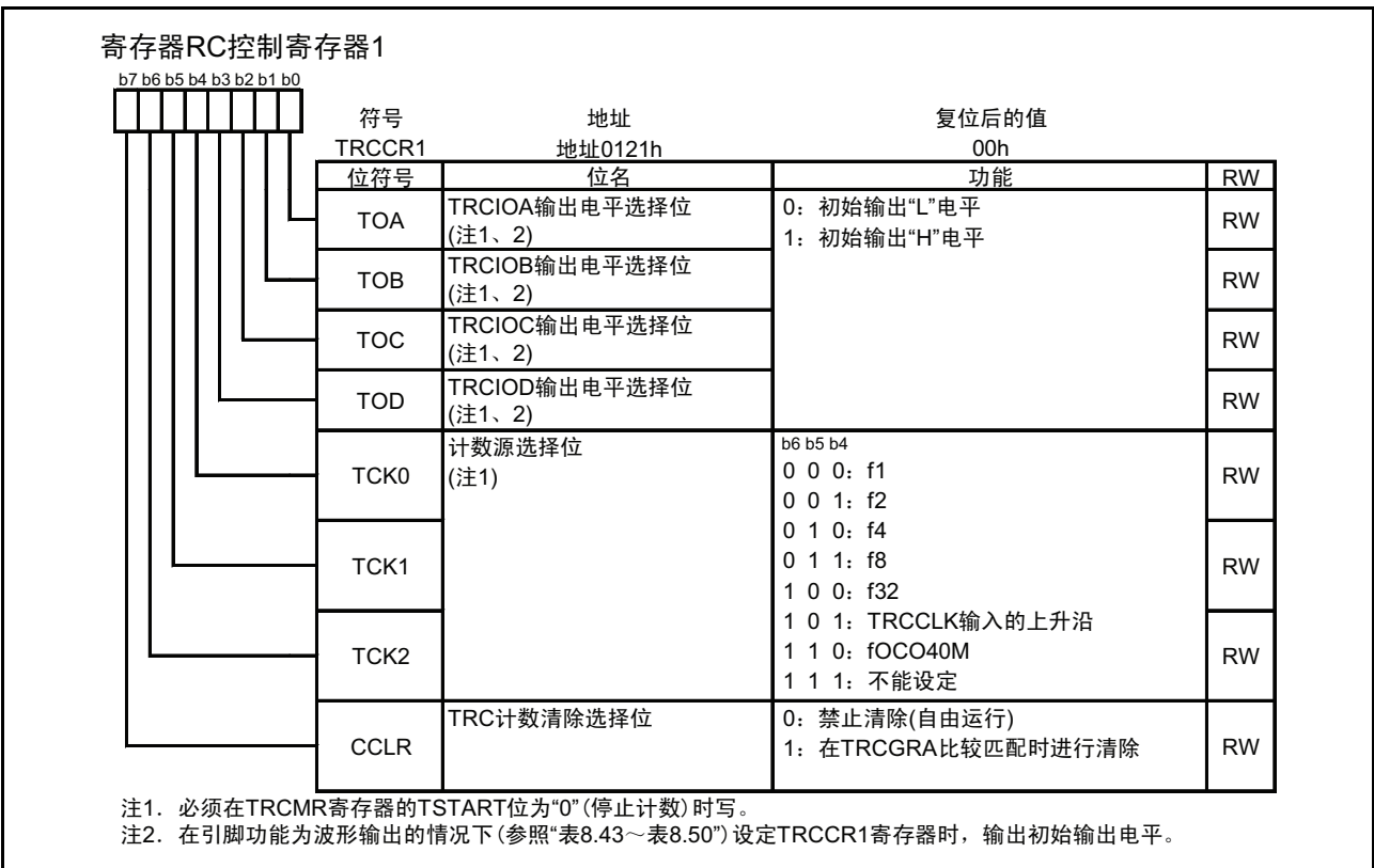
图 15.50 输出比较功能时的 TRCCR1 寄存器
