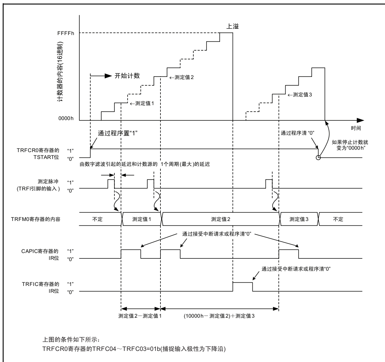
图 15.177 输入捕捉模式的运行例
