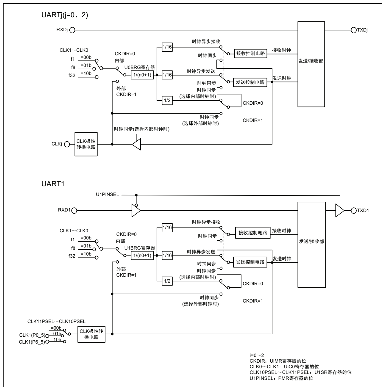
图 16.1 UARTi (i=0 ~ 2) 框图
