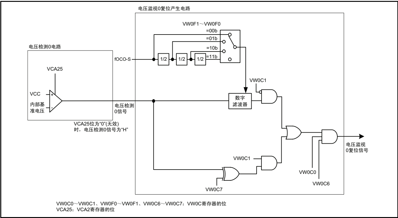
图 7.2 电压监视 0 复位产生电路的框图
