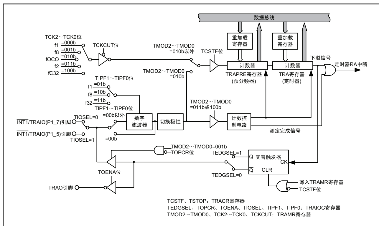
图 15.1 定时器 RA 框图
