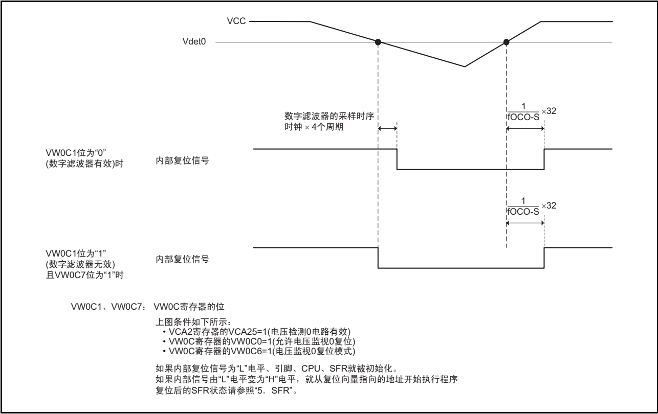
图 7.9 电压监视 0 复位的运行例
