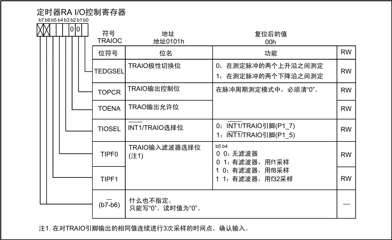
图 15.10 脉冲周期测定模式时的 TRAIOC 寄存器
