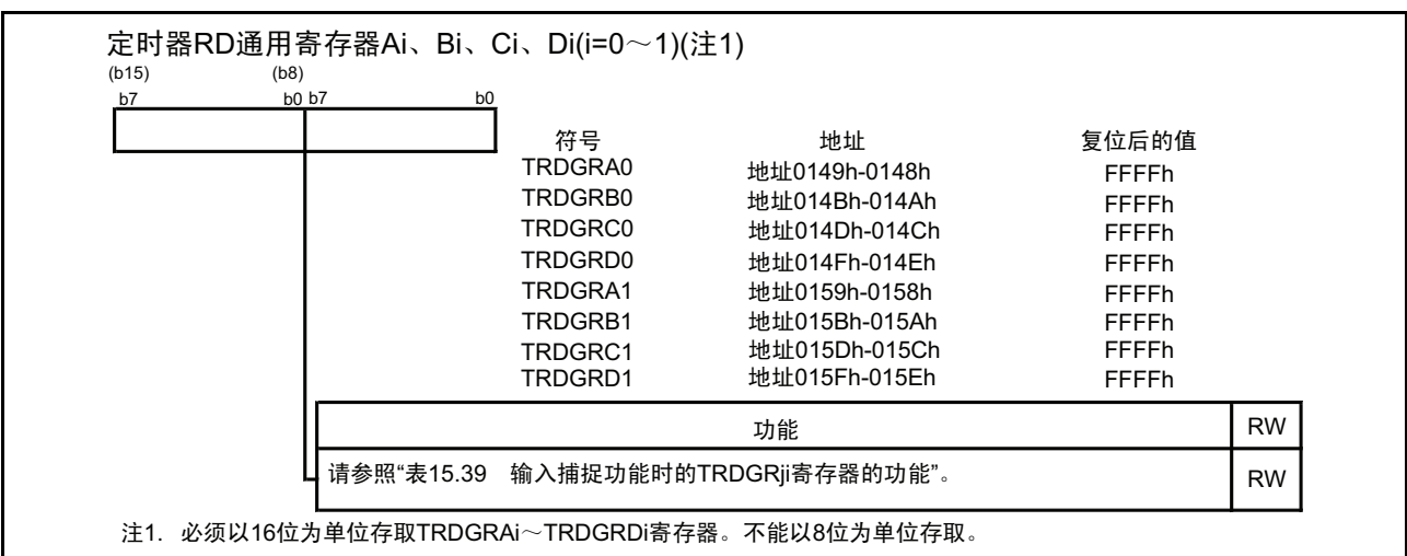
图 15.80 输入捕捉功能时的 TRDGRAi、TRDGRBi、TRDGRCi、TRDGRDi 寄存器
