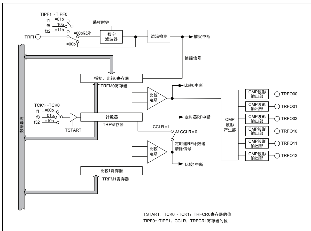
图 15.170 定时器 RF 的框图
