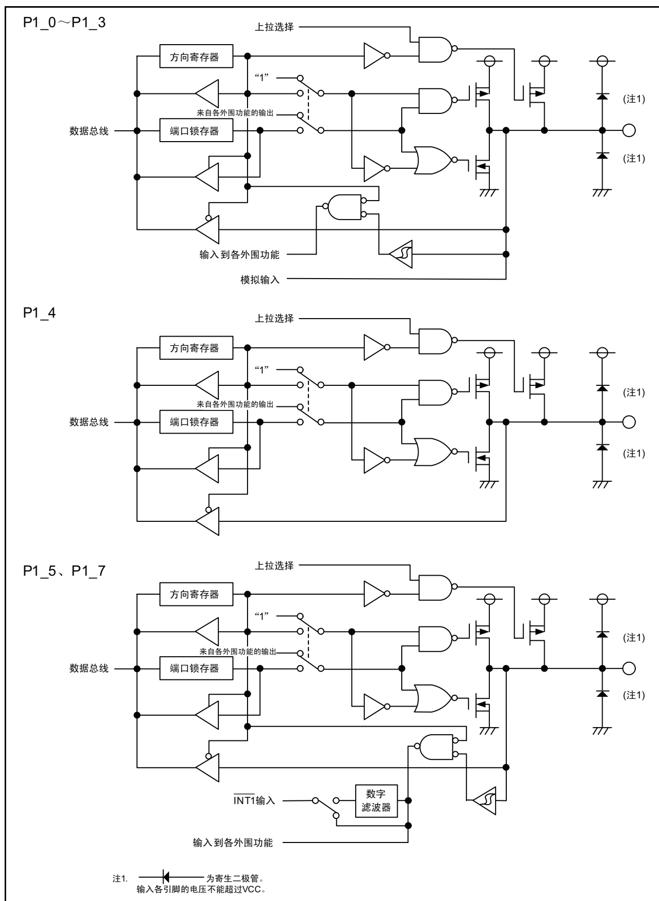
图 8.2 可编程输入 / 输出端口的结构 (2)
