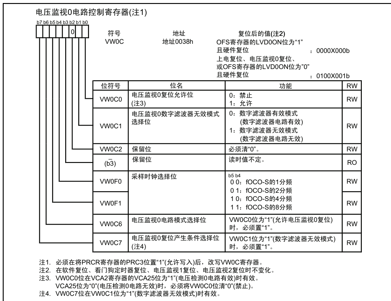
图 7.6 VW0C 寄存器
