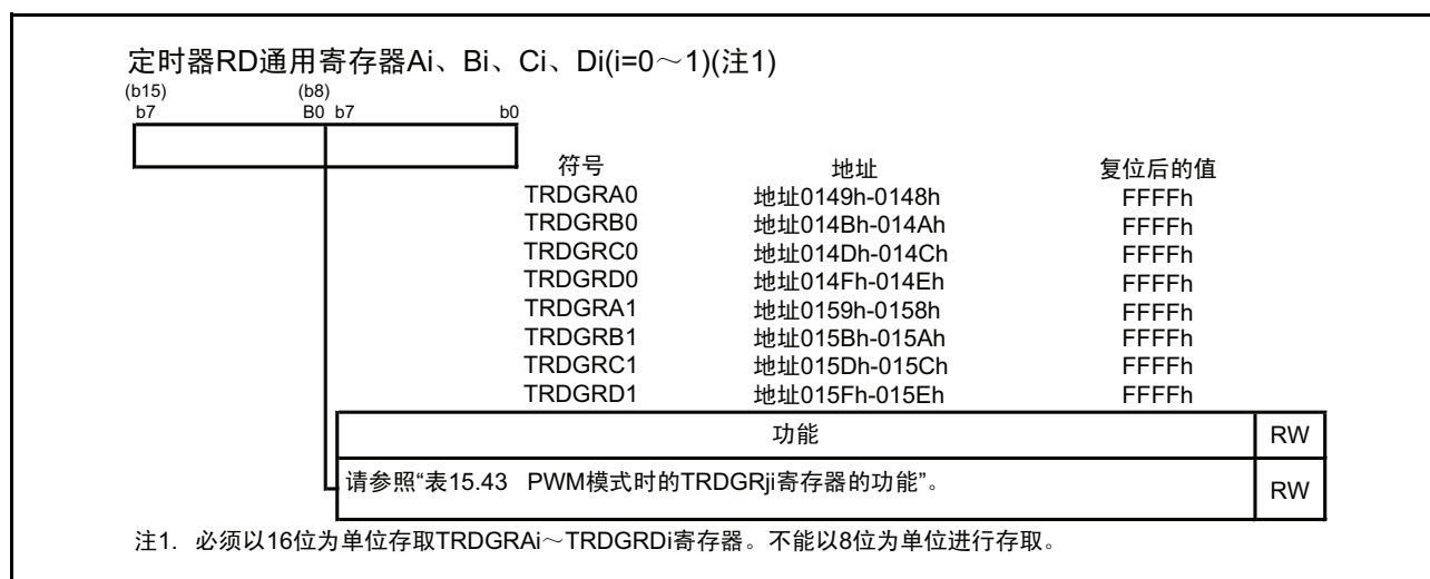
图 15.110 PWM 模式时的 TRDGRAi、TRDGRBi、TRDGRCi、TRDGRDi 寄存器
