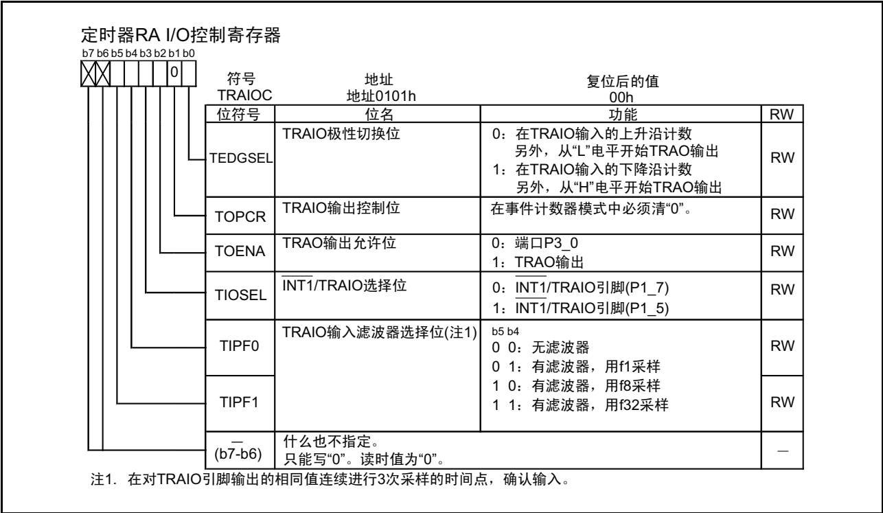
图 15.7 事件计数器模式时的 TRAIOC 寄存器
