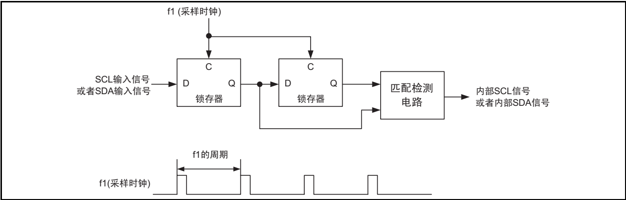
图 17.49 噪声消除电路的框图
