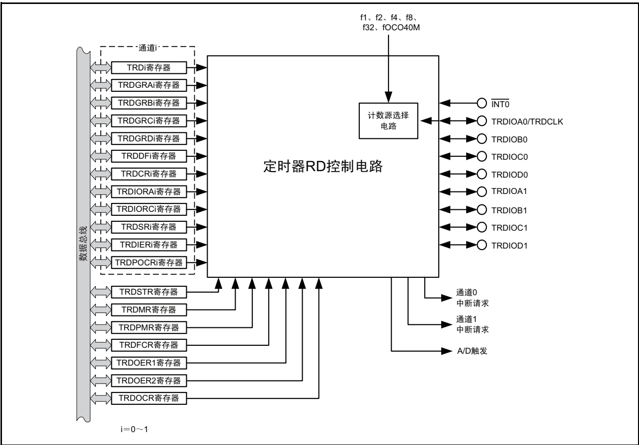
图 15.62 定时器 RD 的框图
