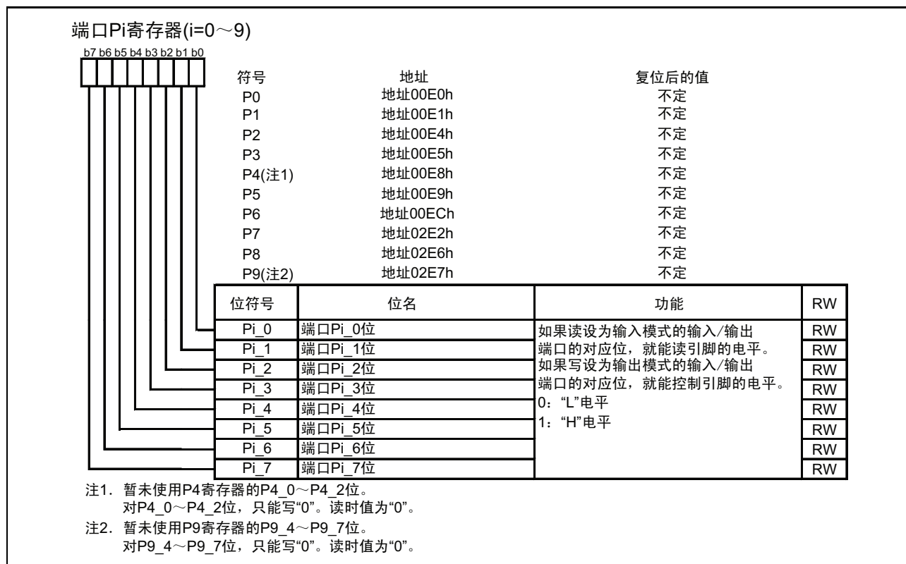
图 8.14 Pi 寄存器
