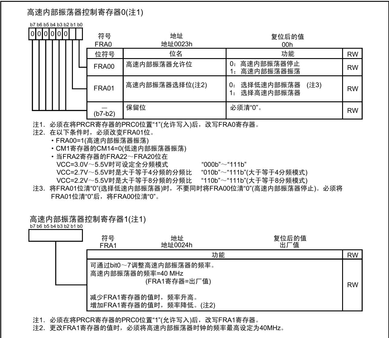
图 11.6 FRA0、FRA1 寄存器
