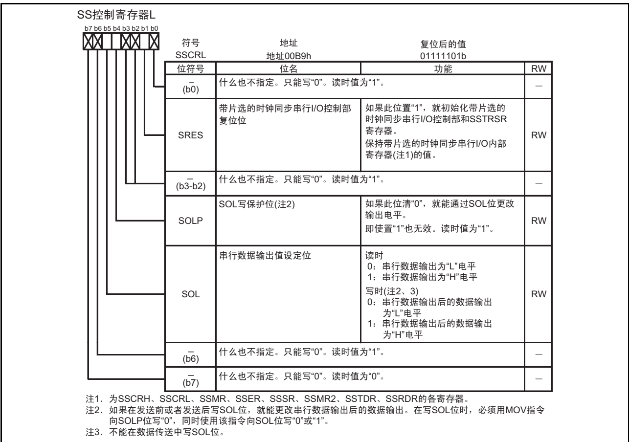
图 17.4 SSCRL 寄存器
