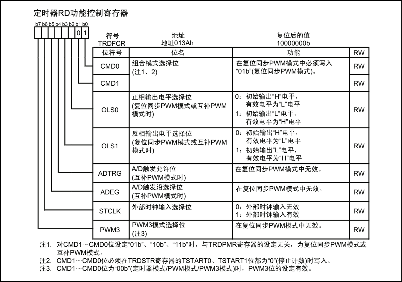
图 15.116 复位同步 PWM 模式时的 TRDFCR 寄存器
