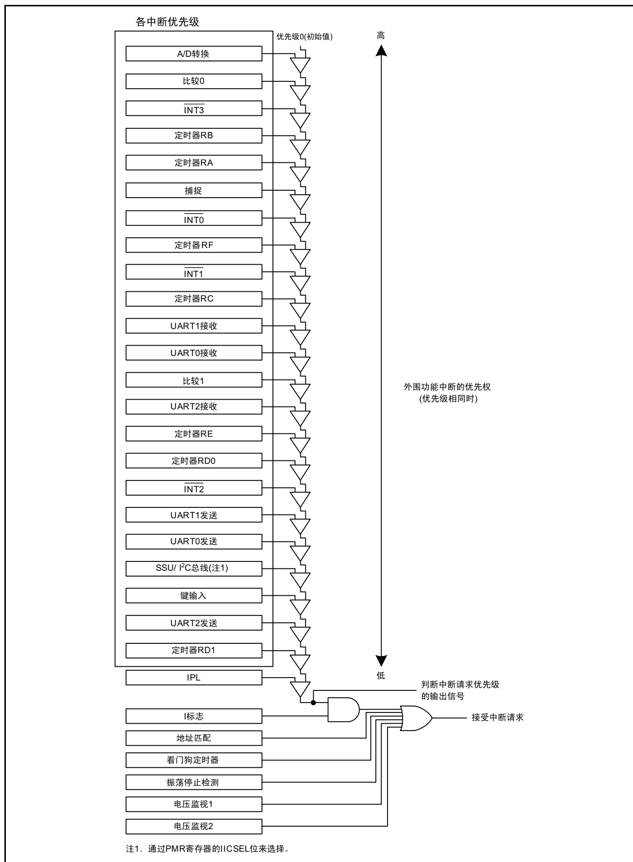
图 13.11 中断优先级判定电路
