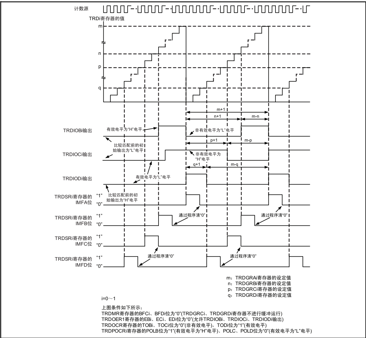
图 15.111 PWM 模式的运行例
