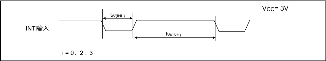
图 22.17 V_{CC}=3V 时的外部中断 \overline{\text{INTi}} 输入时序
