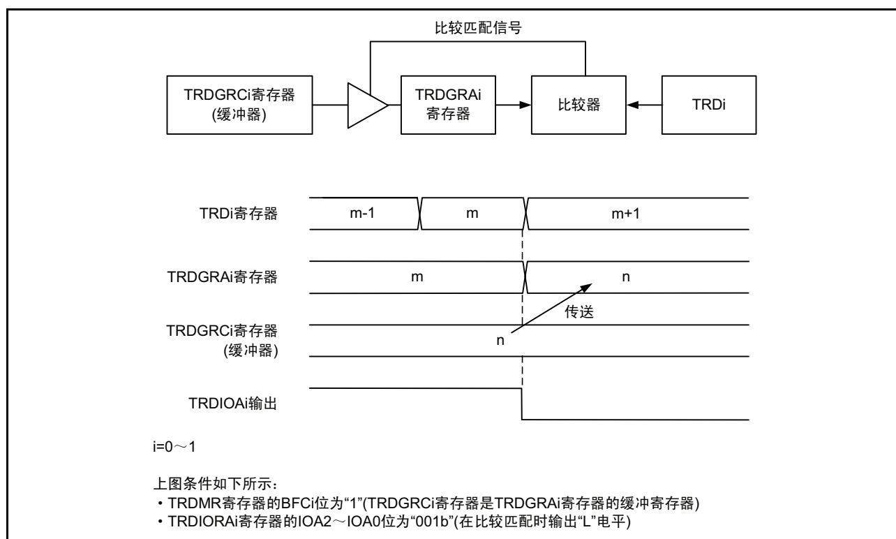
图 15.65 输出比较功能的缓冲器运行
