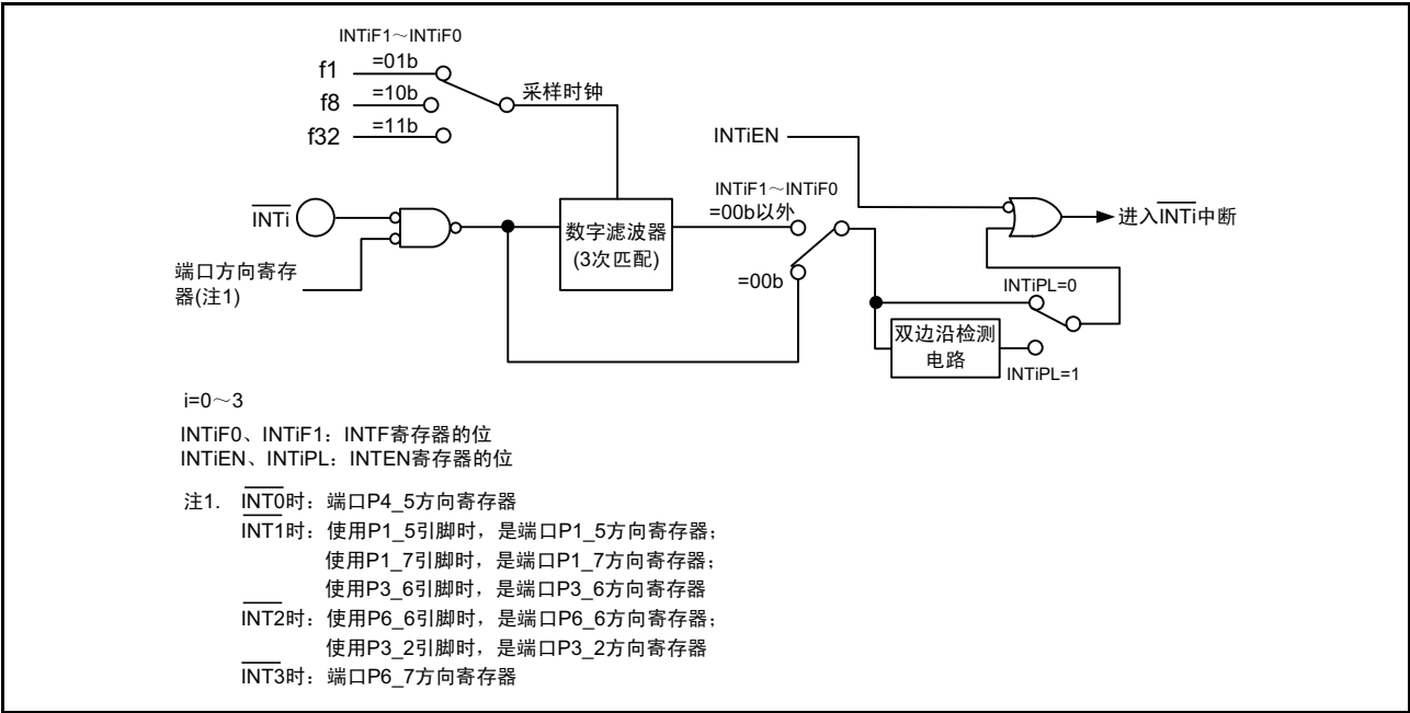
图 13.16 \overline{\text{INTi}} 输入滤波器的结构
