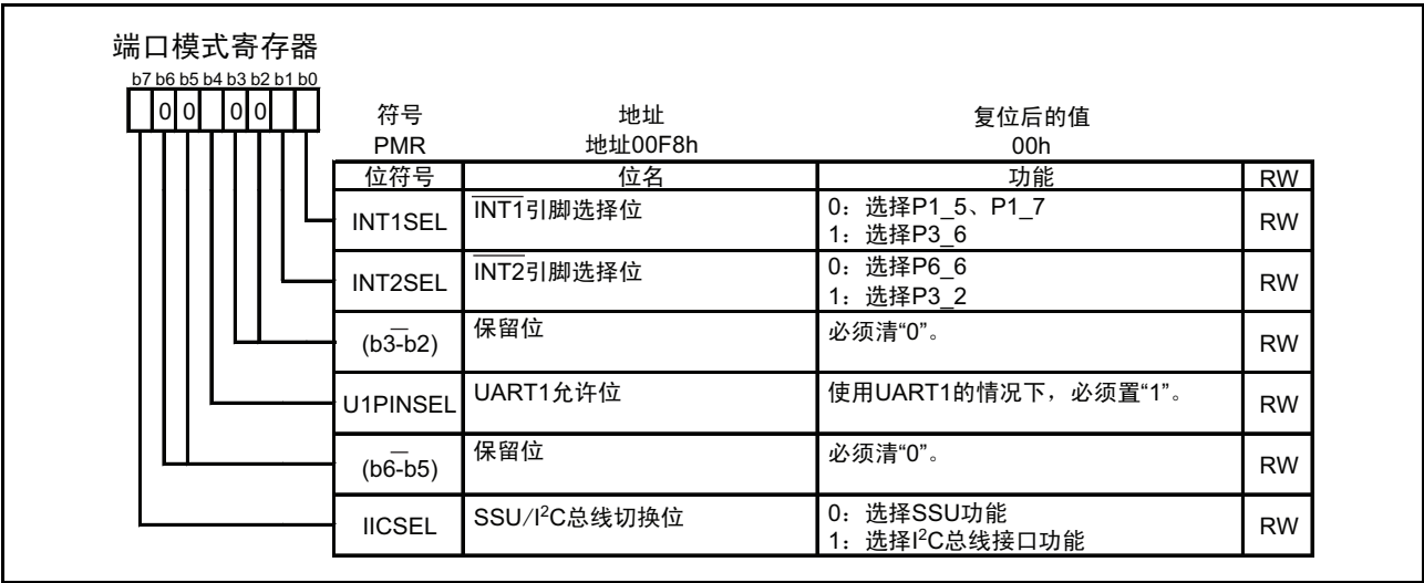
图 13.12 PMR 寄存器
