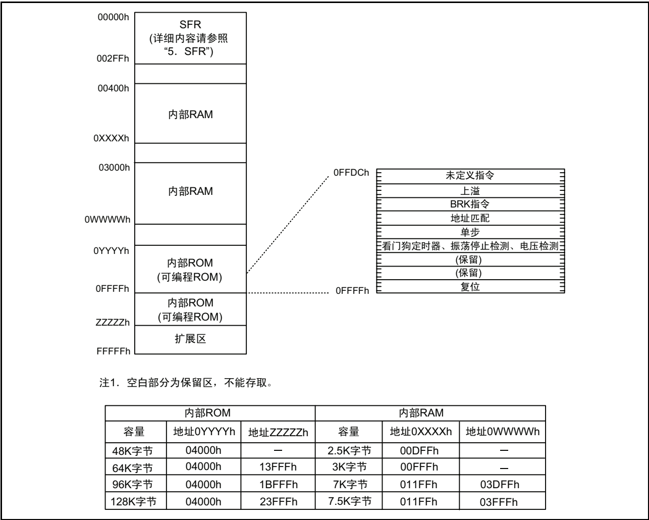
图 4.1 R8C/2C 群的存储器分配图
