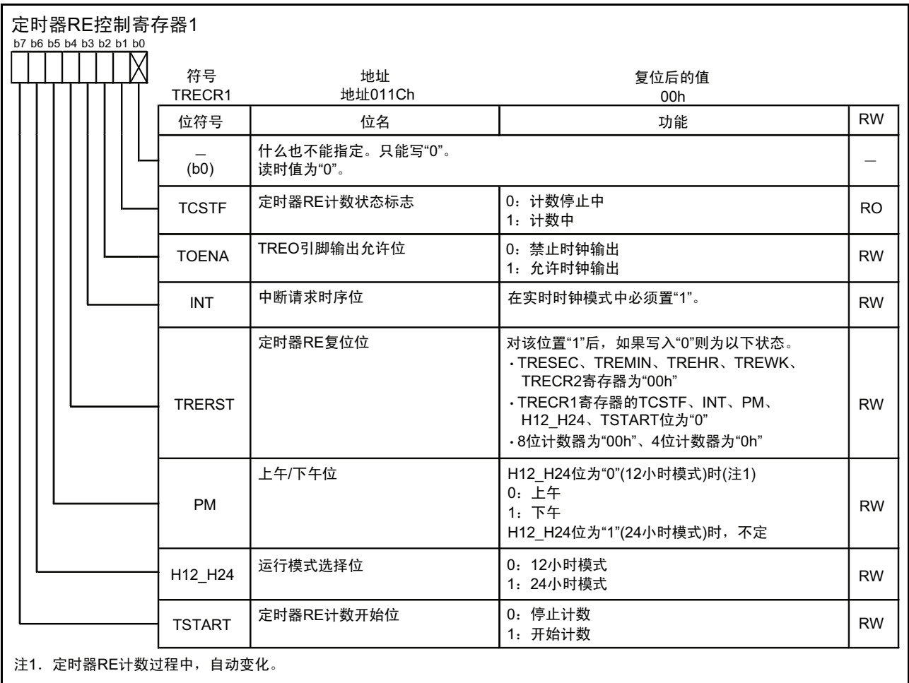
图 15.157 实时时钟模式时的 TRECR1 寄存器
