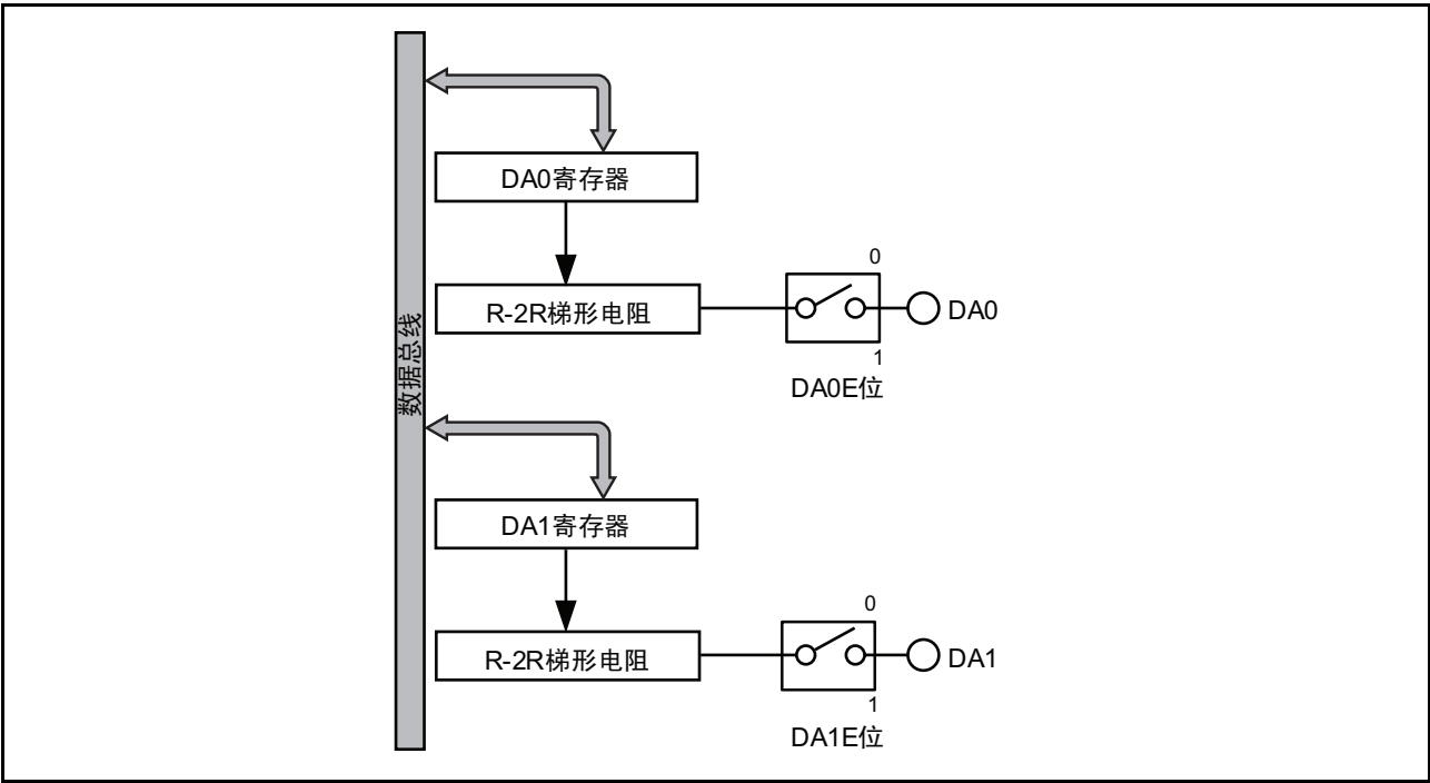
图 20.1 D/A 转换器框图
