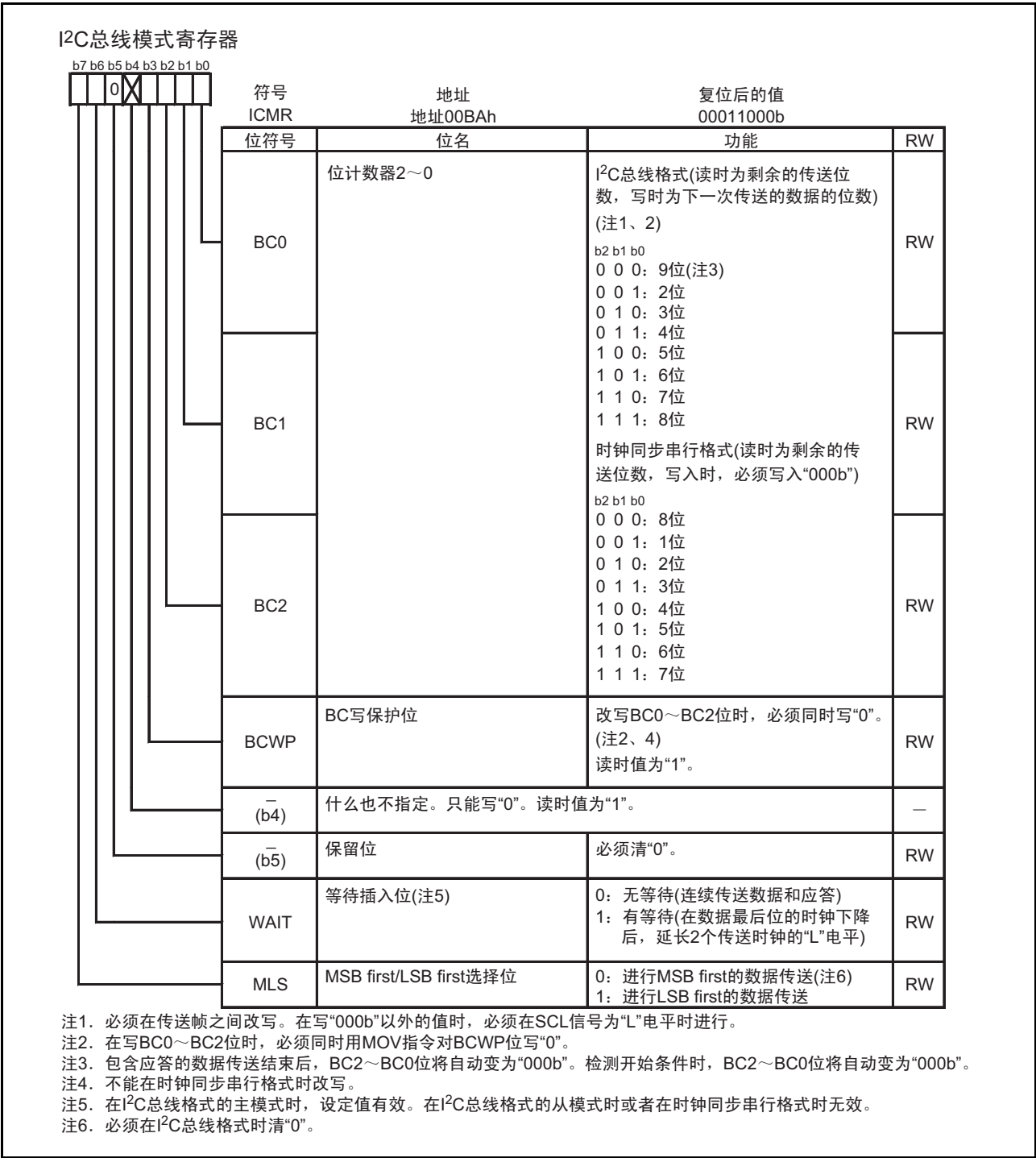
图 17.28 ICMR 寄存器
