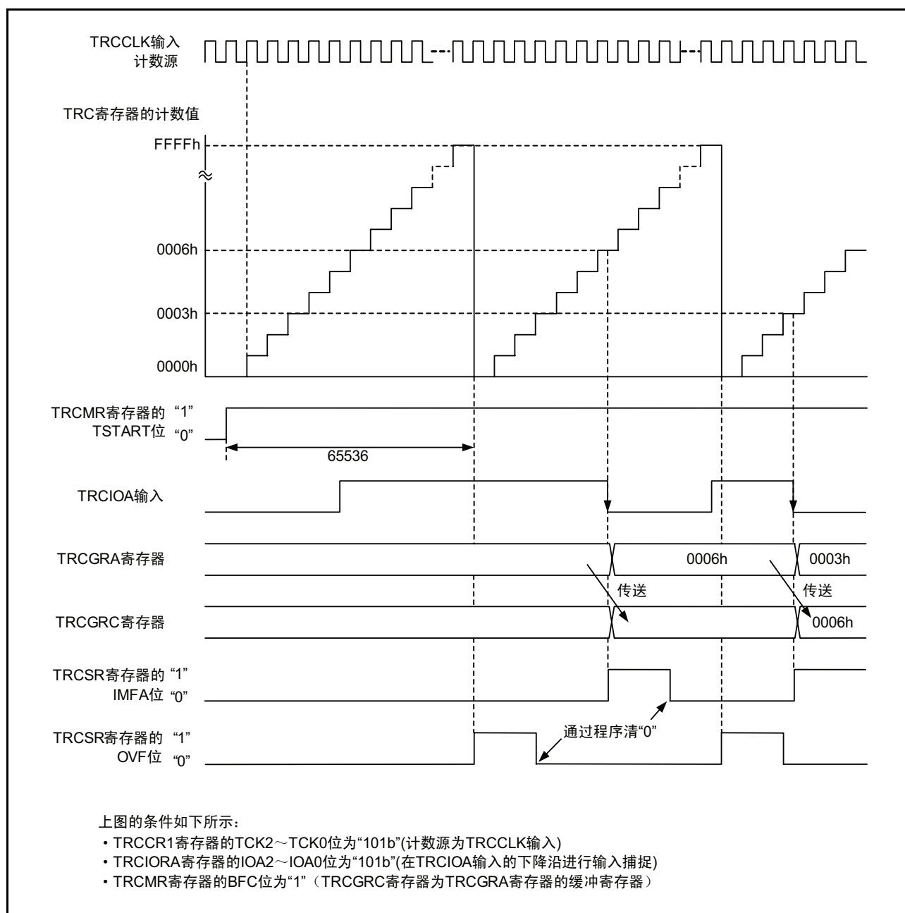
图 15.46 输入捕捉功能的运行例
