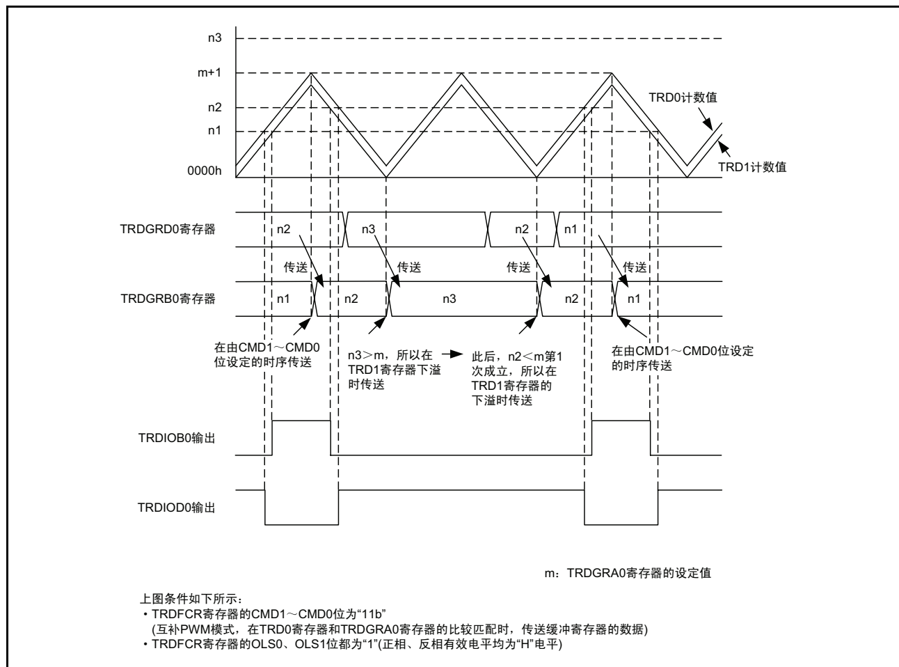
图 15.150 互补 PWM 模式时的缓冲寄存器的值 \geq TRDGRA0 寄存器的值时的运行例
