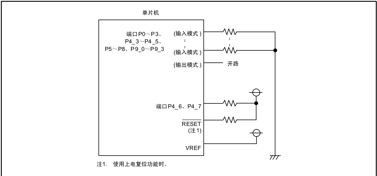
图 8.18 未使用引脚的处理例
