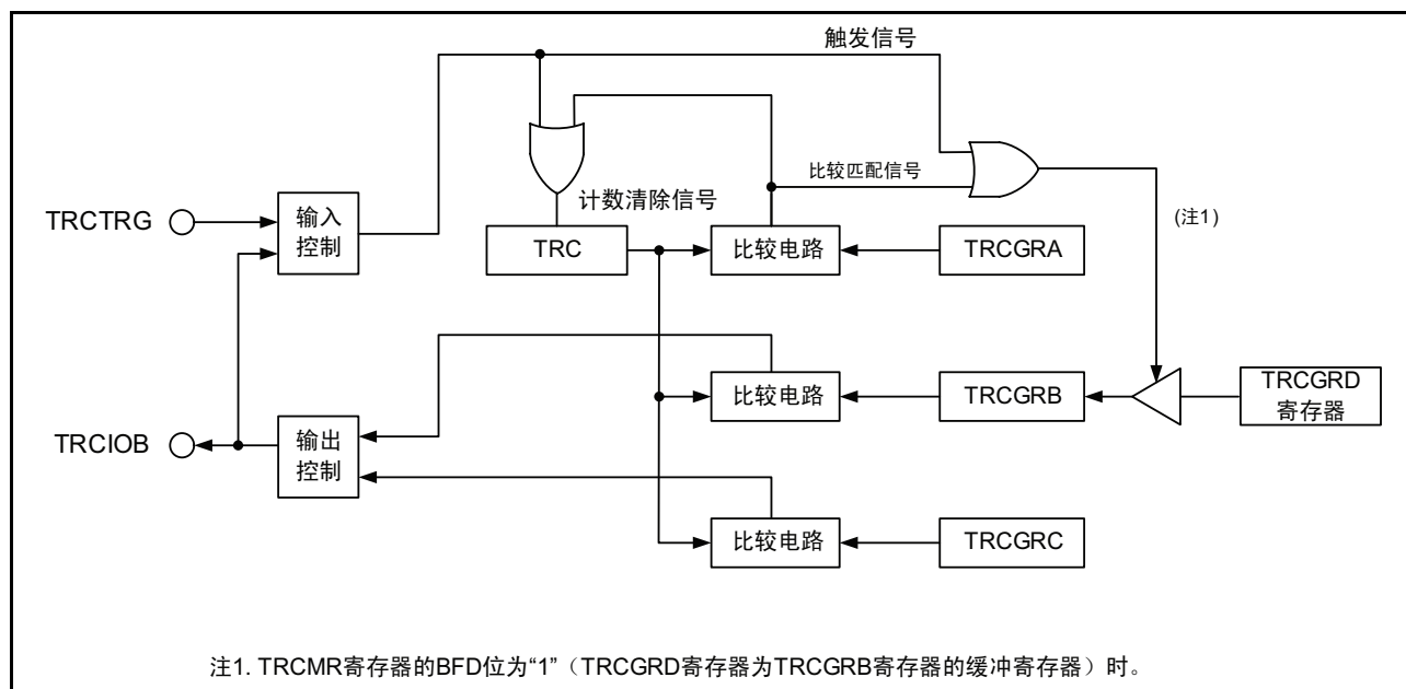
图 15.56 PWM2 模式的框图
