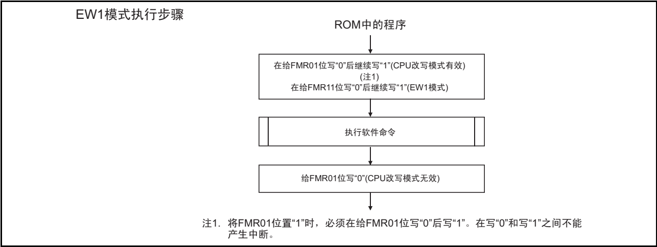
图 21.10 EW1 模式的设定和解除方法
