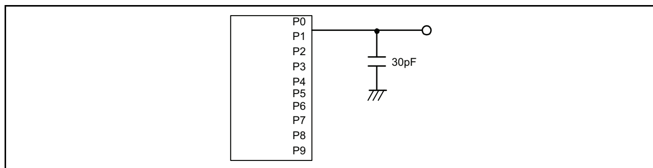
图 22.1 端口 P0 ~ P9 的时序测定电路
