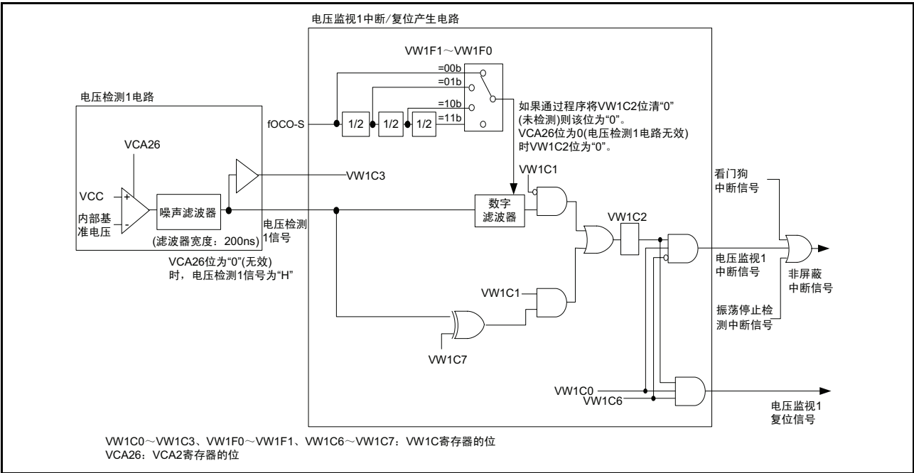
图 7.3 电压监视 1 中断 / 复位产生电路的框图
