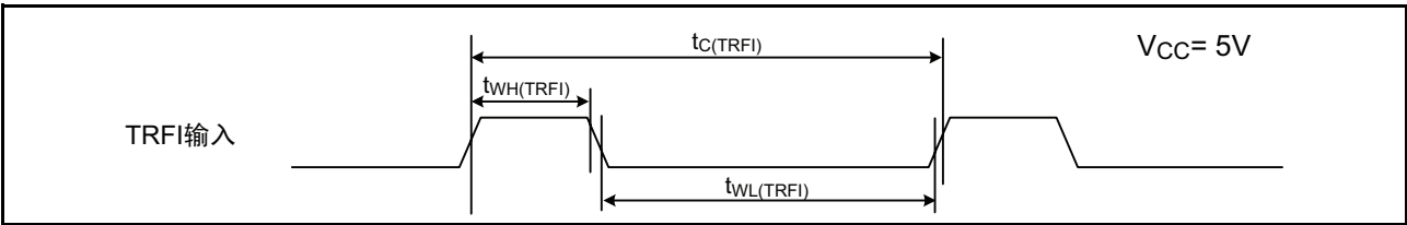
图 22.10 V CC =5V 时的 TRFI 输入时序
