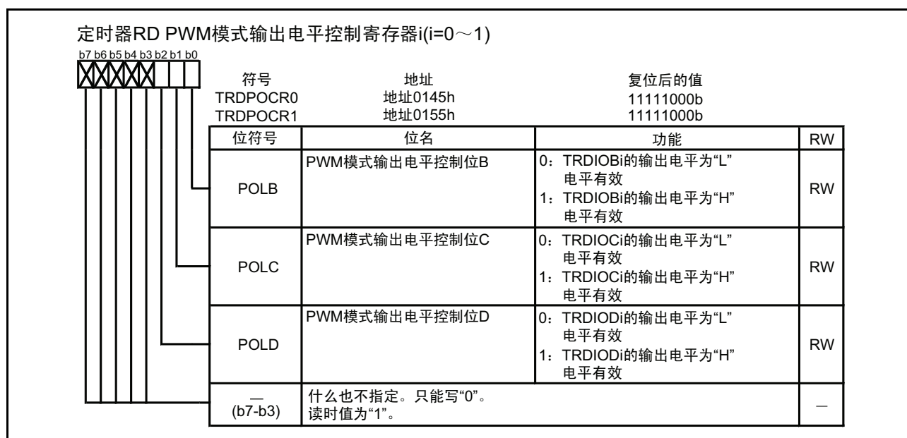
图 15.108 PWM 模式时的 TRDPOCR0 ~ TRDPOCR1 寄存器
