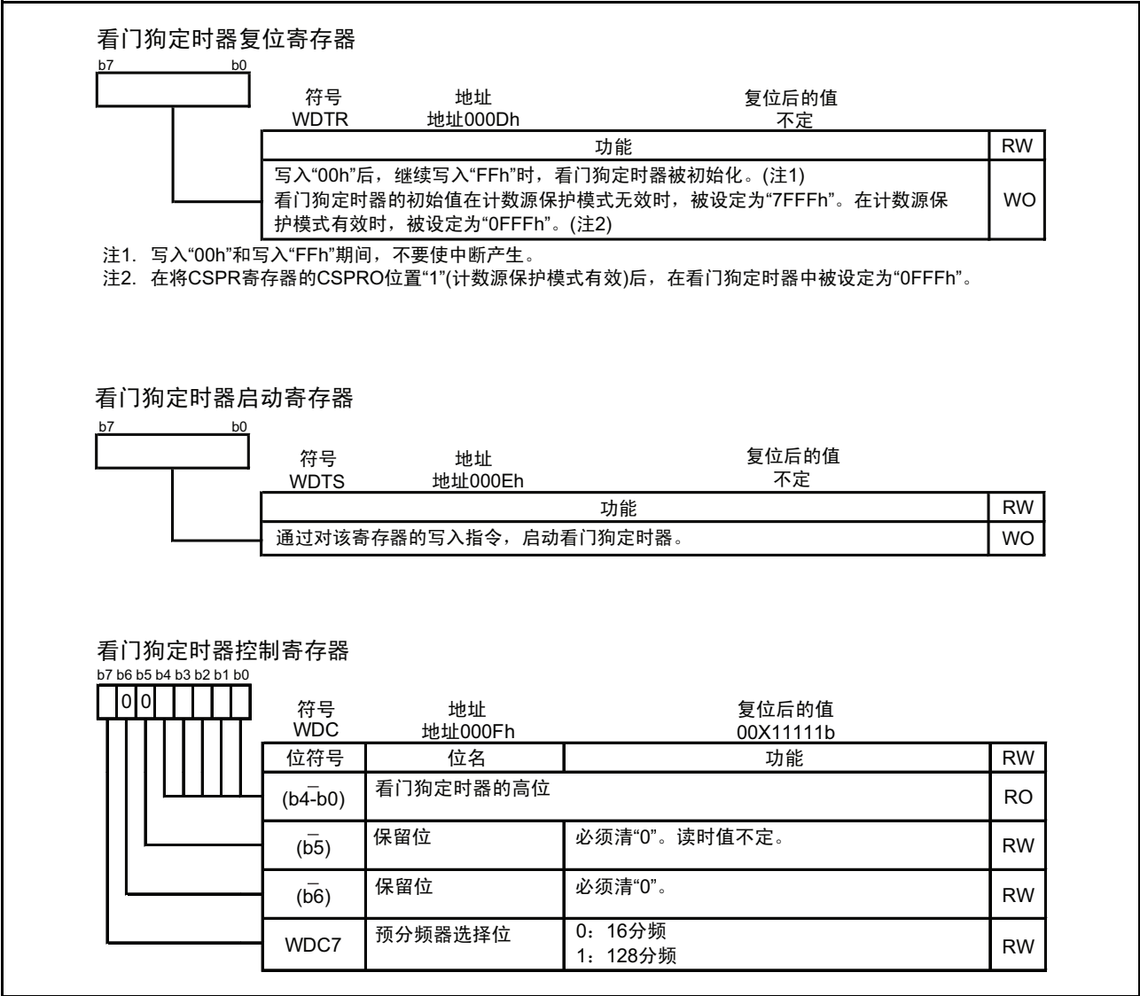
图 14.2 WDTR、WDTS、WDC 寄存器
