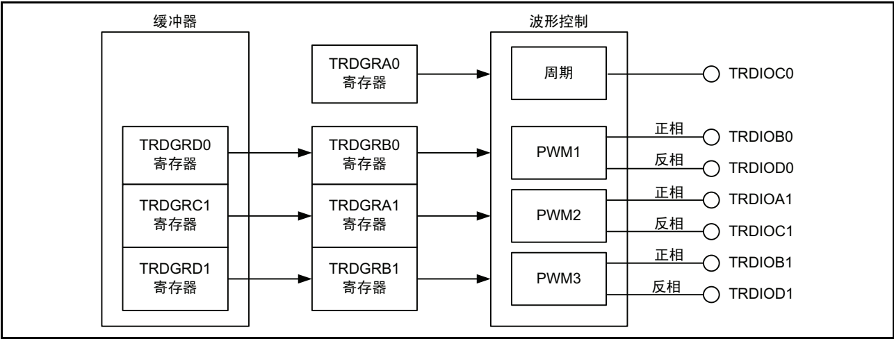
图 15.124 互补 PWM 模式的框图
