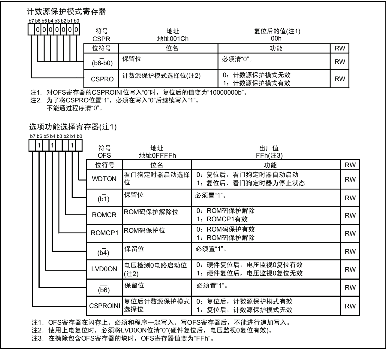
图 14.3 CSPR、OFS 寄存器
