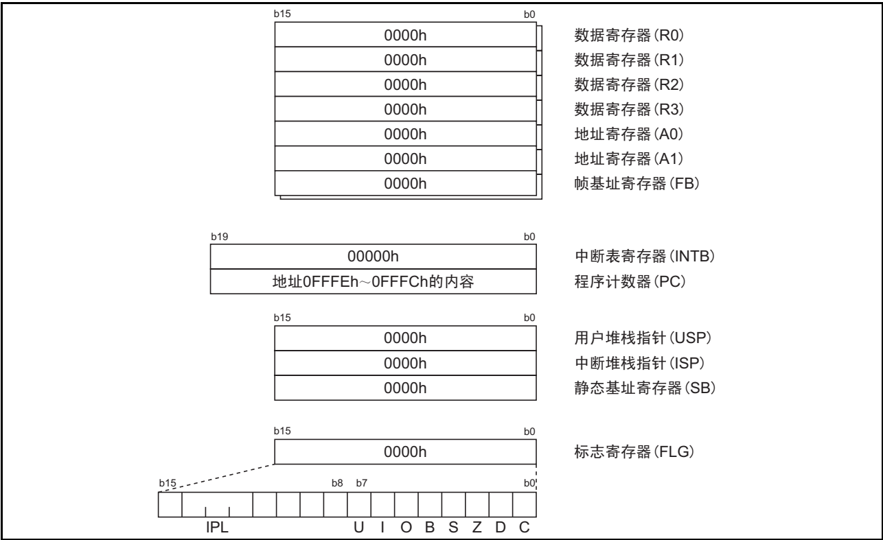
图 6.2 复位后的 CPU 寄存器状态
