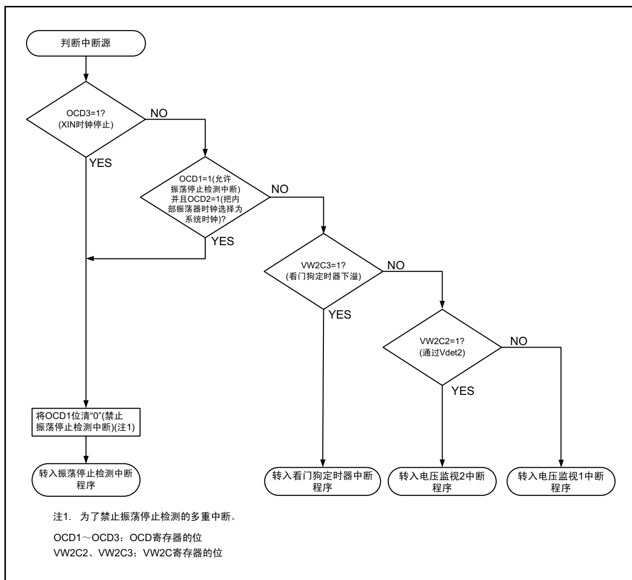
图 11.18 振荡停止检测中断、看门狗定时器中断、电压监视 1 中断和电压监视 2 中断的中断源判断方法的例
