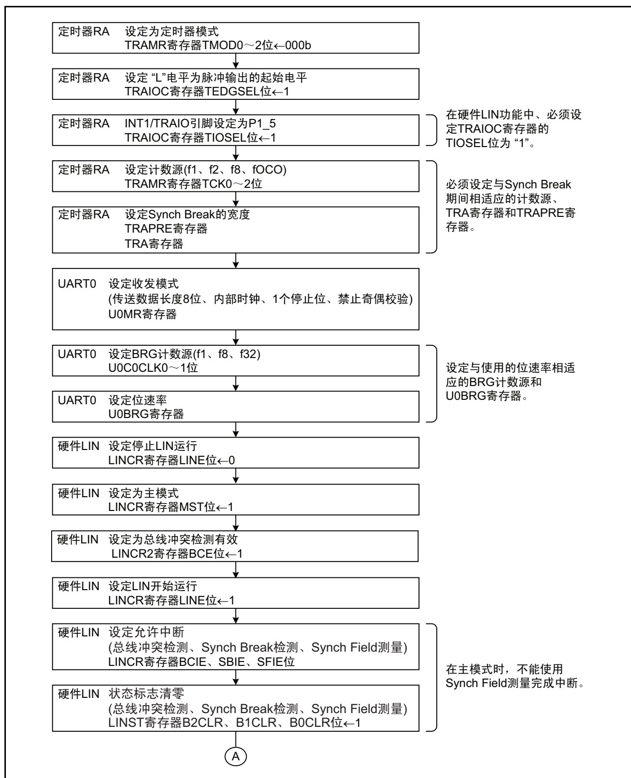
图 18.5 发送头字段的流程图的例子 (1)
