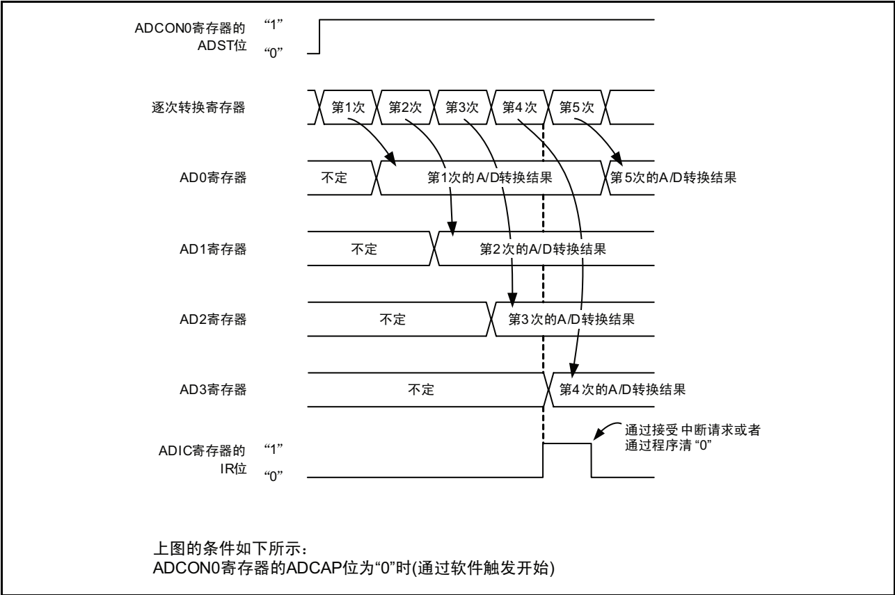
图 19.8 重复模式 1 时的运行例
