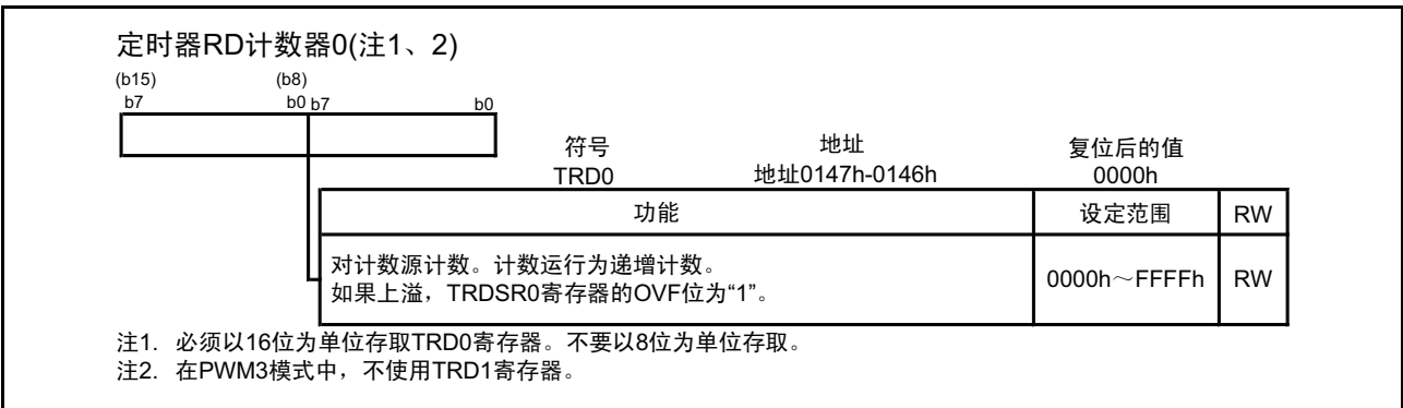
图 15.144 PWM3 模式时的 TRD0 寄存器
