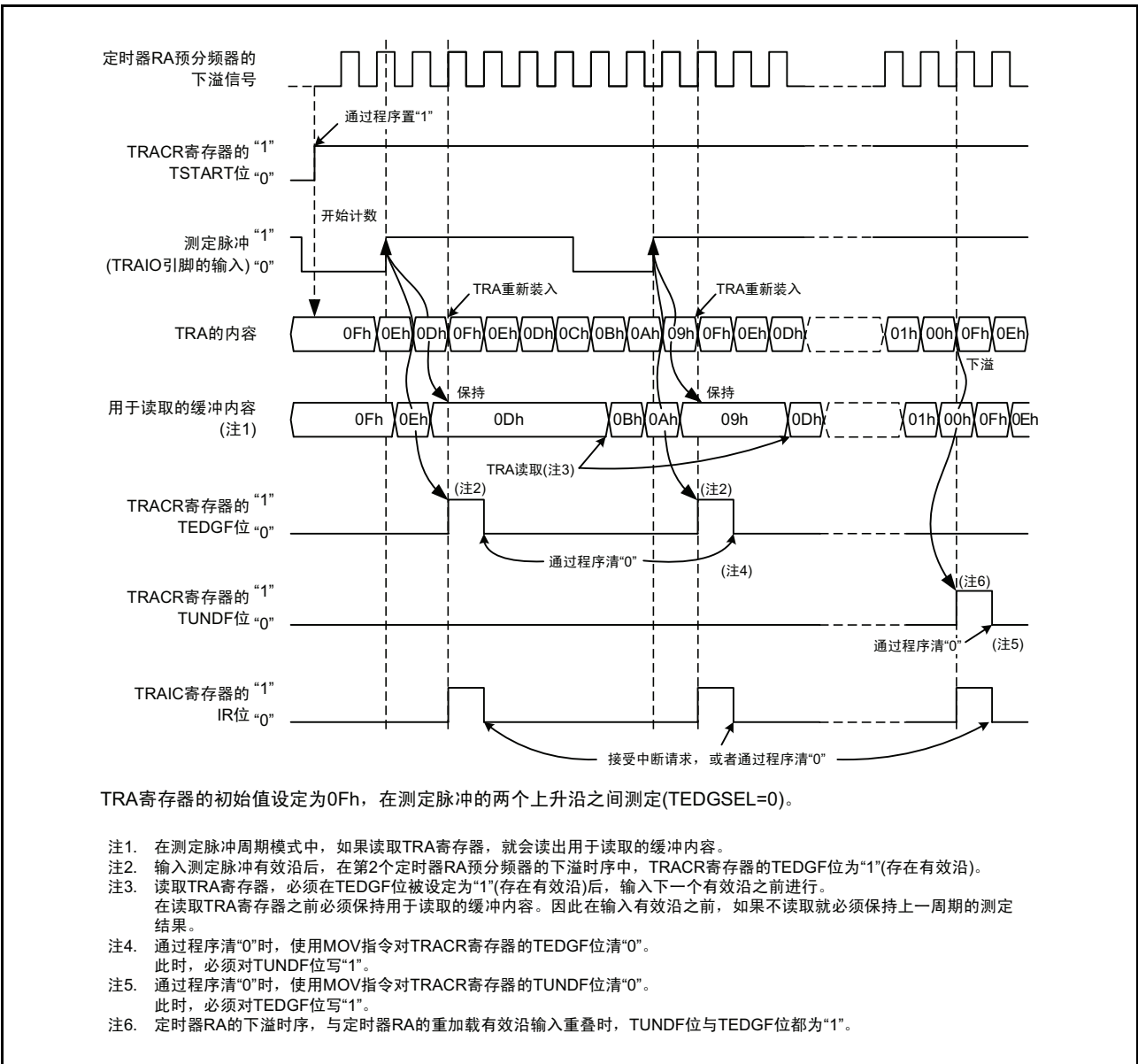
图 15.11 脉冲周期测定模式时的运行例
