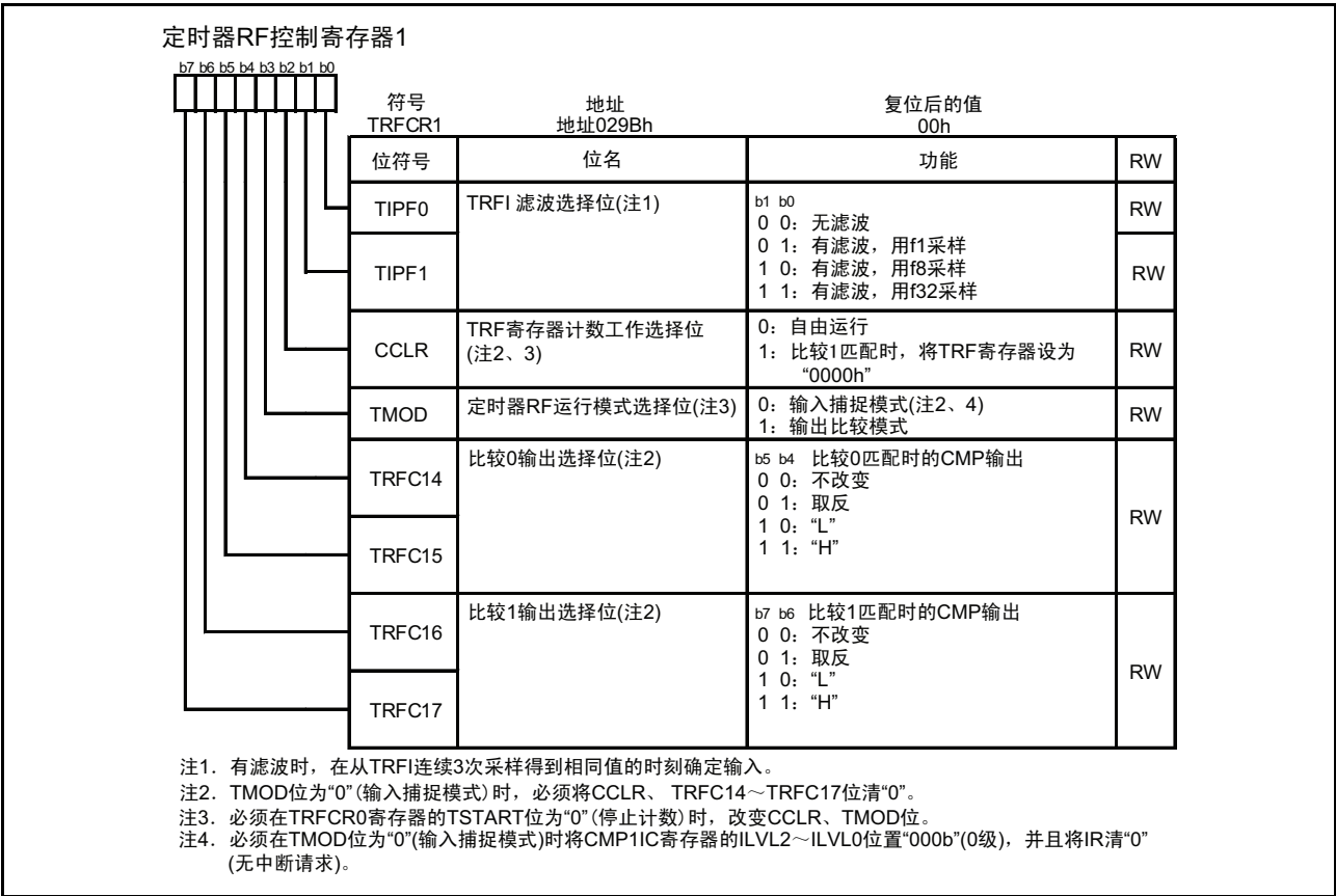
图 15.175 TRFCR1 寄存器
