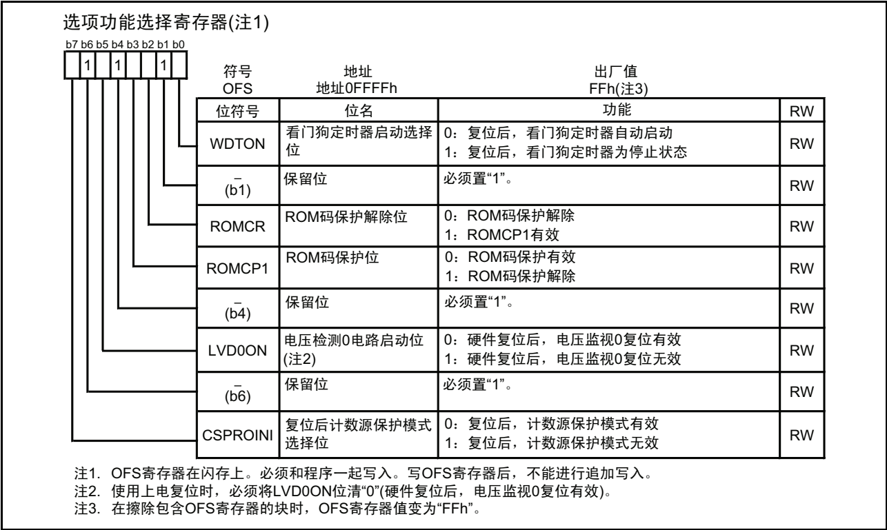
图 21.4 OFS 寄存器
