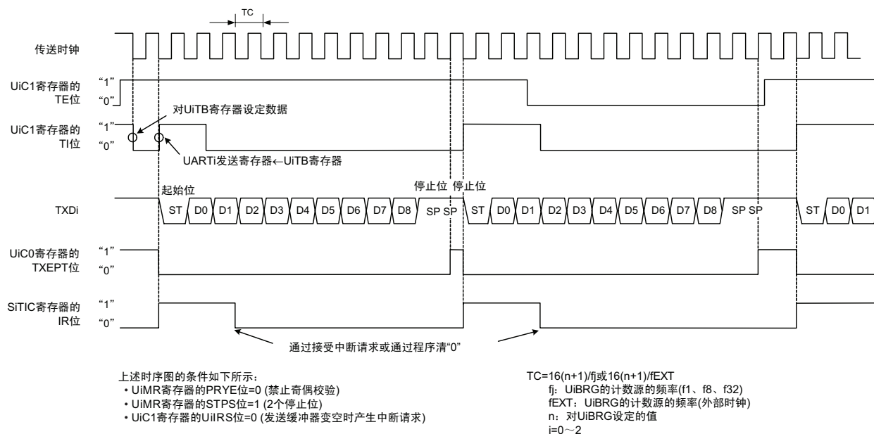
图 16.12 UART 模式时的发送时序
