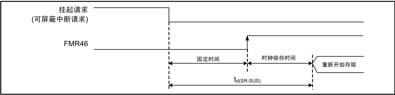
图 22.2 挂起的转移时间
