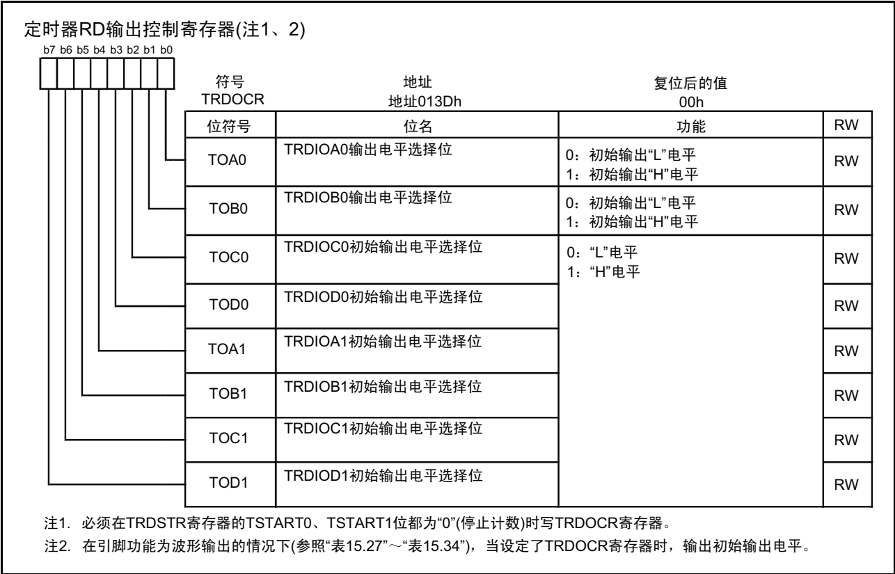
图 15.89 输出比较功能时的 TRDOCR 寄存器
