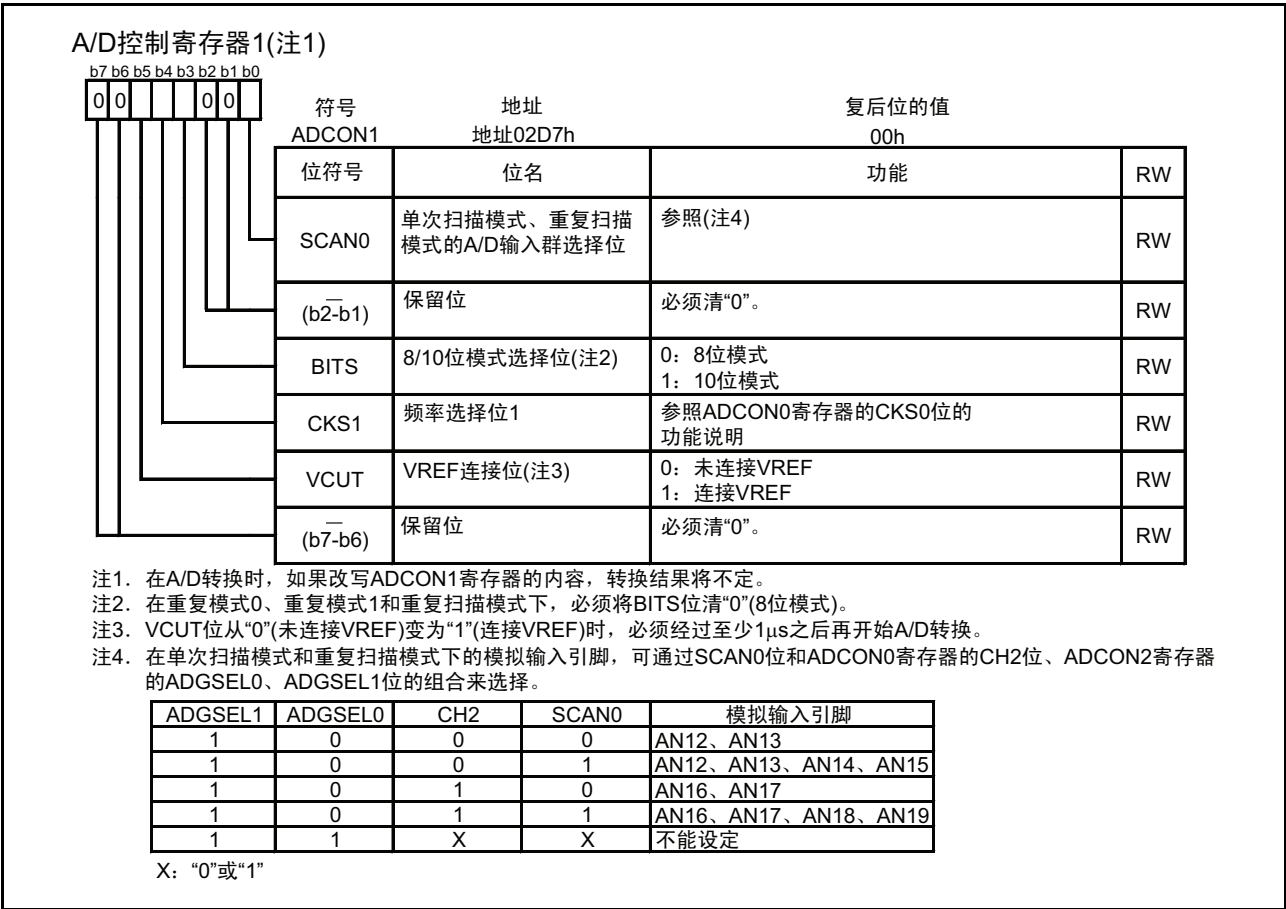
图 19.4 ADCON1 寄存器
