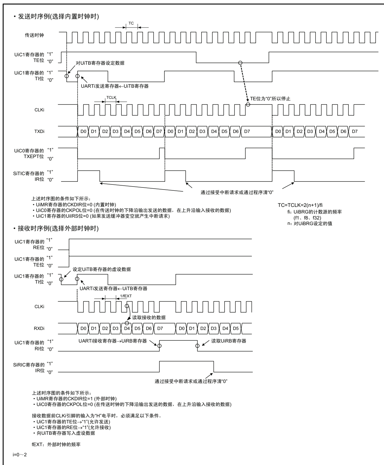
图 16.9 时钟同步串行 I/O 模式时的发送和接收时序例
