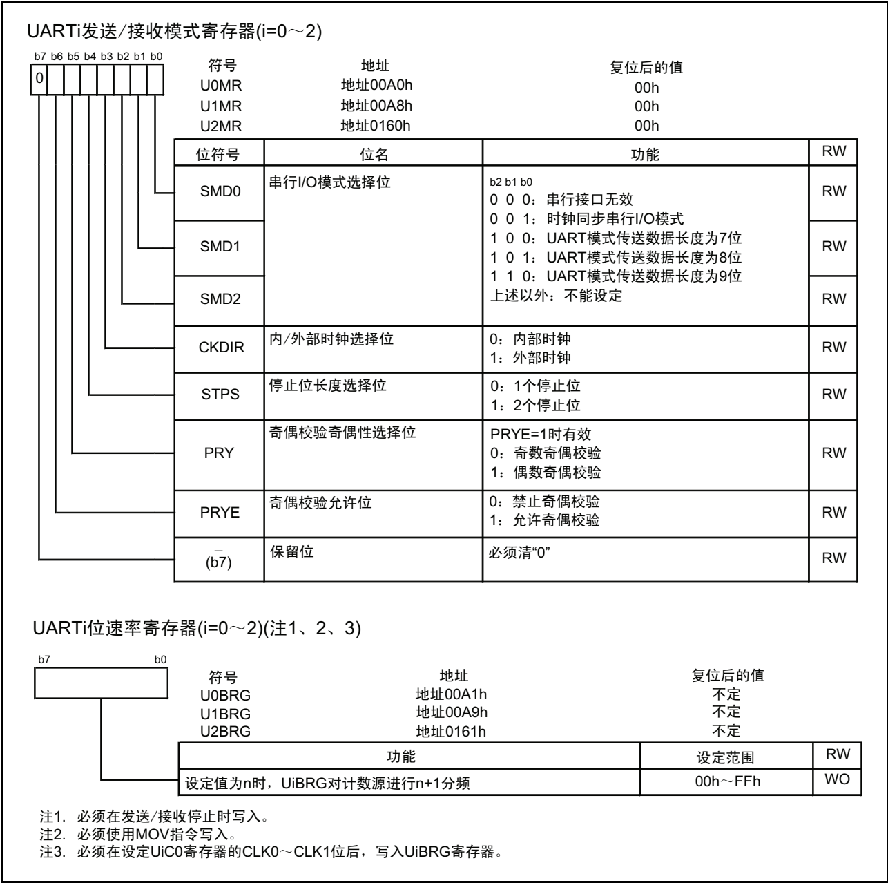
图 16.4 U0MR ~ U2MR、U0BRG ~ U2BRG 寄存器
