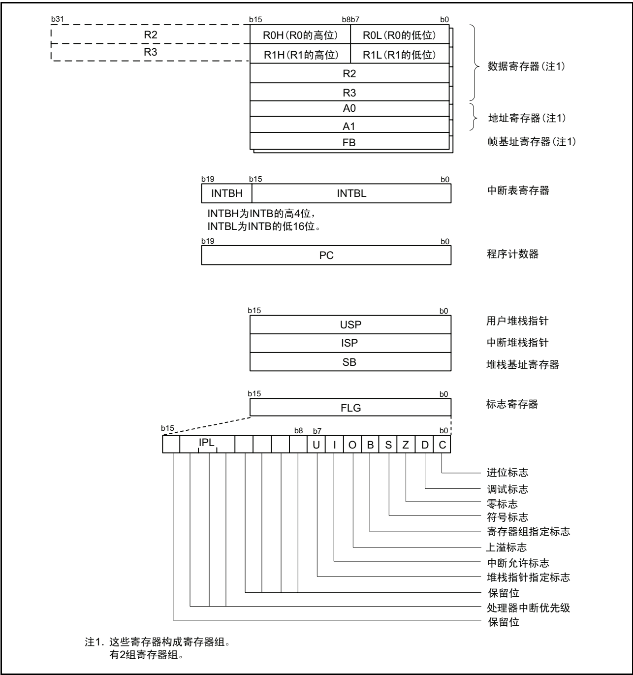
图 3.1 CPU 的寄存器
