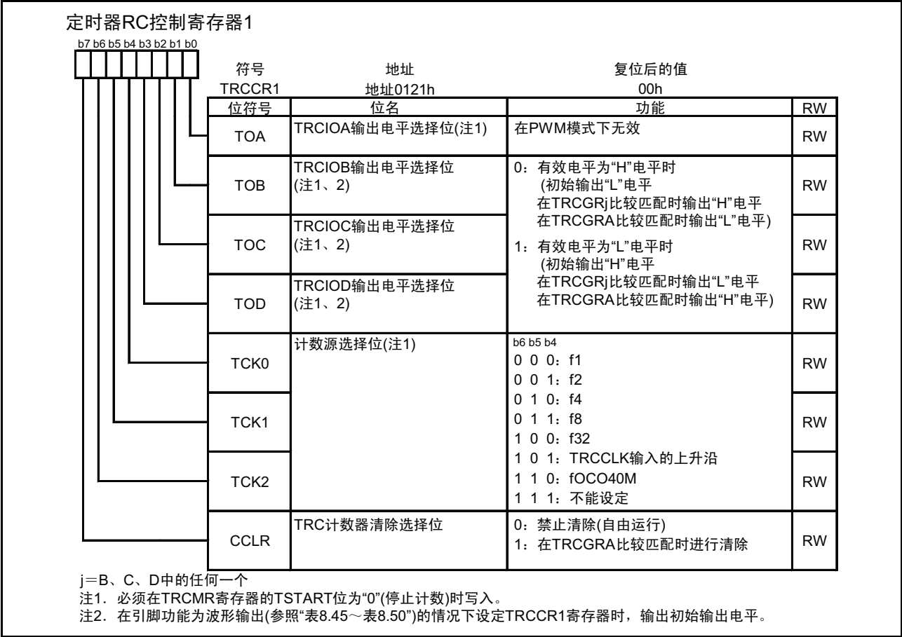
图 15.53 PWM 模式时的 TRCCR1 寄存器
