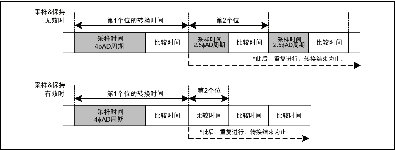
图 19.5 A/D 转换时序图
