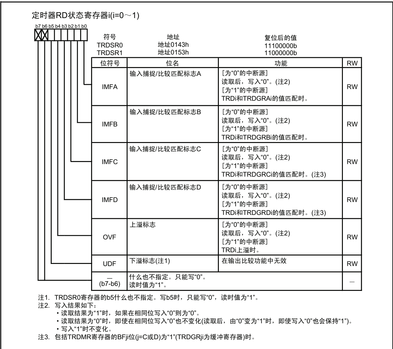
图 15.93 输出比较功能时的 TRDSR0 ~ TRDSR1 寄存器
