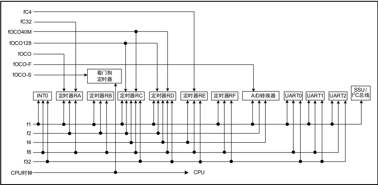
图 11.2 外围功能的时钟
