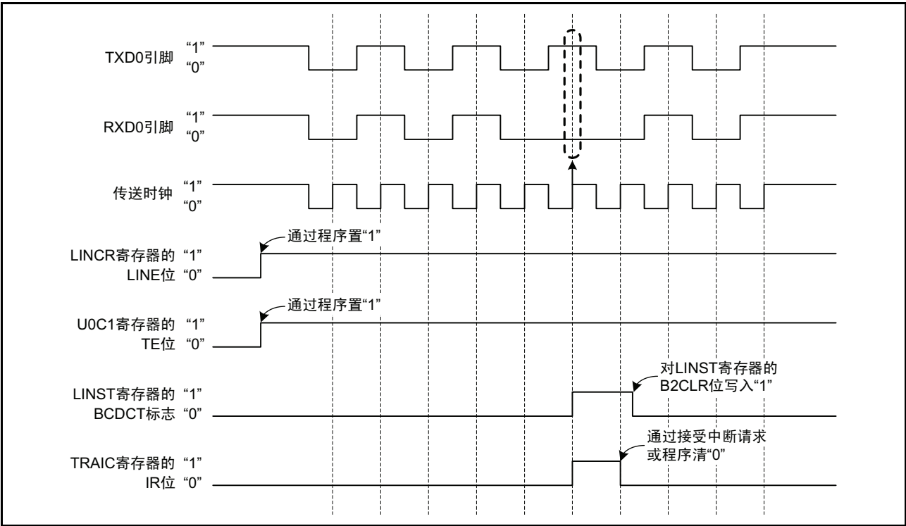
图 18.11 检测总线冲突时的运行例
