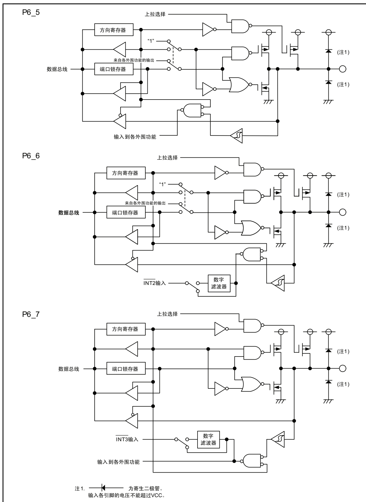
图 8.9 可编程输入 / 输出端口的结构 (9)
