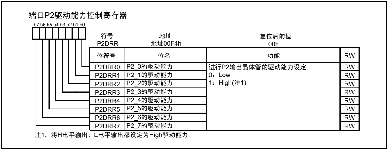
图 8.15 P2DRR 寄存器
