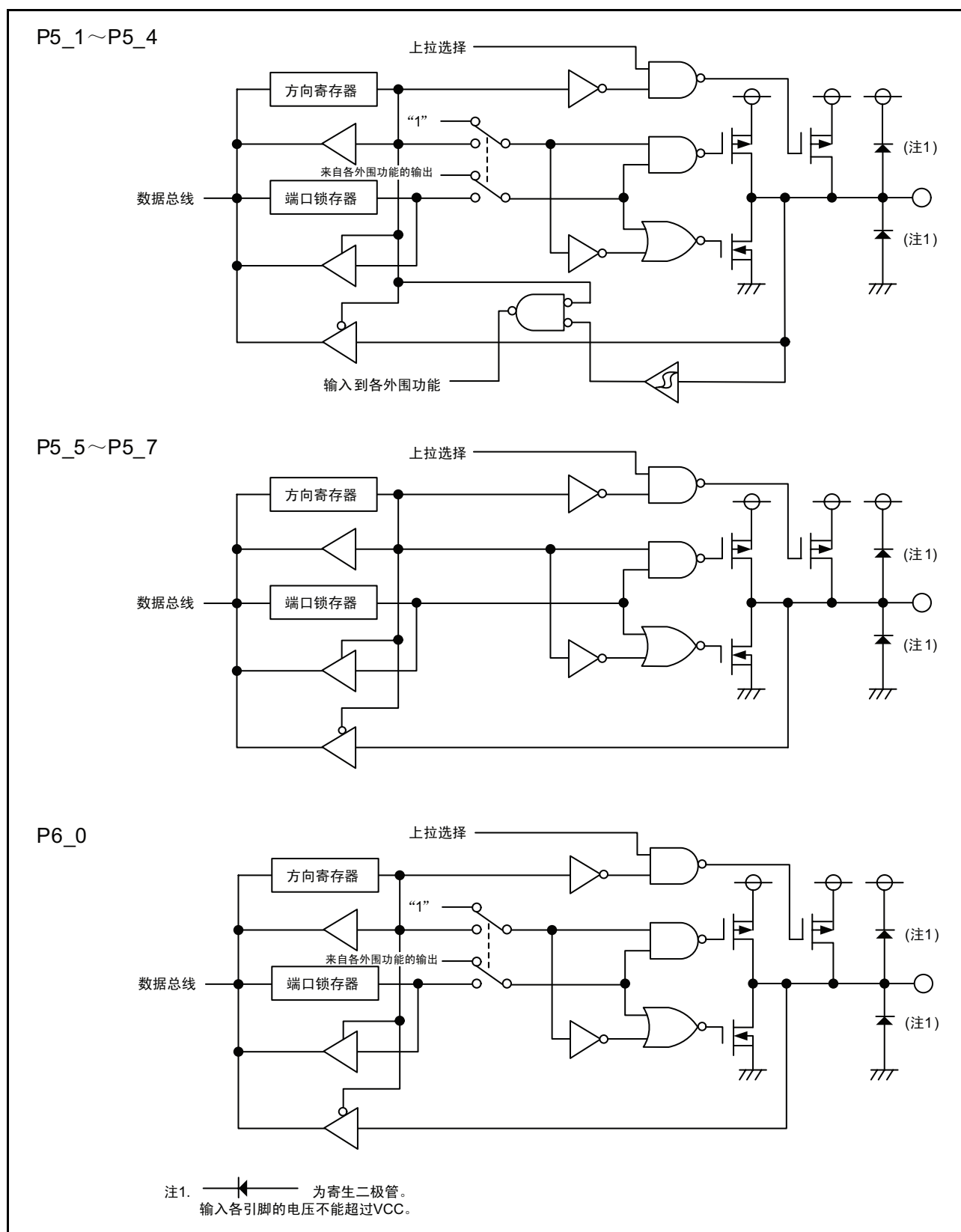
图 8.7 可编程输入 / 输出端口的结构 (7)
