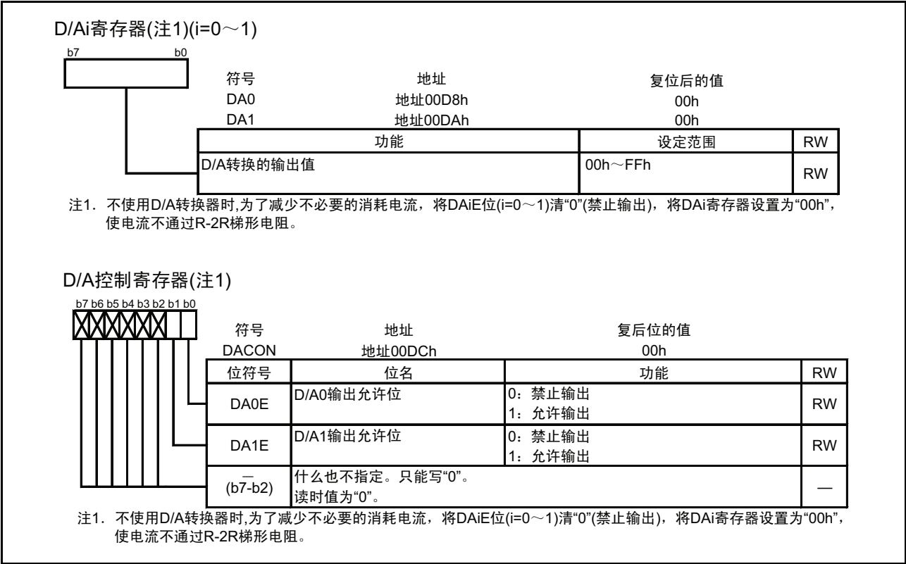
图 20.2 DA0 ~ DA1、DACON 寄存器
