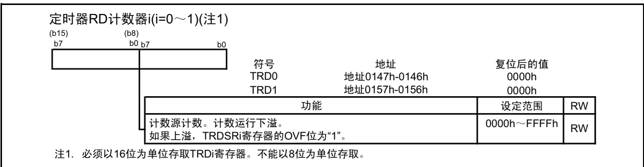
图 15.79 输入捕捉功能时的 TRD0 ~ TRD1 寄存器
