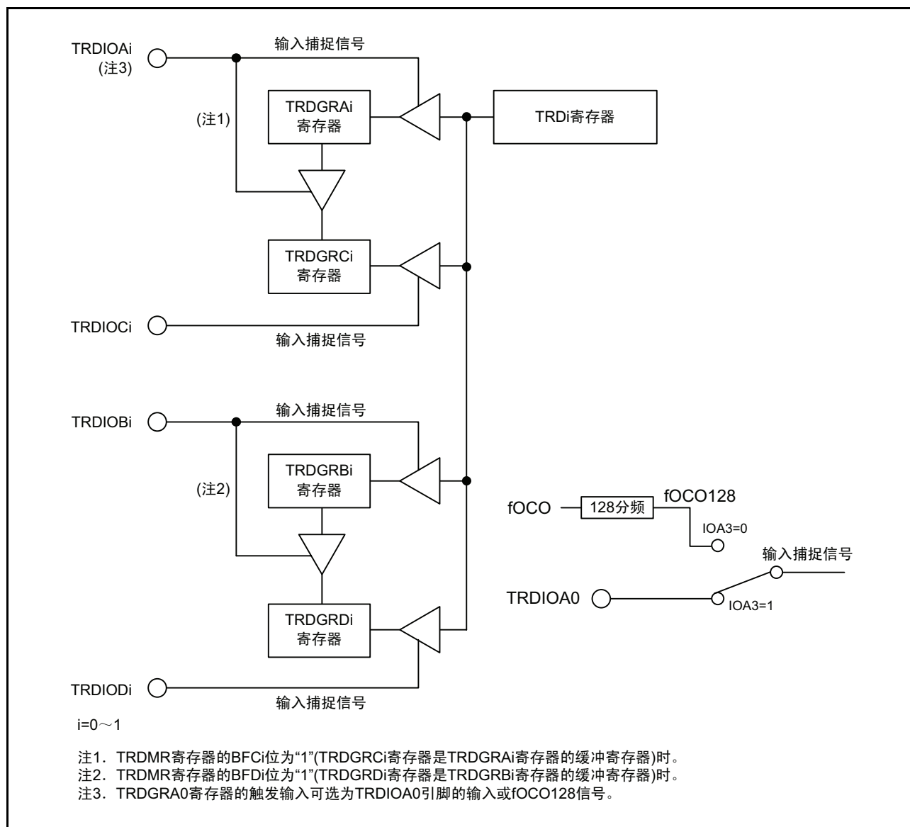
图 15.68 输入捕捉功能的框图
