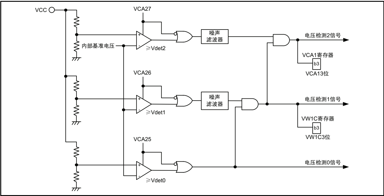
图 7.1 电压检测电路的框图
