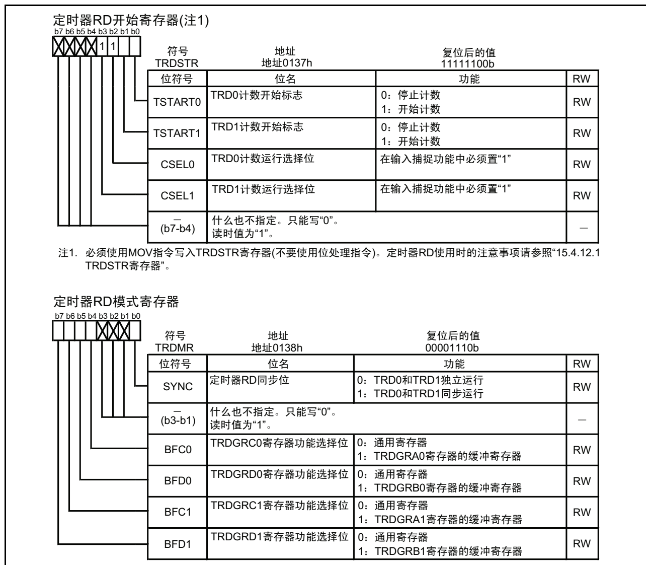
图 15.70 输入捕捉功能时的 TRDSTR、TRDMR 寄存器
