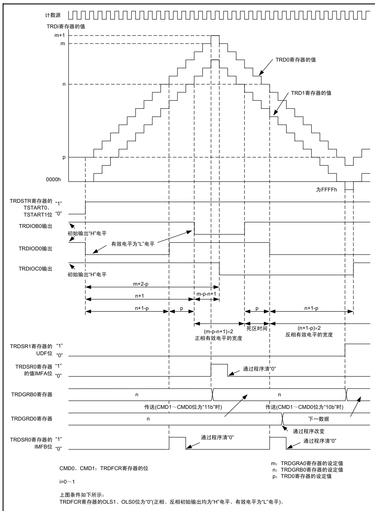
图 15.135 互补 PWM 模式的运行例
