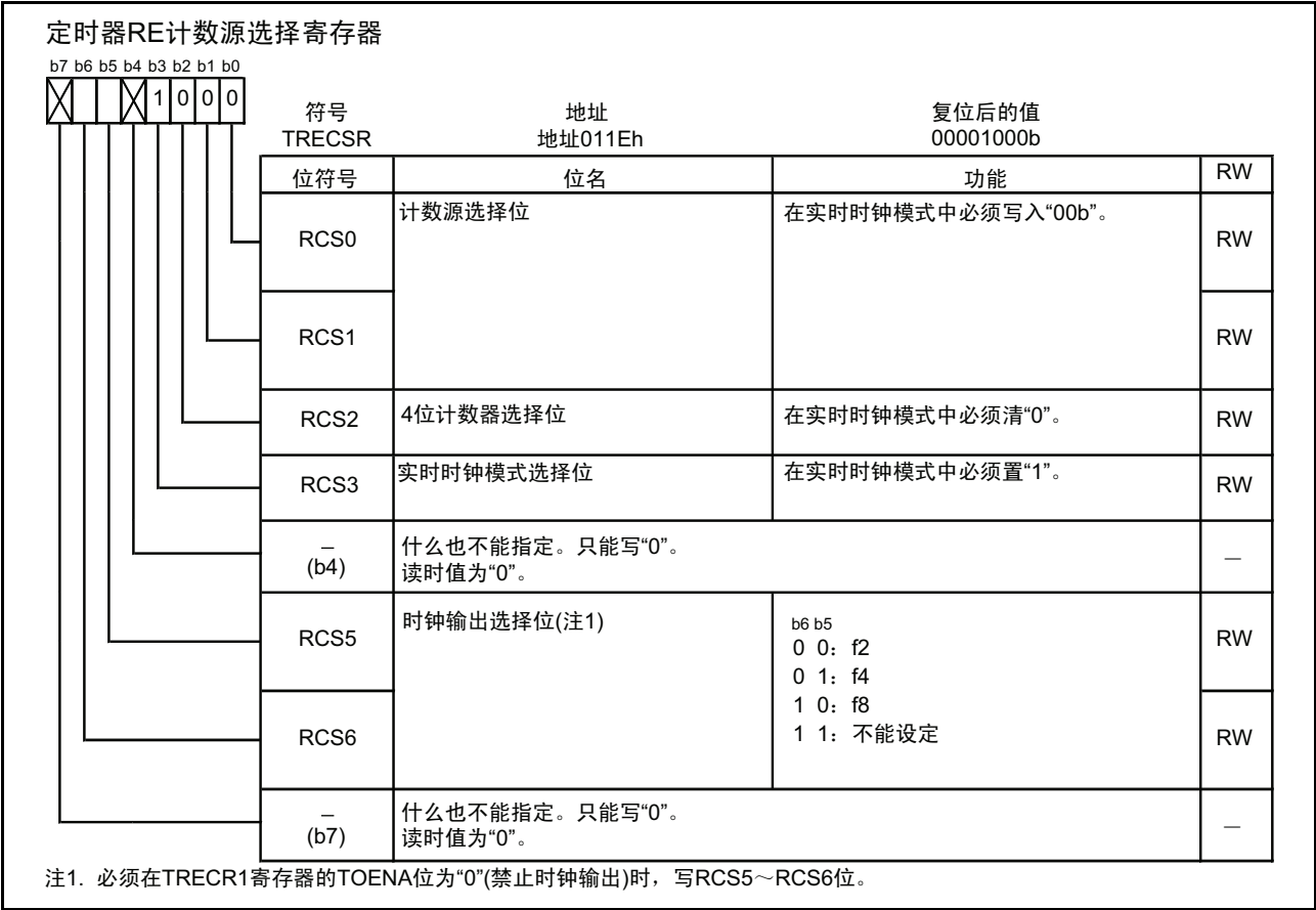
图 15.160 实时时钟模式时的 TRECSR 寄存器
