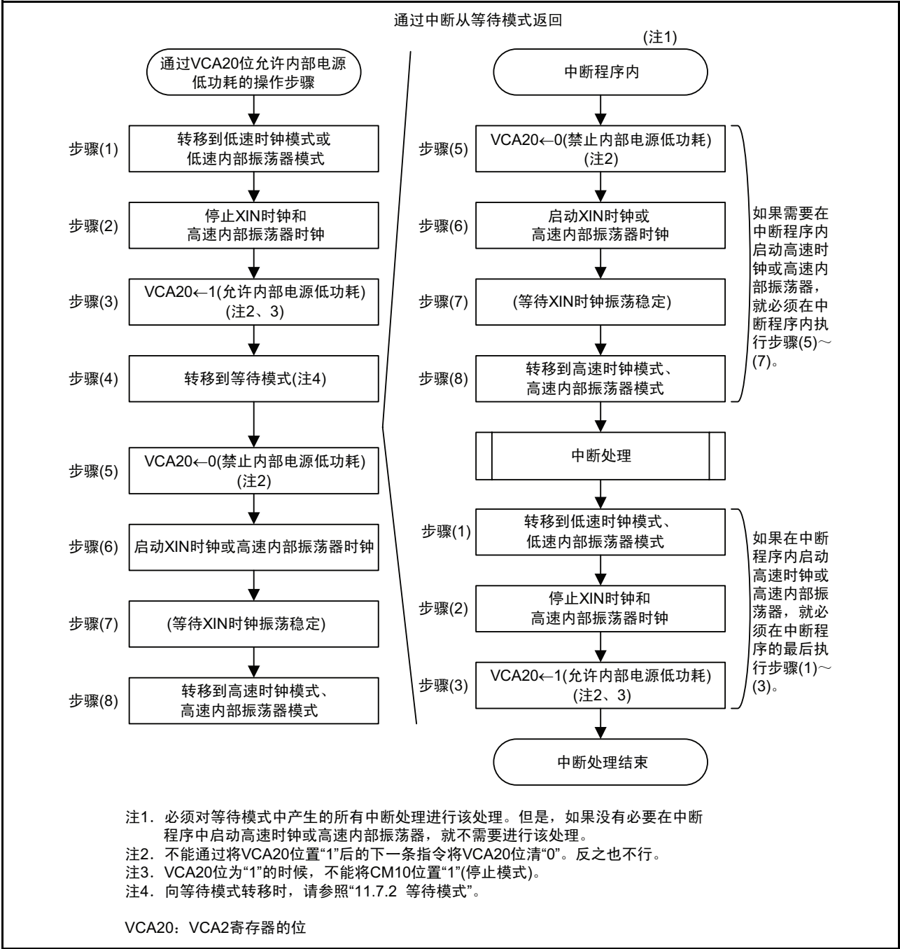
图 11.10 通过 VCA20 位使内部电源低功耗的操作步骤
