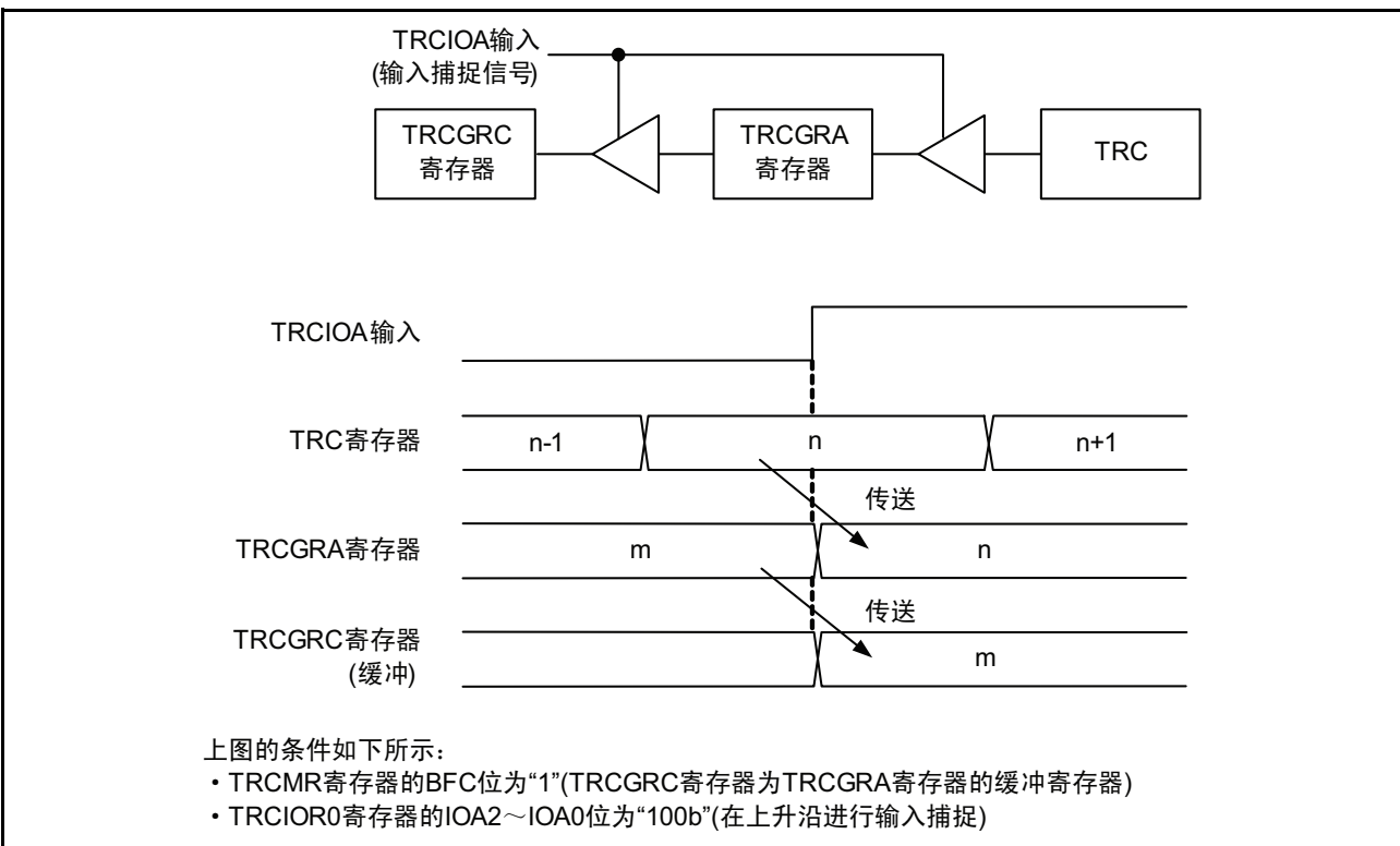
图 15.39 输入捕捉功能的缓冲器运行
