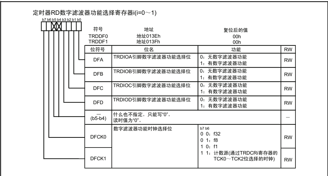
图 15.73 输入捕捉功能时的 TRDDF0 ~ TRDDF1 寄存器
