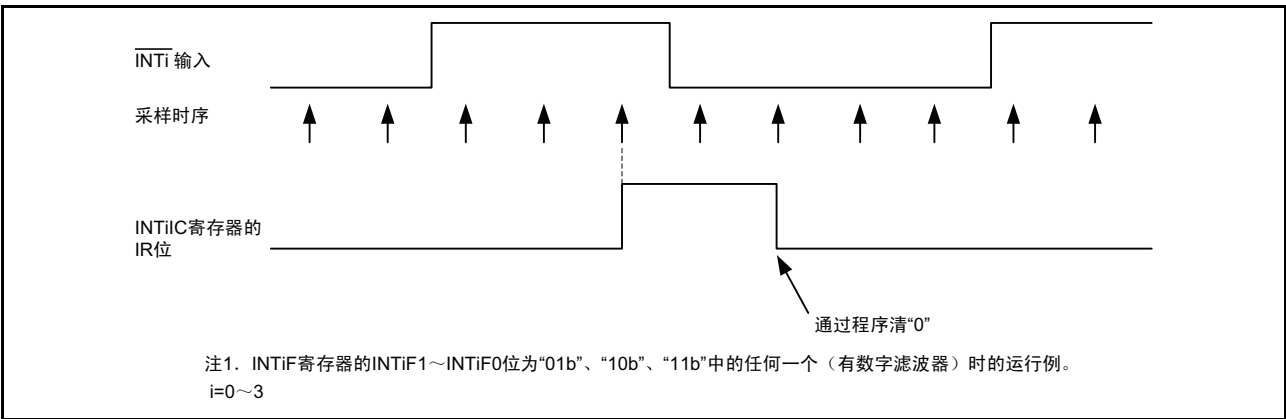
图 13.17 \overline{\text{INTi}} 输入滤波器的运行例
