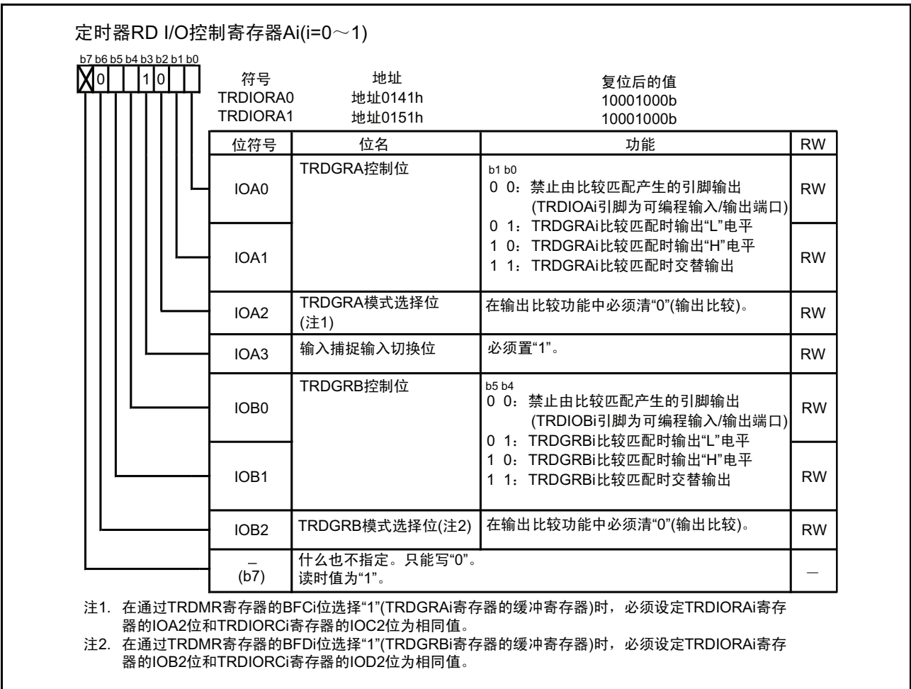
图 15.91 输出比较功能时的 TRDIOA0 ~ TRDIOA1 寄存器
