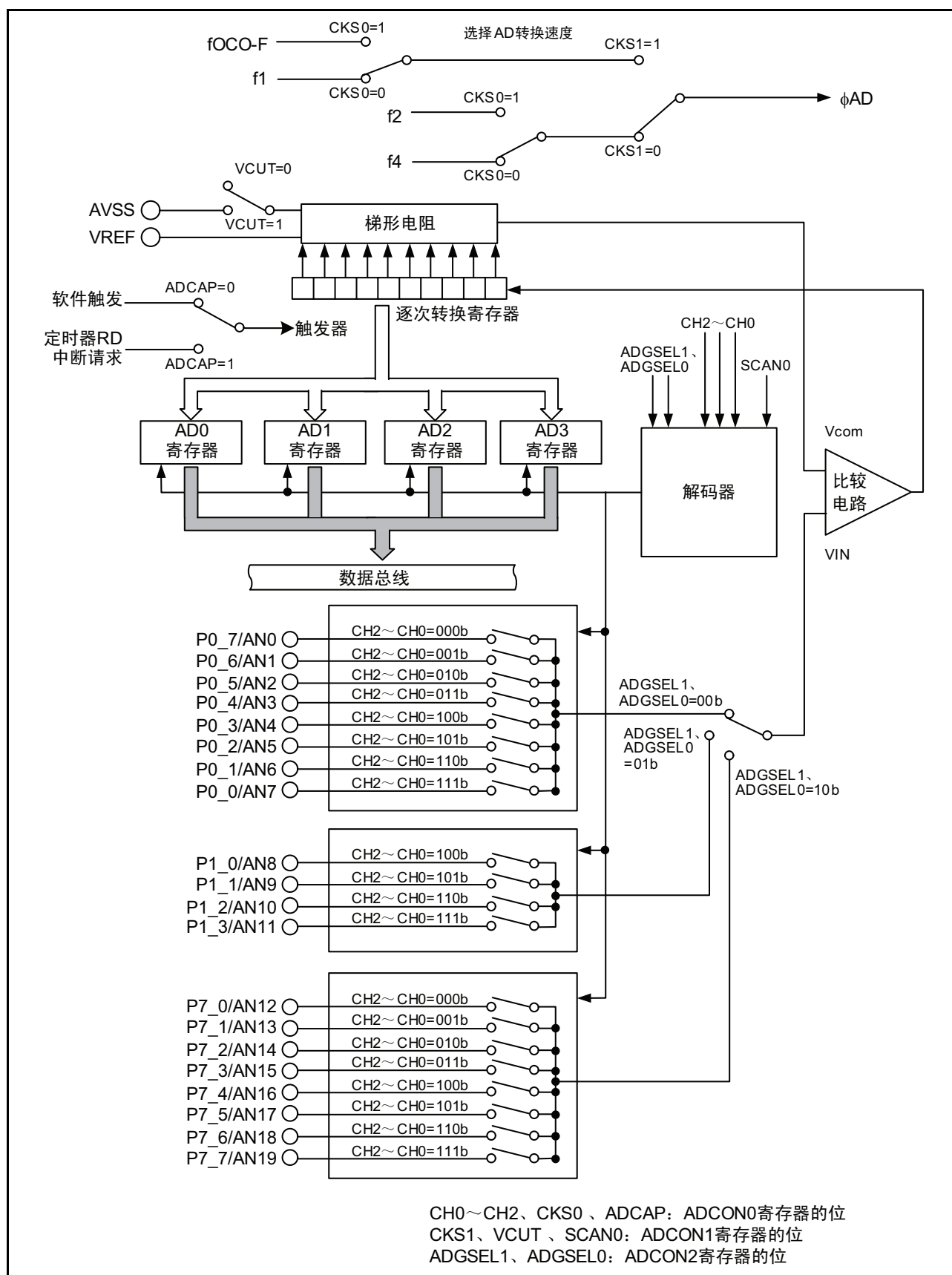
图 19.1 A/D 转换器的框图
