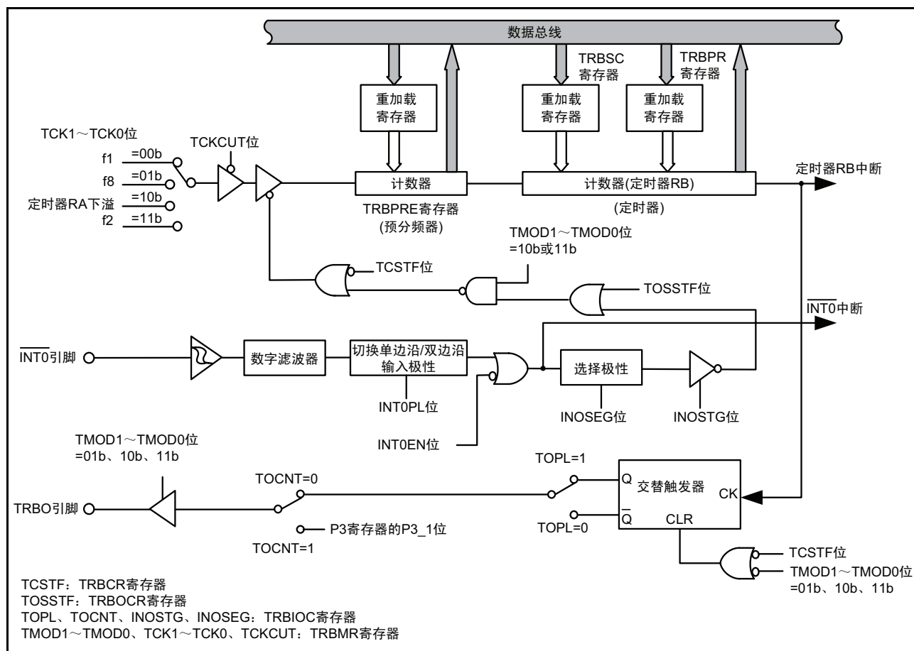
图 15.12 定时器 RB 的框图
