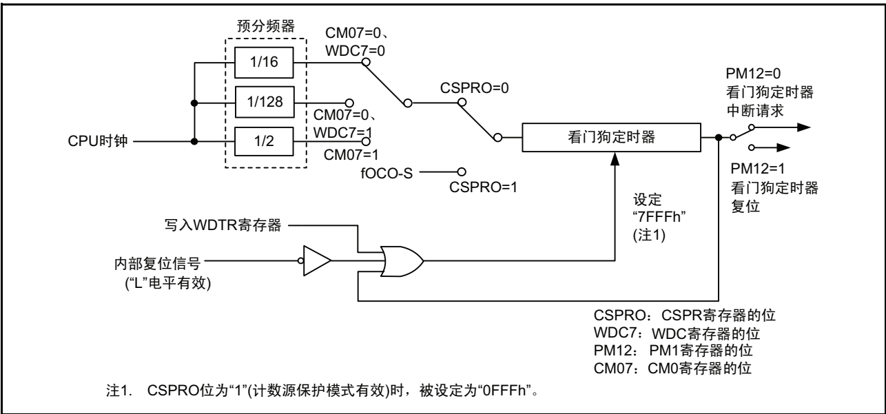
图 14.1 看门狗定时器的框图
