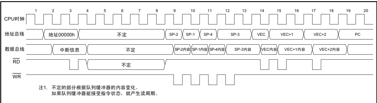
图 13.6 中断响应顺序的执行时间
