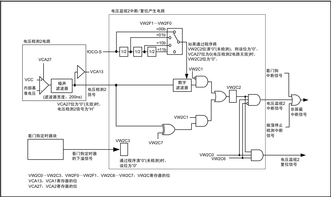
图 7.4 电压监视 2 中断 / 复位产生电路的框图
