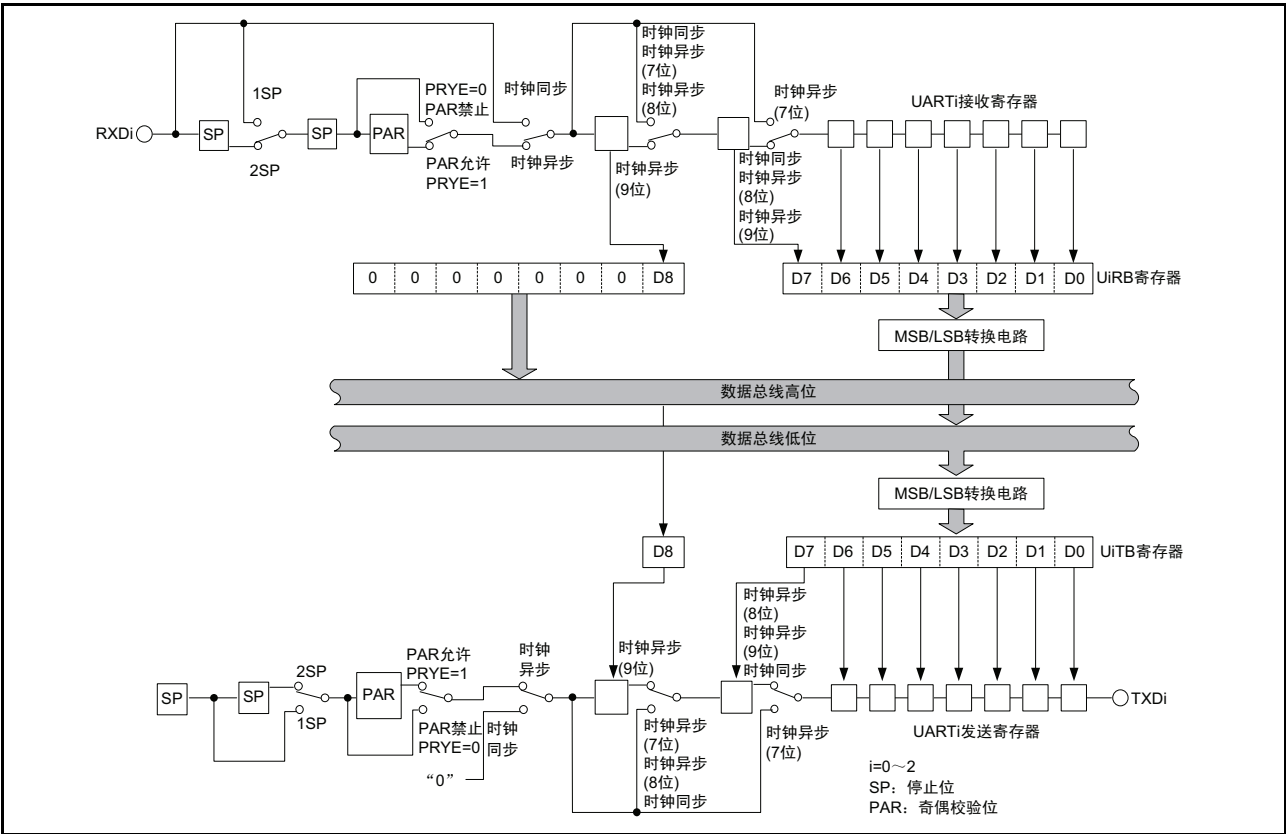
图 16.2 发送和接收部的框图
