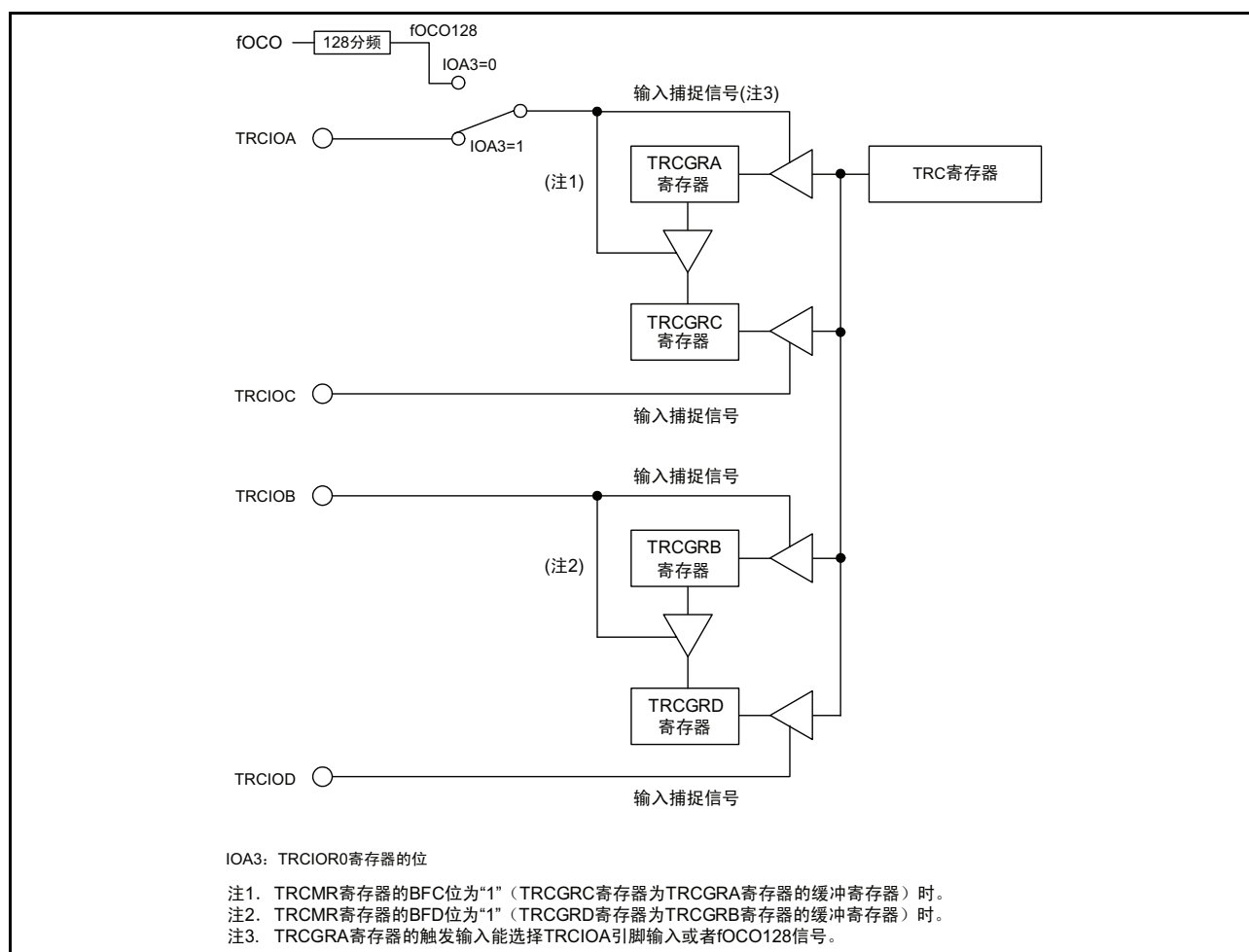
图 15.43 输入捕捉功能的框图
