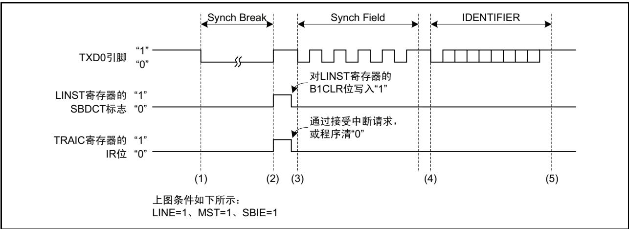
图 18.4 发送头字段时的运行例
