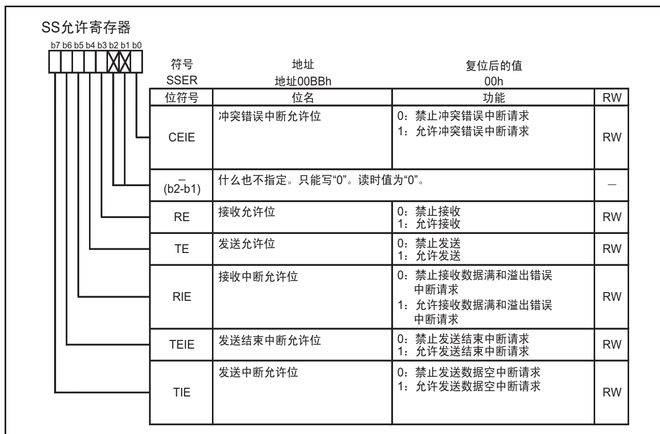
图 17.6 SSER 寄存器
