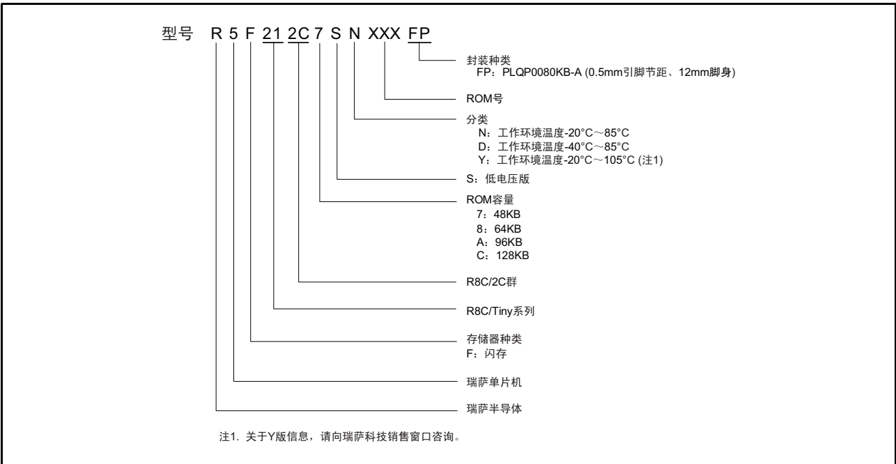
图 1.1 R8C/2C 群的型号和存储器容量、封装
