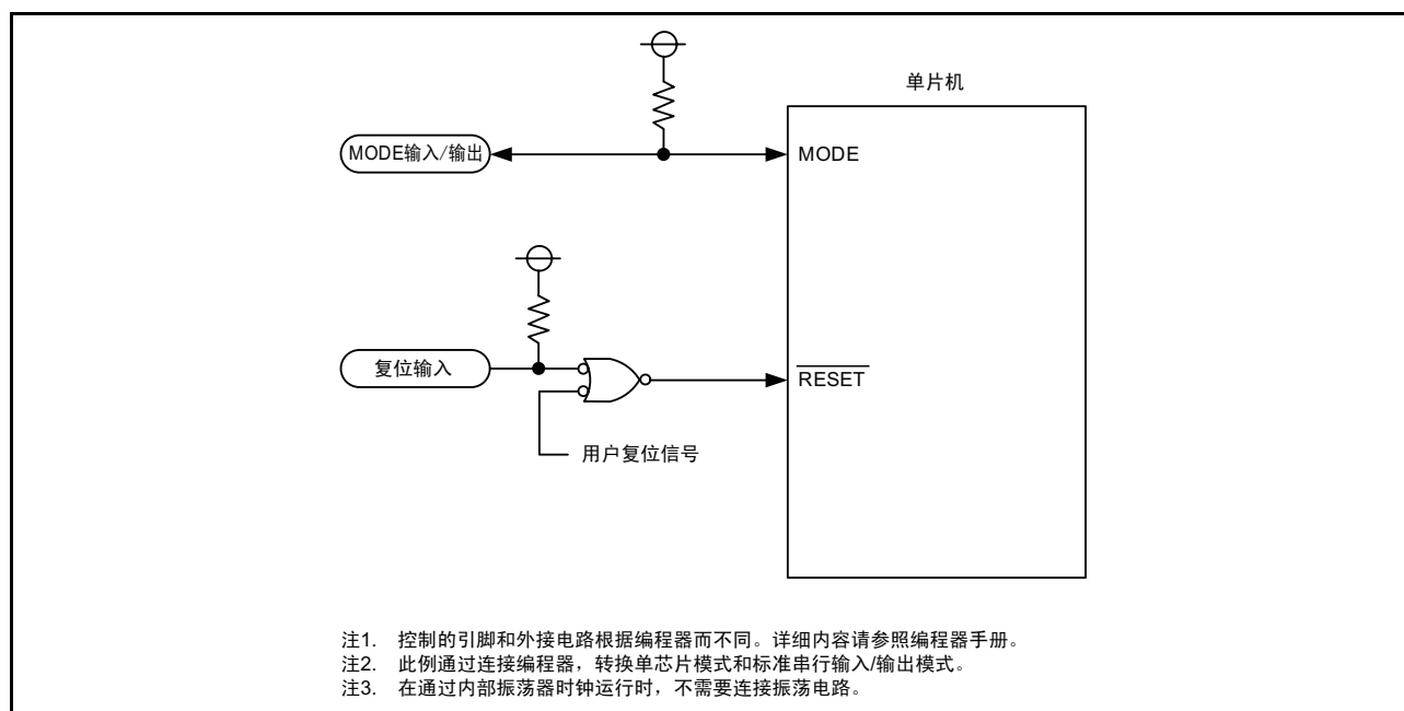
图 21.19 使用标准串行输入 / 输出模式 3 时的引脚处理例
