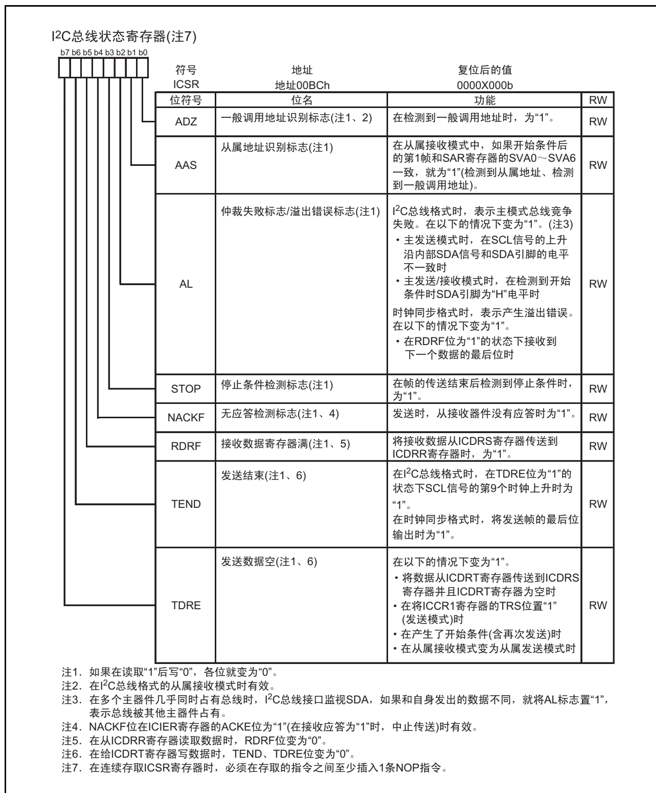
图 17.30 ICSR 寄存器
