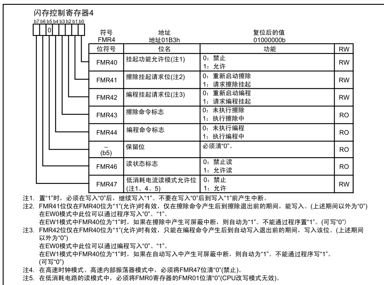
图 21.7 FMR4 寄存器
