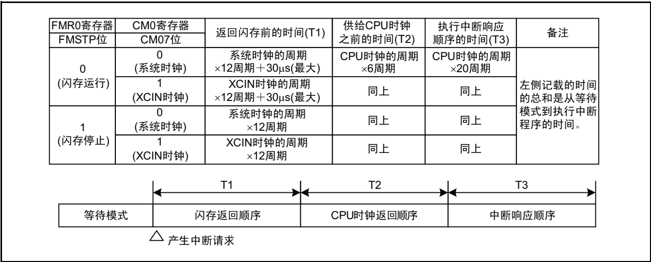
图 11.13 从等待模式到执行中断程序前的时间
