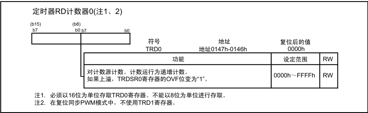
图 15.121 复位同步 PWM 模式时的 TRD0 寄存器
