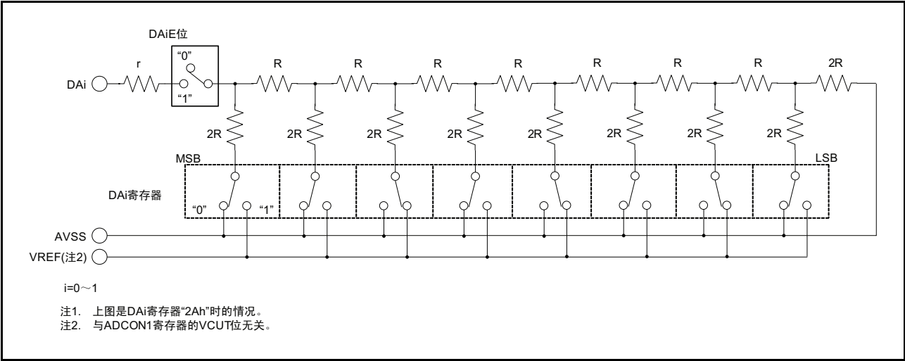
图 20.3 D/A 转换器的等效电路
