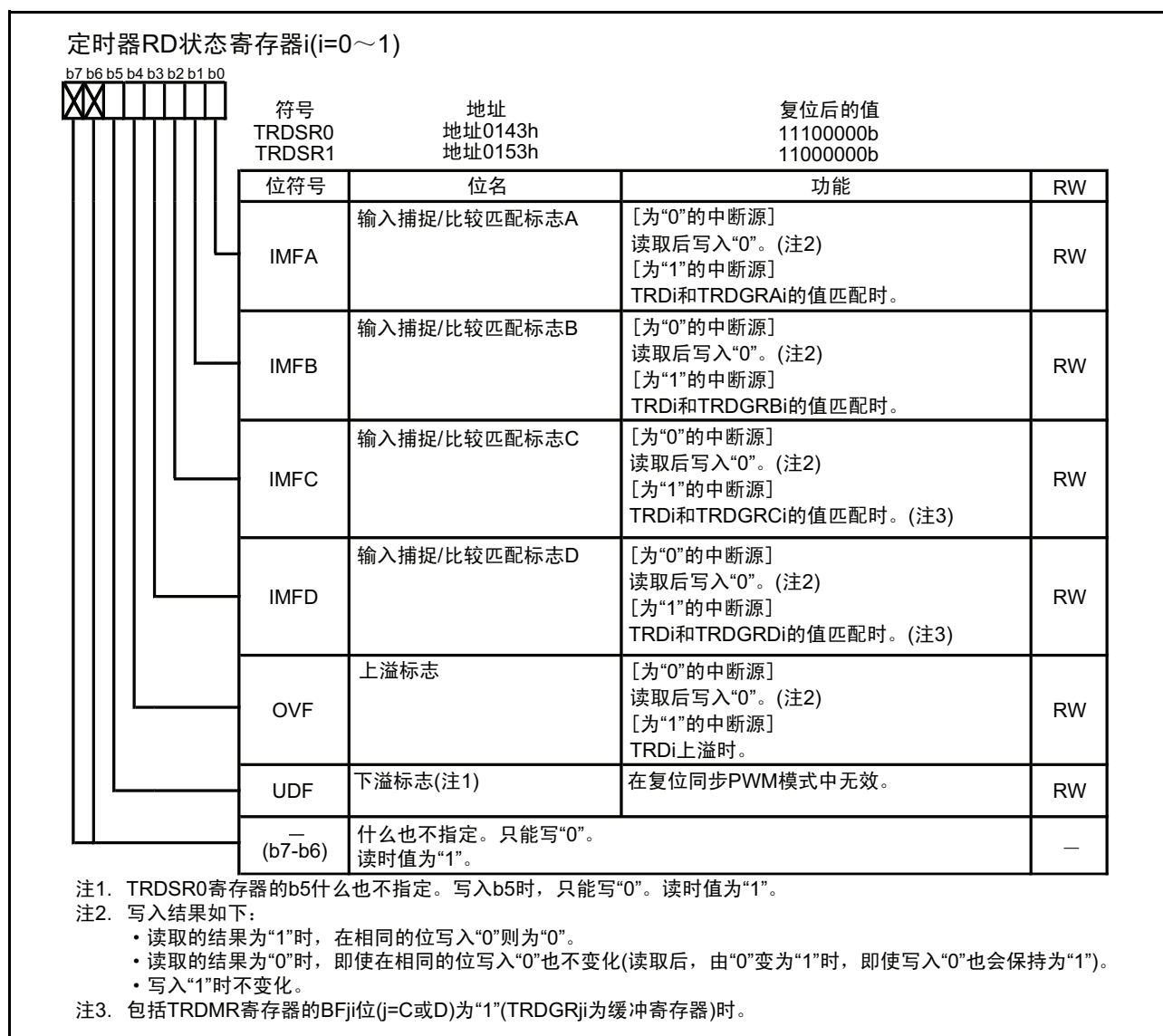
图 15.119 复位同步 PWM 模式时的 TRDSR0 ~ TRDSR1 寄存器
