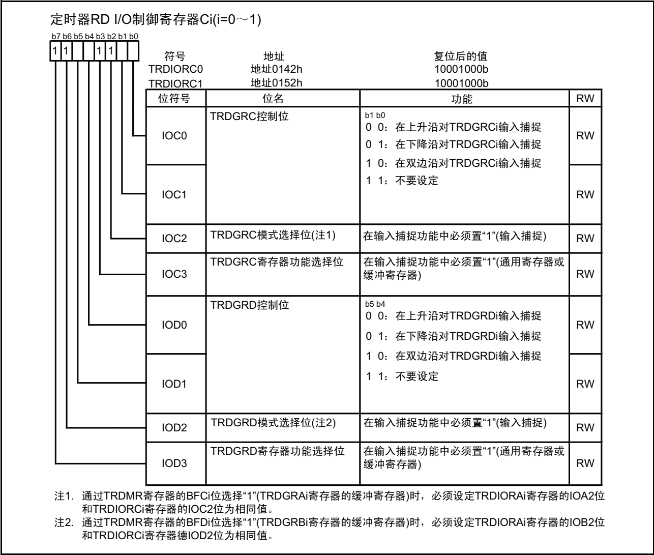
图 15.76 输入捕捉功能时的 TRDIORC0 ~ TRDIORC1 寄存器
