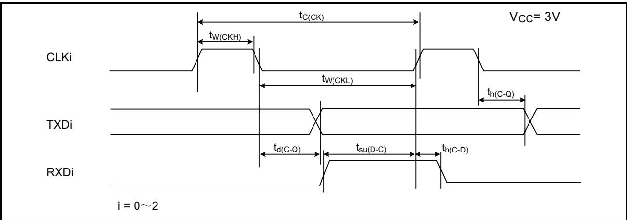
图 22.16 V_{CC}=3V 时的串行接口时序
