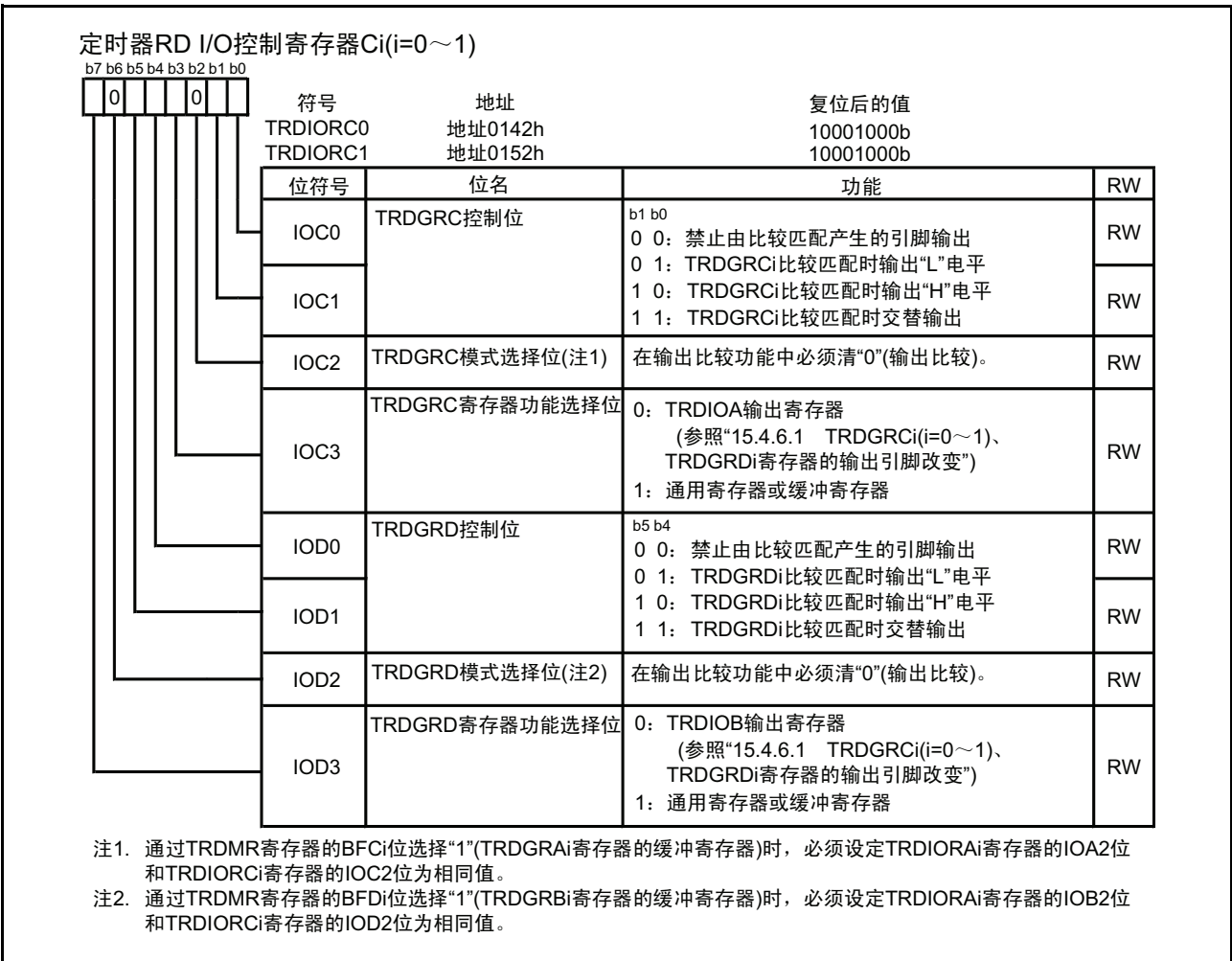
图 15.92 输出比较功能时的 TRDIORC0 ~ TRDIORC1 寄存器
