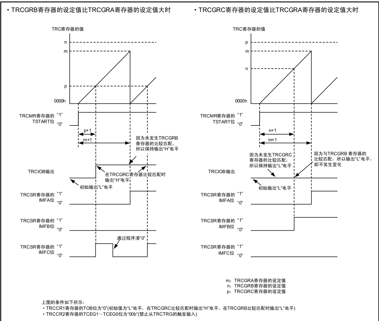
图 15.60 PWM2 模式的运行例（占空比 0%、占空比 100%）
