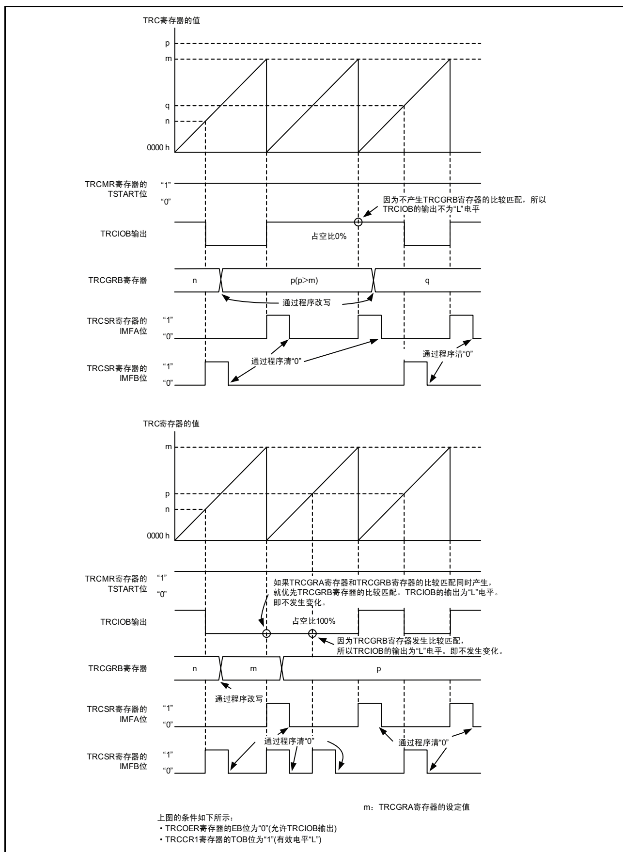
图 15.55 PWM 模式的运行例（站空比 0%、站空比 100%）
