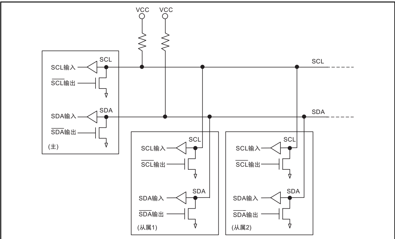
图 17.24 SCL、SDA 引脚的外部电路的连接例
