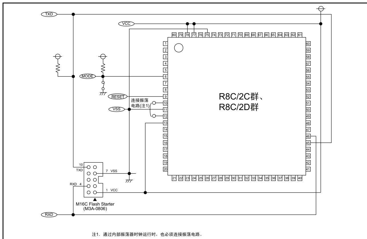
附图 2.1 和 M16C Flash Starter 的连接例（M3A-0806）
