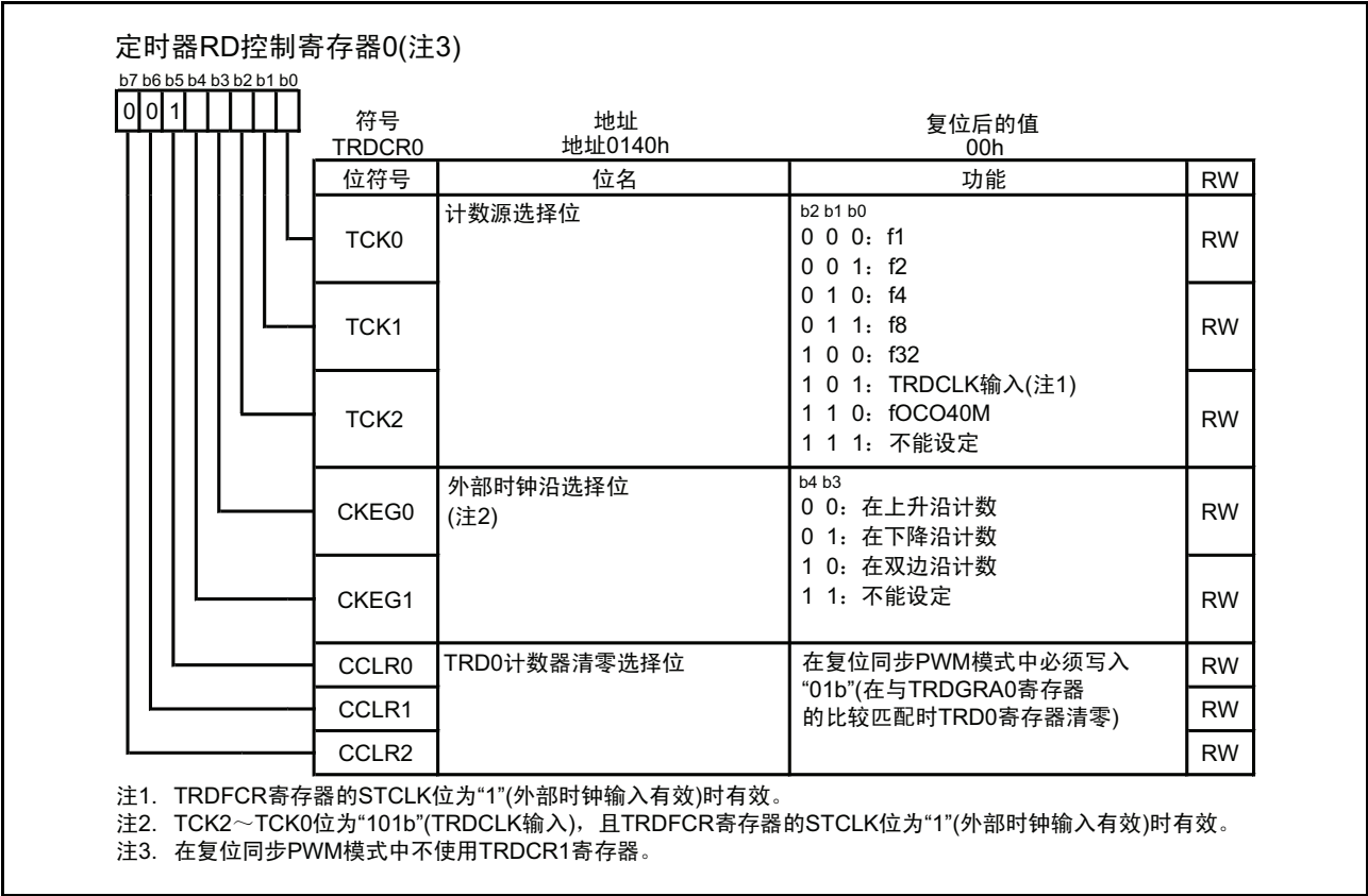
图 15.118 复位同步 PWM 模式时的 TRDCR0 寄存器
