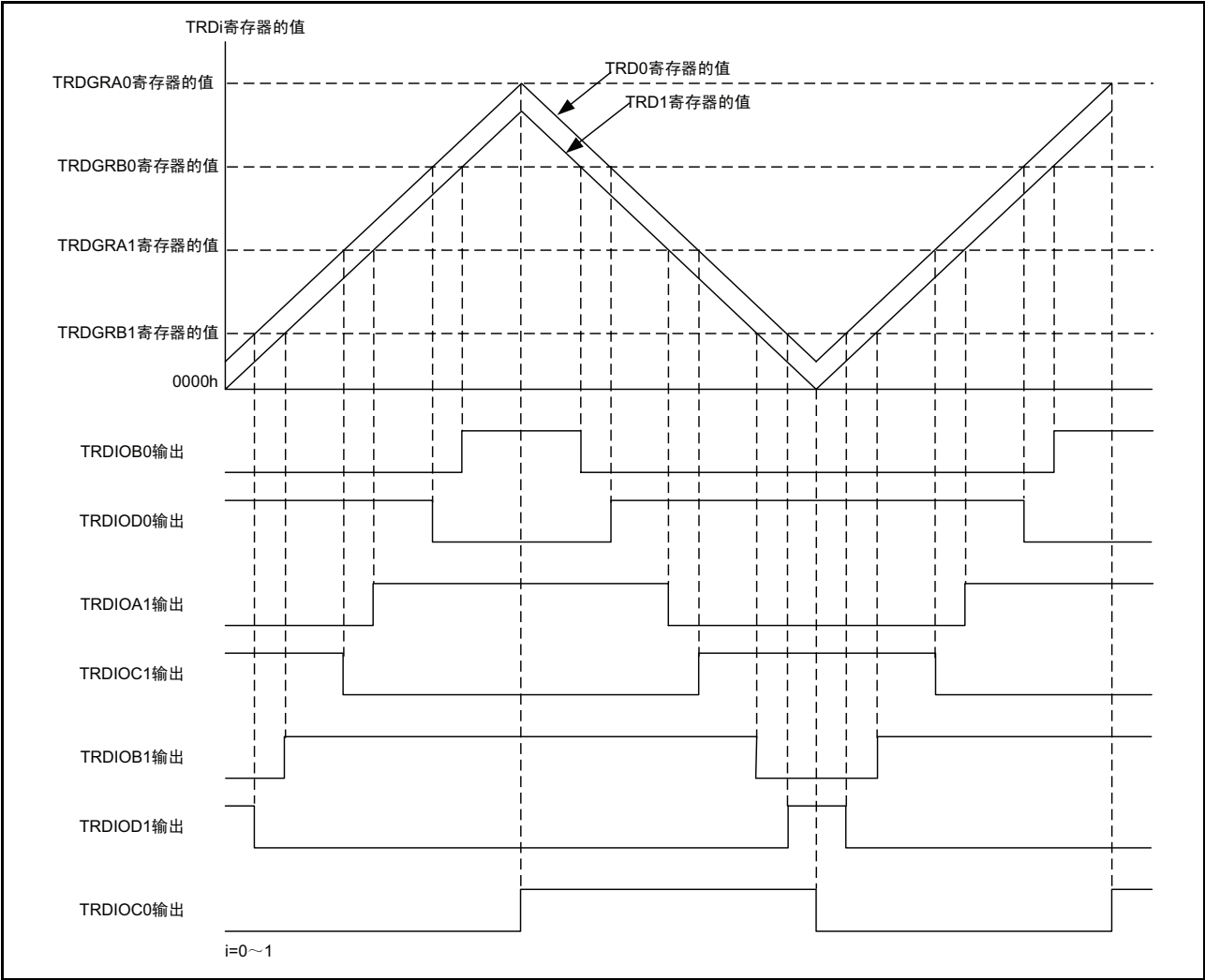
图 15.134 互补 PWM 模式的输出模型
