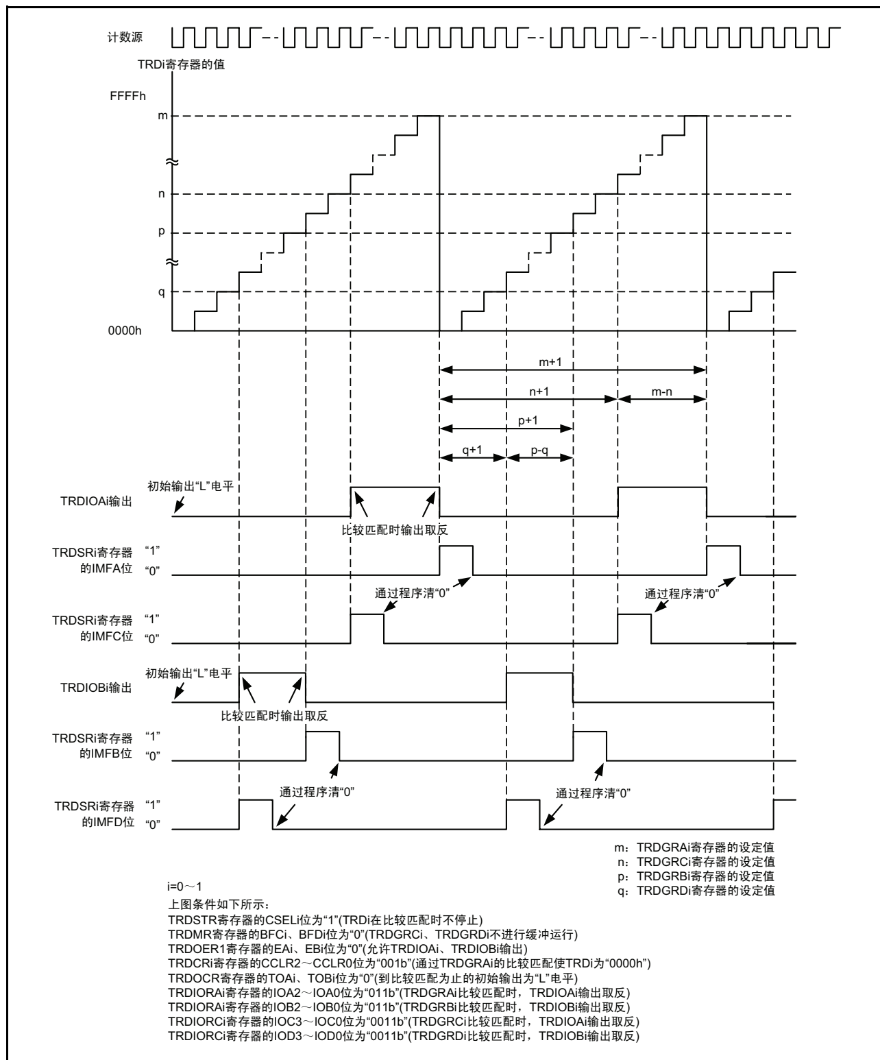
图 15.99 TRDGRCi 用作 TRDIOAi 引脚的输出控制，TRDGRDi 用作 TRDIOBi 引脚的输出控制时的运行例
