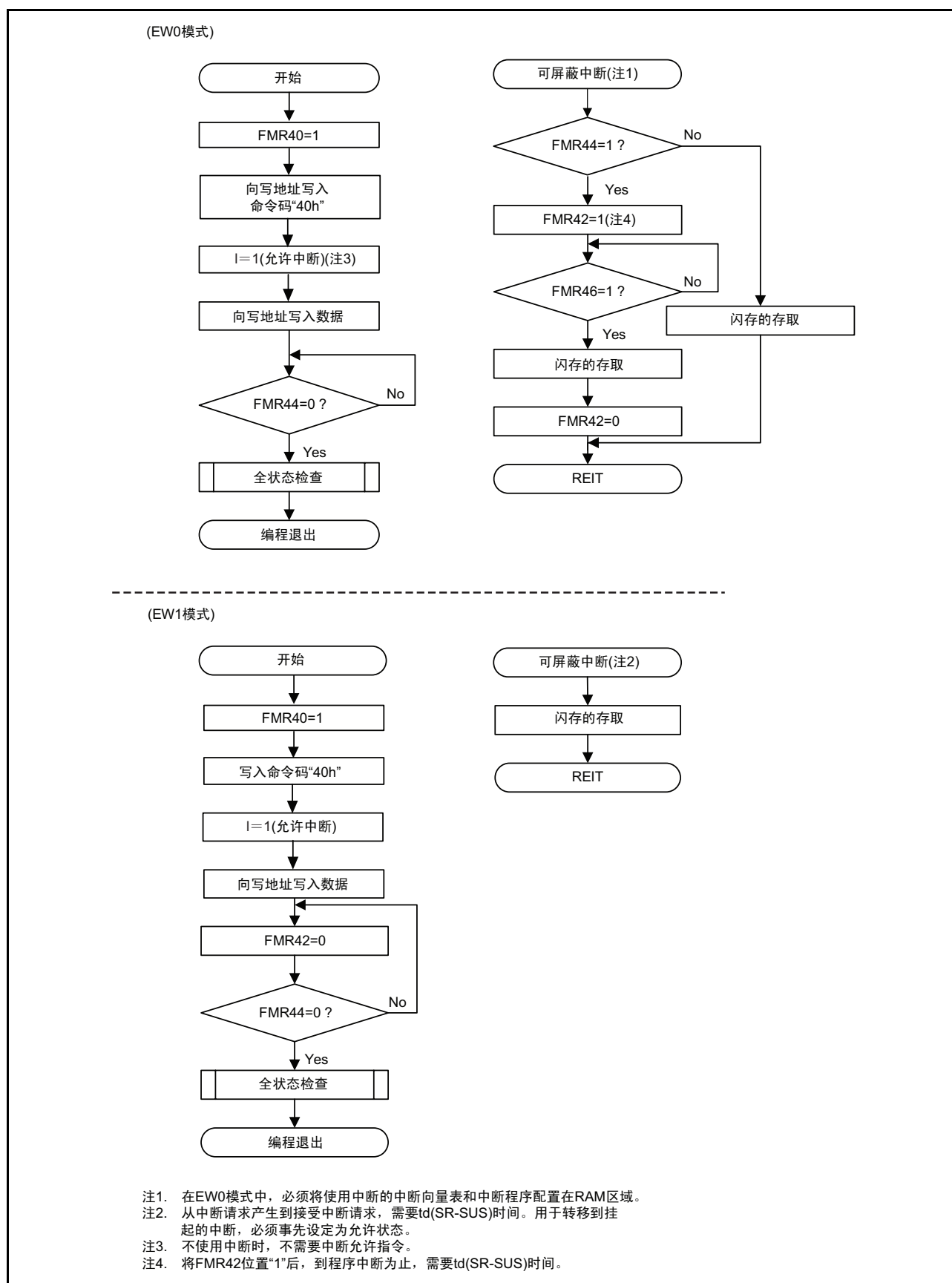
图 21.13 编程的流程图（允许挂起功能时）
