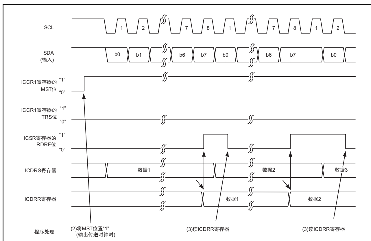
图 17.44 接收模式的运行时序（时钟同步串行模式）
