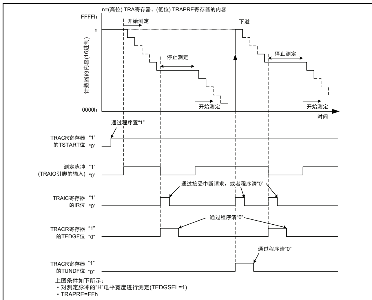
图 15.9 脉宽测定模式时的运行例
