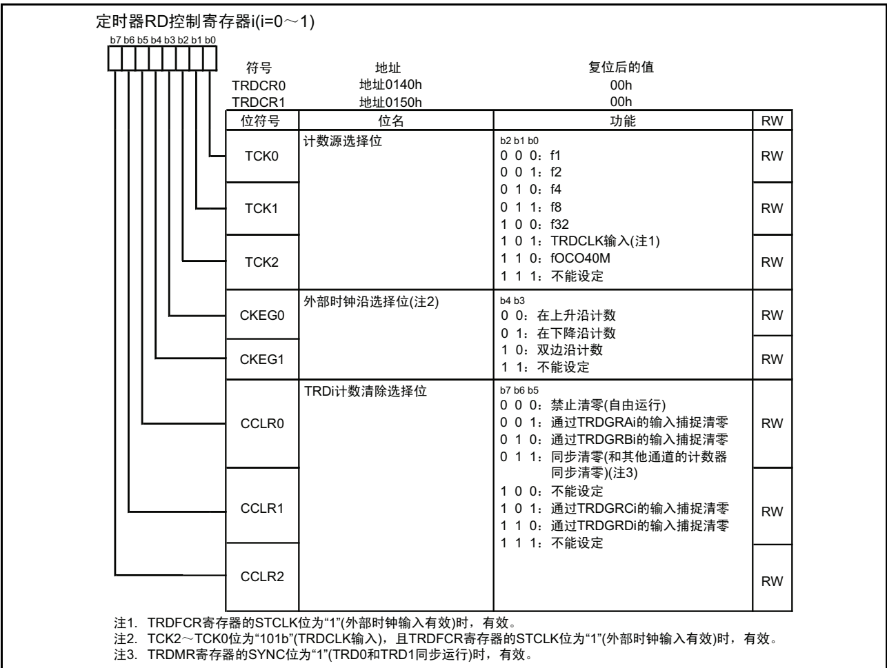
图 15.74 输入捕捉功能时的 TRDCR0 ~ TRDCR1 寄存器
