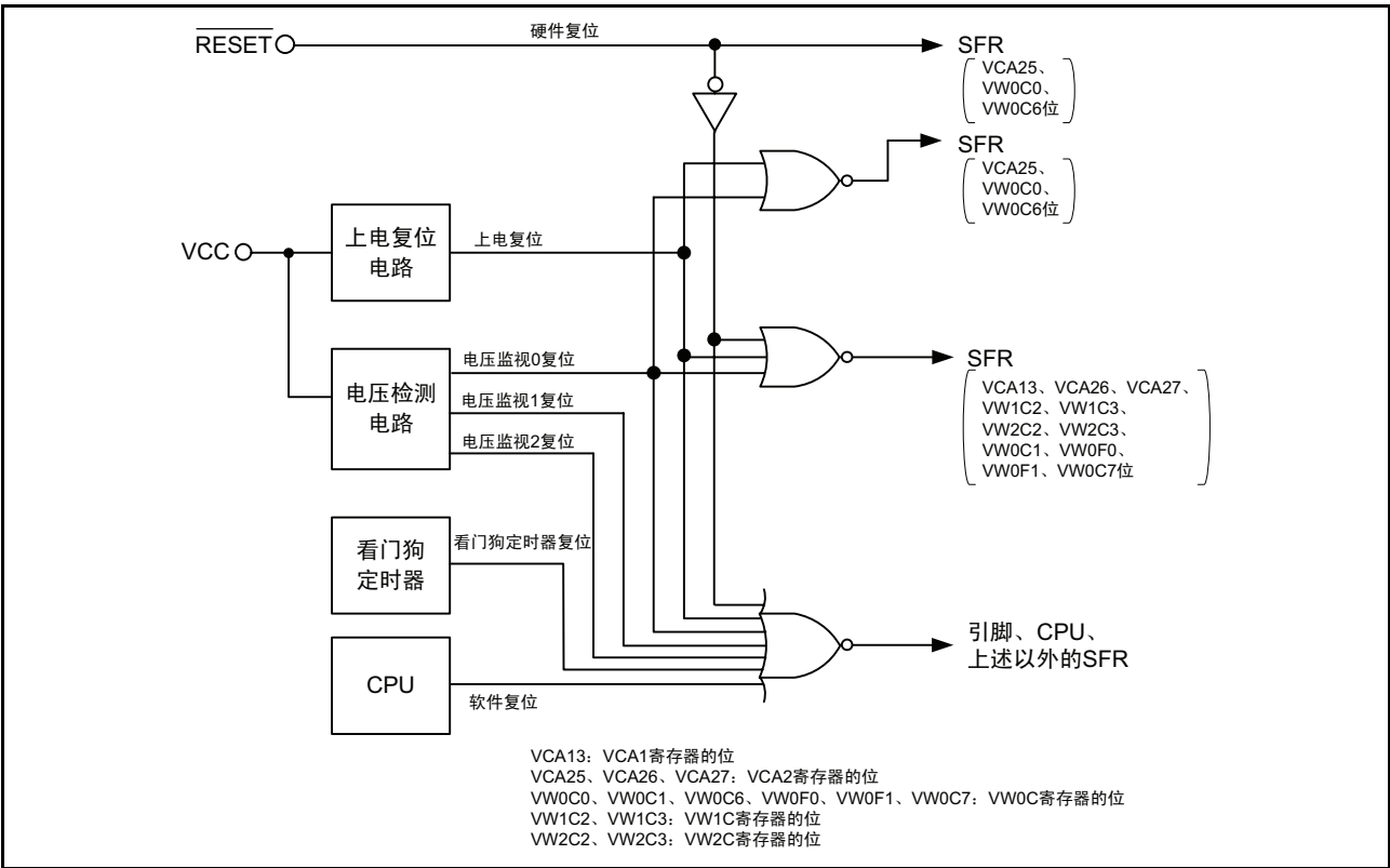
图 6.1 复位电路的框图
