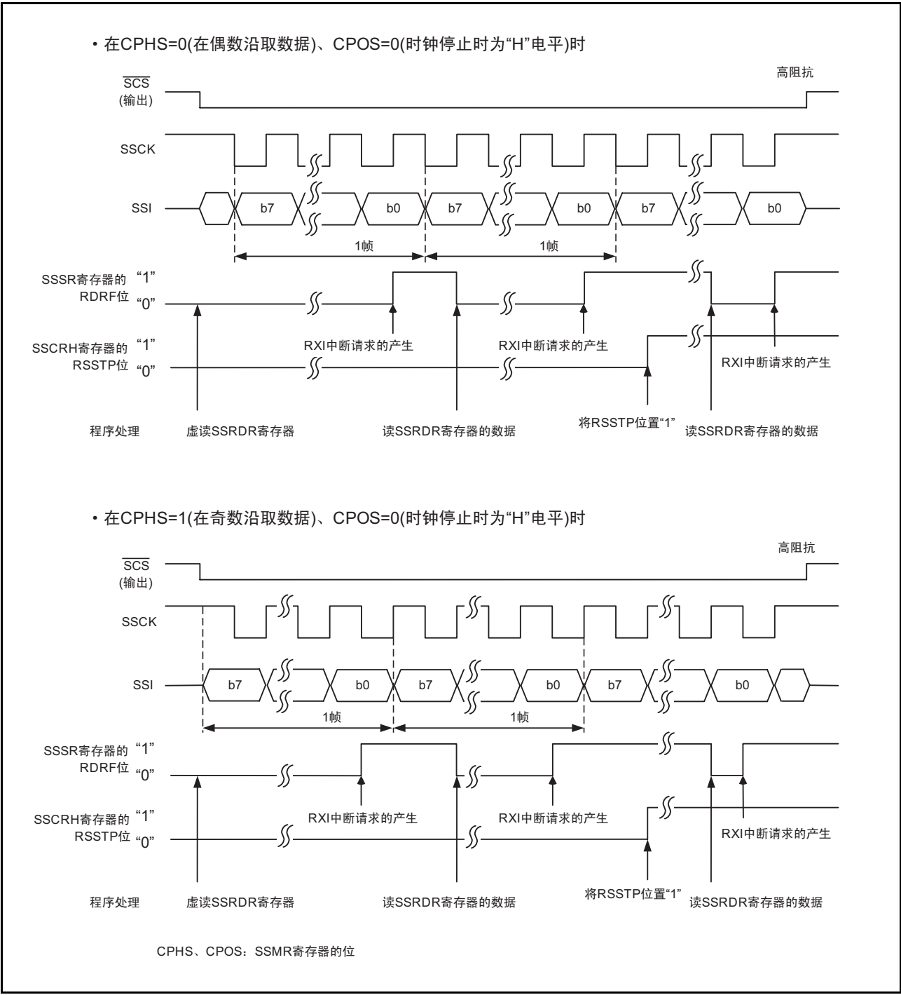
图 17.21 接收数据时的运行例（4 线方式总线通信模式）
