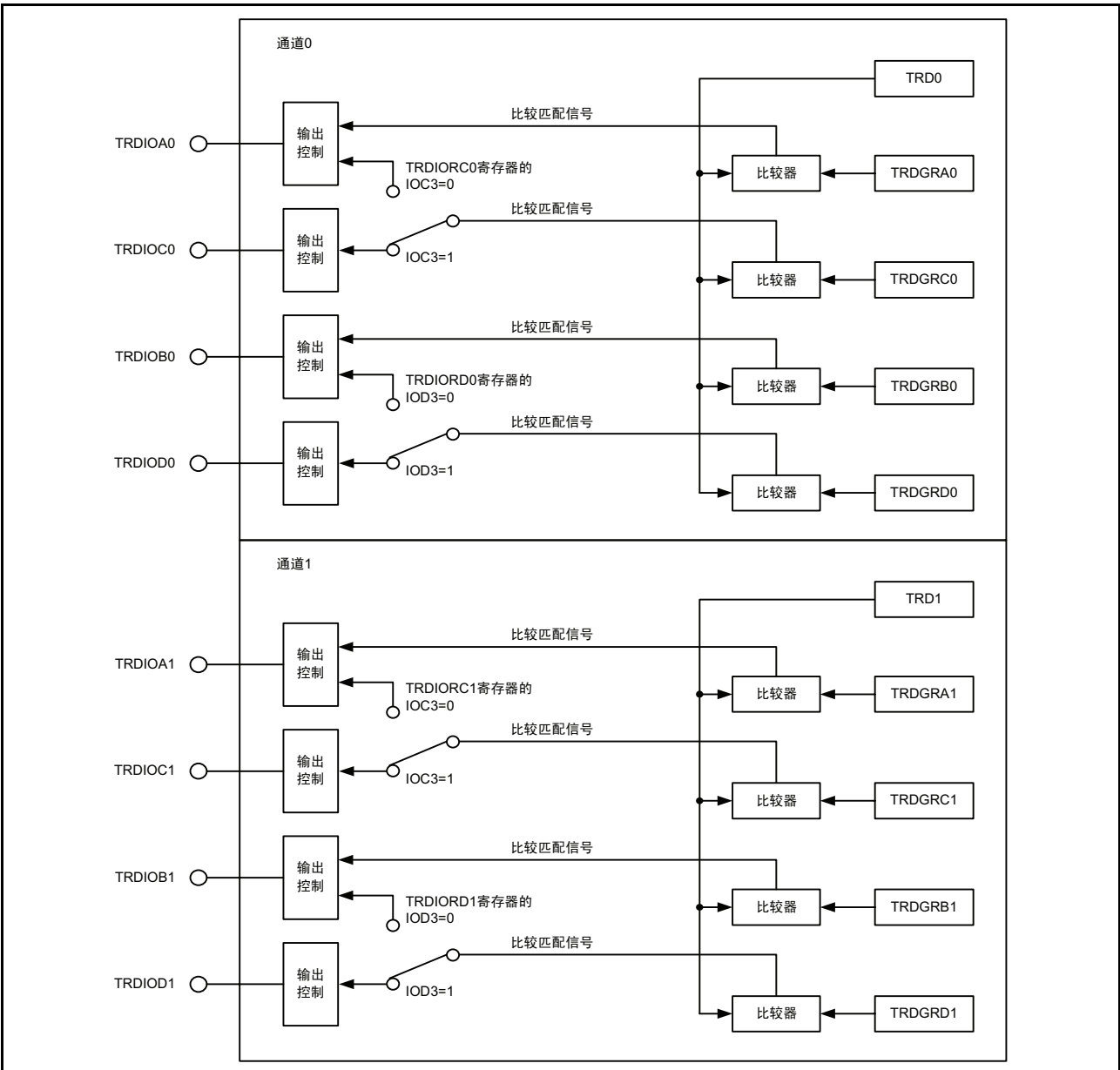
图 15.83 输出比较功能的框图
