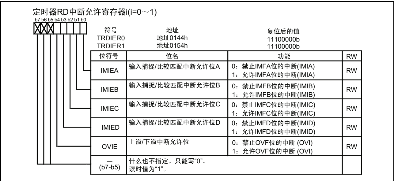
图 15.94 输出比较功能时的 TRDIER0 ~ TRDIER1 寄存器
