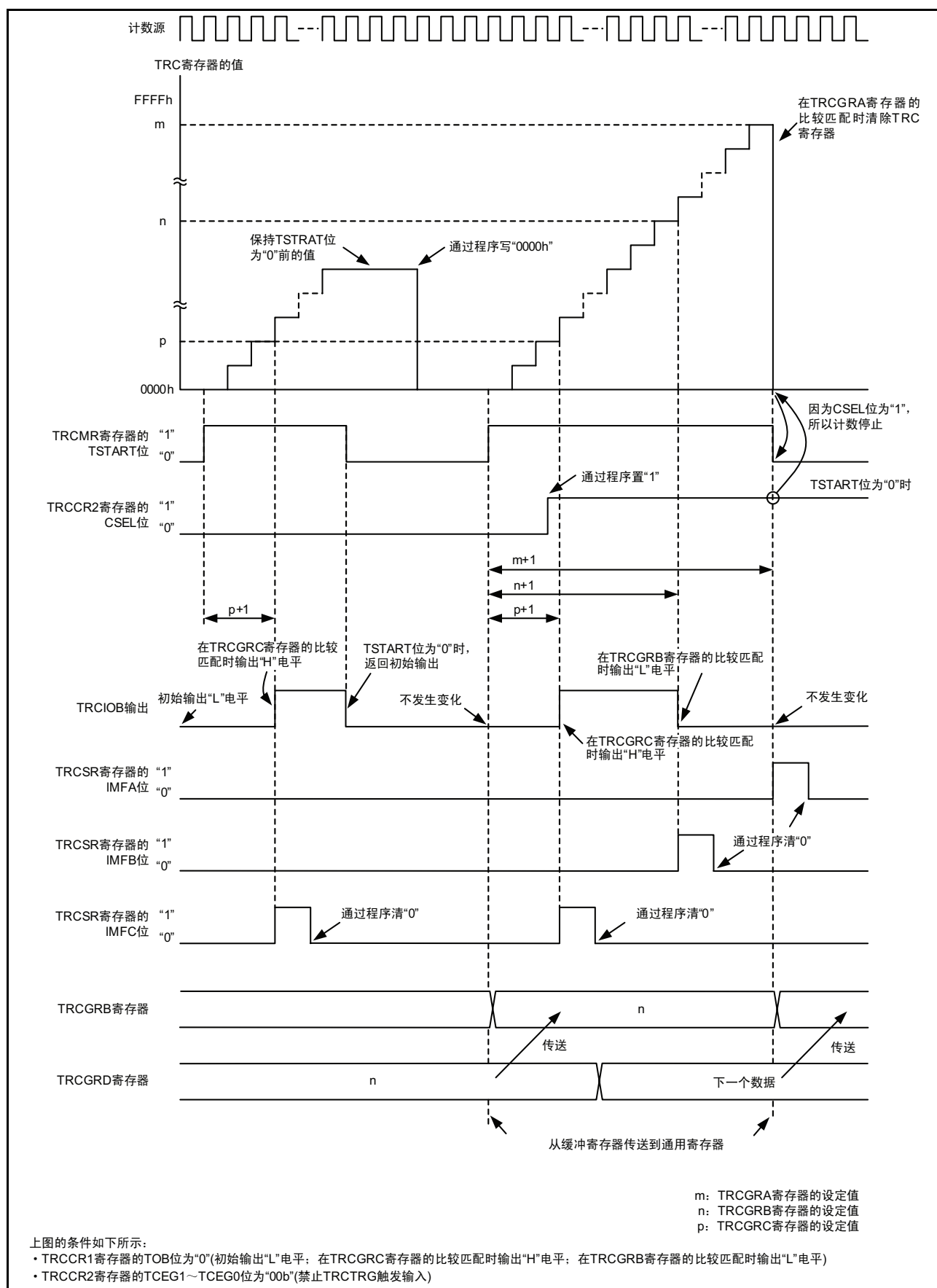
图 15.58 PWM2 的运行例 (禁止 TRCTRG 触发输入时)
