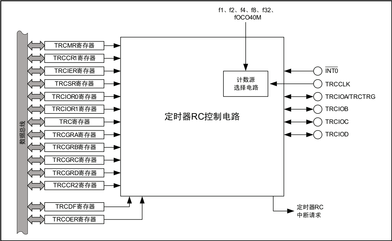
图 15.26 定时器 RC 的框图
