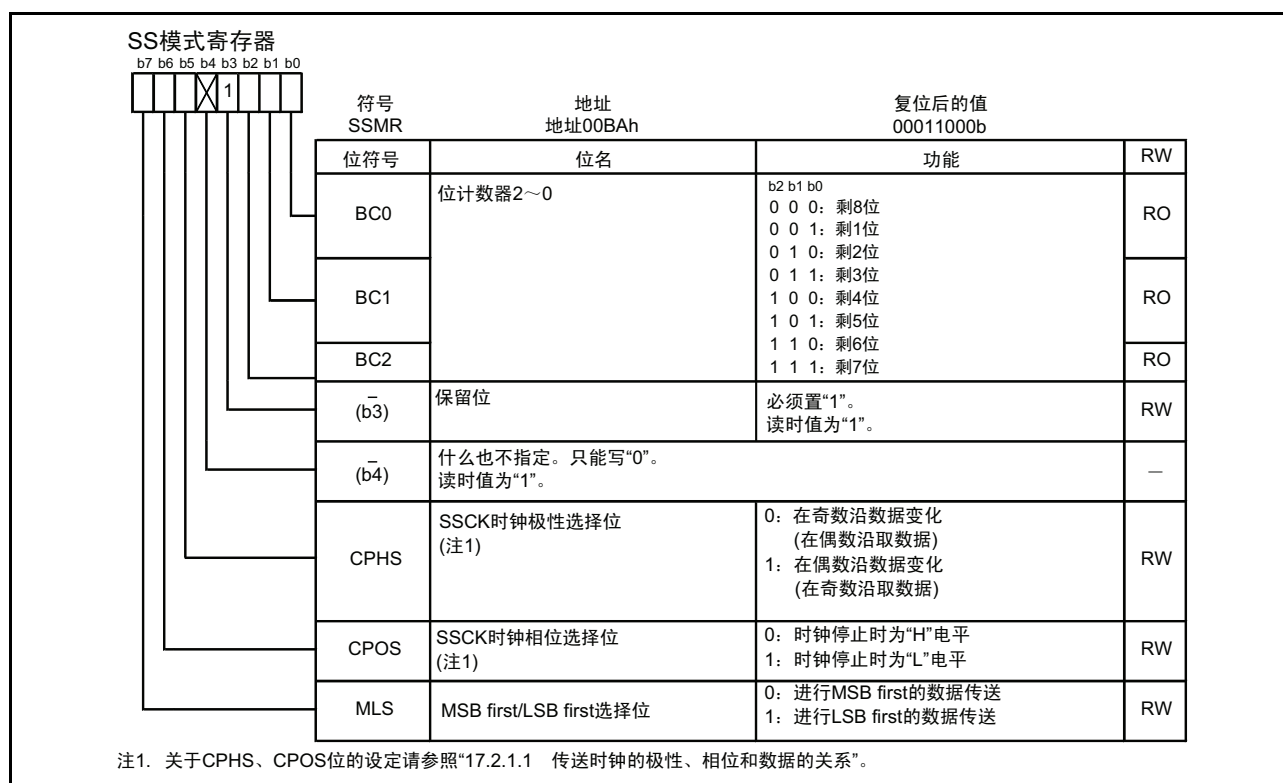
图 17.5 SSMR 寄存器
