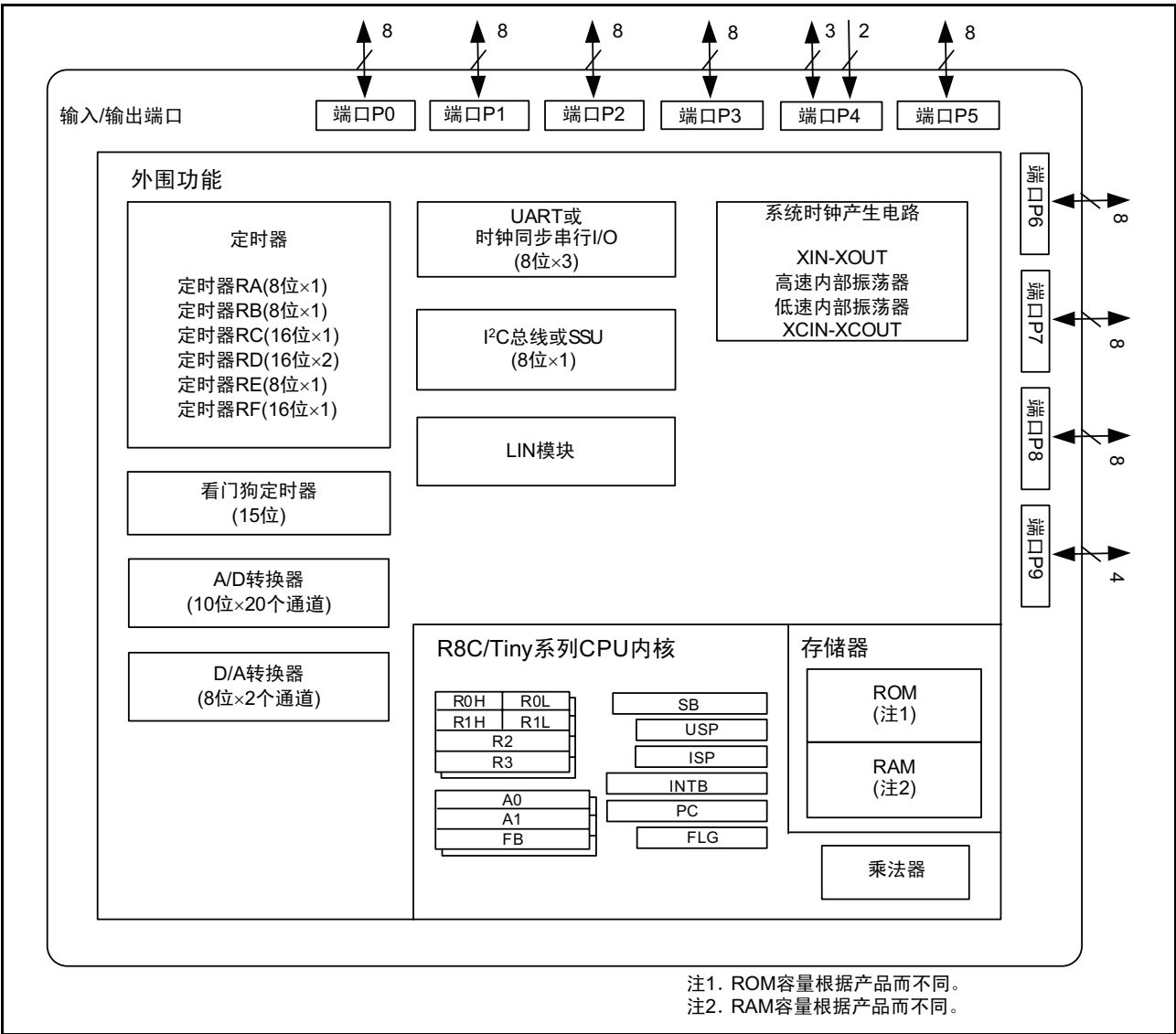
图 1.3 框图
