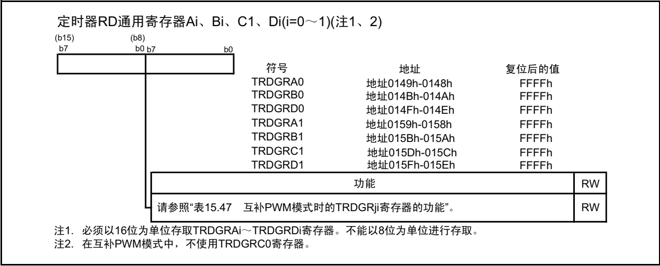
图 15.133 互补 PWM 模式时的 TRDGRAi、TRDGRBi、TRDGRC1、TRDGRDi 寄存器
