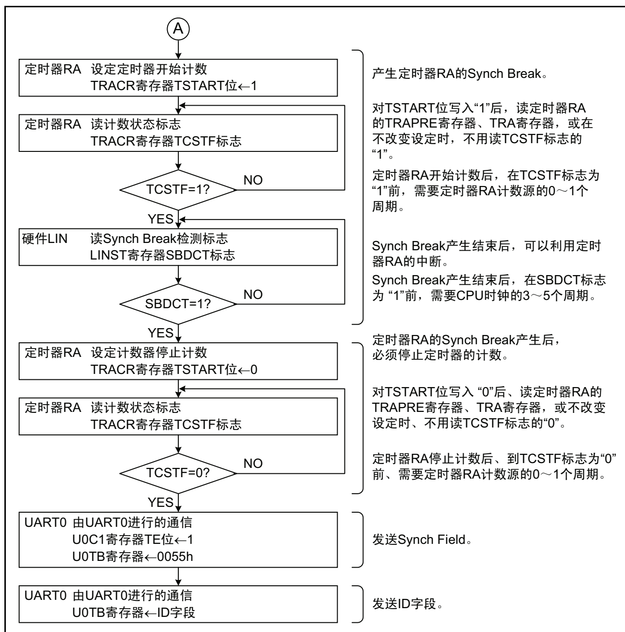
图 18.6 发送头字段的流程图的例子 (2)
