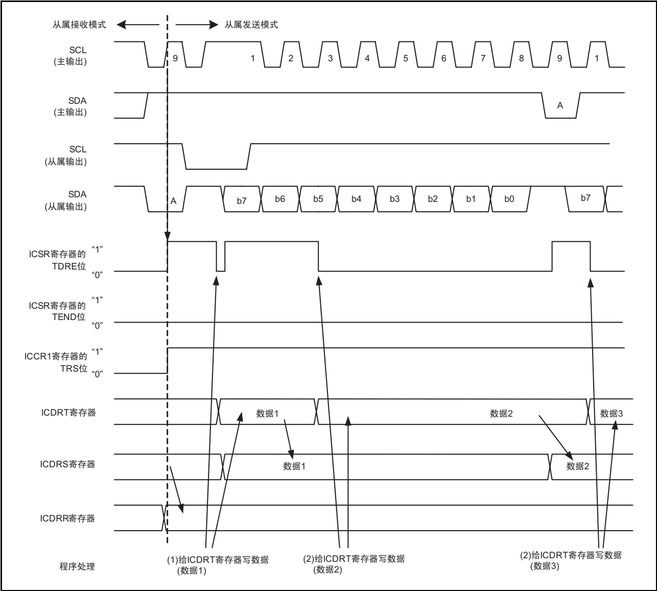
图 17.38 从属发送模式的运行时序 (I 2 C 总线接口模式) (1)
