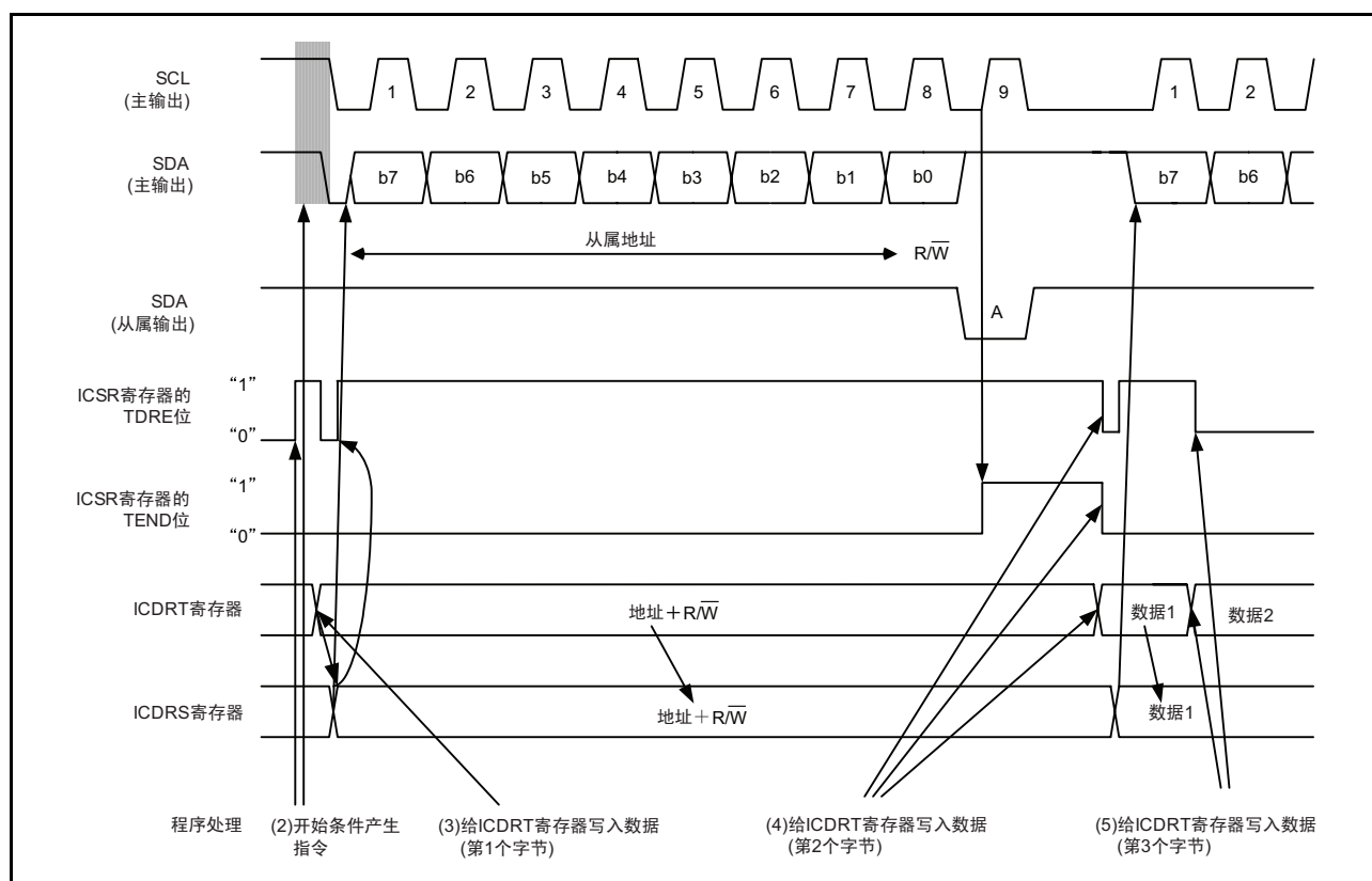
图 17.34 主发送模式的运行时序 (I2C 总线接口模式) (1)
