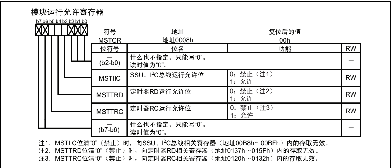
图 17.25 MSTCR 寄存器
