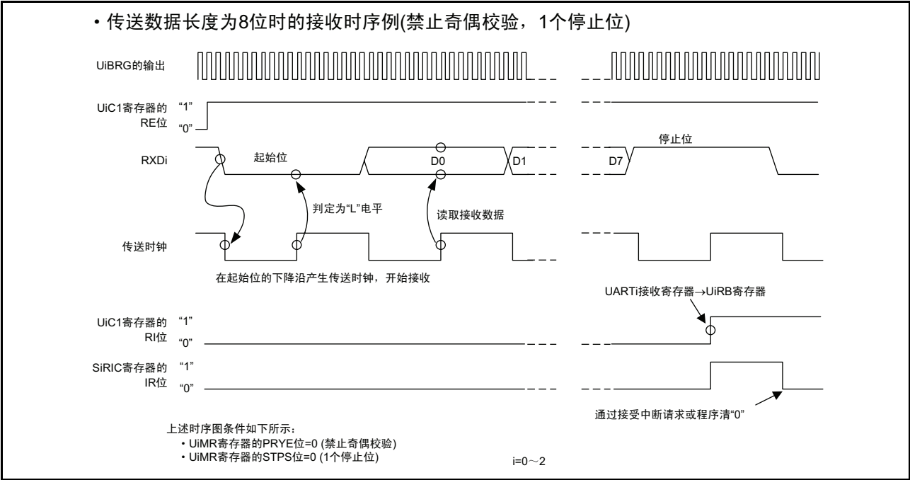
图 16.13 UART 模式时的接收时序例
