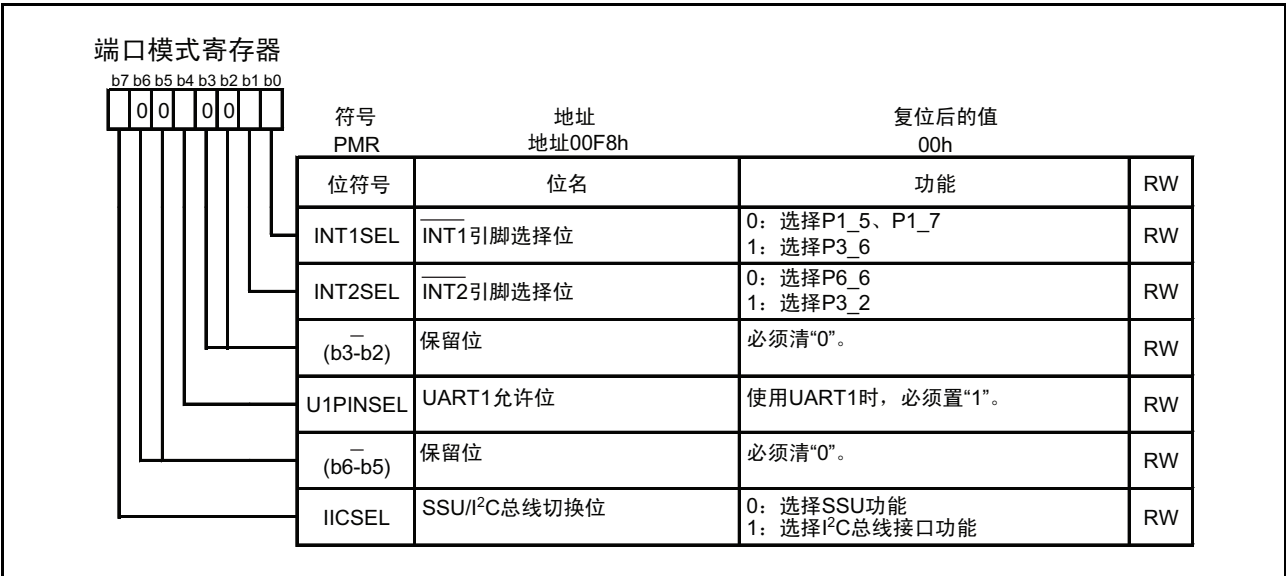
图 8.16 PMR 寄存器
