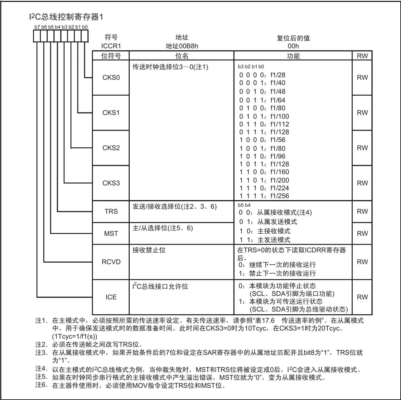
图 17.26 ICCR1 寄存器
