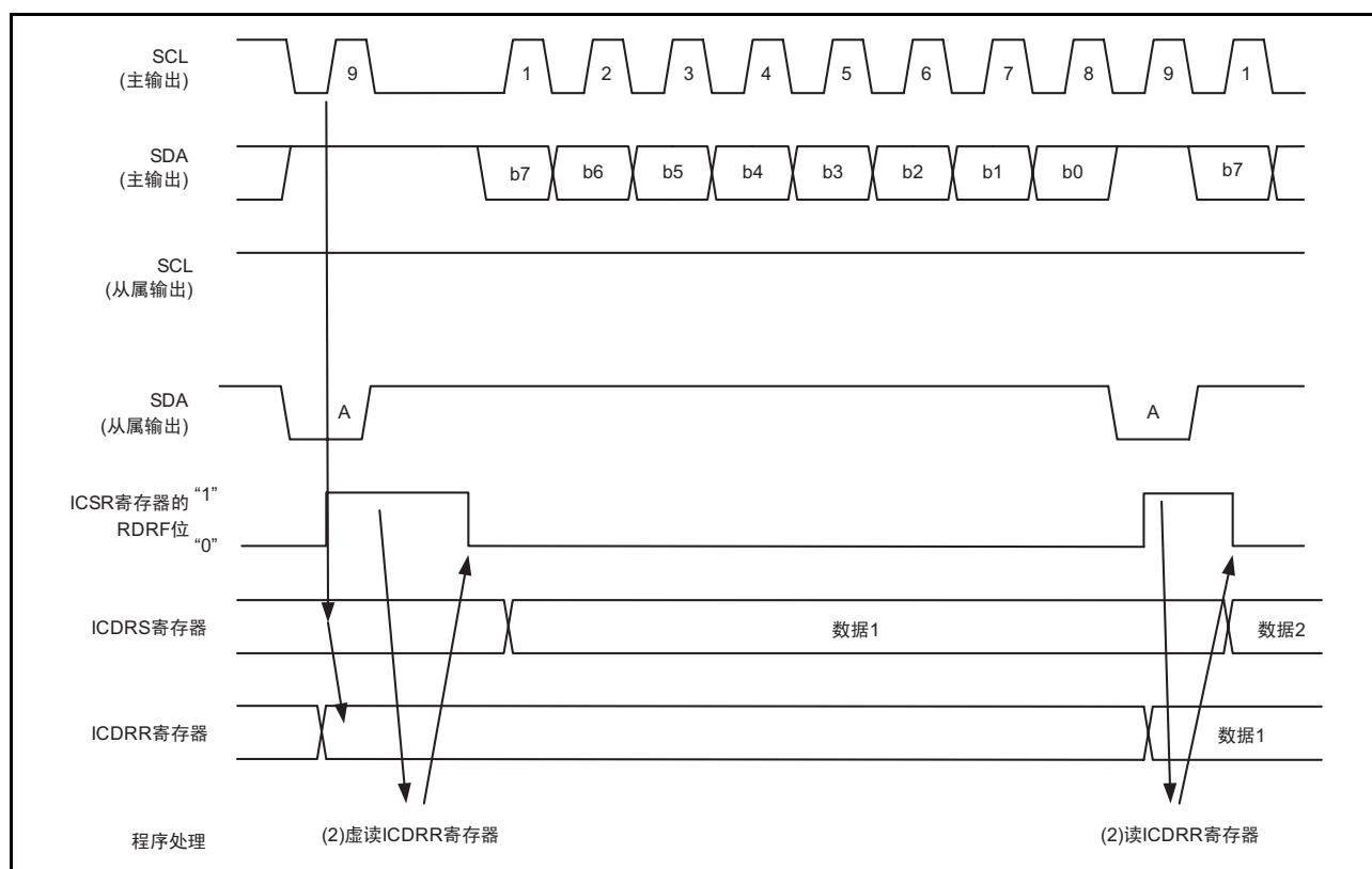
图 17.40 从属接收模式的运行时序（I 2 C 总线接口模式）（1）
