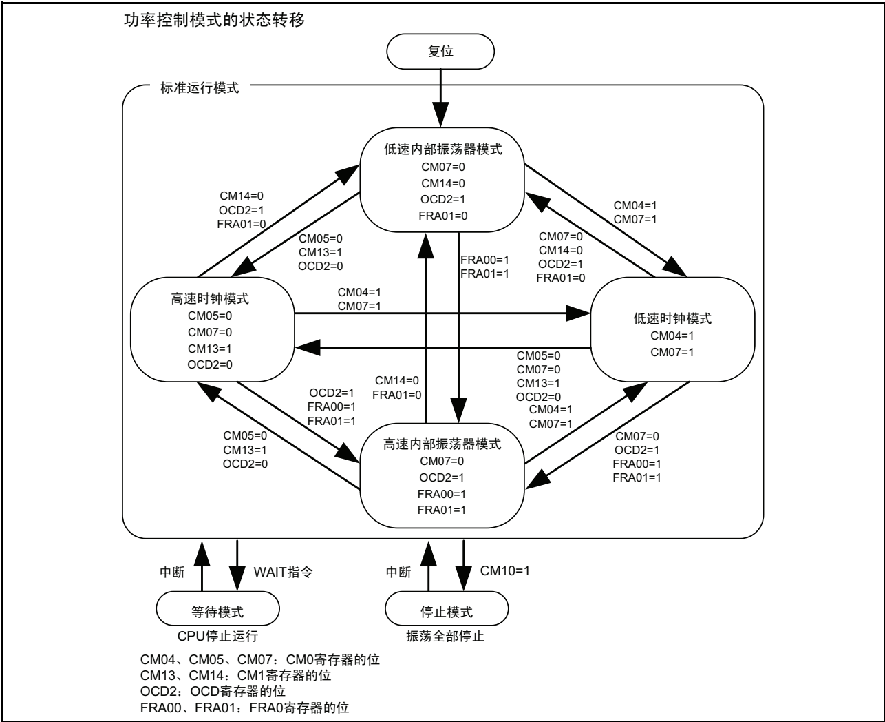
图 11.16 功率控制的状态转移
