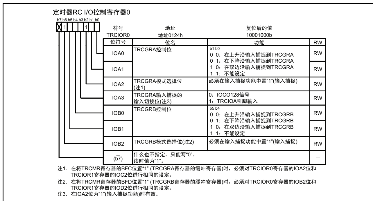
图 15.44 输入捕捉功能时的 TRCIOR0 寄存器
