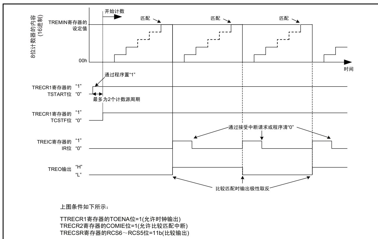
图 15.168 输出比较模式的运行例
