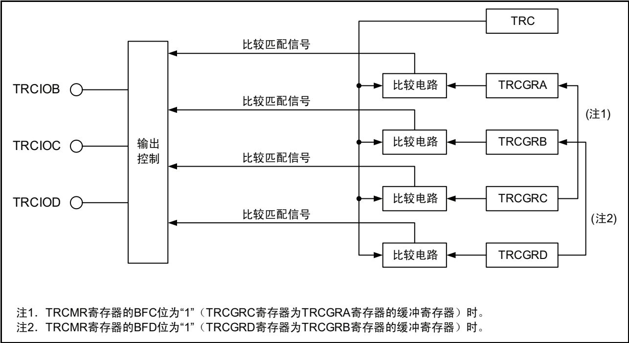
图 15.52 PWM 模式的框图
