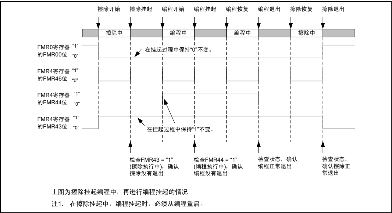
图 21.8 有关挂起运行的时序
