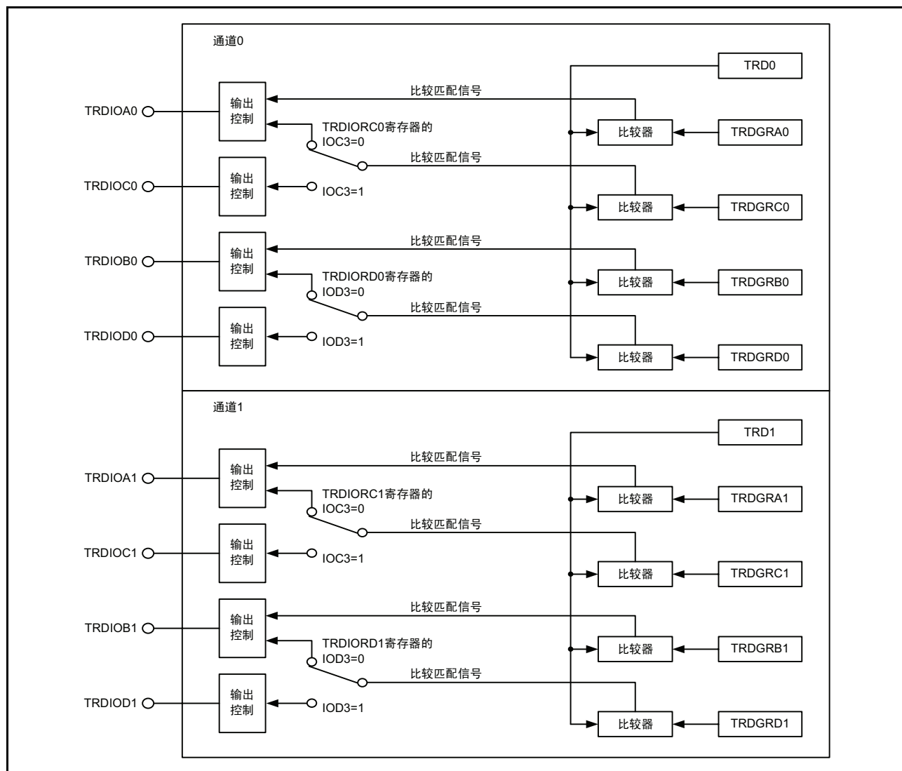
图 15.98 TRDGRCi、TRDGRDi 的输出引脚改变
