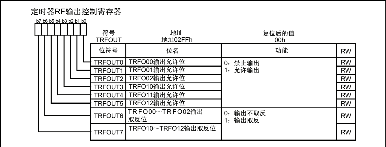
图 15.176 TRFOUT 寄存器
