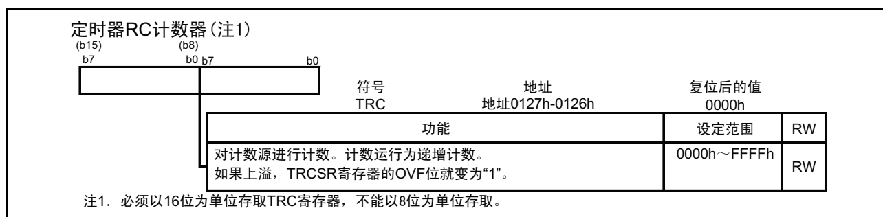
图 15.32 TRC 寄存器
