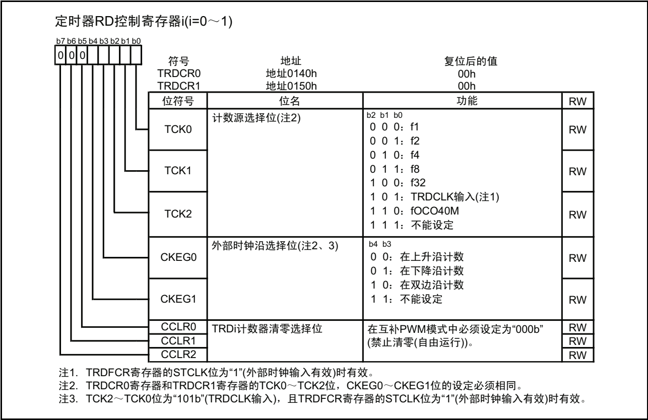
图 15.129 互补 PWM 模式时的 TRDCR0 ~ TRDCR1 寄存器
