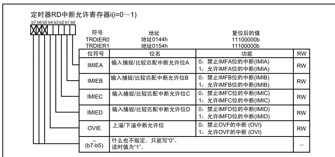
图 15.143 PWM3 模式时的 TRDIER0 ~ TRDIER1 寄存器
