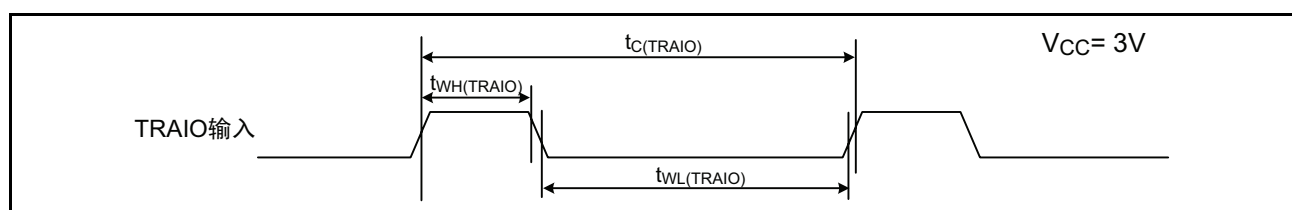
图 22.14 V_{CC}=3V 时的 TRAIO 输入、 \overline{INT1} 输入时序
