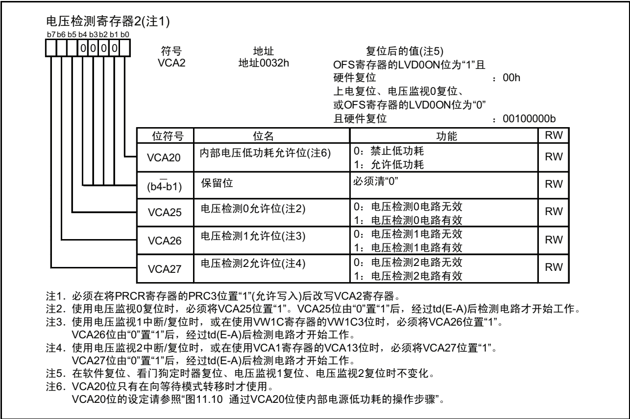
图 11.9 VCA2 寄存器
