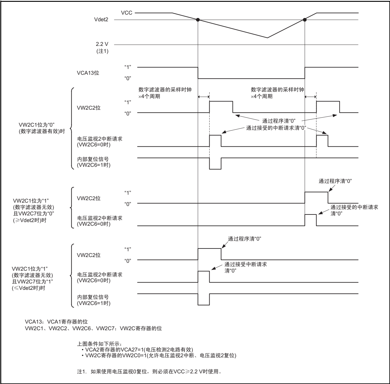
图 7.11 电压监视 2 中断、电压监视 2 复位的运行例
