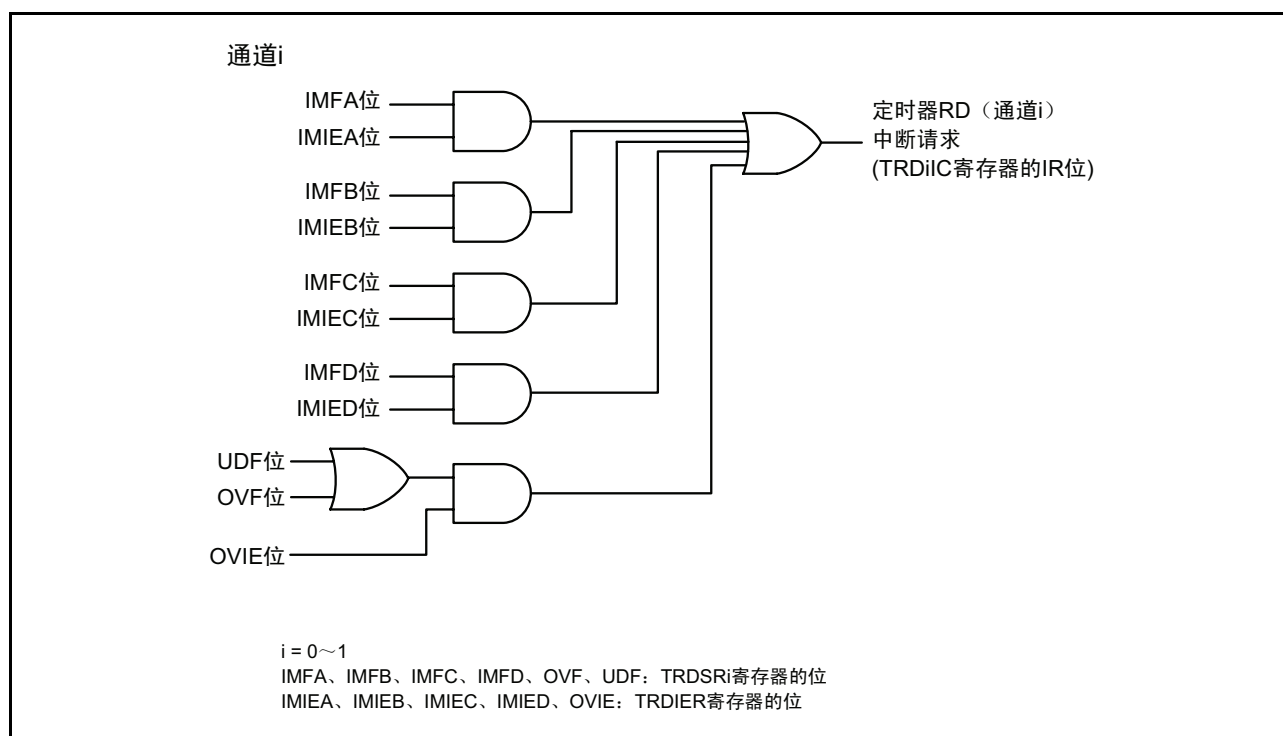
图 13.21 定时器 RD 中断的框图
