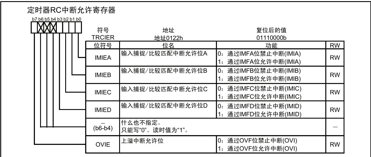
图 15.30 TRCIER 寄存器
