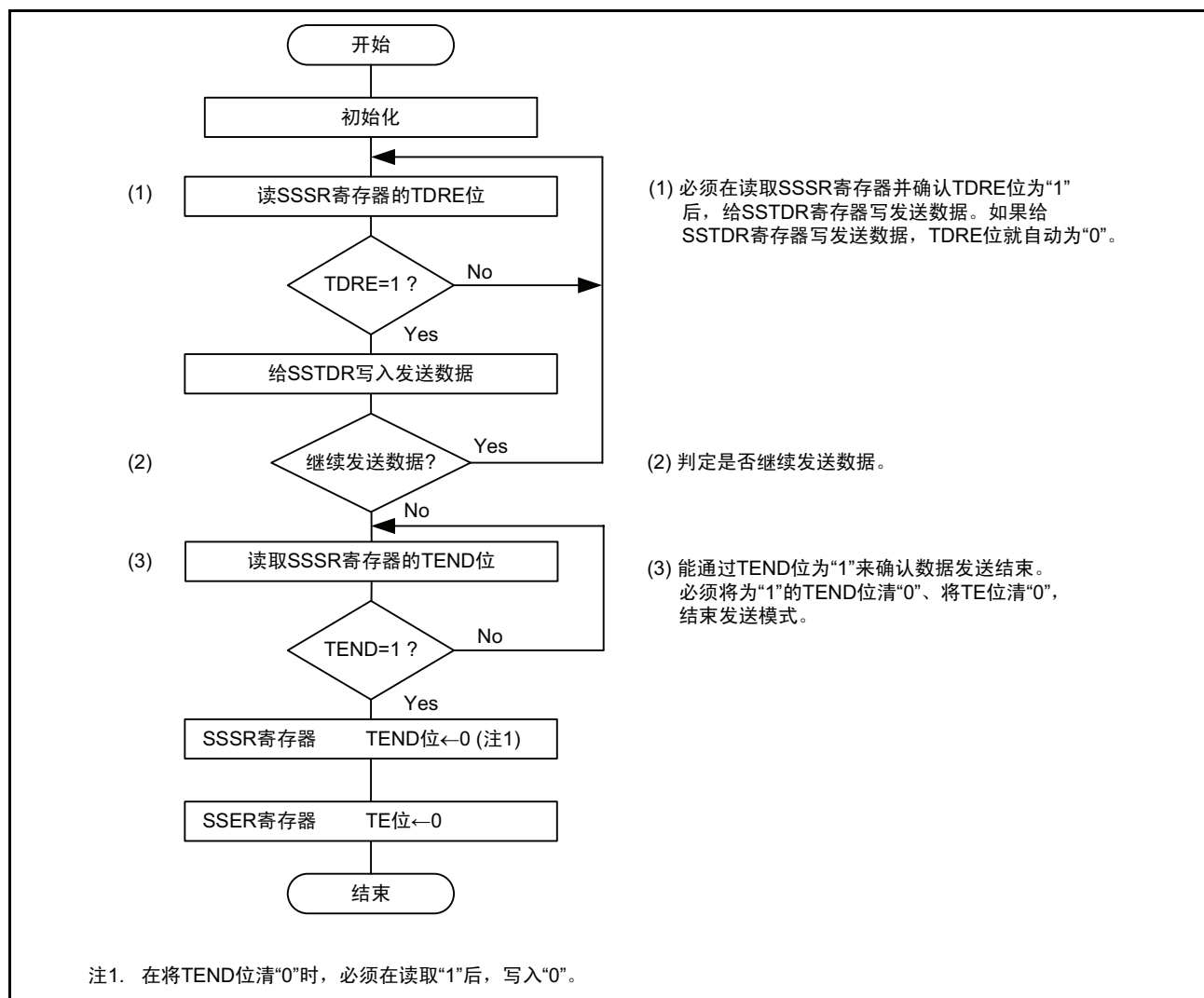
图 17.15 发送数据的流程图的例子（时钟同步通信模式）
