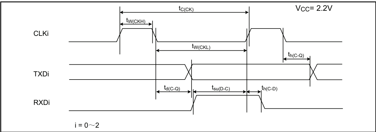
图 22.21 V_{CC}=2.2V 时的串行接口时序
