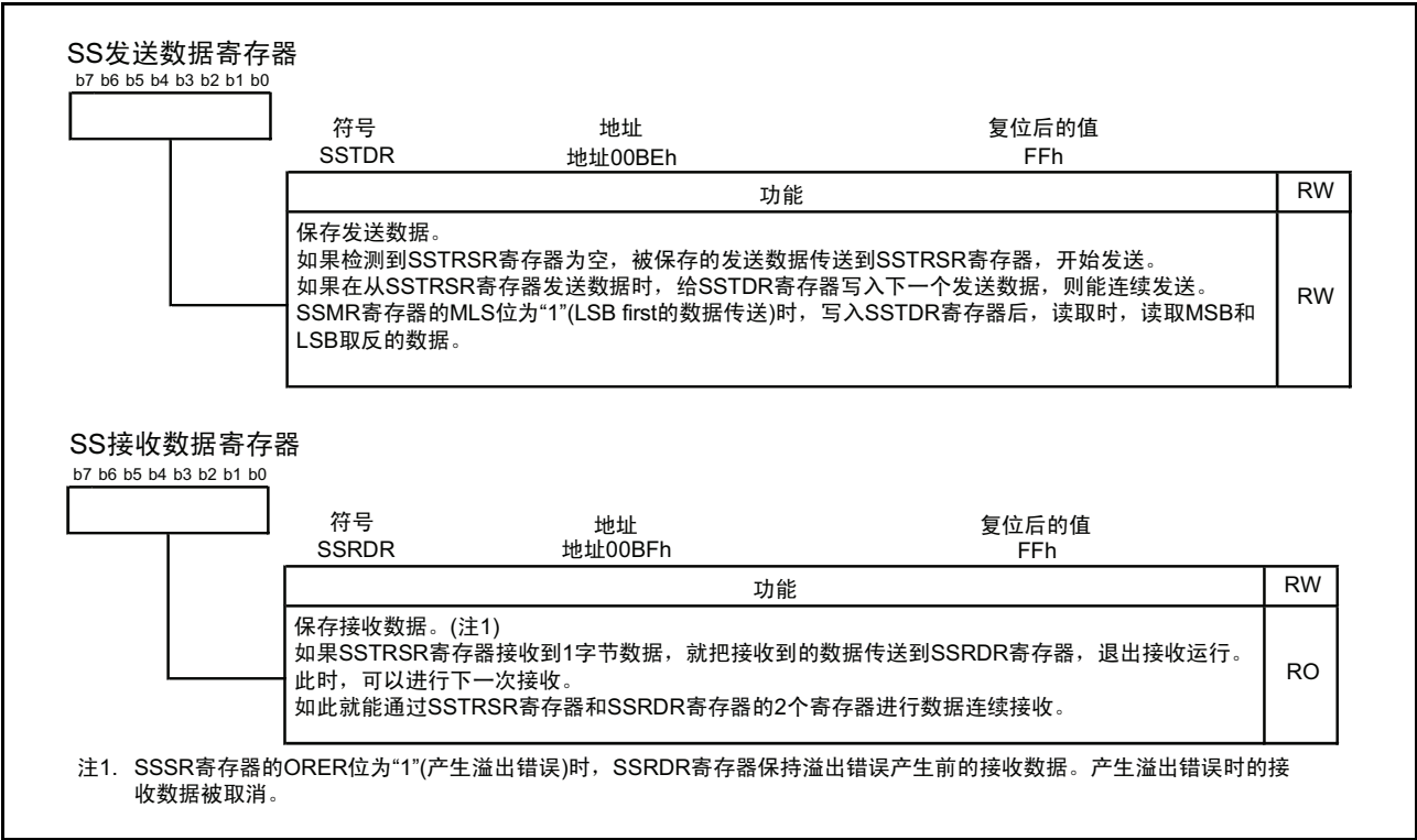
图 17.9 SSTDR、SSRDR 寄存器
