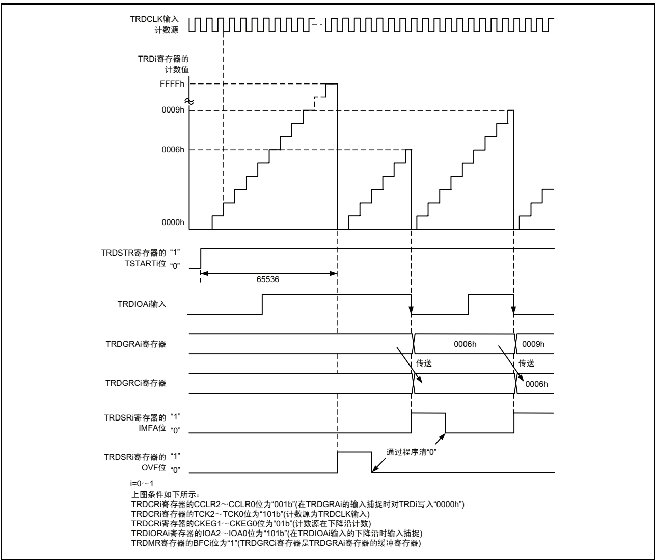
图 15.81 输入捕捉功能的运行例
