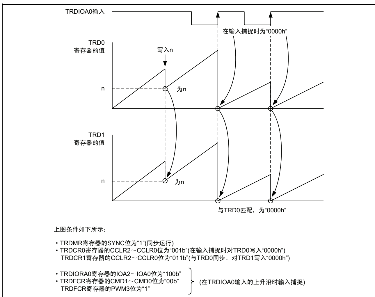
图 15.66 同步运行
