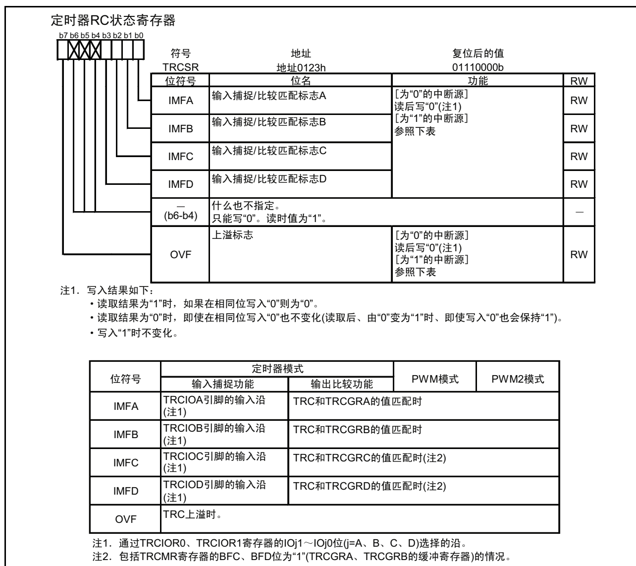
图 15.31 TRCSR 寄存器
