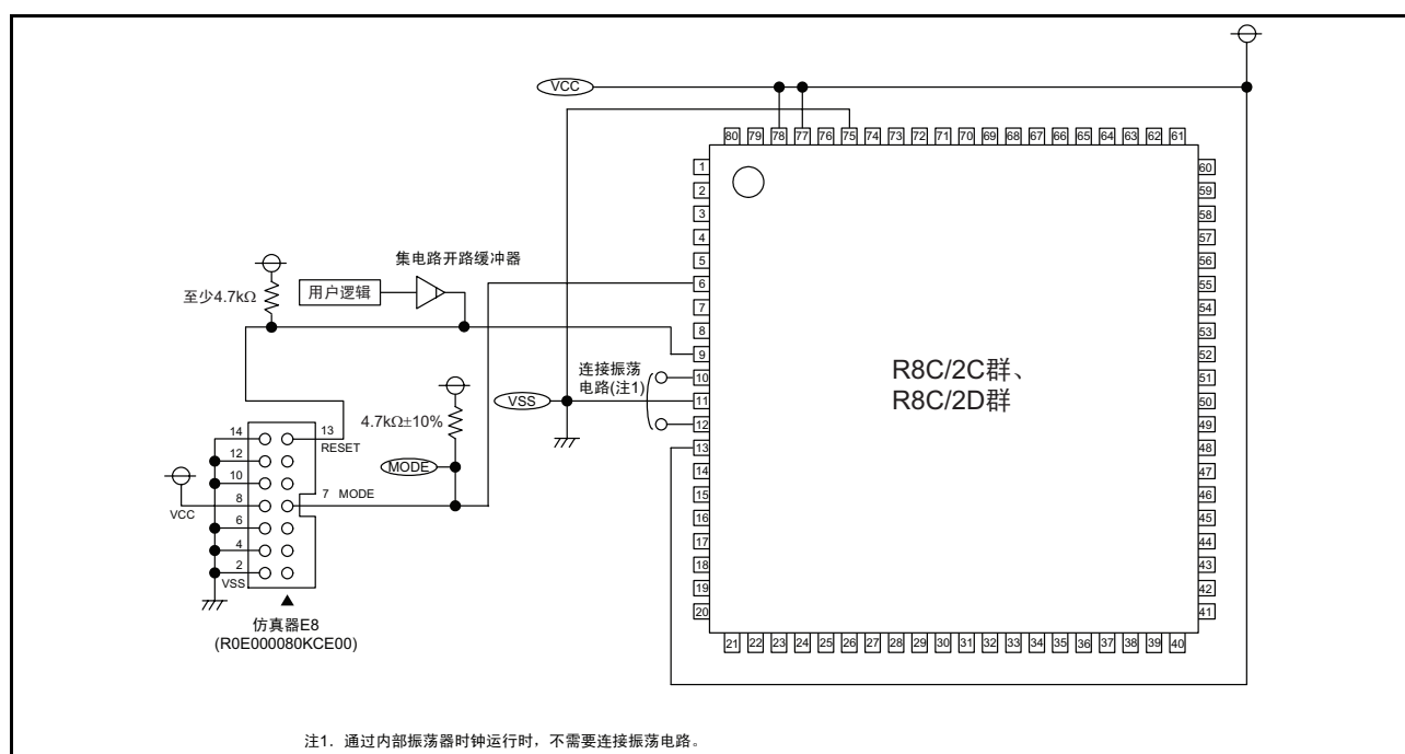
附图 2.2 和仿真器 E8（R0E000080KCE00）的连接例
