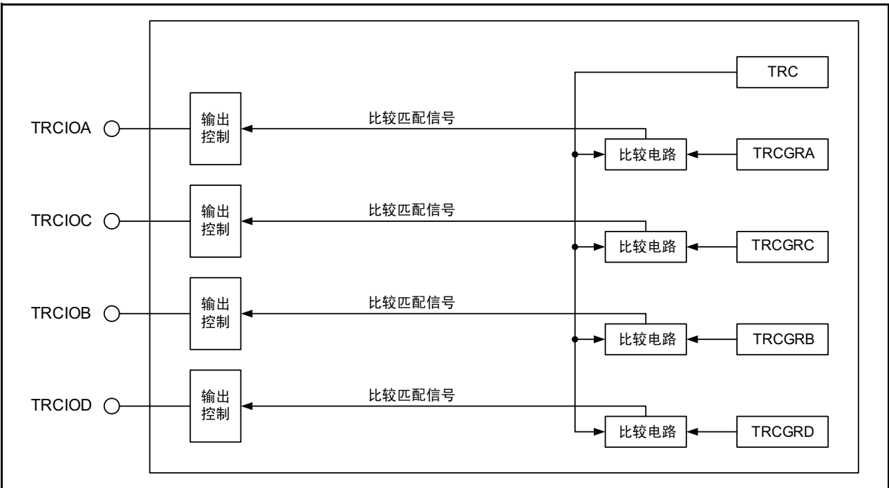
图 15.47 输出比较功能的框图
