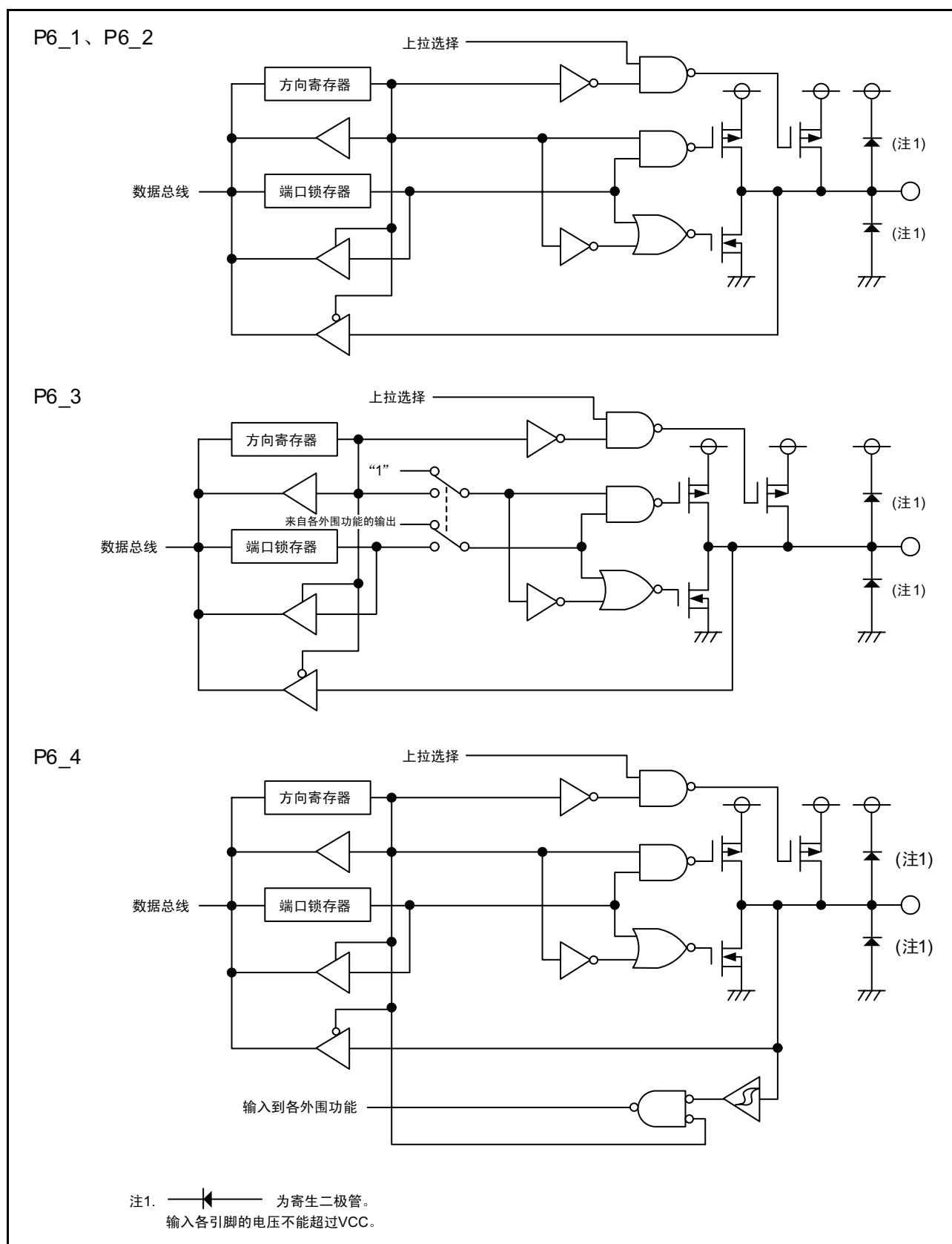
图 8.8 可编程输入 / 输出端口的结构 (8)
