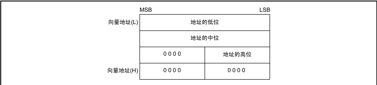
图 13.2 中断向量
