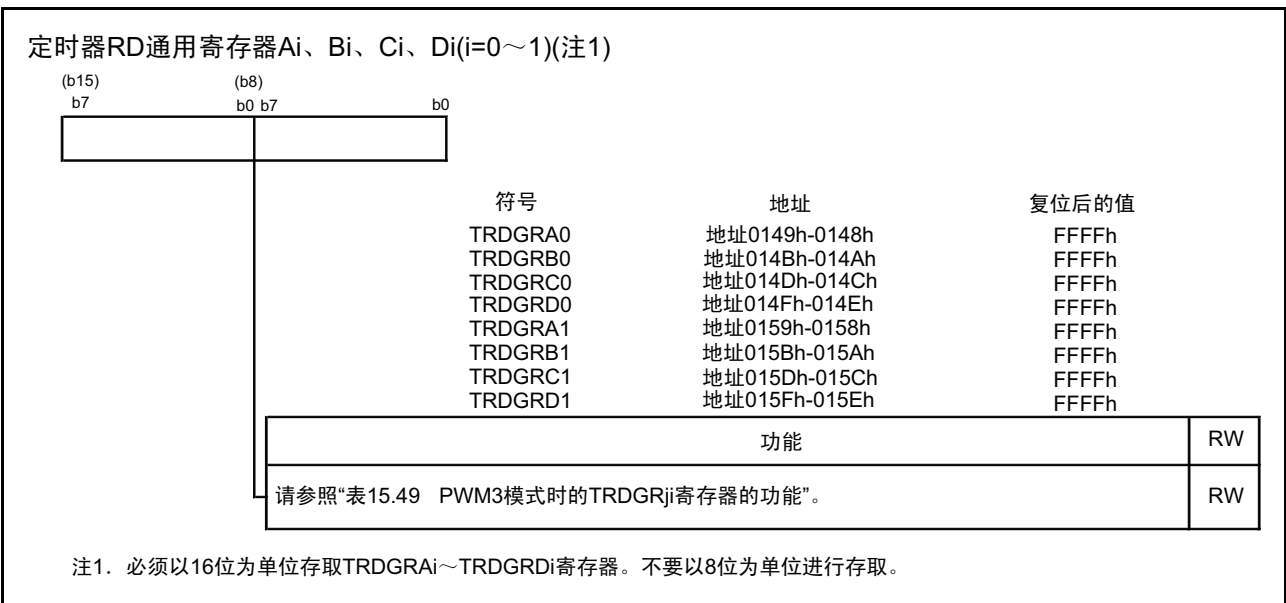
图 15.145 PWM3 模式时的 TRDGRAi、TRDGRBi、TRDGRCi、TRDGRDi 寄存器
