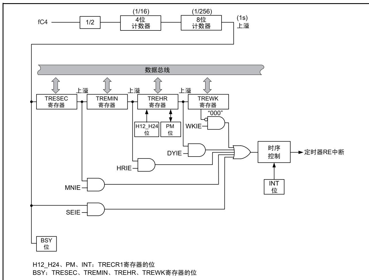
图 15.152 实时时钟模式的框图
