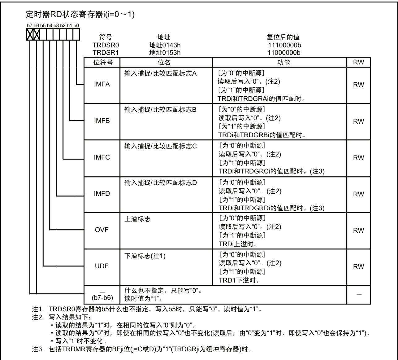
图 15.130 互补 PWM 模式时的 TRDSR0 ~ TRDSR1 寄存器
