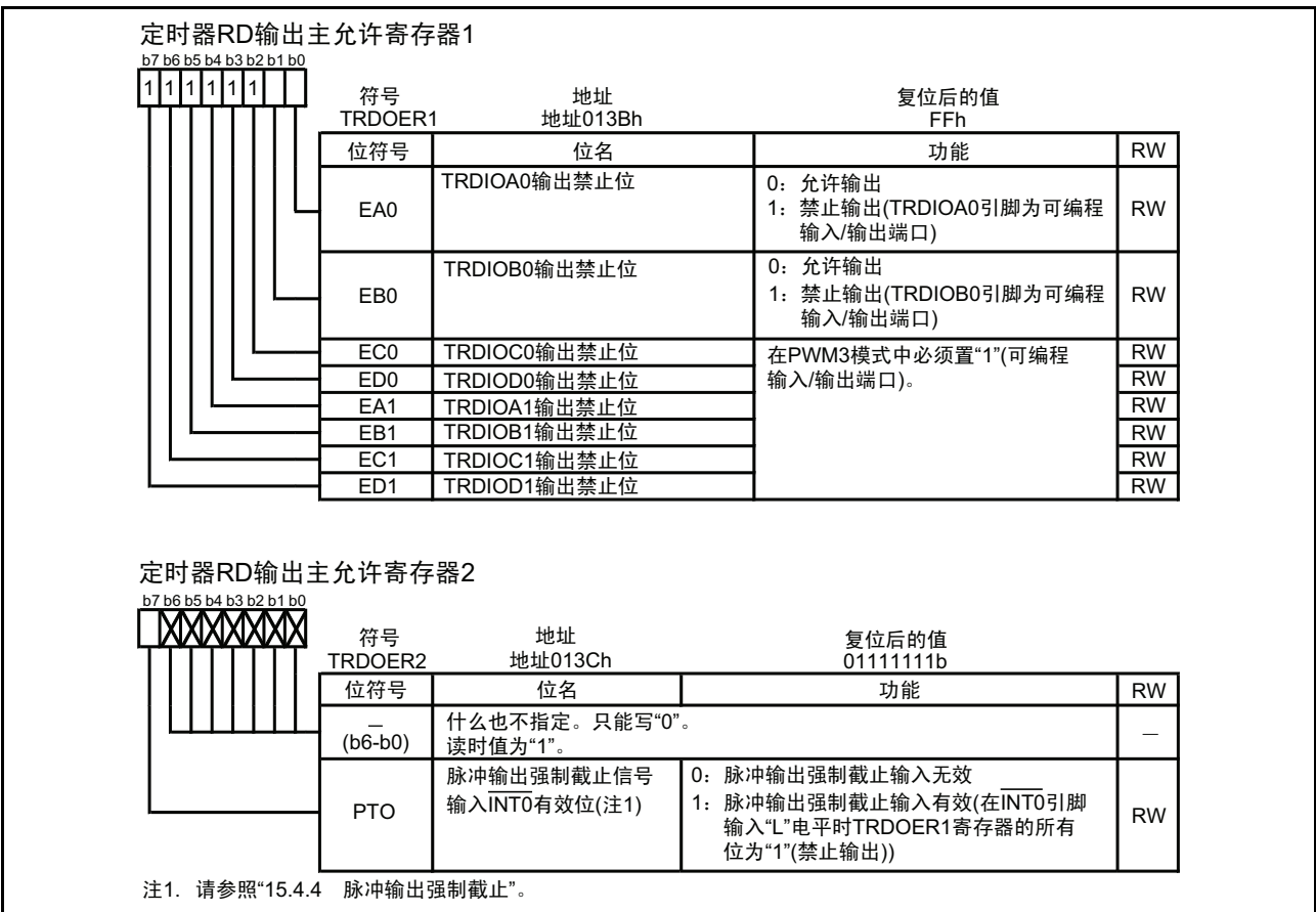
图 15.140 PWM3 模式时的 TRDOER1 ~ TRDOER2 寄存器
