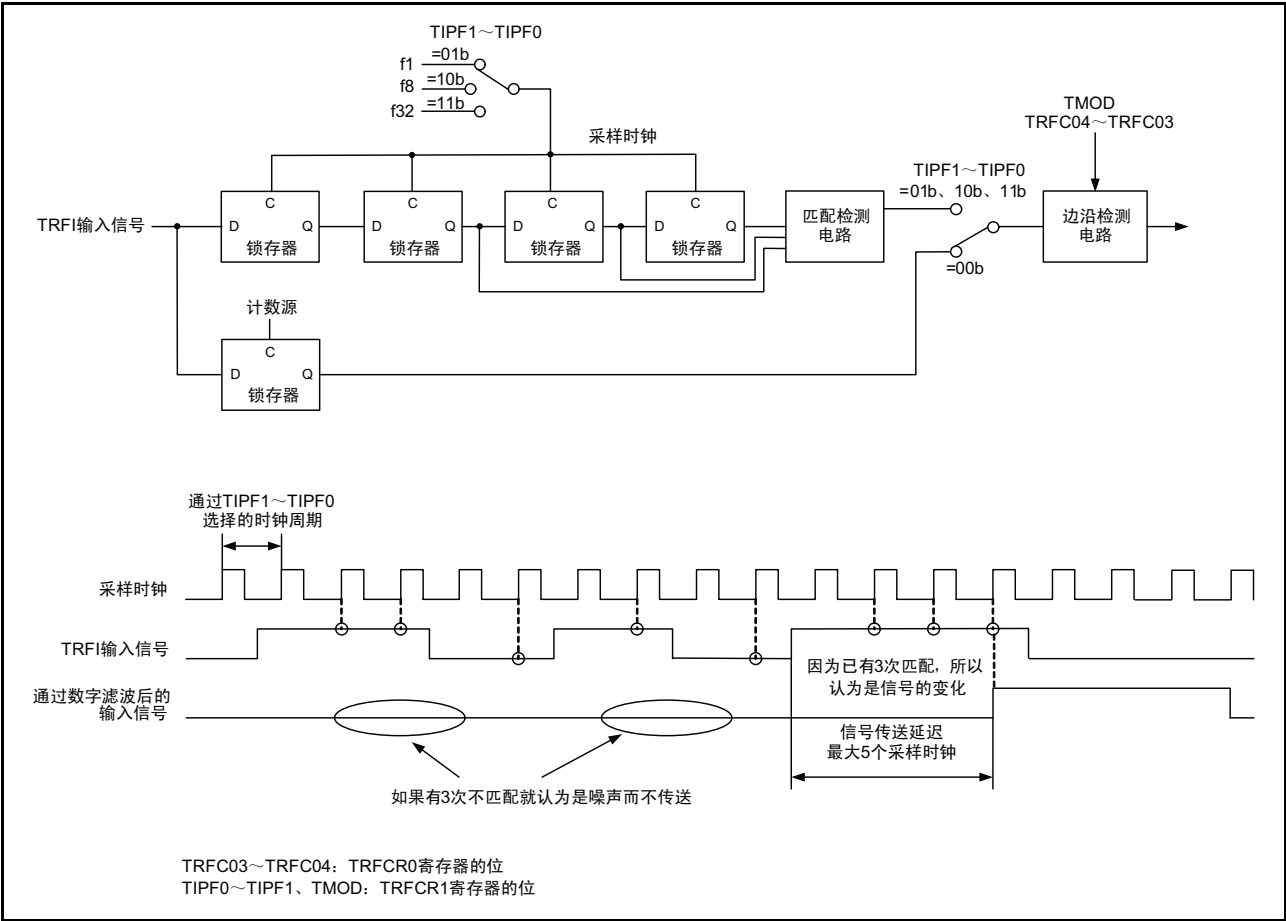
图 15.178 数字滤波器
