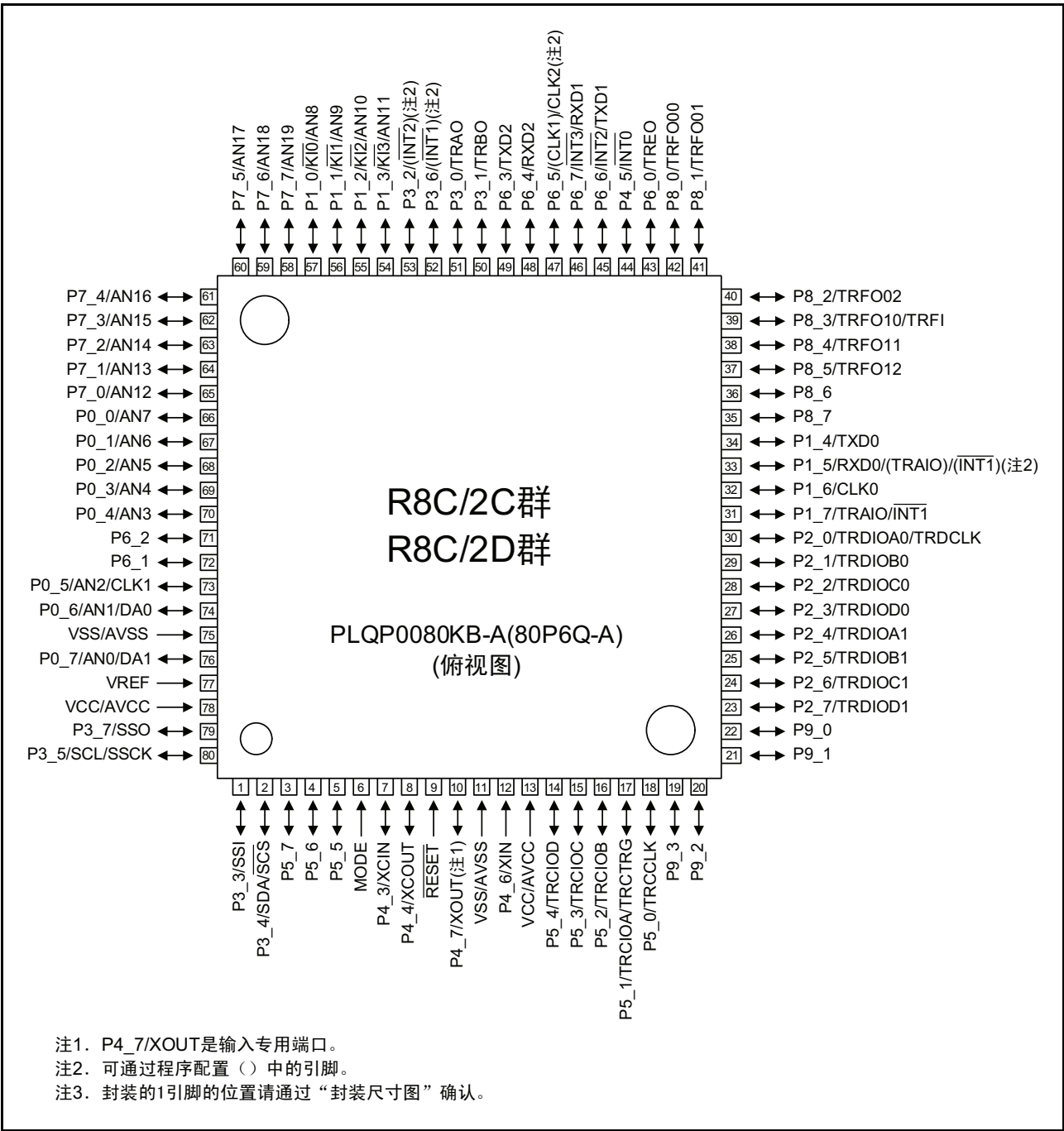
图 1.4 引脚配置图（俯视图）
