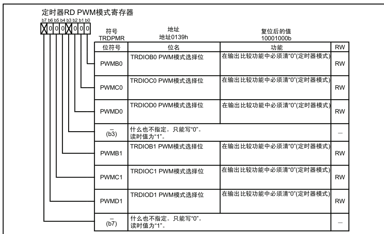
图 15.86 输出比较功能时的 TRDPMR 寄存器
