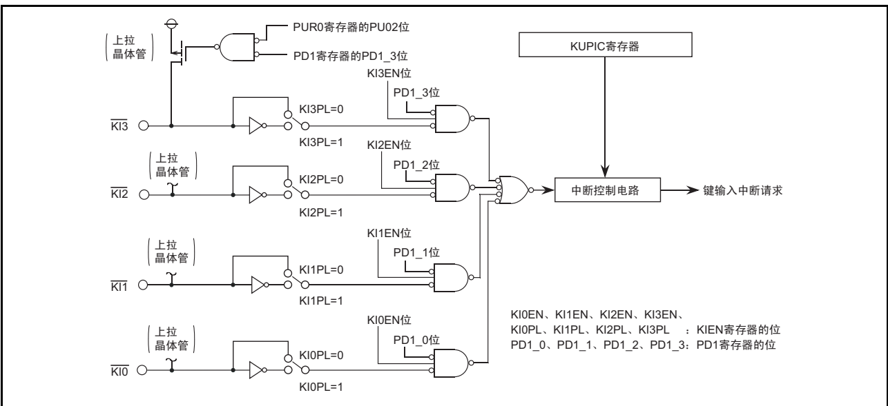
图 13.18 键输入中断的框图
