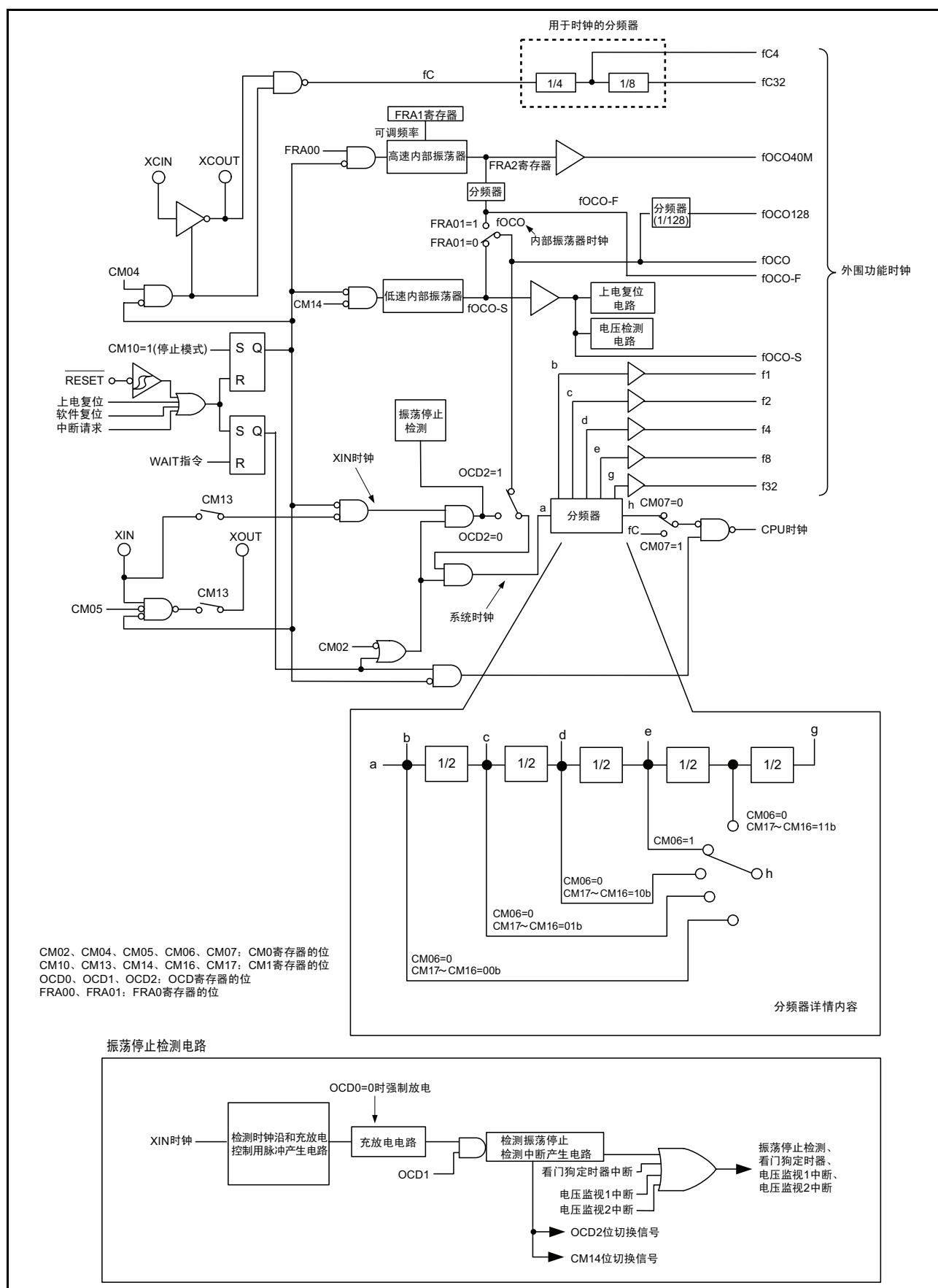
图 11.1 时钟产生电路
