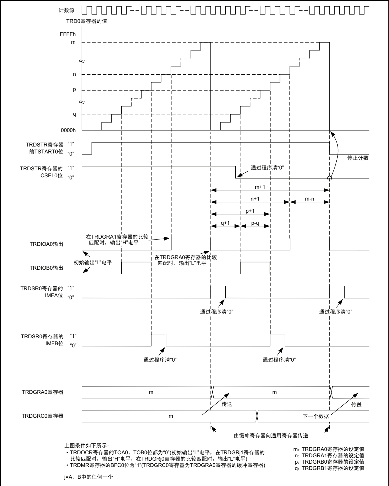
图 15.146 PWM3 模式的运行例
