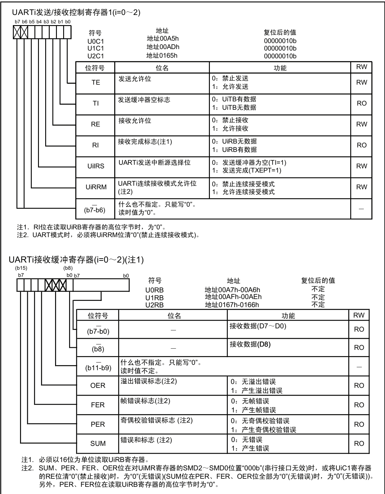
图 16.6 U0C1 ~ U2C1、U0RB ~ U2RB 寄存器
