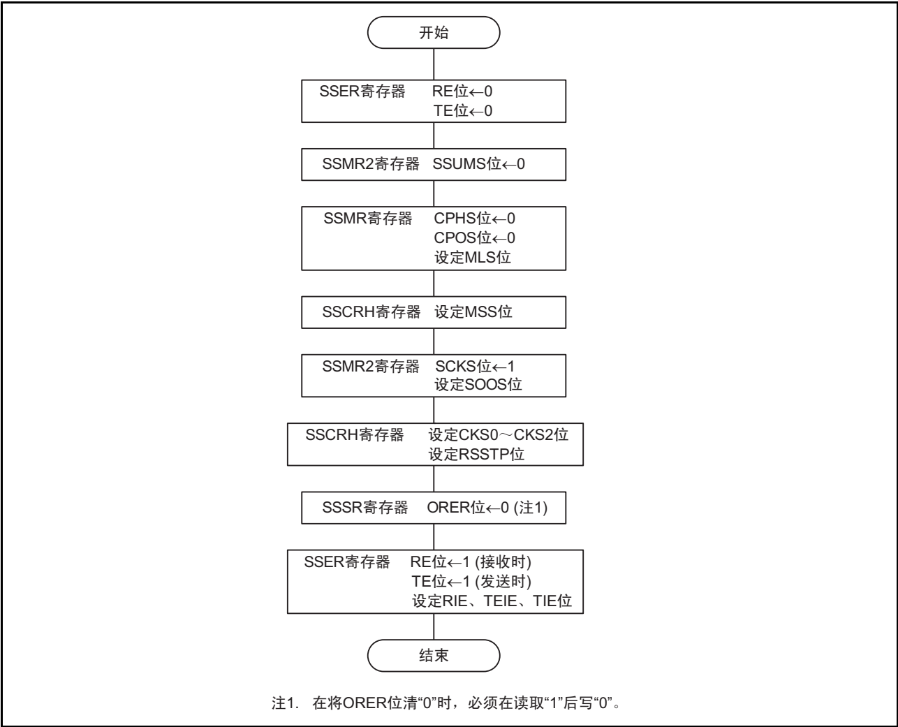
图 17.13 时钟同步通信模式的初始化
