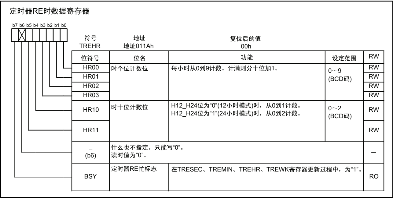
图 15.155 实时时钟模式时的 TREHR 寄存器
