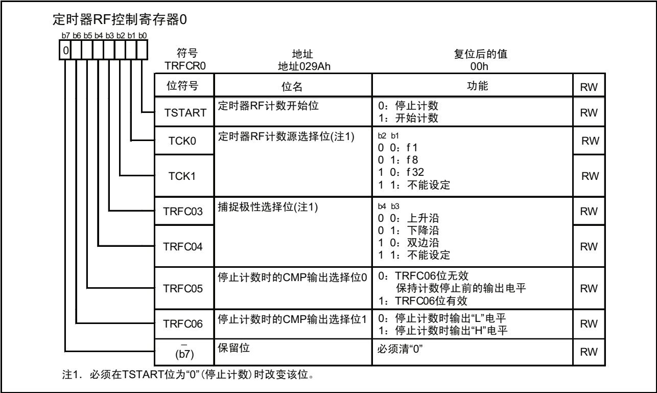
图 15.174 TRFCR0 寄存器
