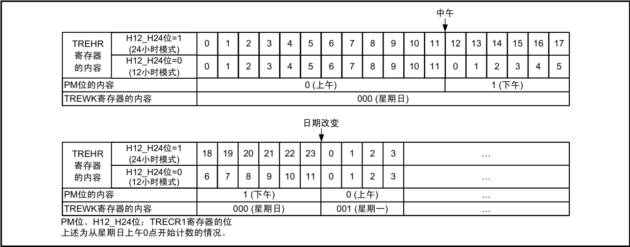
图 15.158 时间显示的定义
