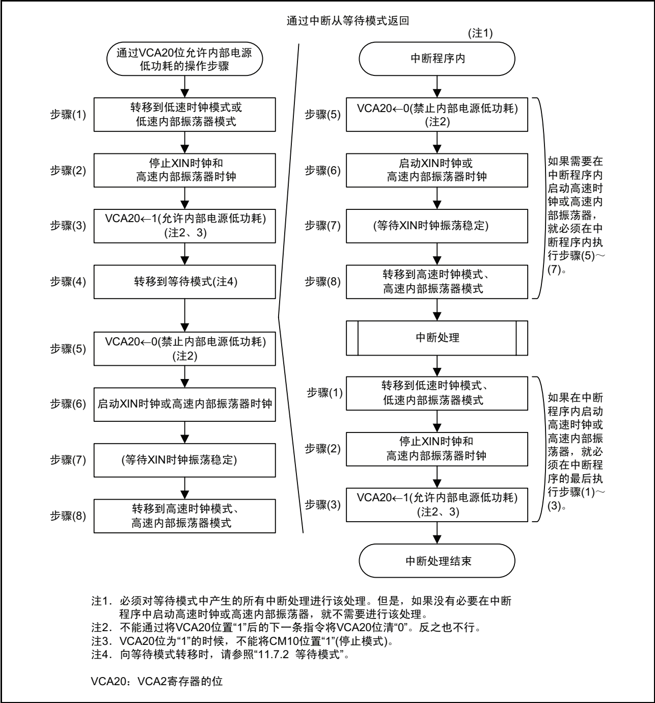
图 11.14 通过 VCA20 位使内部电源低功耗的操作步骤
