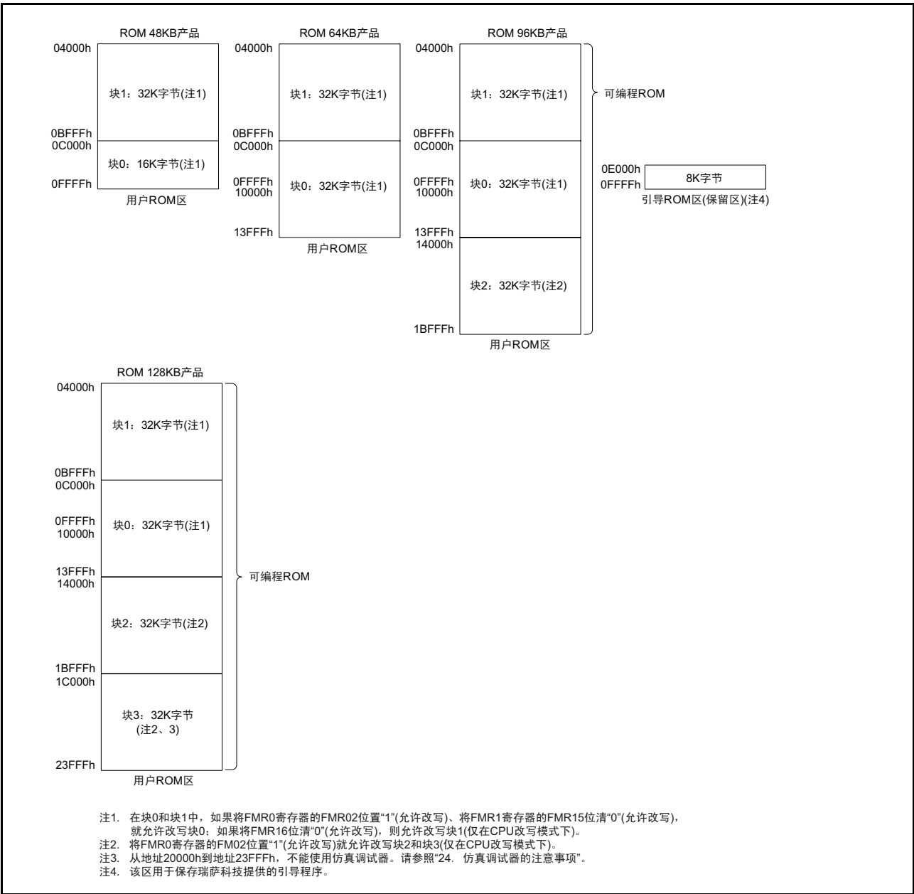
图 21.1 R8C/2C 群的闪存框图
