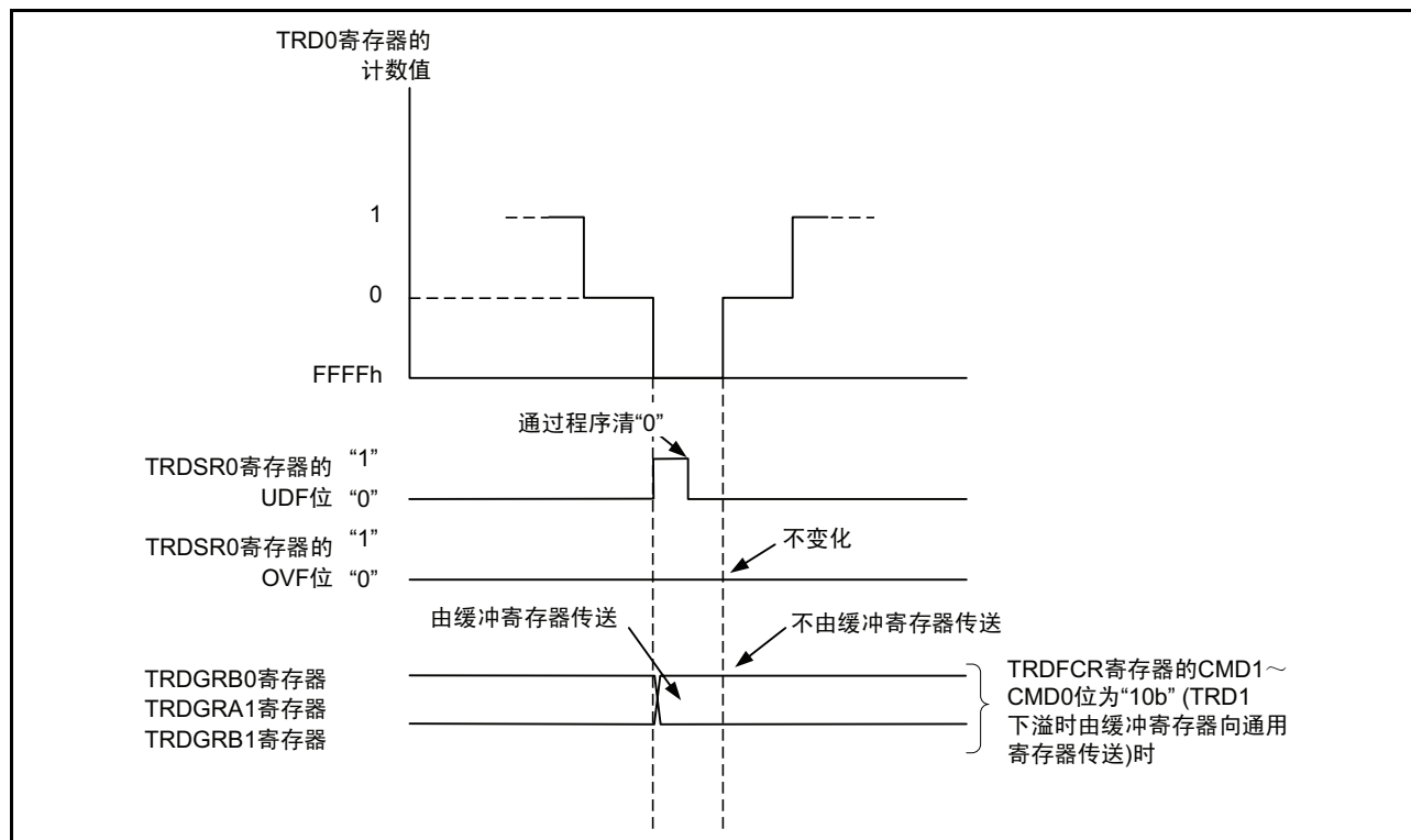
图 2.5 互补 PWM 模式 TRD1 下溢时的运行
