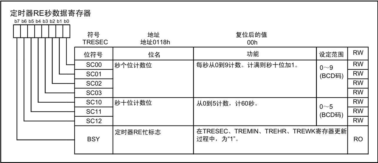
图 15.153 实时时钟模式时的 TRESEC 寄存器
