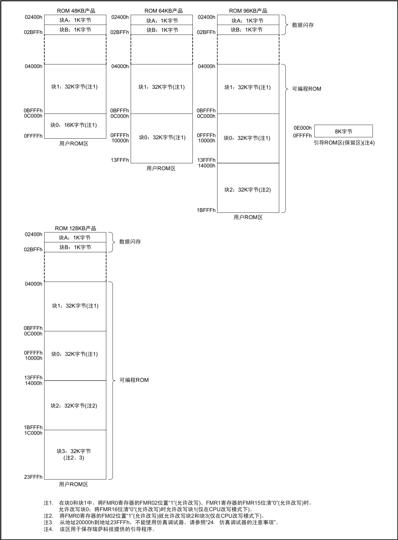
图 21.2 R8C/2D 群的闪存框图
