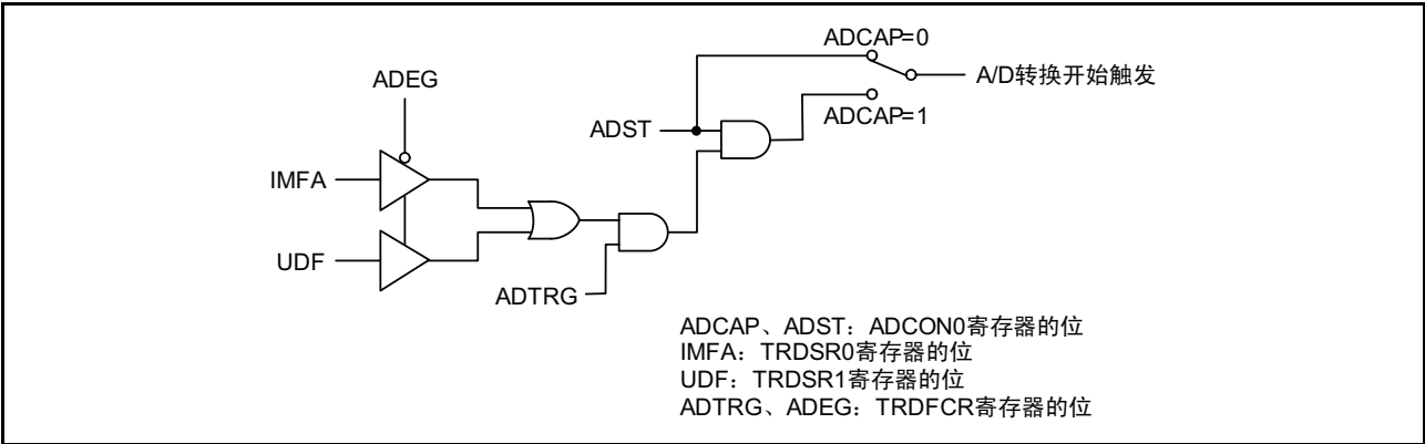
图 19.7 A/D 转换开始控制部的框图
