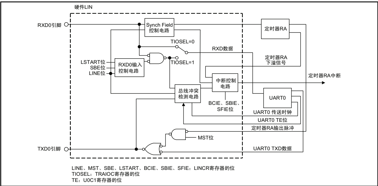
图 18.1 硬件 LIN 的框图
