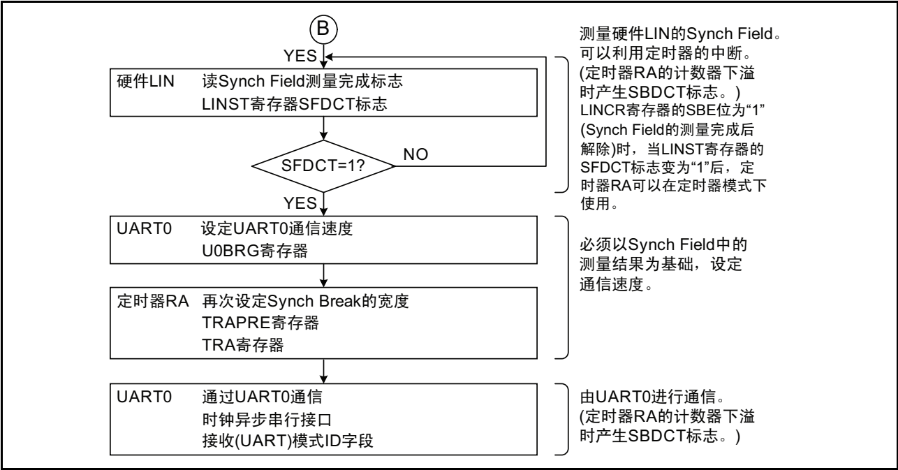
图 18.10 接收头字段的流程图的例子 (3)
