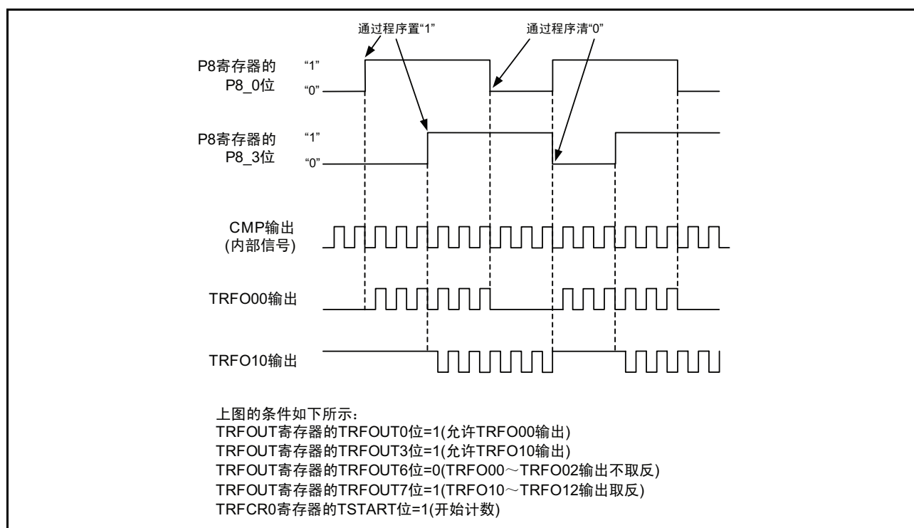
图 15.180 输出比较模式的运行例（计数过程中固定输出“L”电平和“H”电平）
