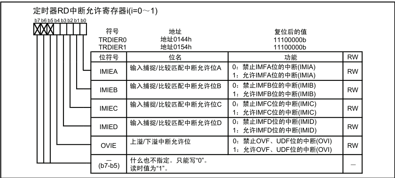
图 15.131 互补 PWM 模式时的 TRDIER0 ~ TRDIER1 寄存器
