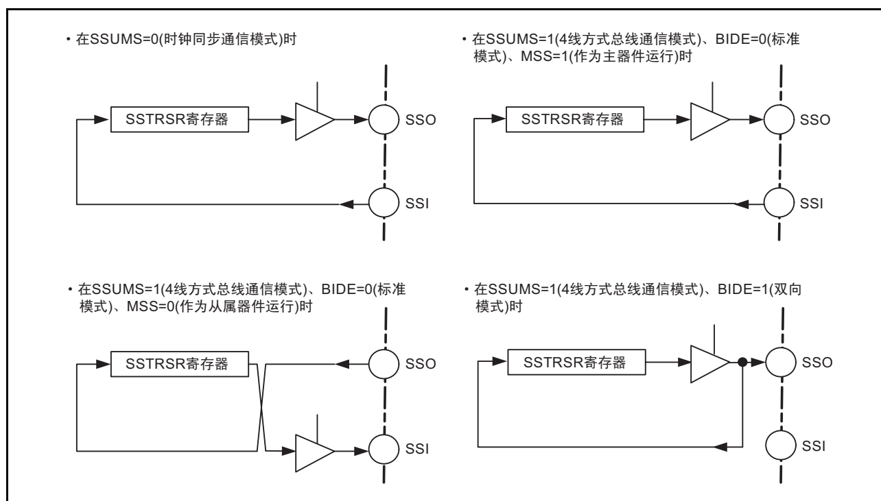
图 17.12 数据输入 / 输出引脚和 SSTRSR 寄存器的连接关系
