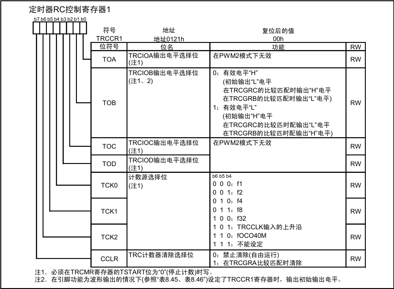
图 15.57 PWM2 模式时的 TRCCR1 寄存器
