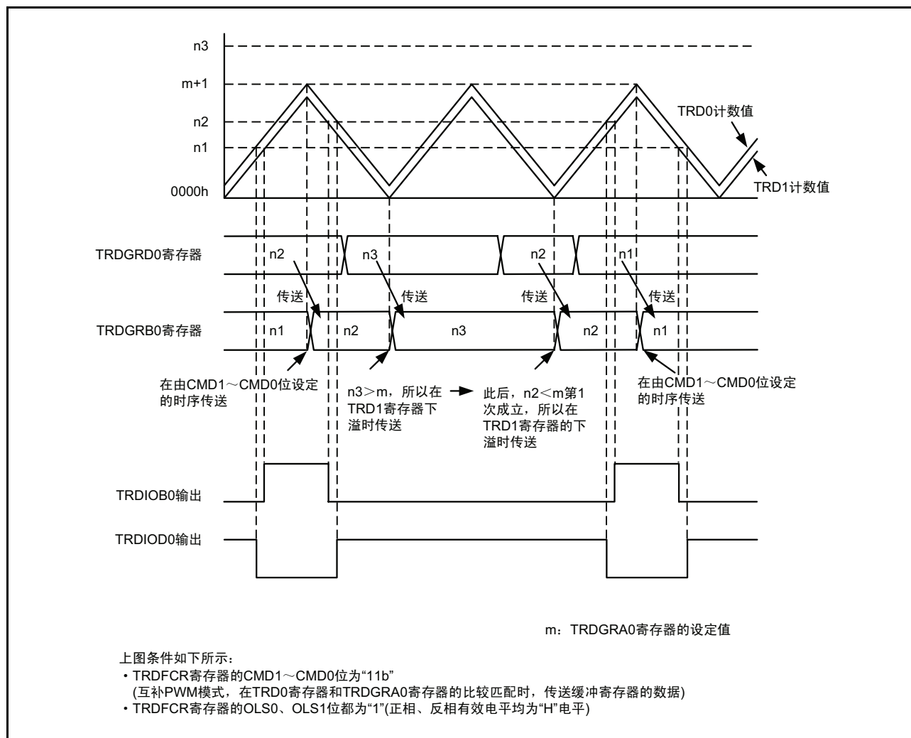
图 2.6 互补 PWM 模式时的缓冲寄存器的值 \geq TRDGRA0 寄存器的值时的运行例
