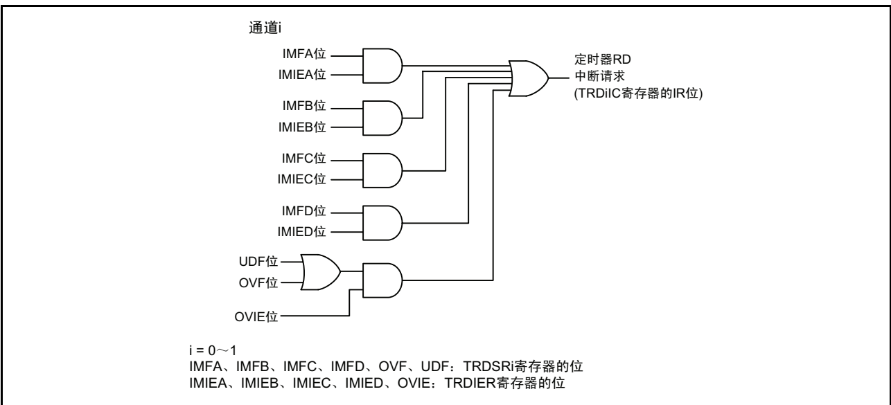
图 15.147 定时器 RD 中断的框图
