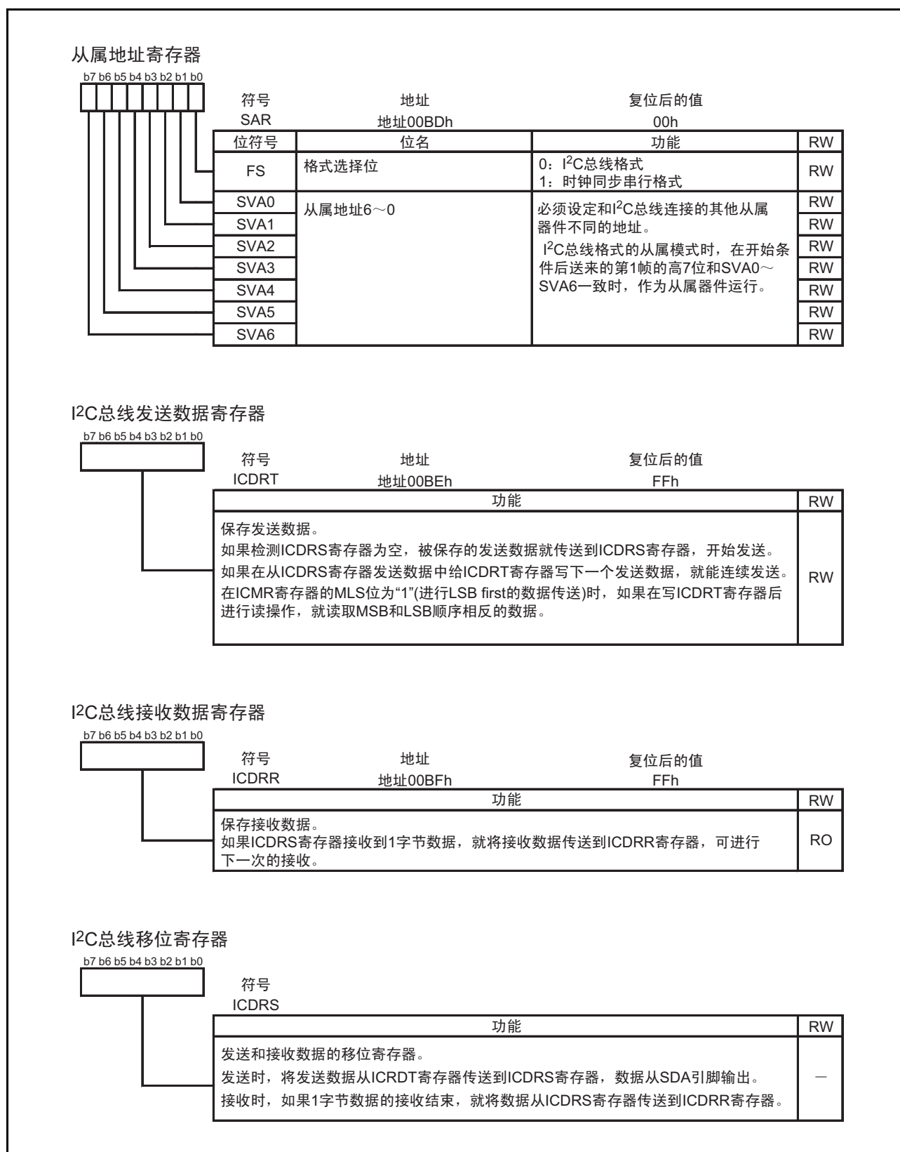
图 17.31 SAR、ICDRT、ICDRR、ICDRS 寄存器
