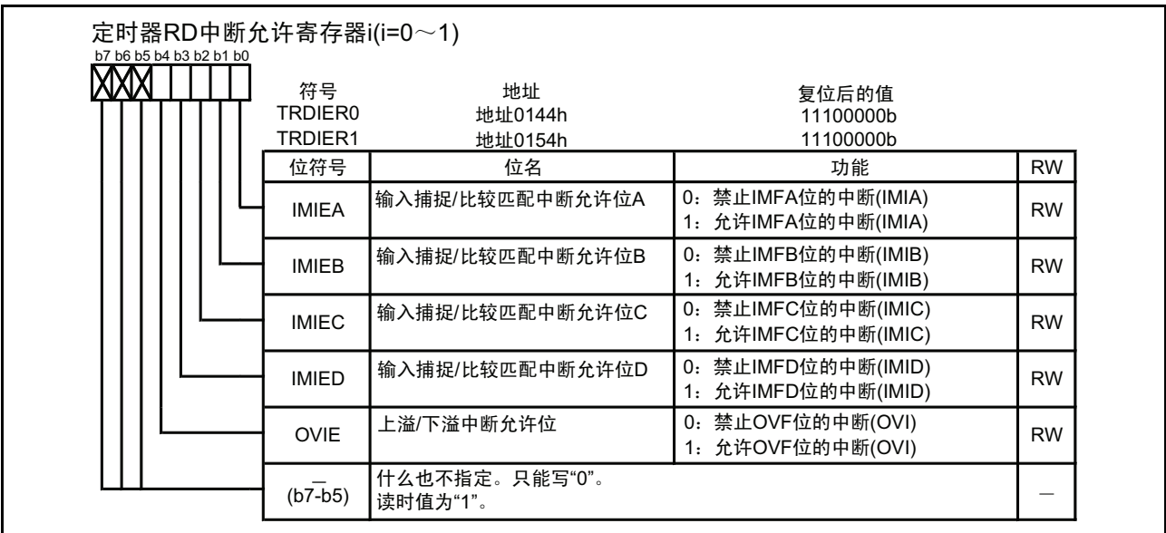
图 15.78 输入捕捉功能时的 TRDIER0 ~ TRDIER1 寄存器
