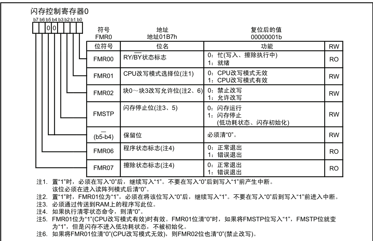
图 21.5 FMR0 寄存器
