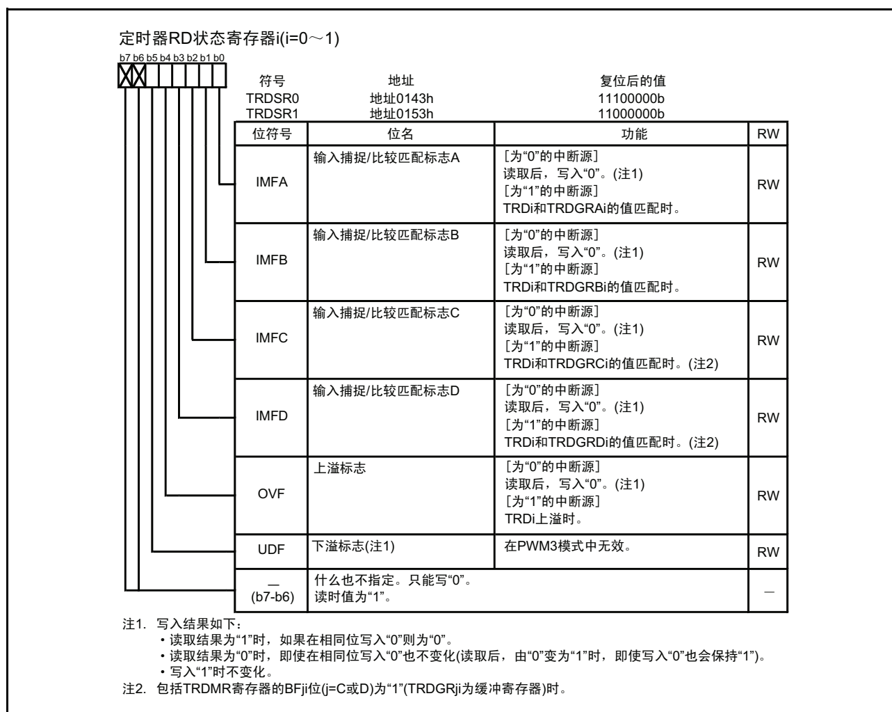
图 15.142 PWM3 模式时的 TRDSR0 ~ TRDSR1 寄存器
