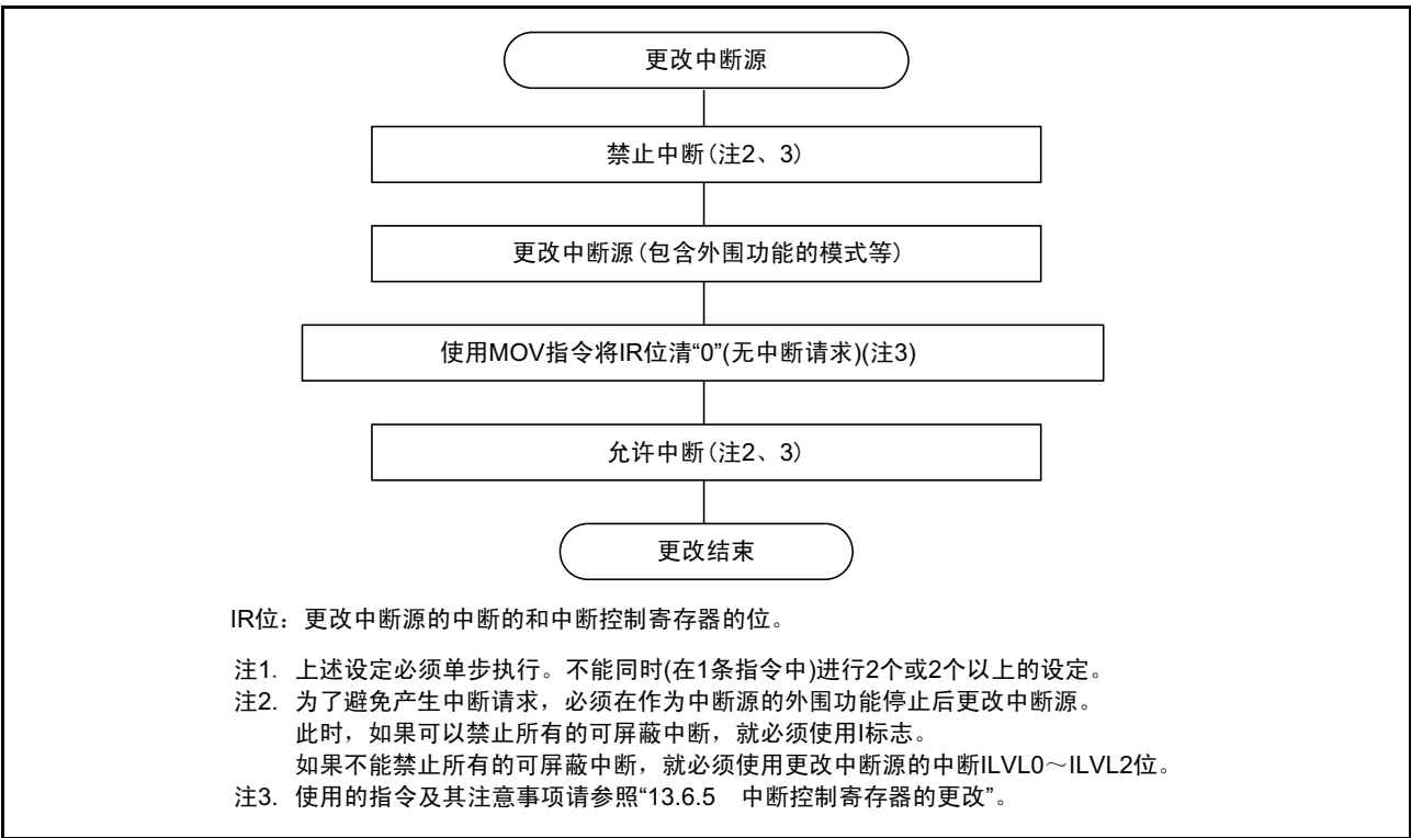
图 13.22 中断源更改步骤的例
