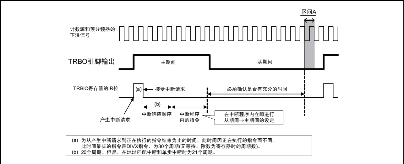
图 15.24 使用对策（a）的定时器 RB 中断的例
