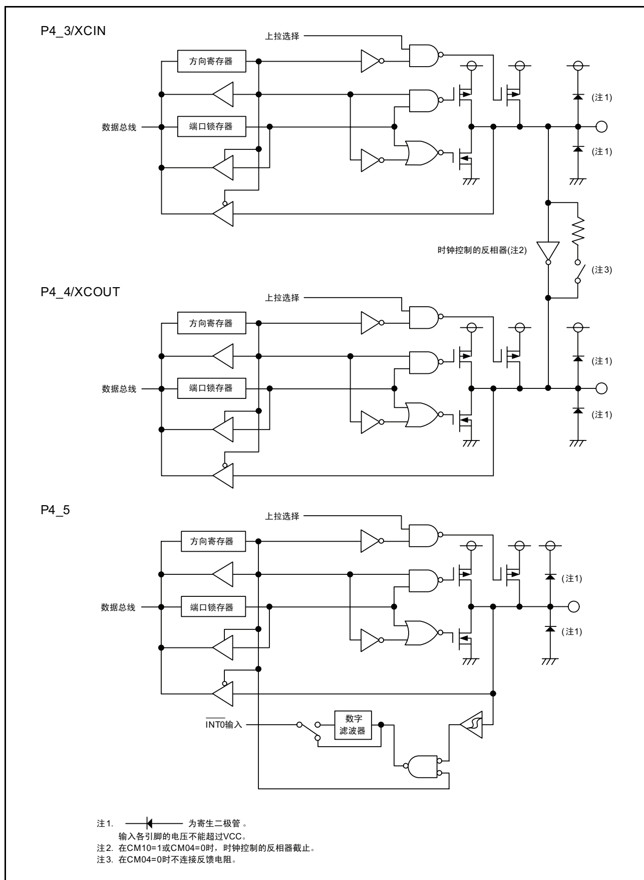
图 8.5 可编程输入 / 输出端口的结构 (5)
