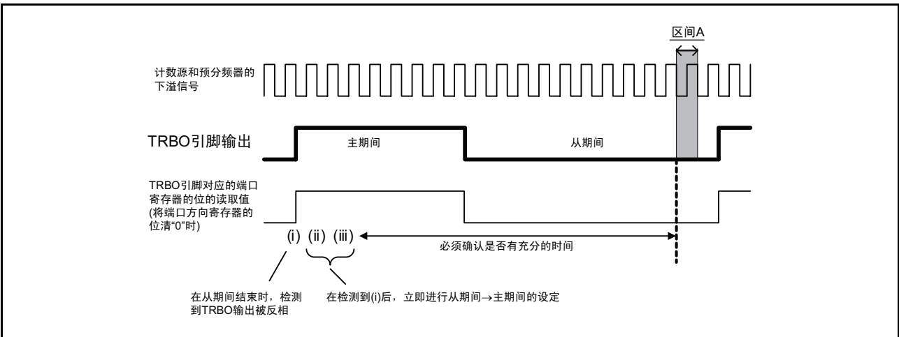
图 15.25 读对策（b）的 TRBO 引脚输出值的例
