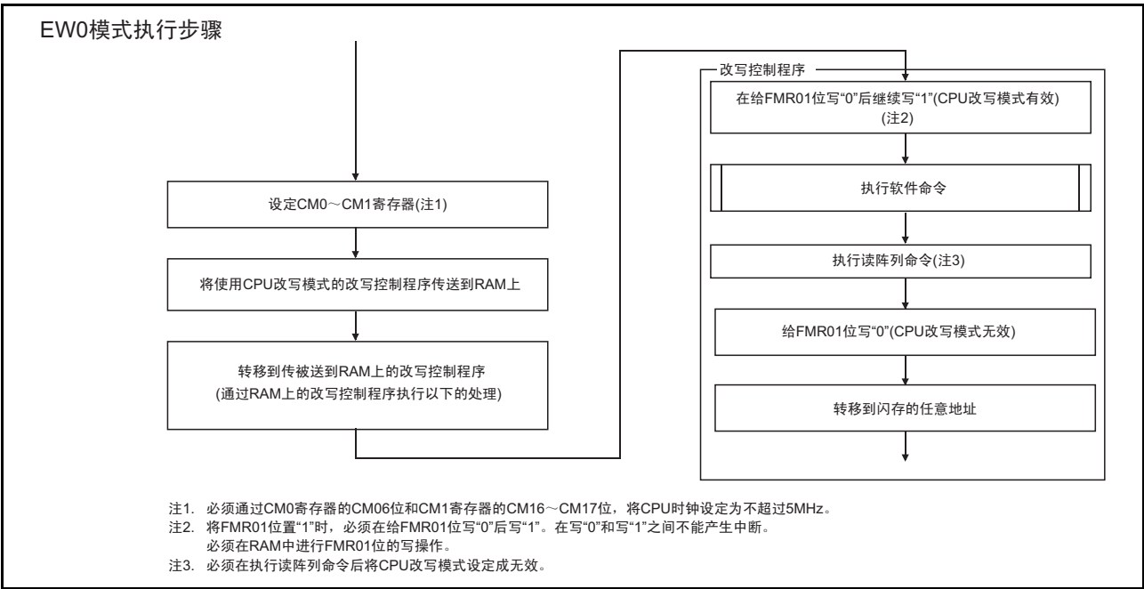
图 21.9 EW0 模式的设定和解除方法
