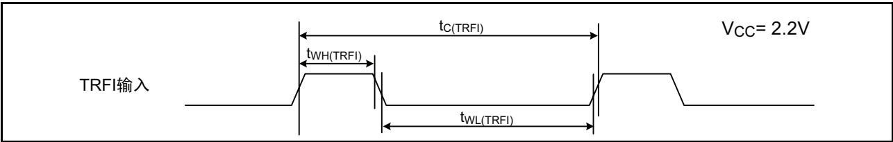
图 22.20 V_{CC}=2.2V 时的 TRFI 输入时序
