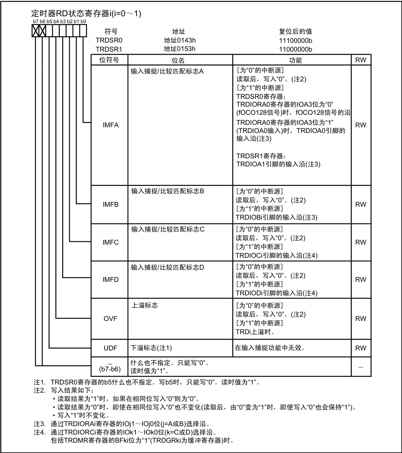
图 15.77 输入捕捉功能时的 TRDSR0 ~ TRDSR1 寄存器
