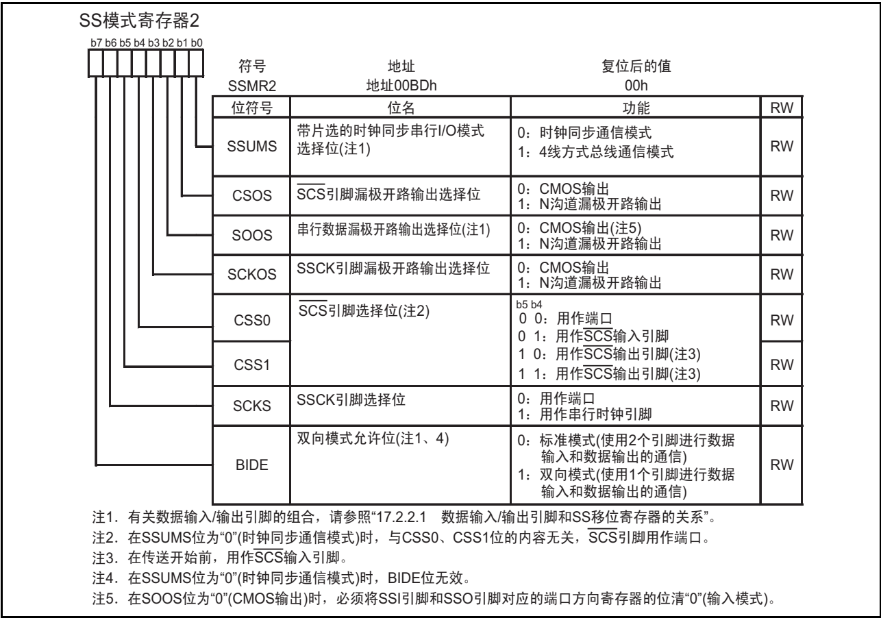
图 17.8 SSMR2 寄存器
