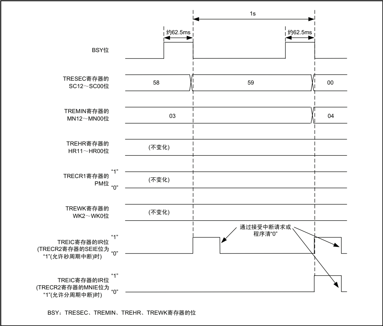
图 15.161 实时时钟模式的运行例
