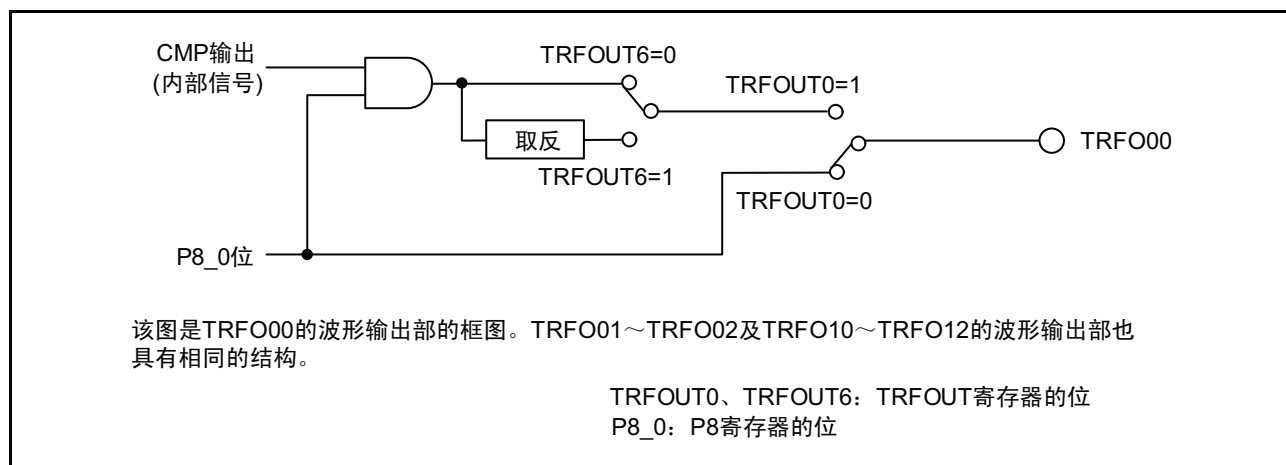
图 15.172 CMP 波形输出部框图
