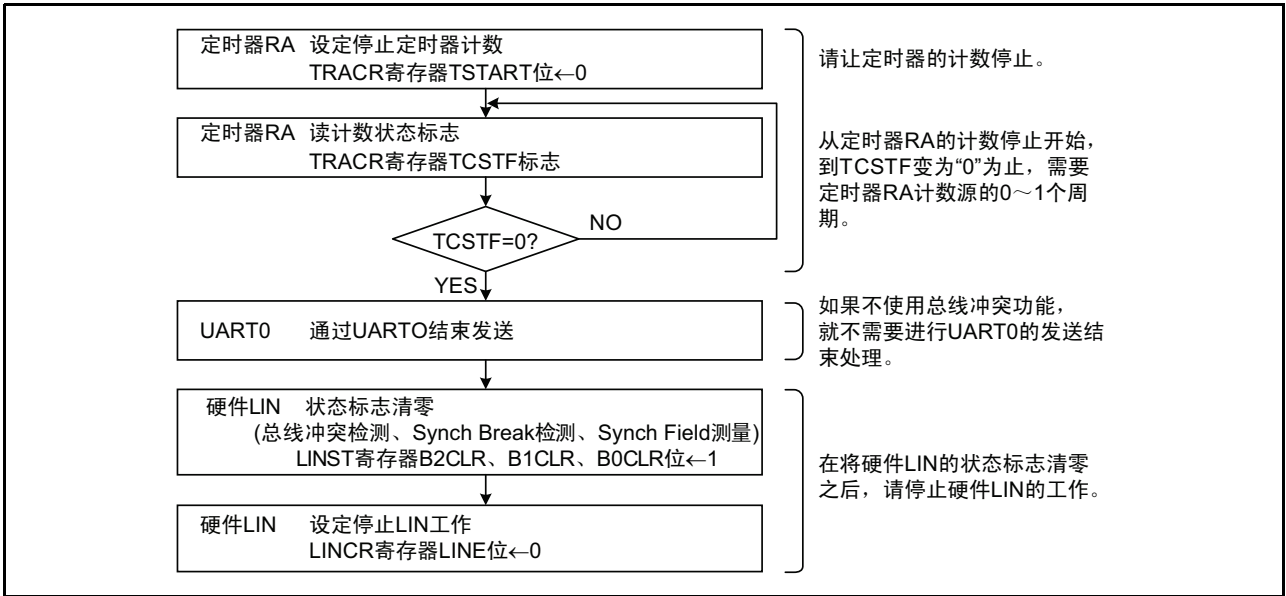
图 18.12 结束 LIN 的流程图的例子
