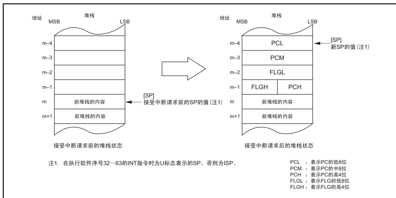
图 13.8 接受中断请求前后的堆栈状态
