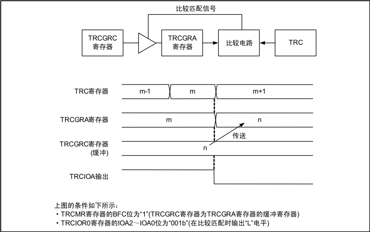
图 15.40 输出比较功能的缓冲器运行
