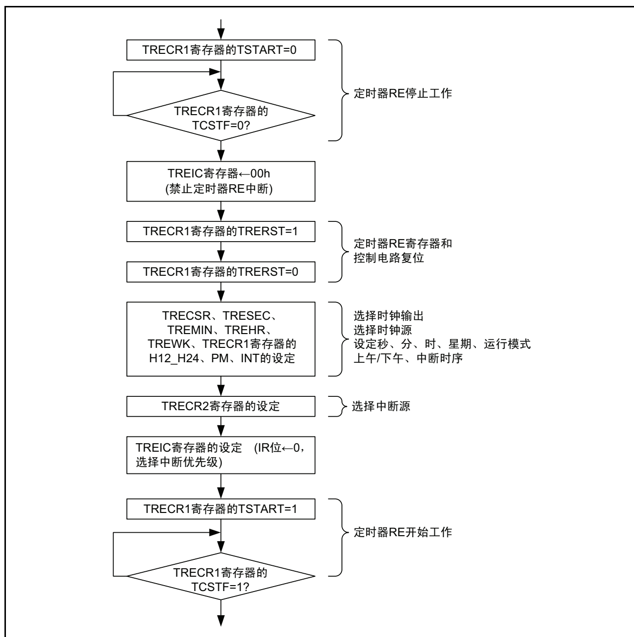
图 2.8 实时时钟模式时的设定例
