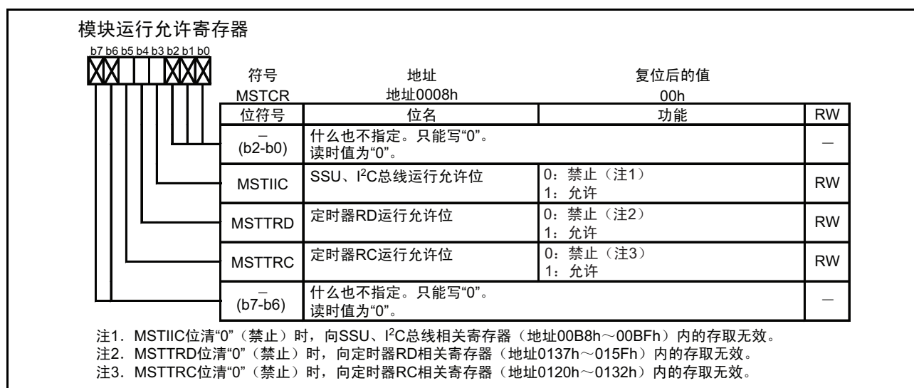
图 15.69 MSTCR 寄存器
