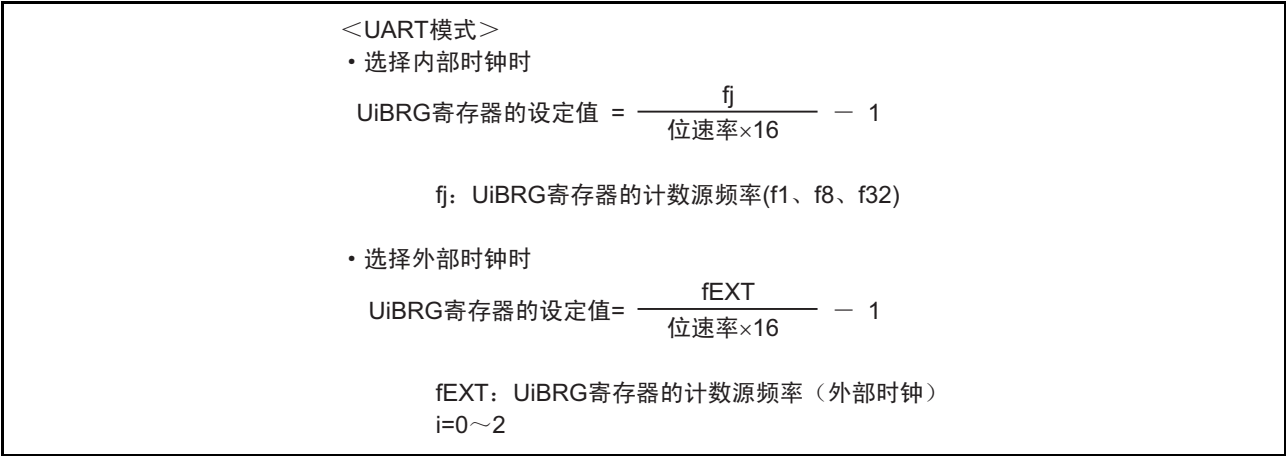
图 16.14 UiBRG 寄存器 (i=0 ~ 2) 的设定值的计算式
