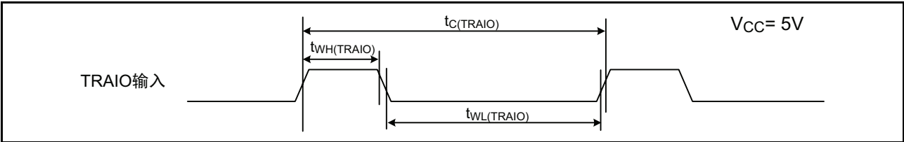
图 22.9 V_{CC}=5V 时的 TRAIO 输入、 \overline{INT1} 输入时序
