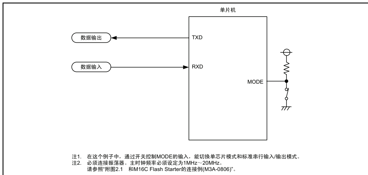
图 21.18 使用标准串行输入 / 输出模式 2 时的引脚处理例
