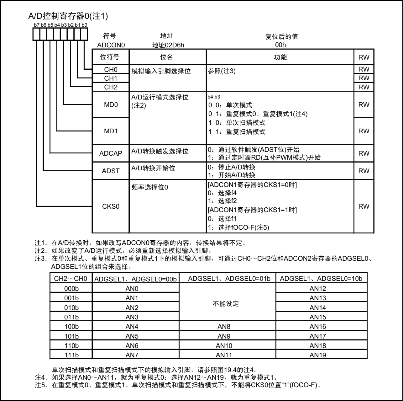
图 19.3 ADCON0 寄存器
