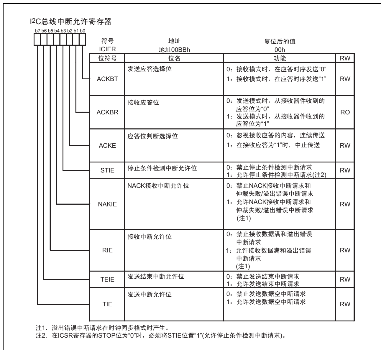
图 17.29 ICIER 寄存器
