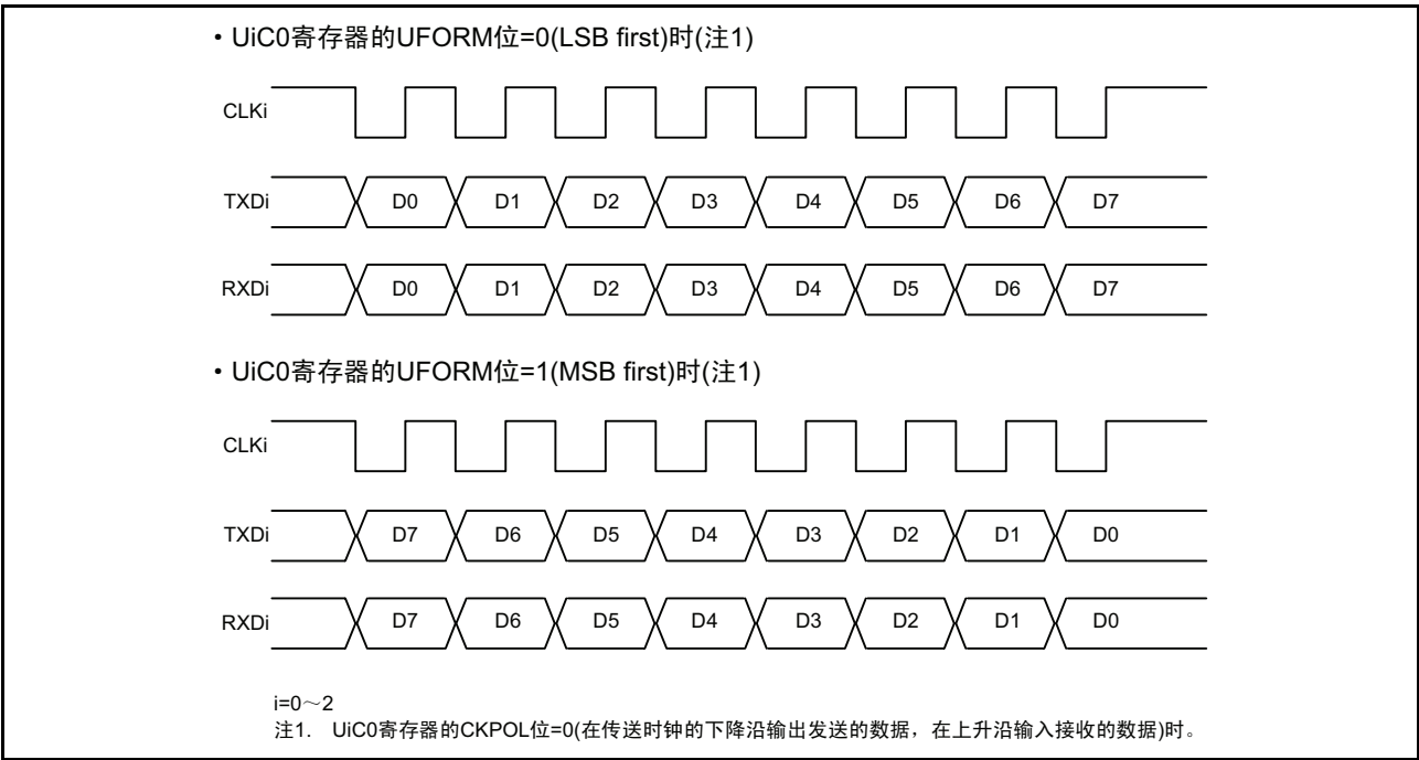
图 16.11 传送格式
