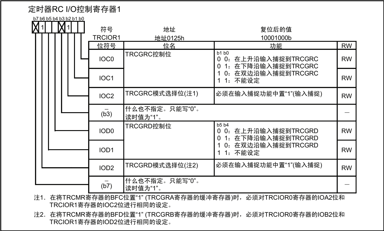
图 15.45 输入捕捉功能时的 TRCIOR1 寄存器
