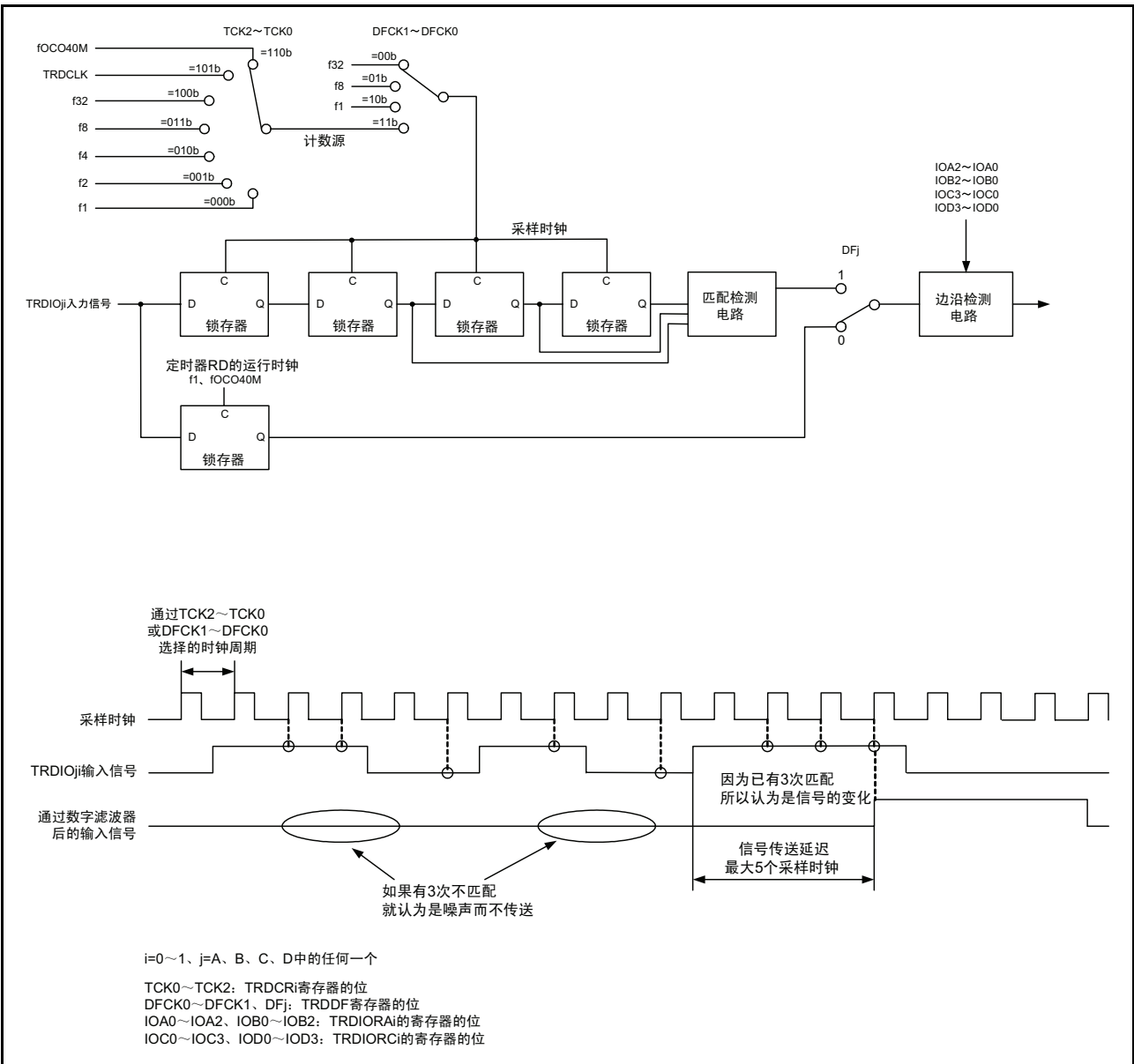
图 15.82 数字滤波器的框图
