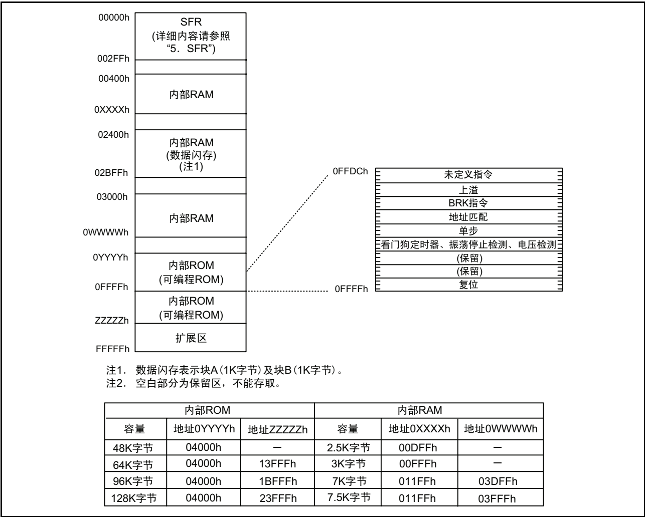
图 4.2 R8C/2D 群的存储器分配图
