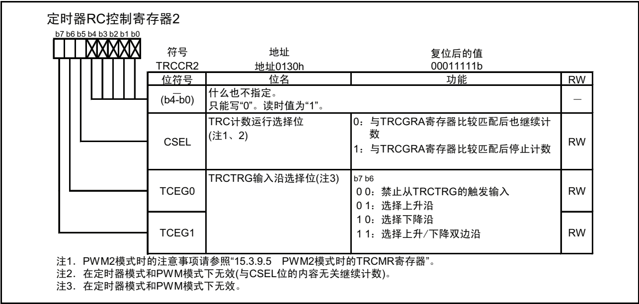
图 15.34 TRCCR2 寄存器
