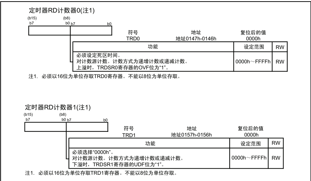
图 15.132 互补 PWM 模式时的 TRD0 ~ TRD1 寄存器
