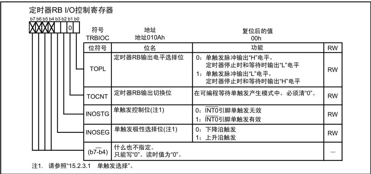
图 15.22 可编程等待单触发生模式时的 TRBIOC 寄存器
