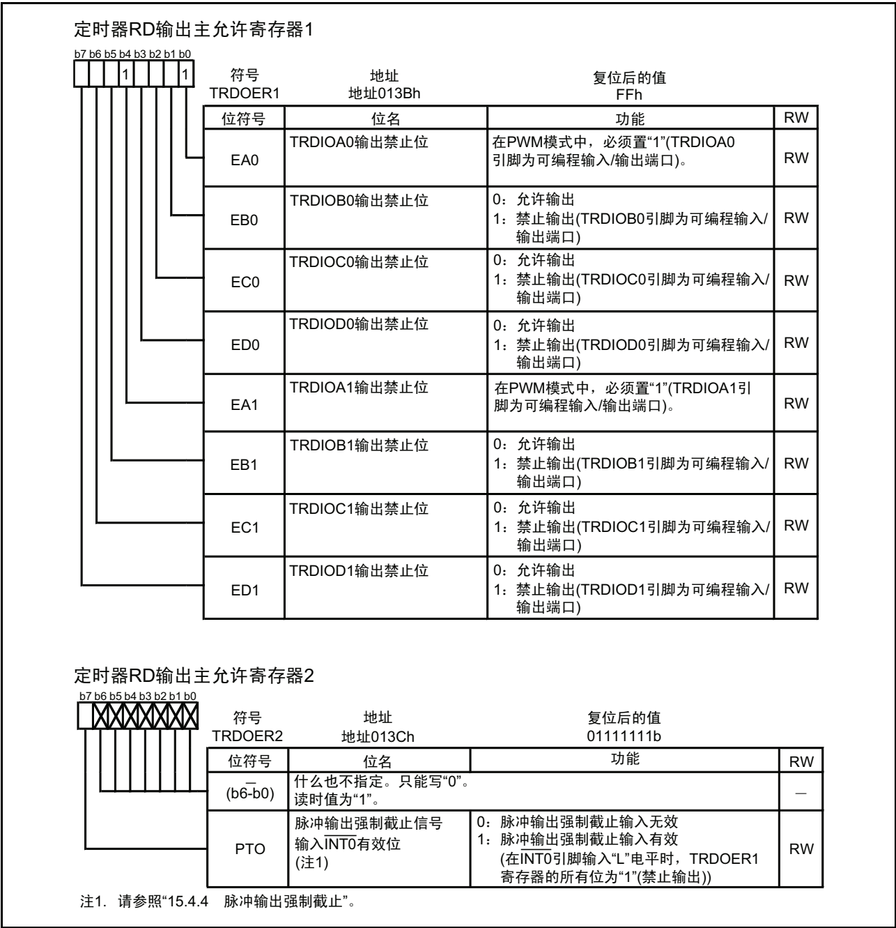
图 15.104 PWM 模式时的 TRDOER1 ~ TRDOER2 寄存器
