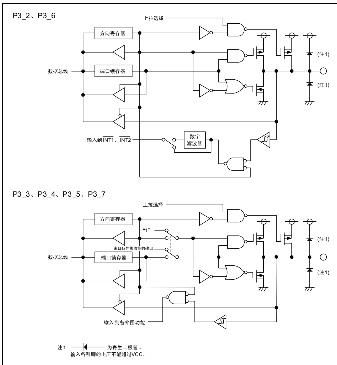
图 8.4 可编程输入 / 输出端口的结构 (4)
