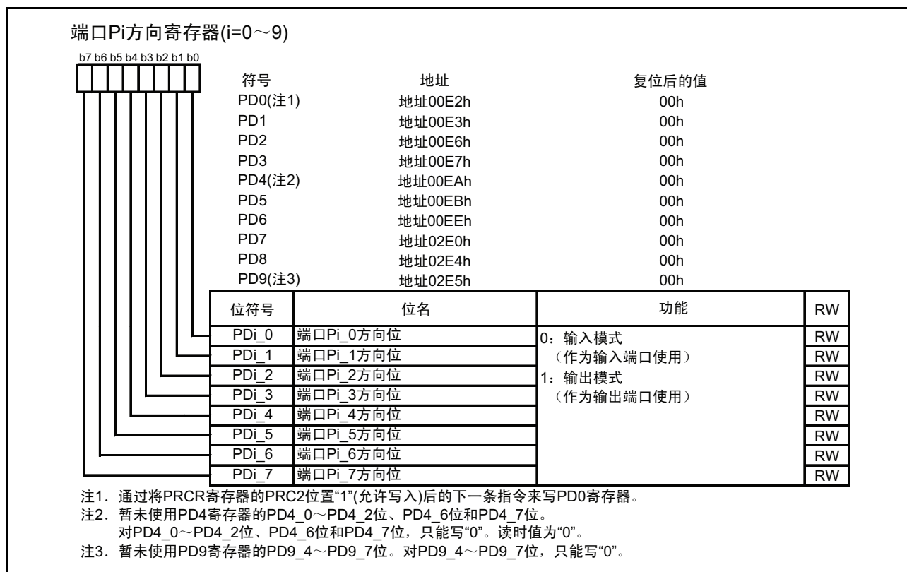
图 8.13 PDi 寄存器
