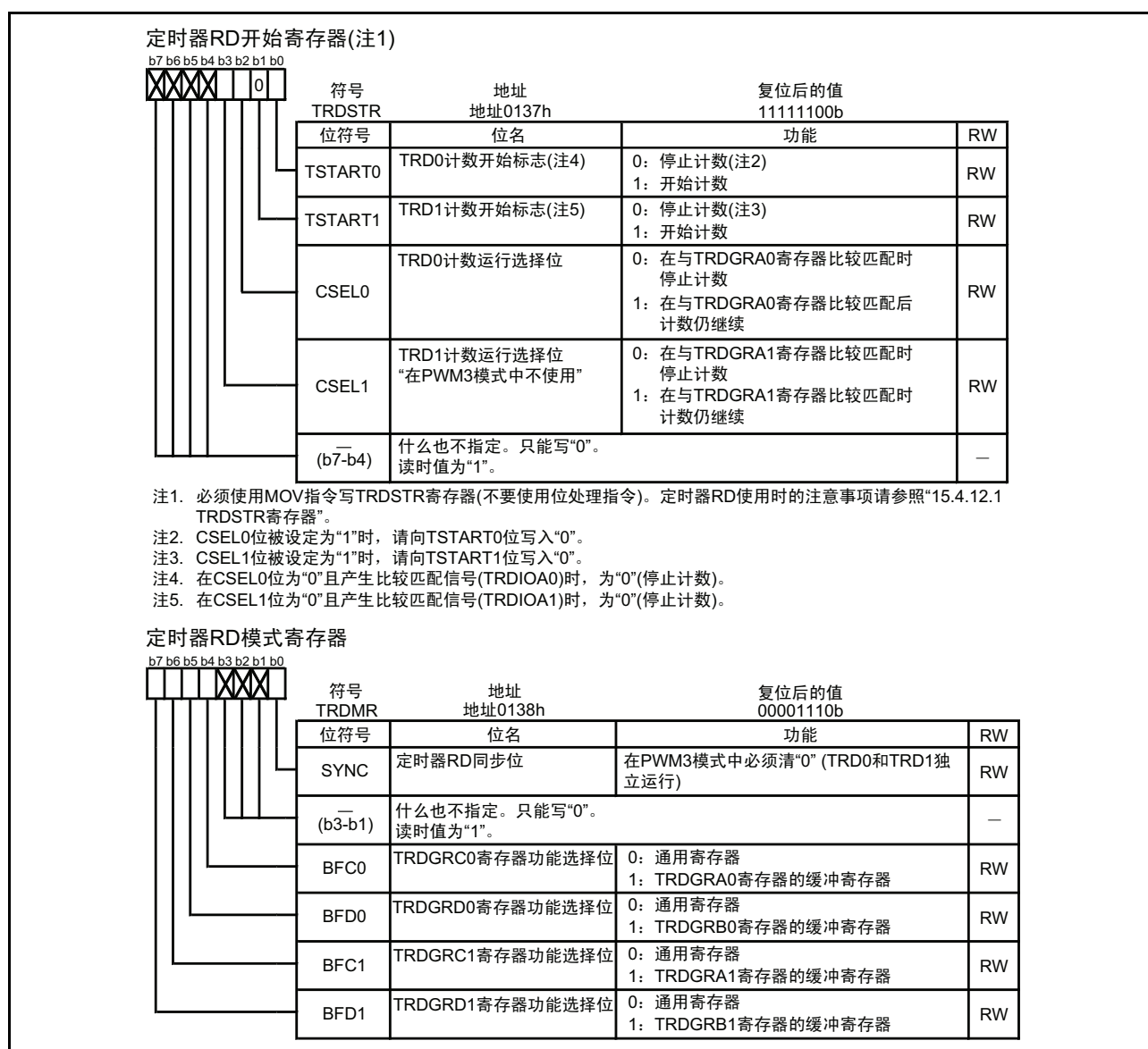
图 15.138 PWM3 模式时的 TRDSTR、TRDMR 寄存器
