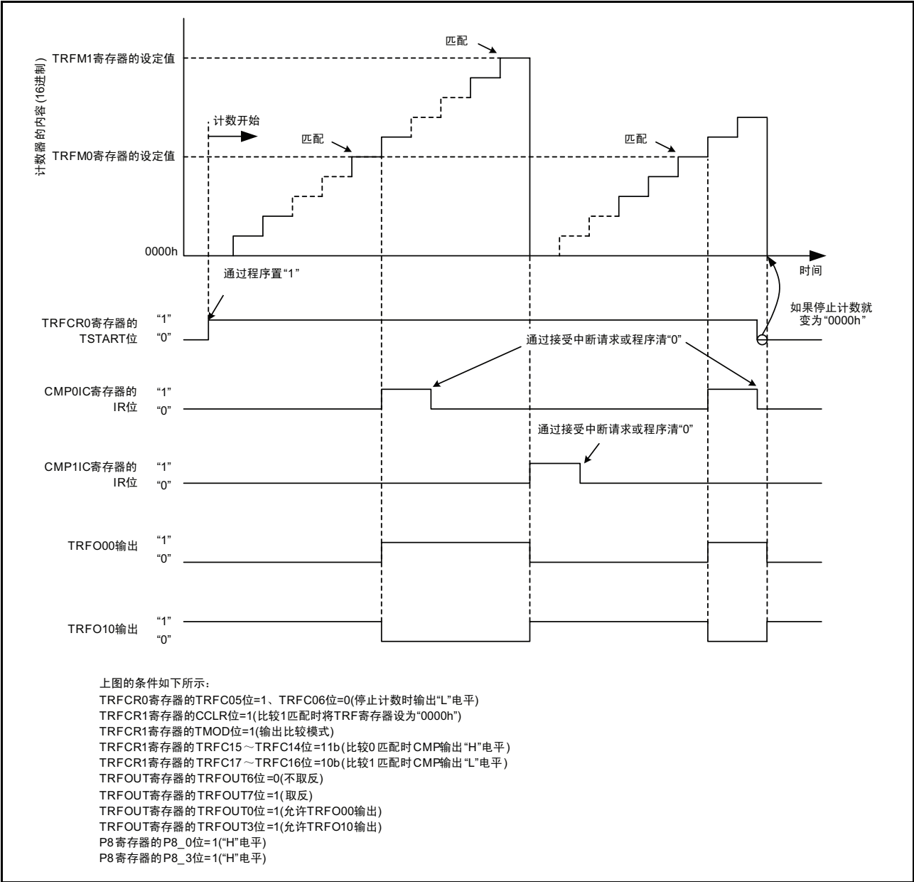
图 15.179 输出比较模式的运行例
