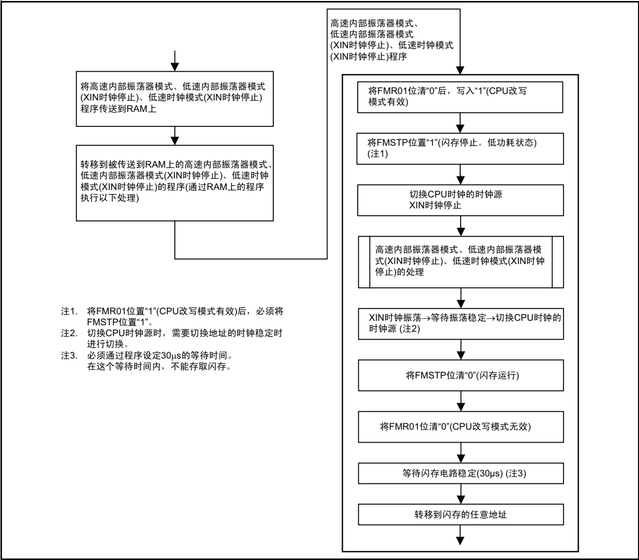
图 21.11 在高速内部振荡器模式、低速内部振荡器模式（XIN 时钟停止）、低速时钟模式（XIN 时钟停止）设定为低功耗的处理
