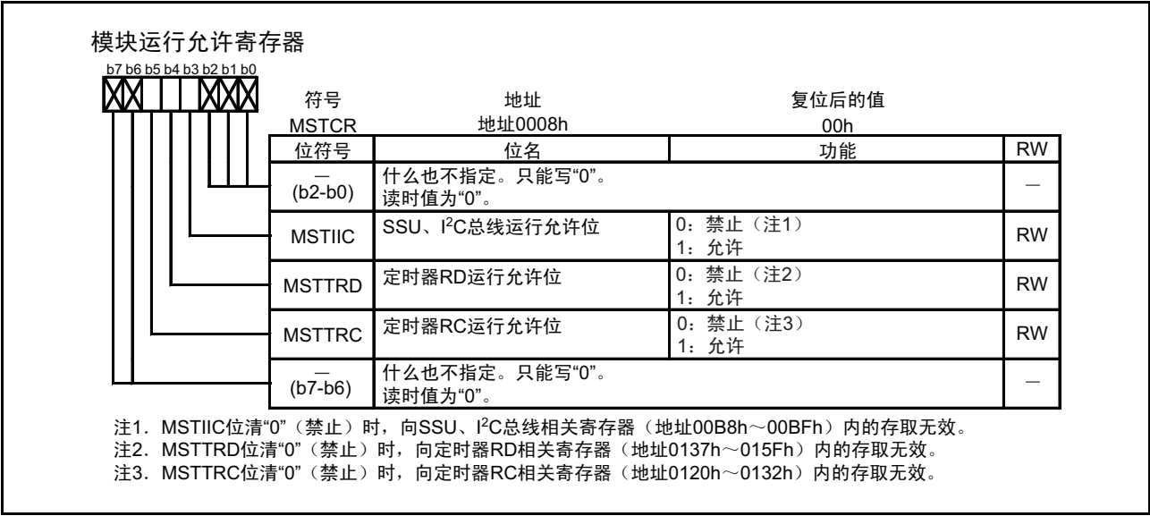
图 15.84 MSTCR 寄存器
