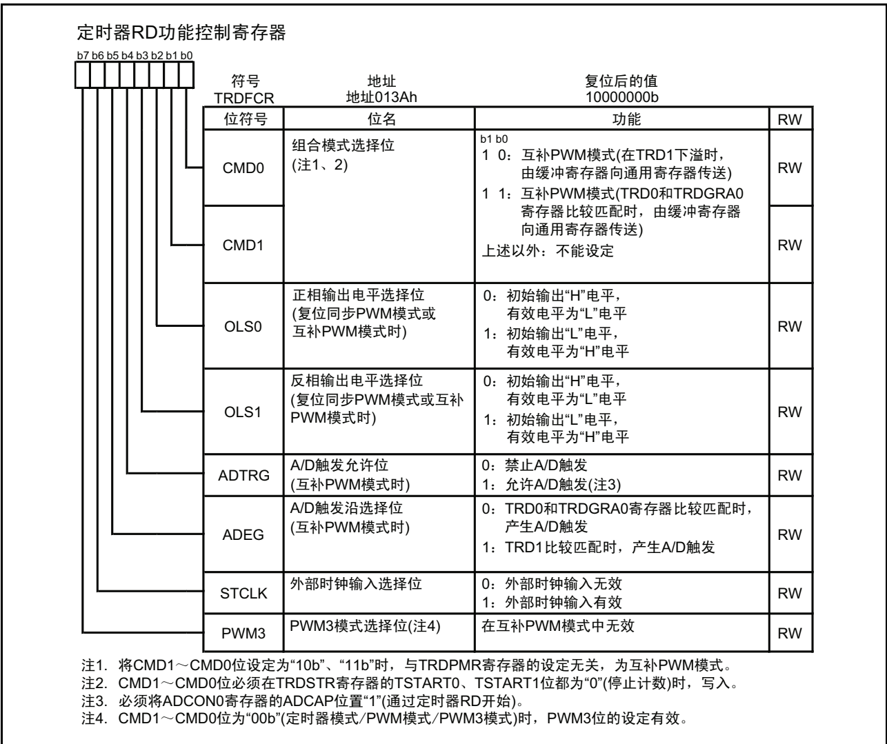
图 15.127 互补 PWM 模式时的 TRDFCR 寄存器
