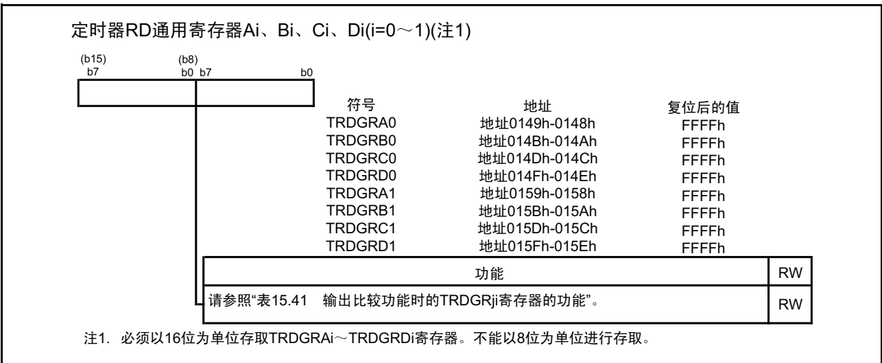
图 15.96 输出比较功能时的 TRDGRAi、TRDGRBi、TRDGRCi、TRDGRDi 寄存器
