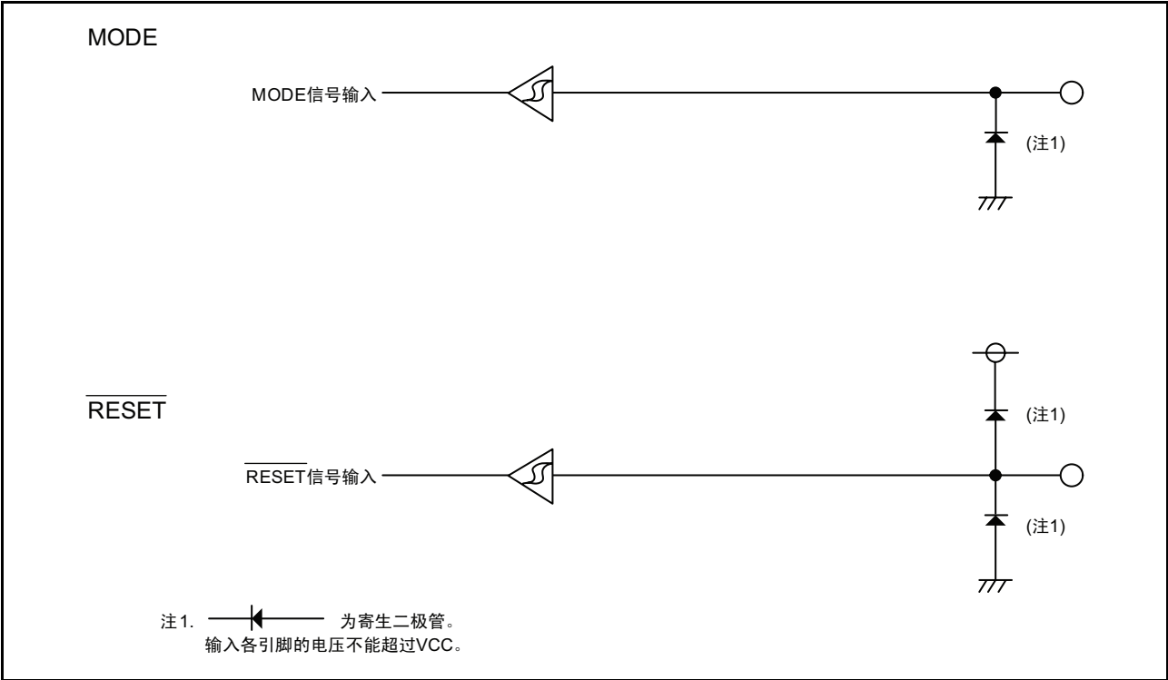
图 8.12 引脚的结构
