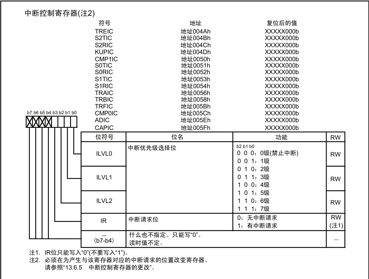
图 13.3 中断控制寄存器
