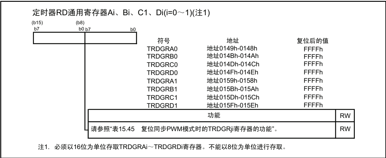
图 15.122 复位同步 PWM 模式时的 TRDGRAi、TRDGRBi、TRDGRCi、TRDGRDi 寄存器
