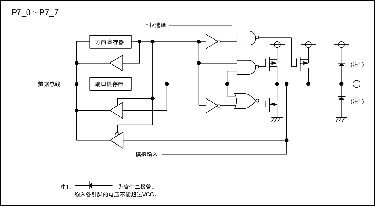
图 8.10 可编程输入 / 输出端口的结构 (10)
