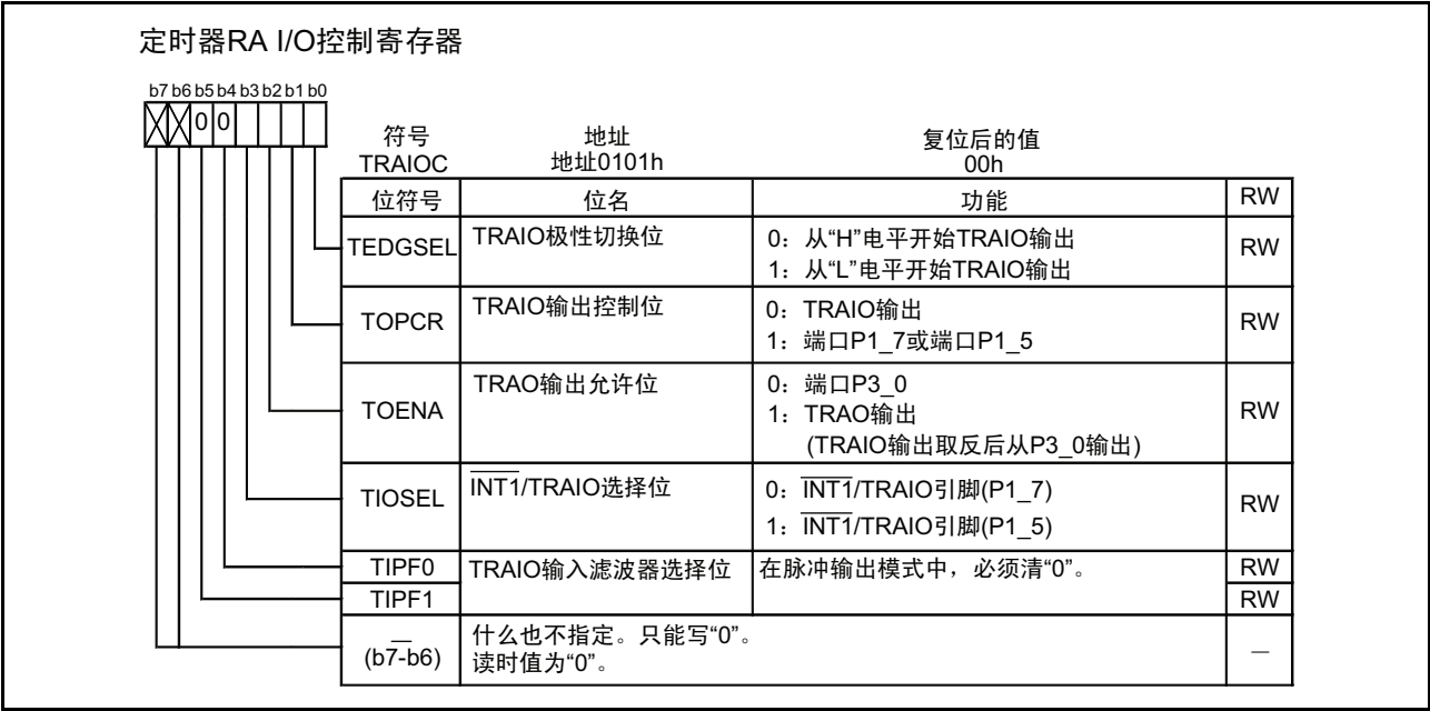
图 15.6 脉冲输出模式时的 TRAIOC 寄存器
