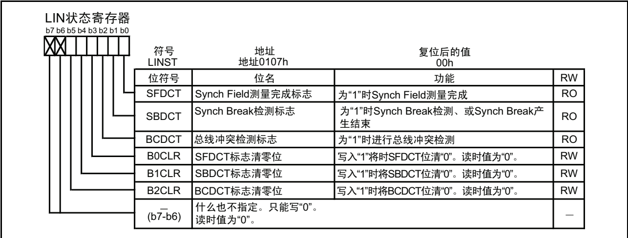
图 18.3 LINST 寄存器
