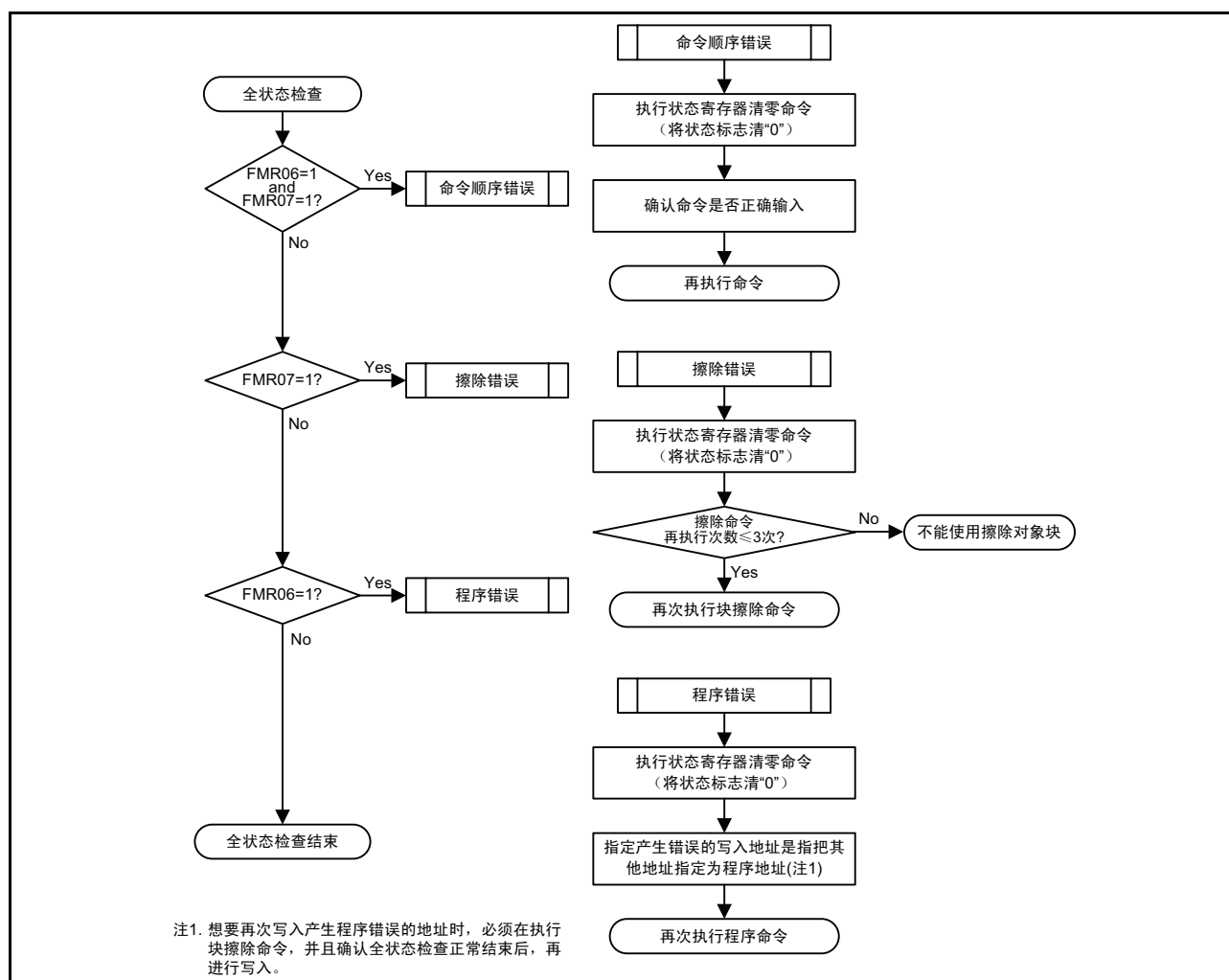
图 21.16 全状态检查流程图和产生各种错误时的处理方法
