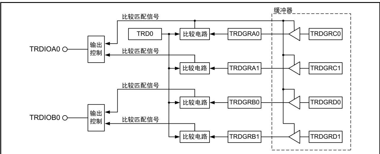
图 15.136 PWM3 模式的框图
