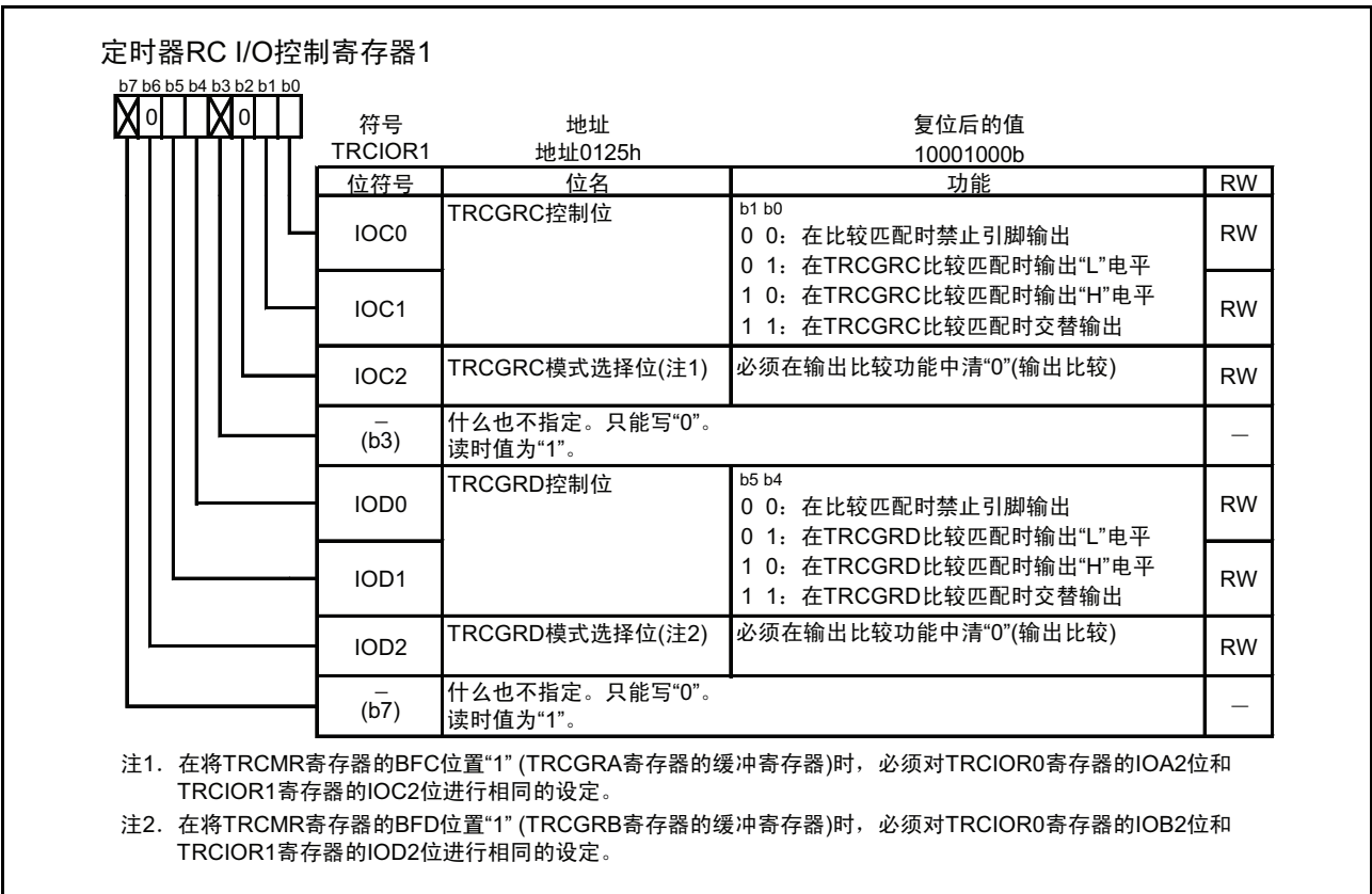
图 15.49 输出比较功能时的 TRCIOR1 寄存器
