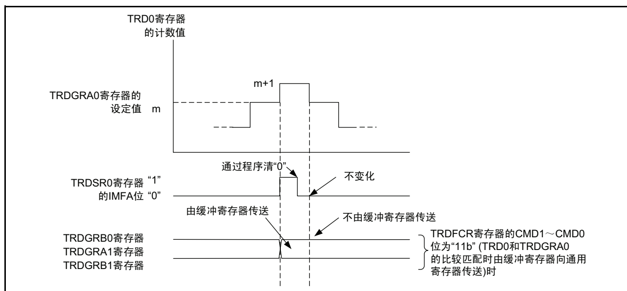
图 15.148 互补 PWM 模式时的 TRD0 和 TRDGRA0 寄存器比较匹配时的运行
