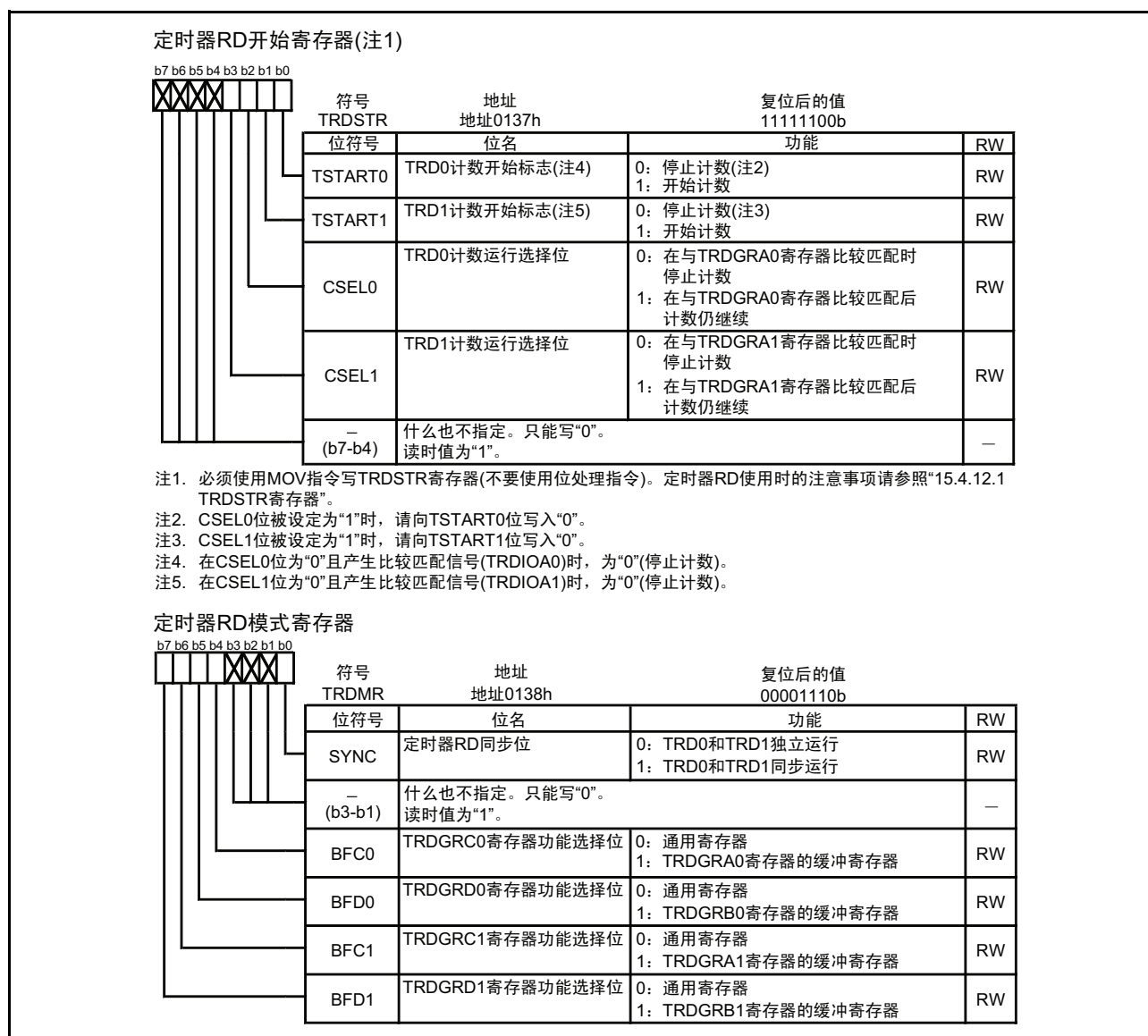
图 15.102 PWM 模式时的 TRDSTR、TRDMR 寄存器
