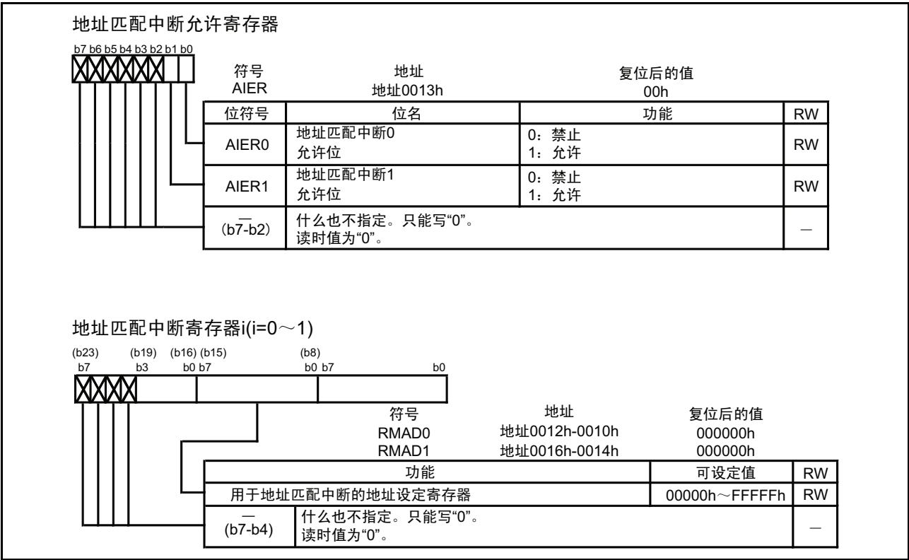
图 13.20 AIER 和 RMAD0 ~ RMAD1 寄存器
