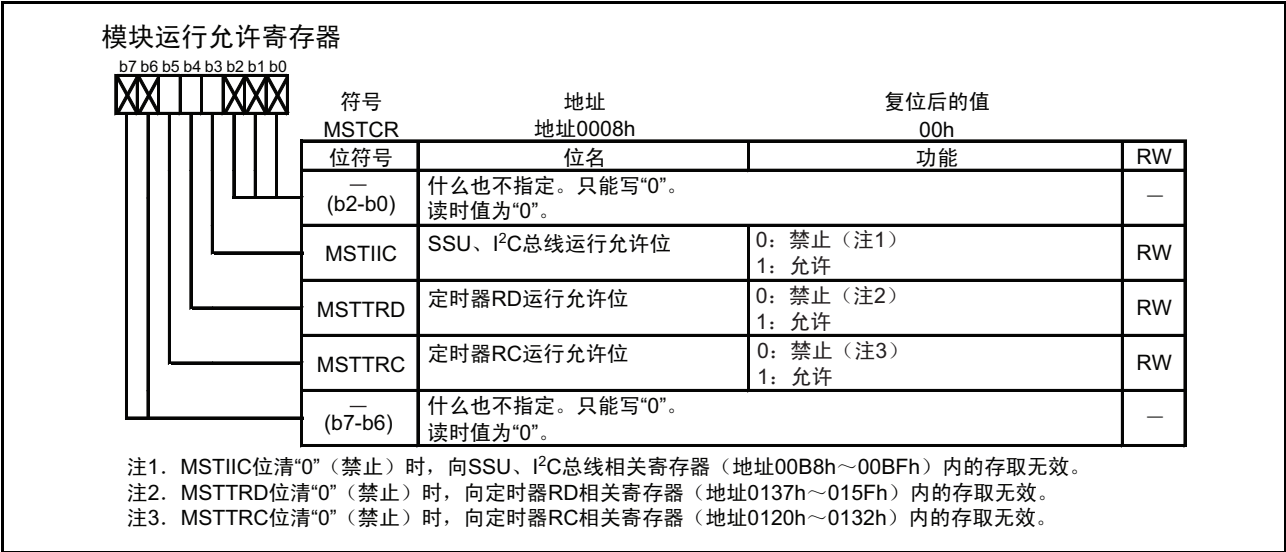
图 15.125 MSTCR 寄存器
