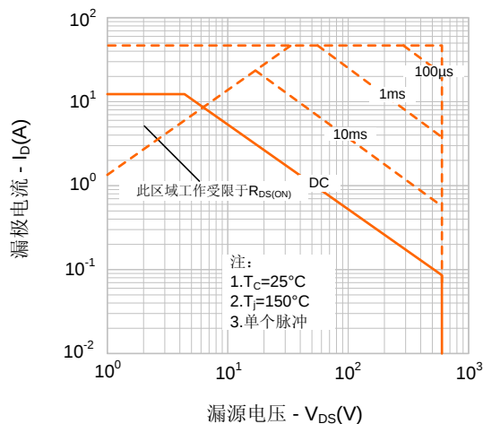
图9-2. 最大安全工作区域(SVF12N60F(G))
