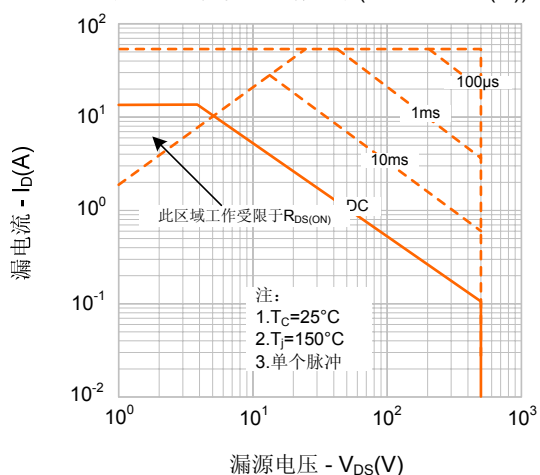
图9-2. 最大安全工作区域(SVF13N50F(G))
