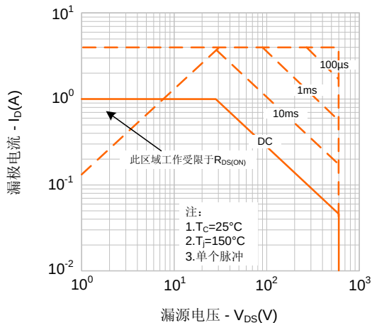
图9. 最大安全工作区域
