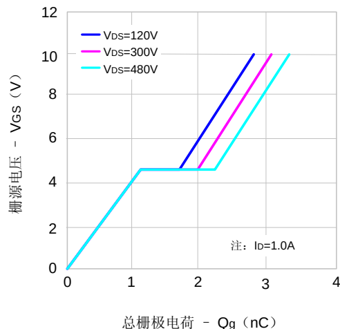
图6. 电荷量特性
