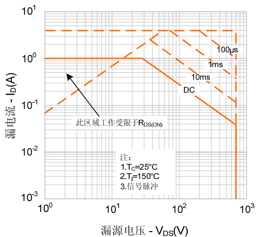
图 9-1. 最大安全工作区域 (SVF1N70M)
