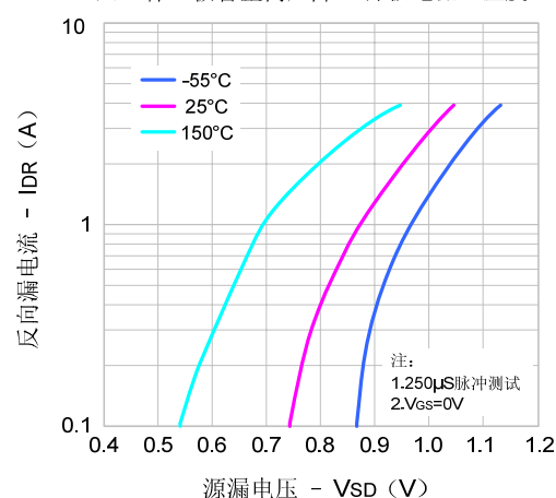
图4. 二极管正向压降vs.源极电流、温度
