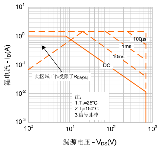
图 9-2. 最大安全工作区域 (SVF1N70B)
