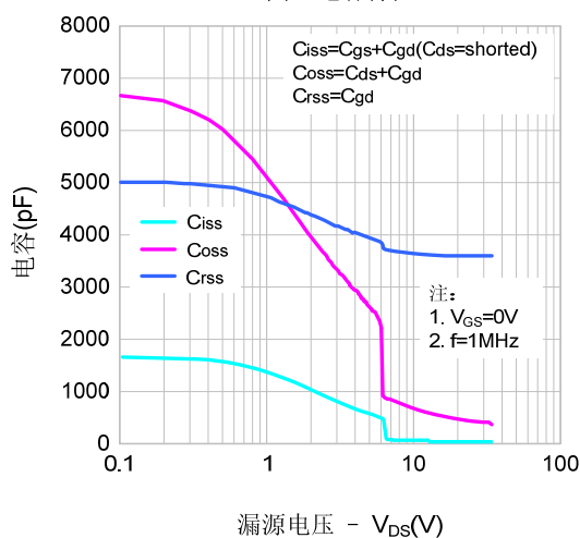
图5. 电容特性
