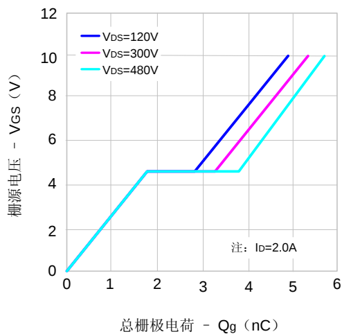
图6. 电荷量特性
