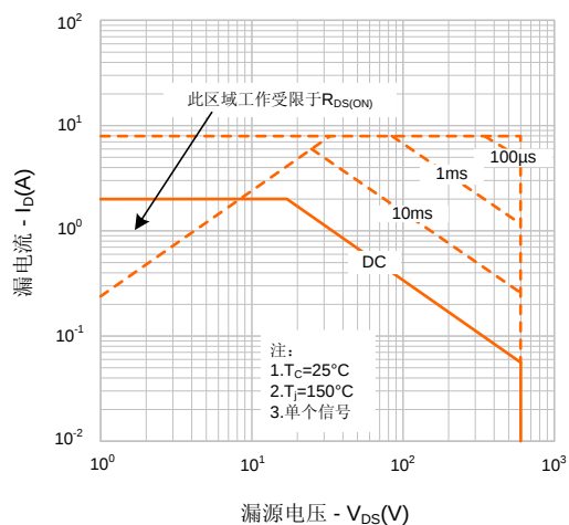
图9-1. 最大安全工作区域(SVF2N60M/D)
