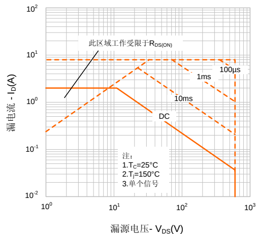
图9-4. 最大安全工作区域(SVF2N60F(G))
