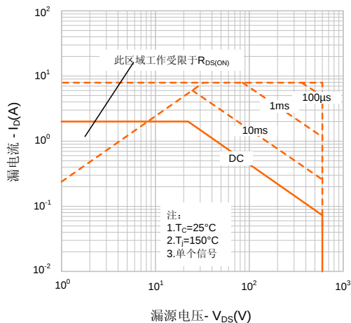
图9-3. 最大安全工作区域(SVF2N60T)
