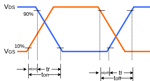
开关时间测试电路及波形图
