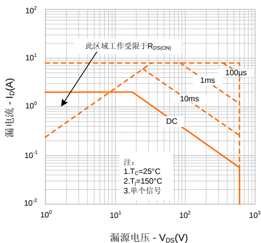
图9-2. 最大安全工作区域(SVF2N60MJ)
