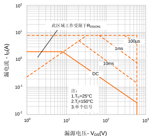
图9-6. 最大安全工作区域(SVF2N60NF)
