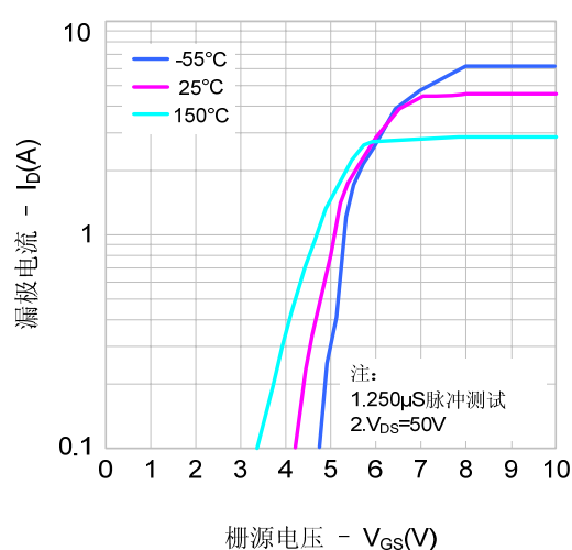
图2. 传输特性
