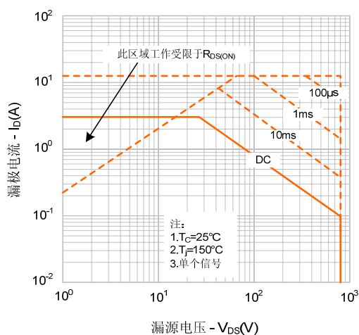
图9-1. 最大安全工作区域(SVF3N80M/D)
