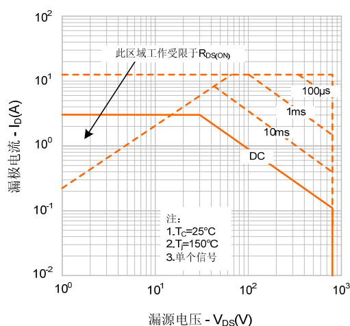
图9-2. 最大安全工作区域(SVF3N80MJ)
