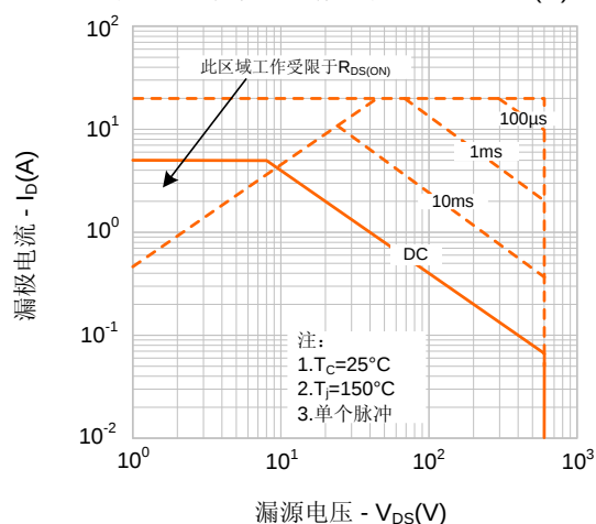
图9-2. 最大安全工作区域 (SVF5N60F(G))
