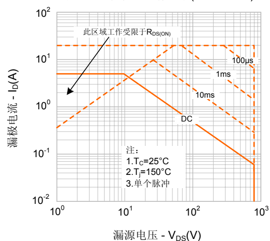
图9-1. 最大安全工作区域(SVF5N80F)
