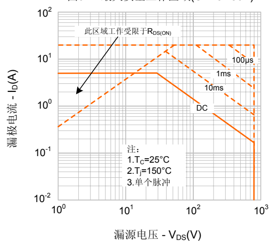
图9-2. 最大安全工作区域(SVF5N80T)
