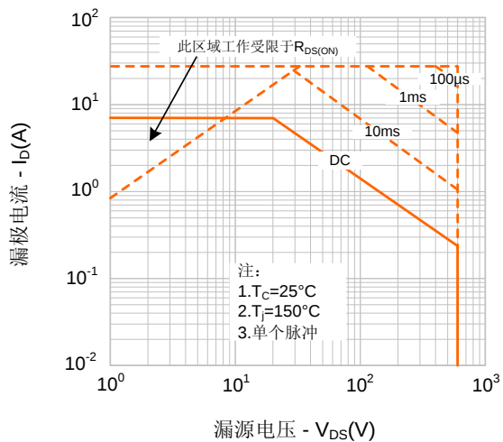
图9-3. 最大安全工作区域(SVF7N60S)
