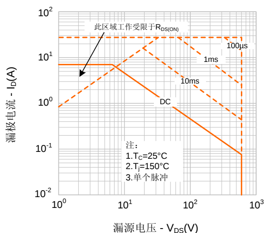
图9-2. 最大安全工作区域(SVF7N60F)
