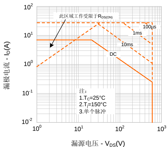
图9-1. 最大安全工作区域(SVF7N60T/MJ)
