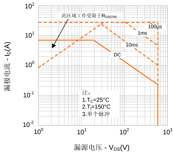
图9-4. 最大安全工作区域(SVF7N60K)
