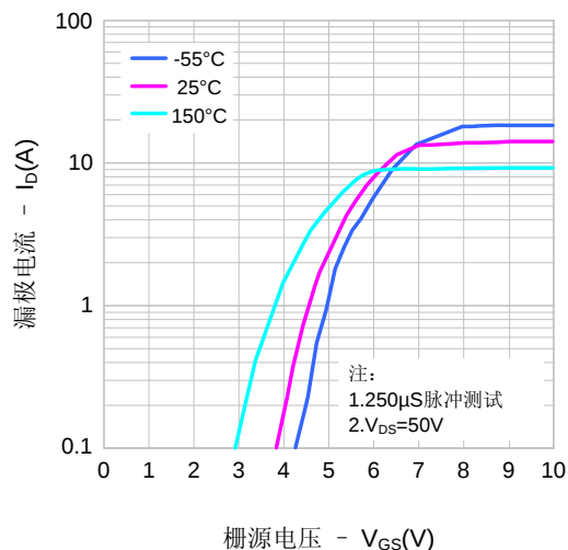
图2. 传输特性
