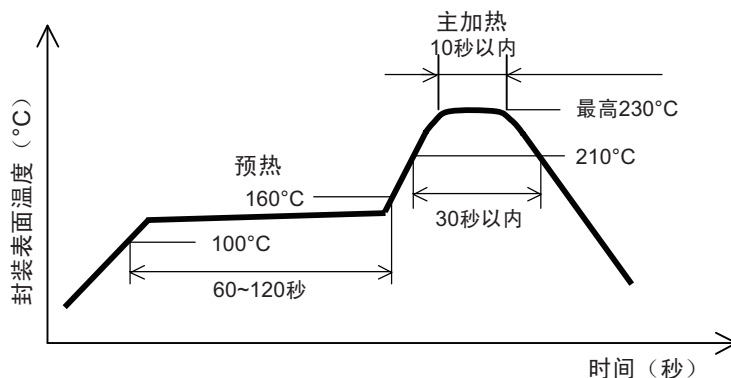
图 4-15 红外回流温度曲线 (IR30)
