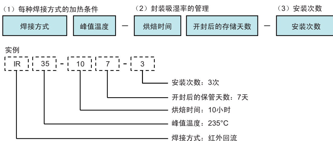
图 4-13 焊接耐热条件的表示实例
