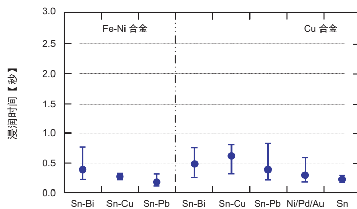
图 4-3 浸润时间测定结果（Sn-3Ag-0.5Cu 焊浴）
