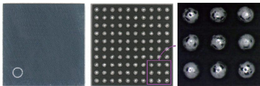
图 5-3 5.17 × 5.17 mm, 100 pin WLBGA 外观
