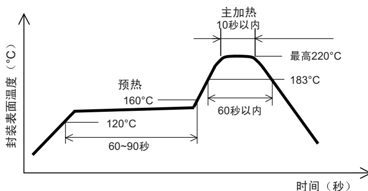
图 4-14 红外回流温度曲线 (IR20)
