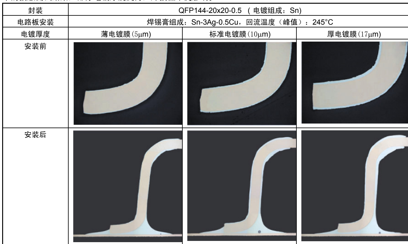
图 4-4 电镀厚度和焊接性
