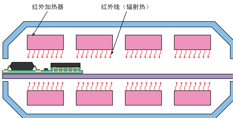
图 1-8 红外法（例）
