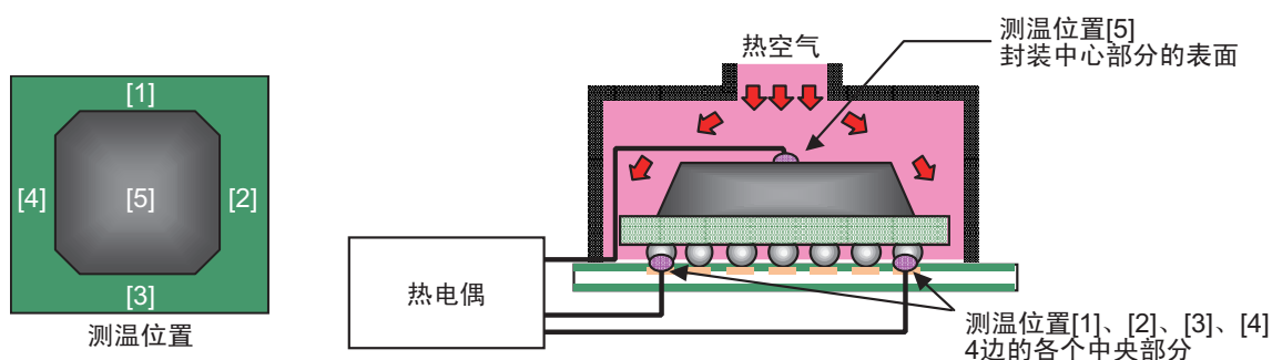
图 3-13 测温时的传感器安装实例
