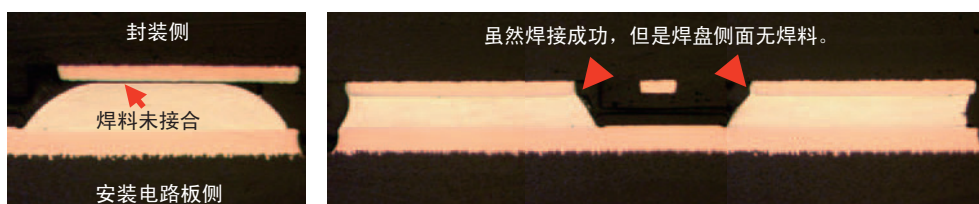
图 5-29 安装后断面（对策前）
