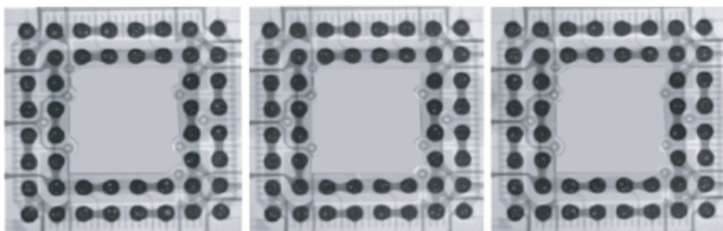
图 5-28 X 线外观（对策后 2）
