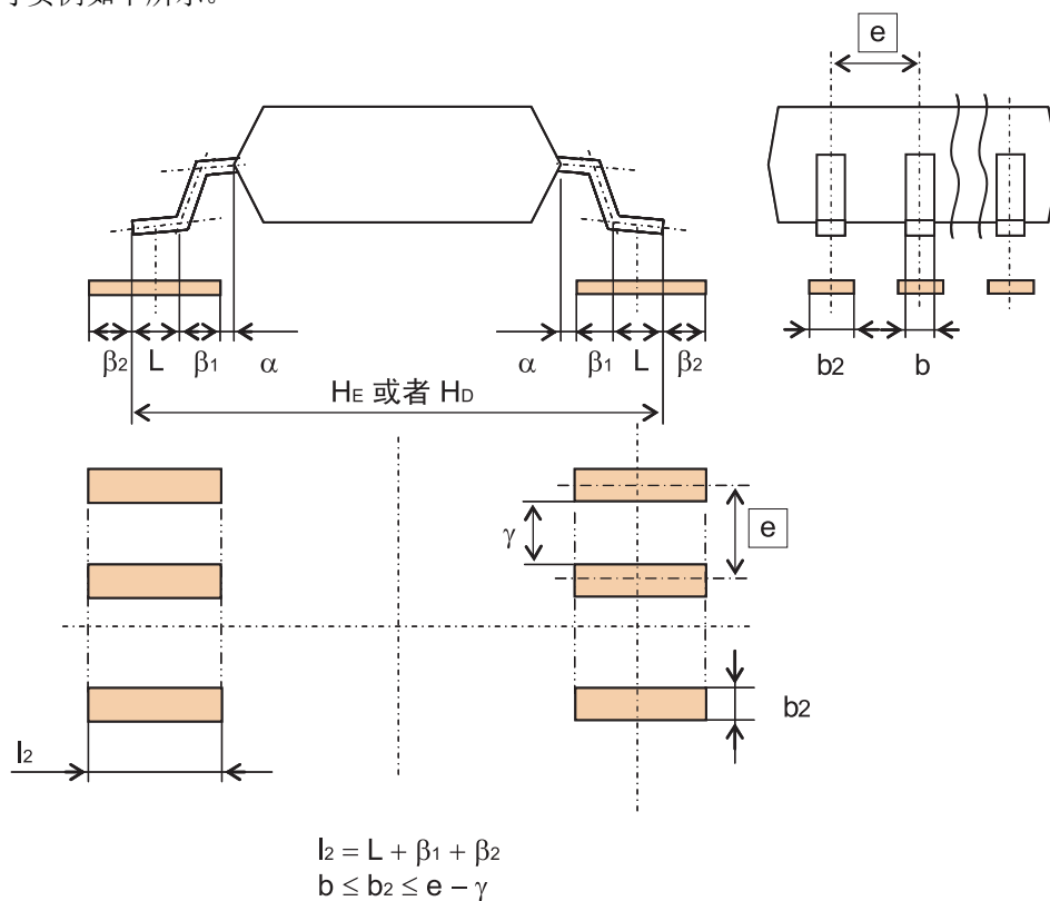
• 瑞萨封装尺寸实例： TSOP 类型 I
