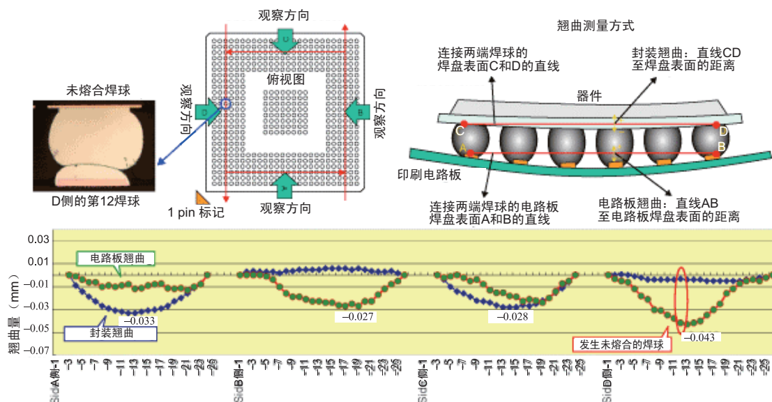
图 5-15 翘曲引起的未熔合案例
