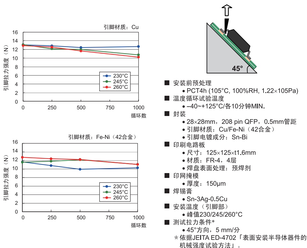
图 6-4 引脚拉力强度
