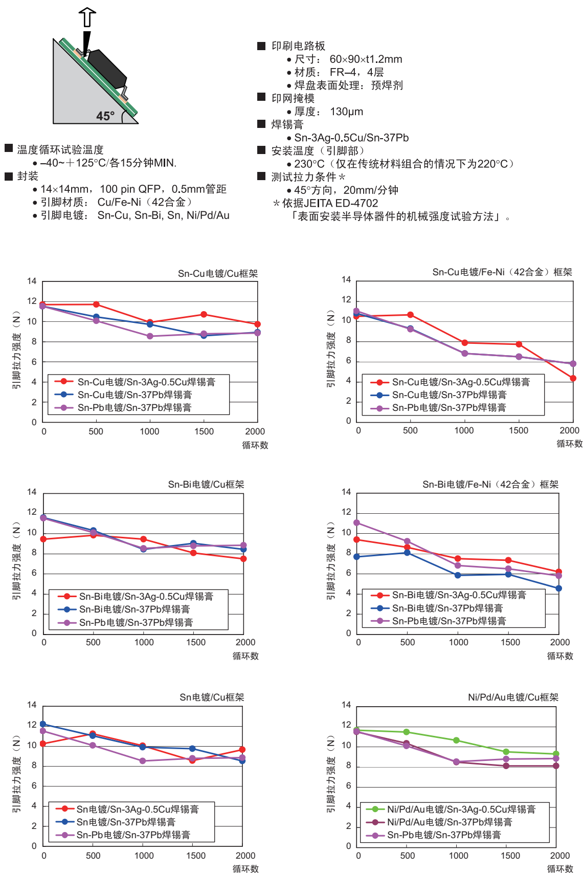
图 6-15 引脚拉力强度
