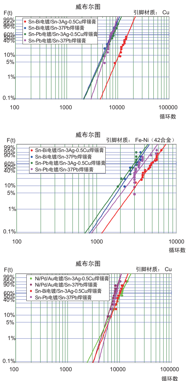
图 6-10 威布尔图 (电镀成分和焊接材料的组合)
