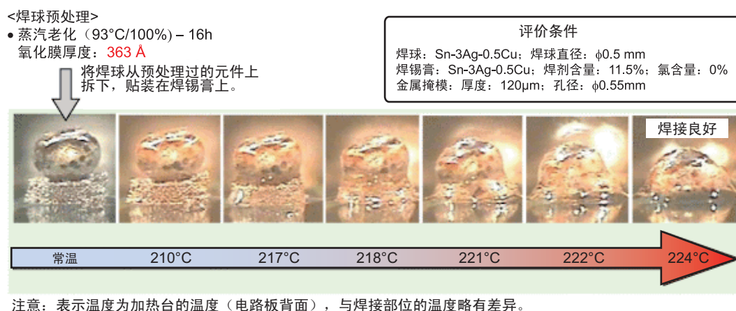
图 5-16 表面氧化膜增厚的焊球焊接性
