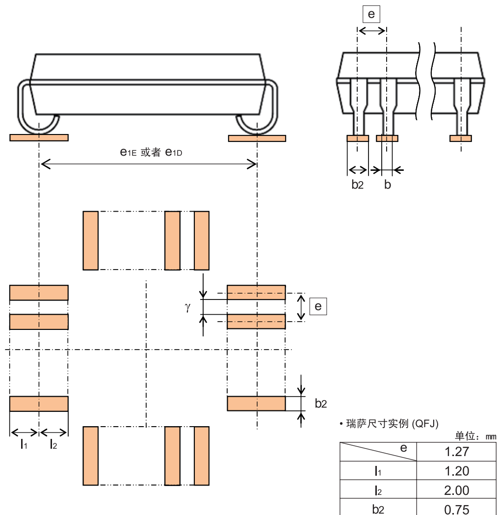
图 2-8 QFJ 实例
