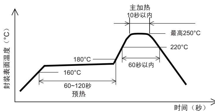
图 4-17 红外回流温度曲线 (IR50)
