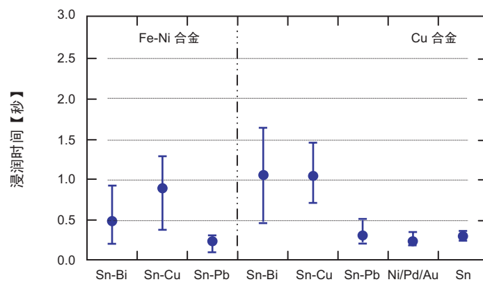
图 4-2 浸润时间测定结果（Sn-37Pb 焊浴）
