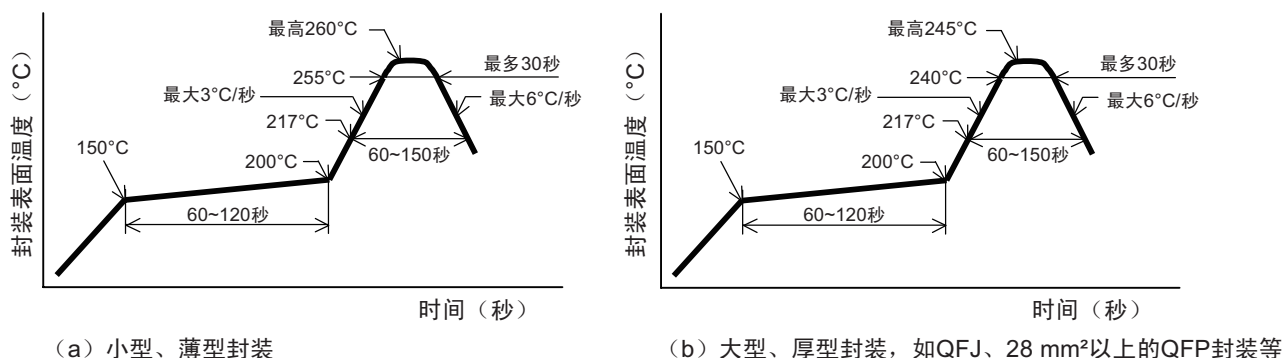
图 4-12 IPC/JEDEC 标准的回流耐热温度曲线
