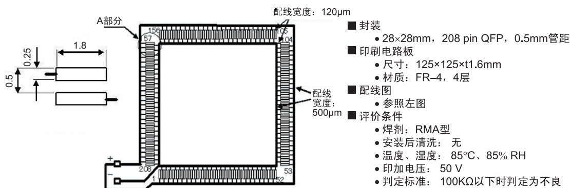
图 6-17 离子迁移评价电路板
