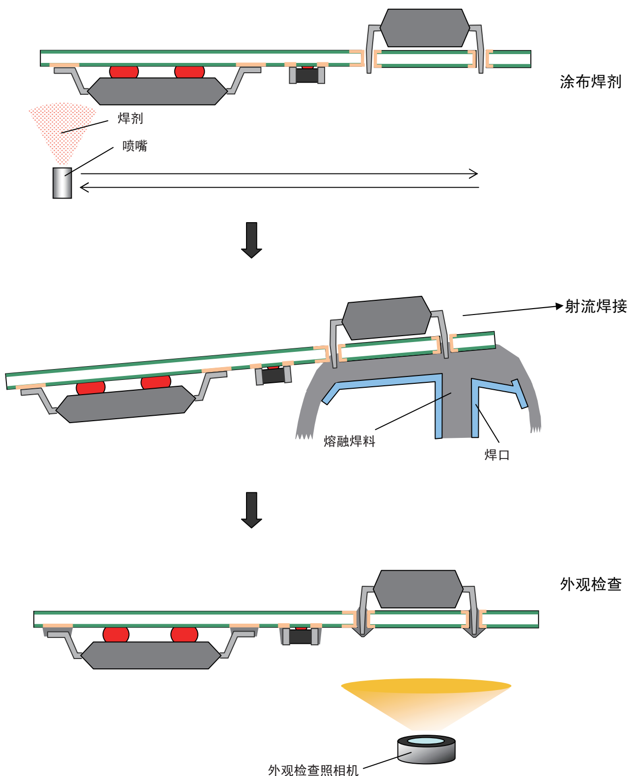
图 1-18 THD/引脚式 SMD 的射流焊接示意图
