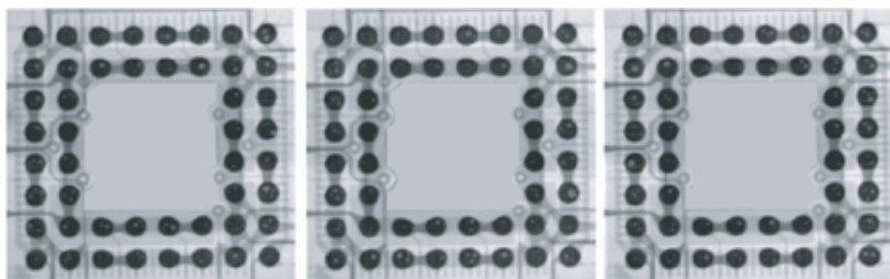
图 5-27 X 线外观（对策后 1）
