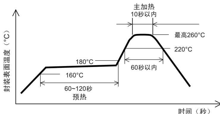
图 4-18 红外回流温度曲线 (IR60)
