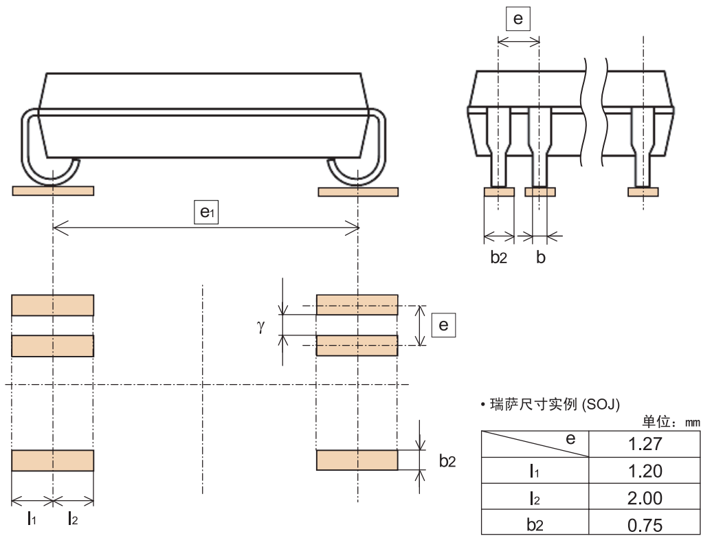
图 2-7 SOJ 实例
