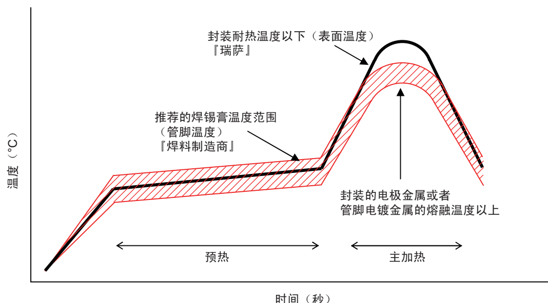
图 4-20 焊接温度
