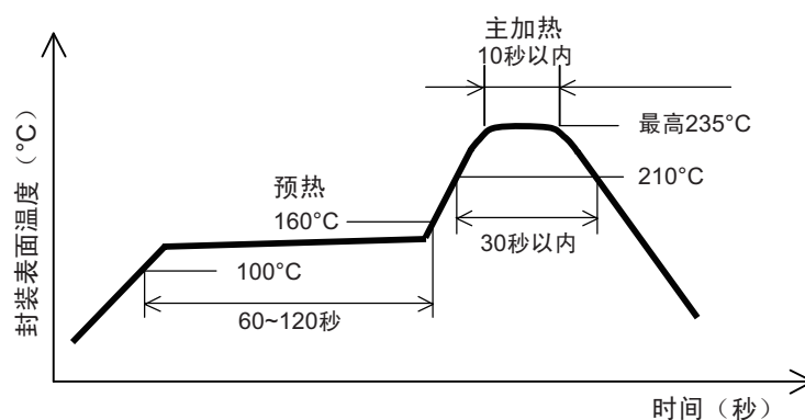
图 4-16 红外回流温度曲线 (IR35)
