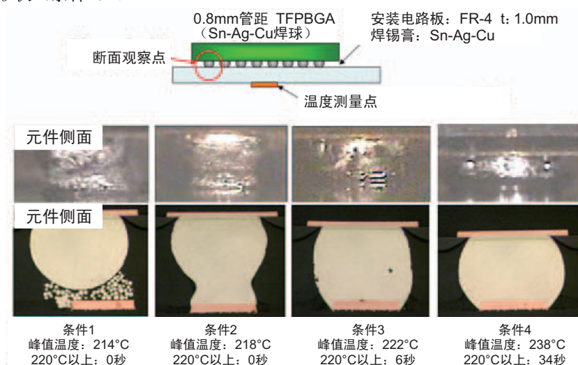
图 5-10 加热条件和焊点状态
