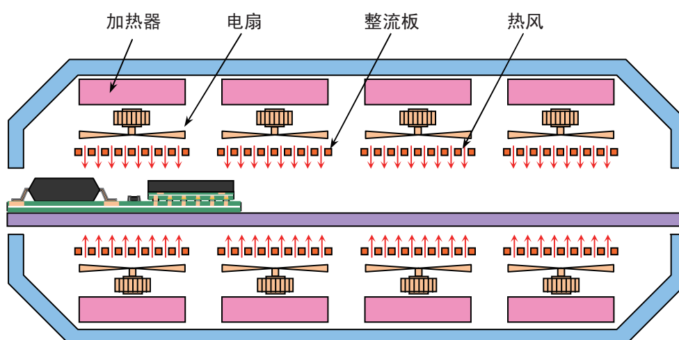
图 1-10 热风法（例）
