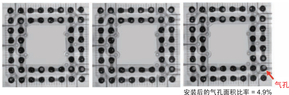
图 5-26 X 线外观（对策前）
